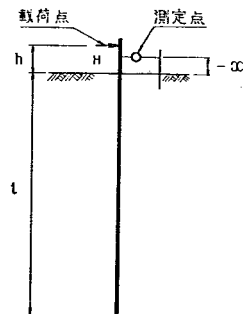
図-3.35 ぐいの変位
