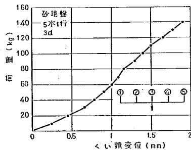
図-4.19 載荷試験結果 (5本1行, 3d, 砂地盤)
