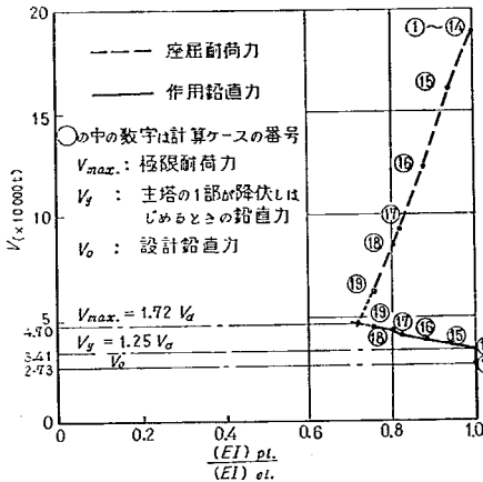
図-5.13 主塔の極限耐荷力
