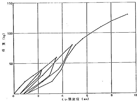
図4.15 載荷試験結果 (単い、砂地盤)
