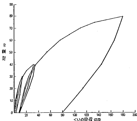
図-6.56 荷重-変位曲線 (No.1, No.3の平均値)
