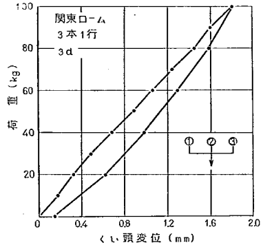
図-4.23 載荷試験結果 (3本1行, 3d, 閉東ローム)
