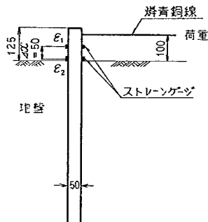
図-4.28 くいの応力度の測定
