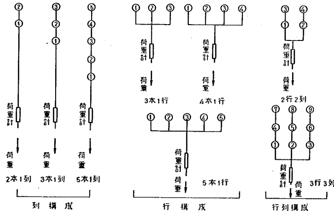
図-4.14 試験のくい構成
