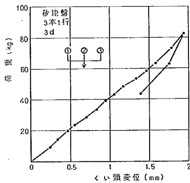
図-4.17 載荷試験結果 (3本1行, 3d, 砂地盤)
