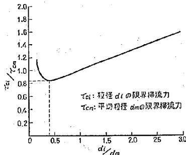
図-3.8 Egiazaroffによる混合粒径の限界掃流力
