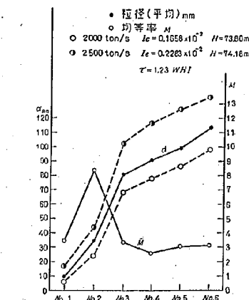
図-3.11 天竜川(44.5km)湾曲部横断方向
