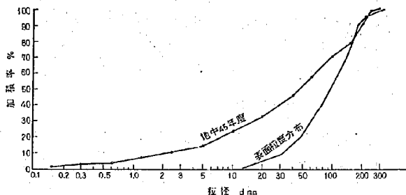
図-3.6 天竜川44km 地点表面と地中の粒徑分布
