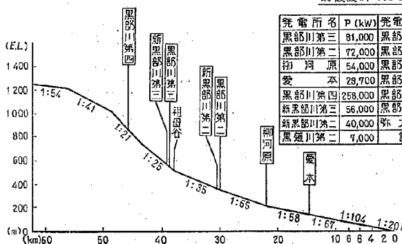
図-3.19 黒部川縦断面図
