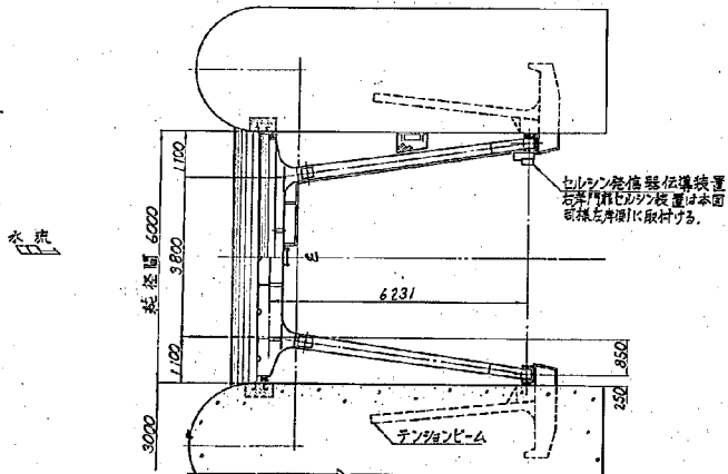
扉体平面图
