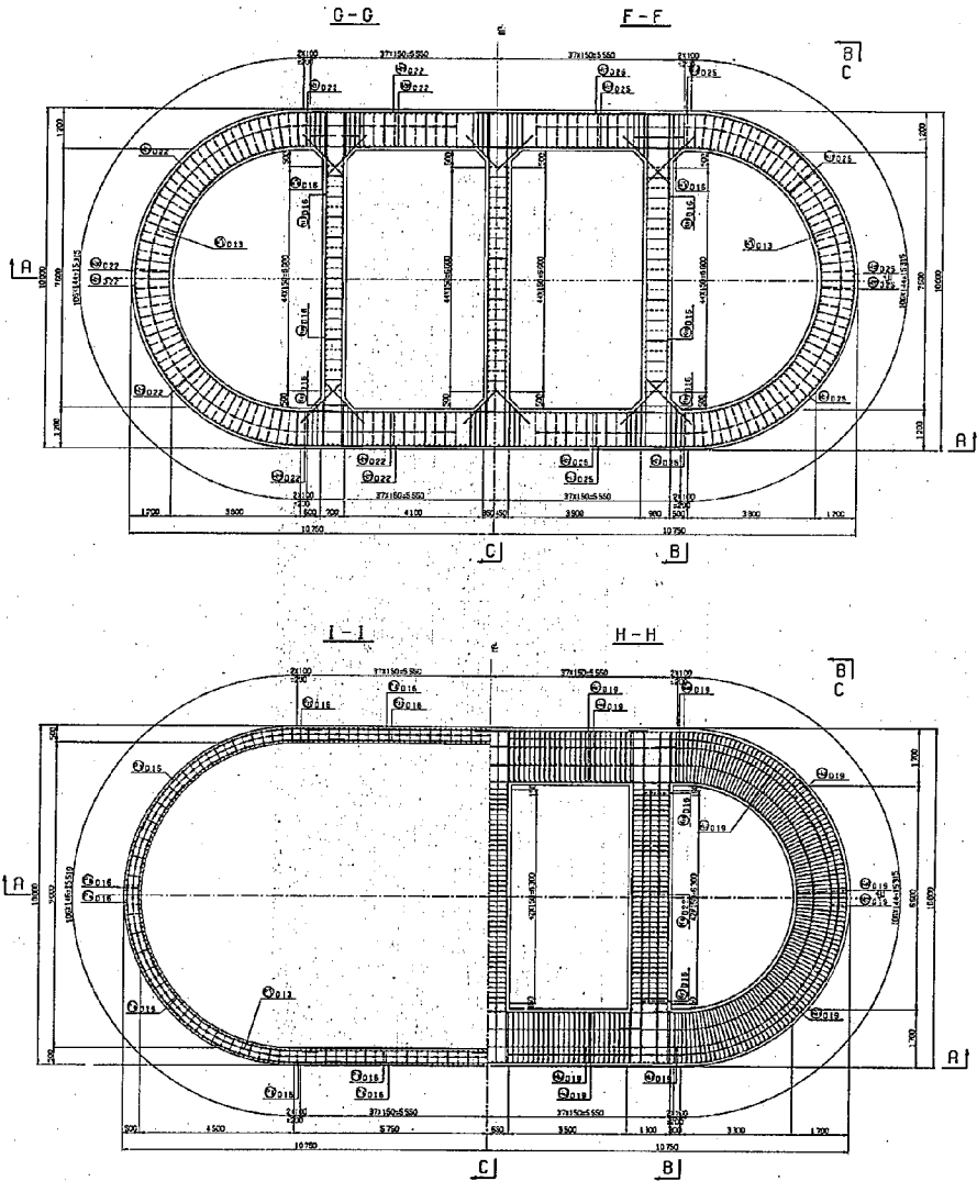
図-72 自動設計プログラムによる図化例(側壁頂版受部, 胸壁平面配筋図)
