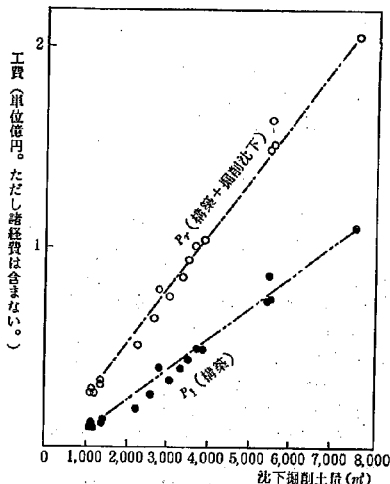
図-1 沈下掘削土量と工費
