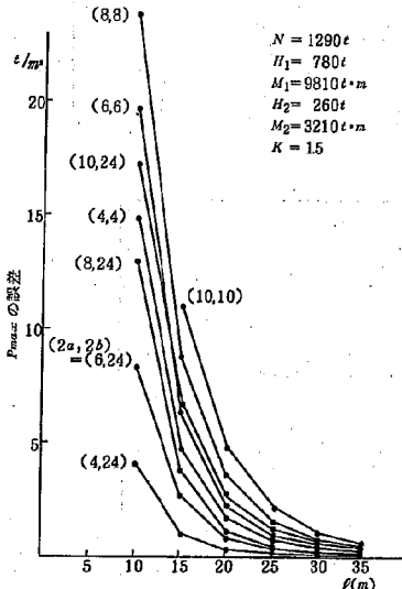
図-43 誤差とケーソン長さとの関係(2)
