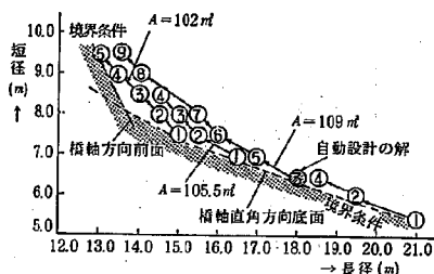
図-13 ① SS 最大によるランクづけ (設計例-2)
