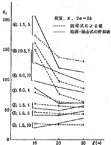
図-49 池原・横山式と回帰式による値の比較 ( q_1 )
