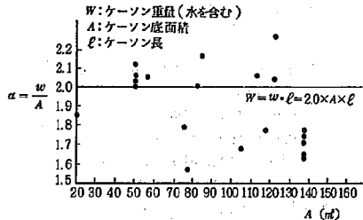
図-36 ケーソンの換算単位体積重量 \alpha
