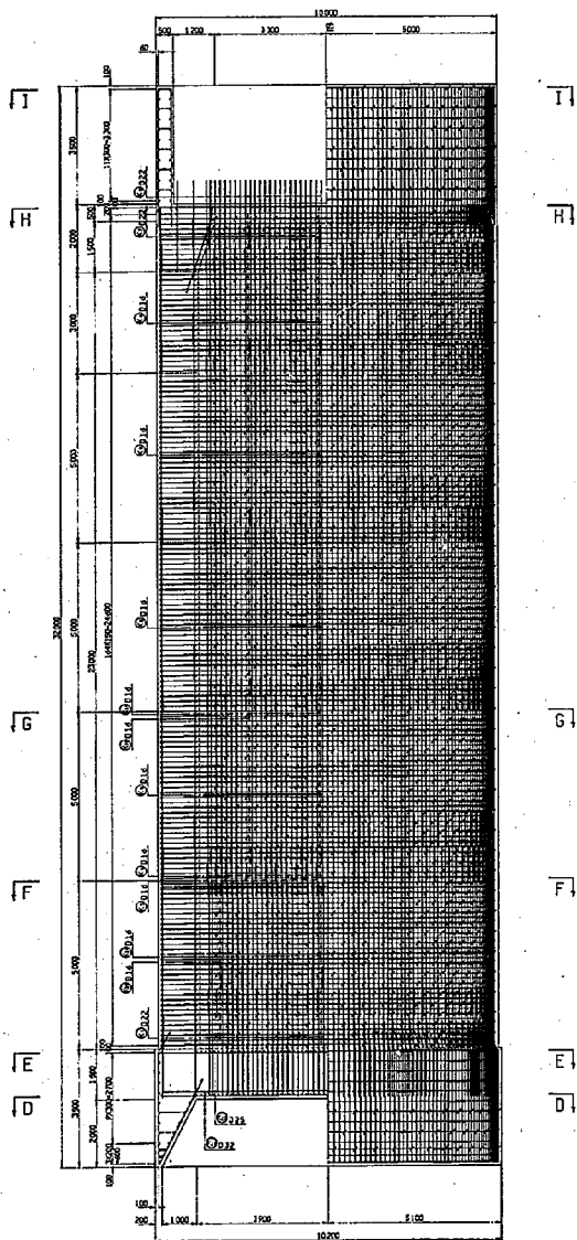
図-71-2 自動設計プログラムによる図化例(側面図, 隔壁展開図)
