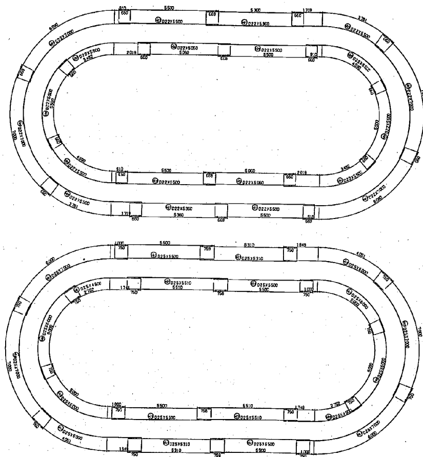
図-74-1 自動設計プログラムによる図化例（鉄筋加工図）
