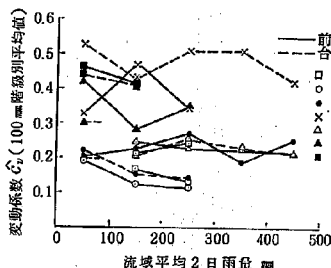
図-13 2日雨量と変動係数 8),9)
