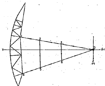
図-13 Bゲート脚柱の格点番号
