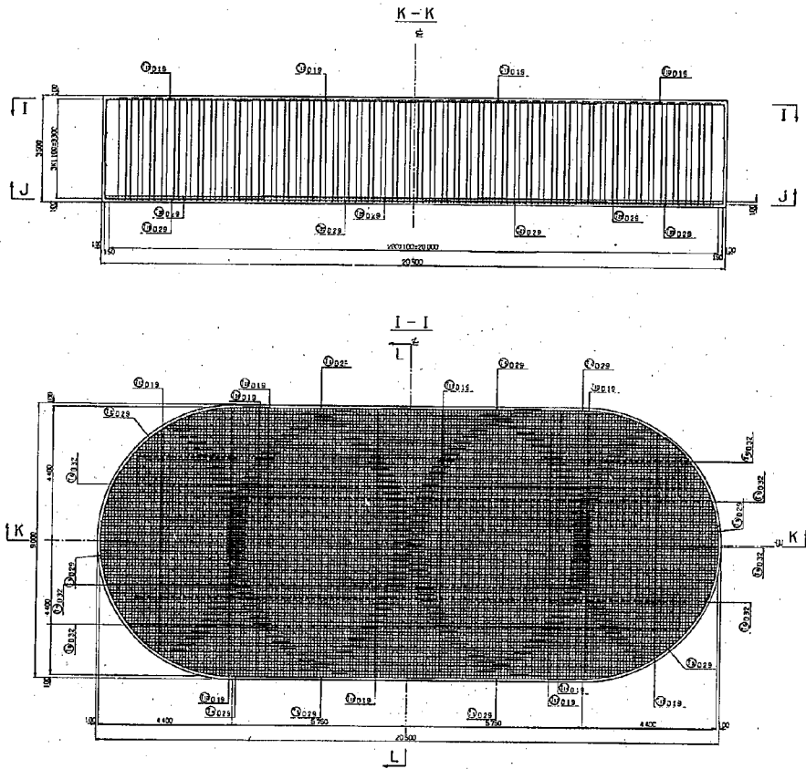
図-75-1 自動設計プログラムによる図化例 (頂版配筋図)
