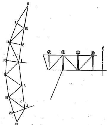
図-20 Dゲート主桁間縦トラスの格点番号
