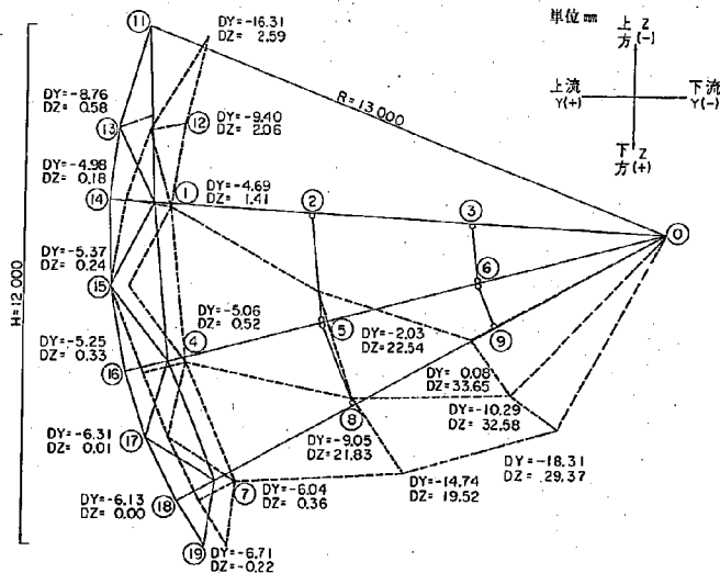
図7-1-1 Aゲート脚柱たわみ図
