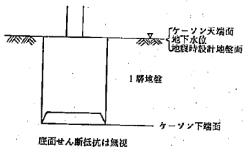
図-51 設計条件
