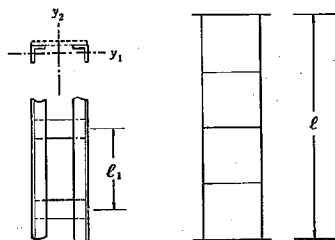
図-5 ラチス柱
