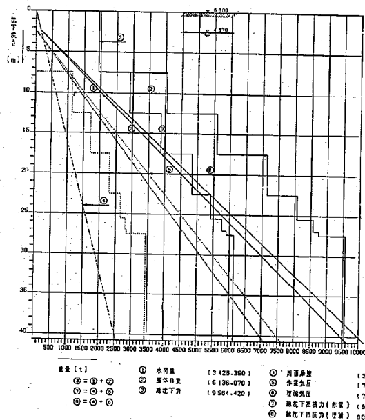
図-69 自動設計プログラムによる図化例 (沈下関係図)
