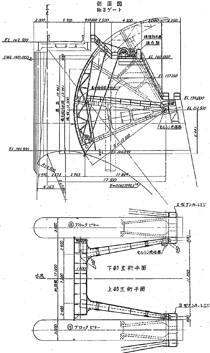
図-17 Dゲート一般図
