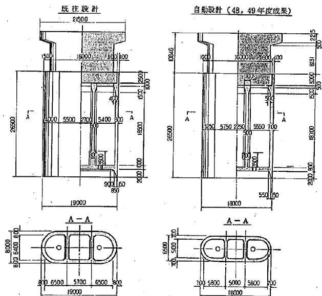
図-63 設計結果の比較 (比較設計例 その2)
