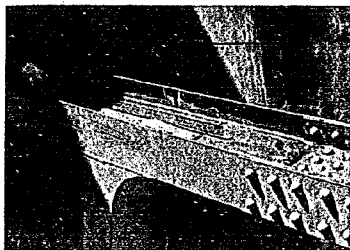
写真3 Cゲート脚柱腹板の変状
