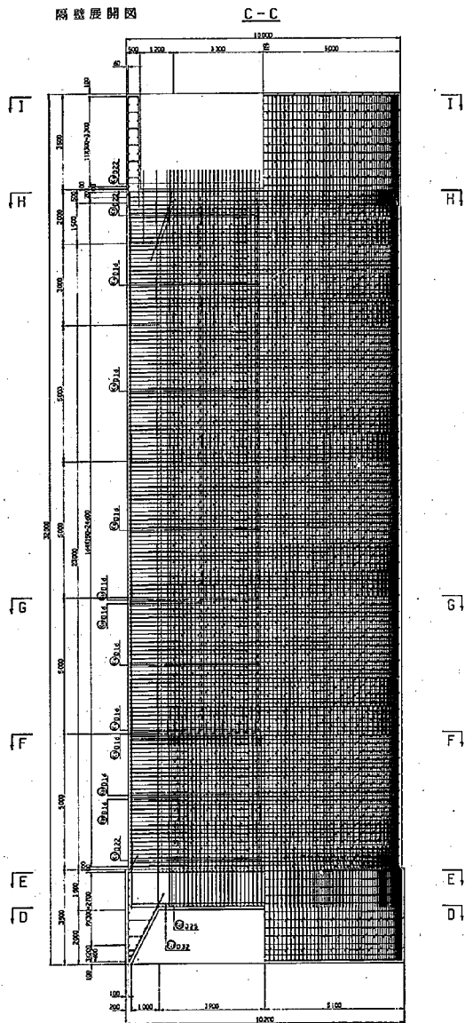
図-71-2 自動設計プログラムによる図化例 (側面図, 隔壁展開図)
