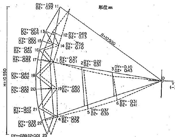
図-12 Bゲート脚柱たわみ図
