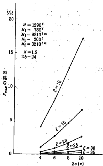
図-39 誤差と側面幅との関係(2)
