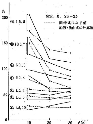
図-49 池原・横山式と回帰式による値の比較 ( q_1 )
