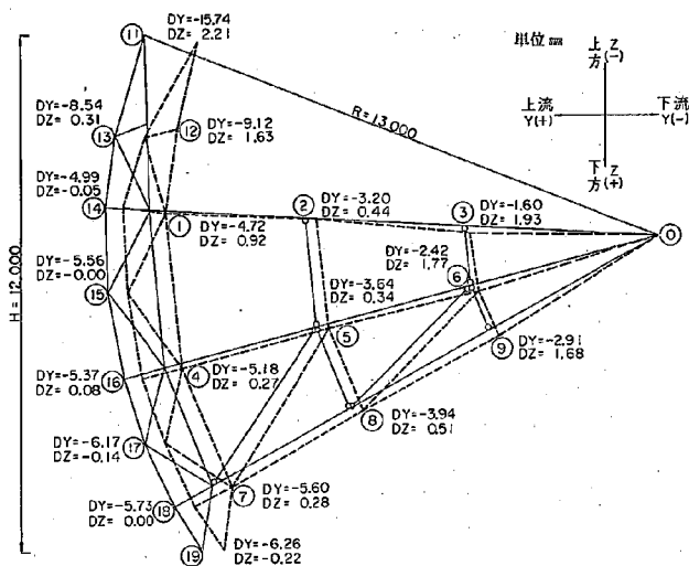
A2Rゲート脚柱たわみ図
