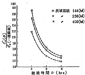
図-10 継続時間による \hat{c}_v の変化(12降雨の平均)
