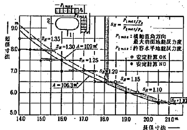
図-9 ケーソン形状と S_H との関係
