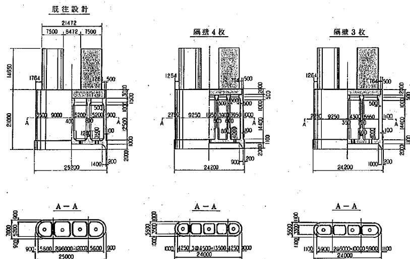
図-67 設計結果の比較 (比較設計例 その6)
