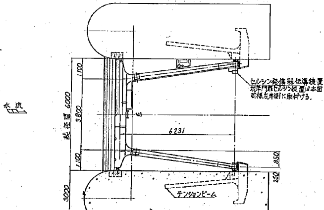
扉体平面图
