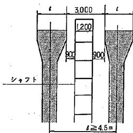
図-27 隔壁間最小間隔と隔壁中心間隔の関係
