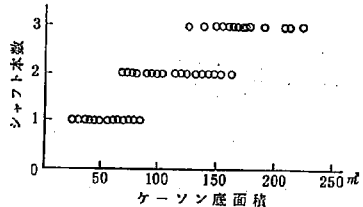
図-31 ケーソン底面積とシャフト本数(施工実績)
