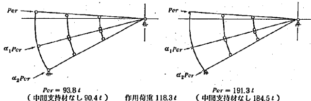
図-1 脚柱先端の条件と座屈荷重
