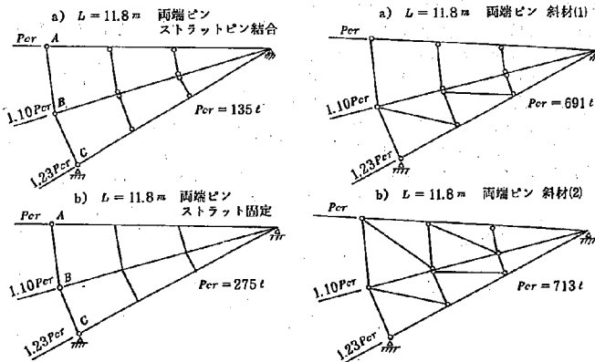
図-2 ストラットの結合方法と座屈荷重
