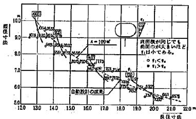
図-4 ケーソン形状と最大底面地盤反力度 (橋軸方向)
