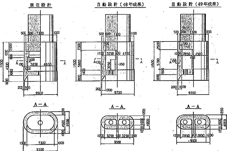
図-65 設計結果の比較（比較設計例 その4）
