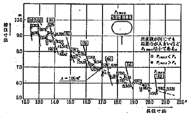
図-6 ケーソン形状と最大前面地盤反力度 (橋軸方向)
