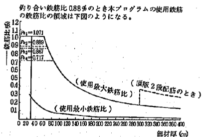
図-23 各部材厚と最大鉄筋比・最小鉄筋比との関係
