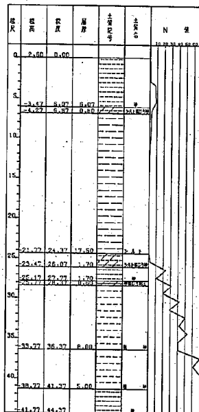
図-69 自動設計プログラムによる図化例 (沈下関係図)
