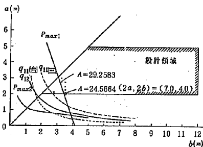
図-52 図式解法の一例
