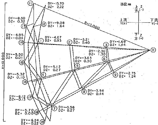
図7-4 Aゲート脚柱たわみ図
