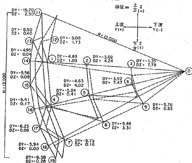
A4Pゲート脚柱たわみ図
