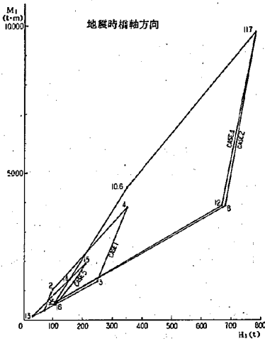
図-35(c) 水平力とモーメントの関係
