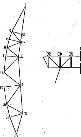
図-14 Bゲート縦トラスの格点番号
