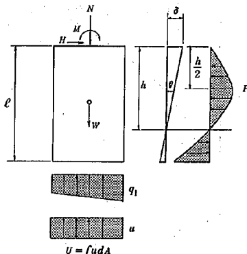
図-16 ケーソンの作用荷重
