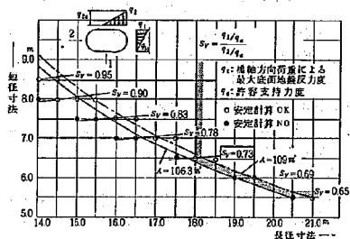
図-8 ケーソン形状と S_V との関係
