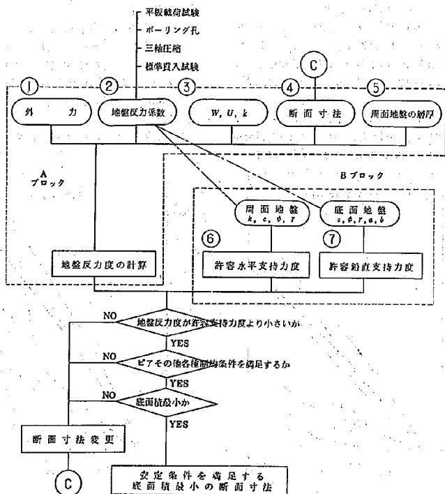
図-34 安定計算における各要因の関係図
