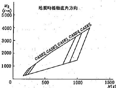
図-35(d) 鉛直力とモーメントの関係
