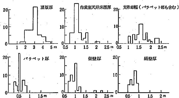
図-20 既往実績部材厚
