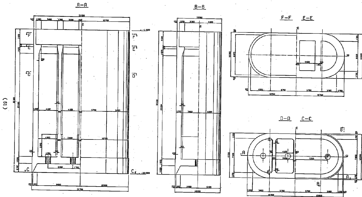
図-68 自動設計による図化例（一般寸法図）
