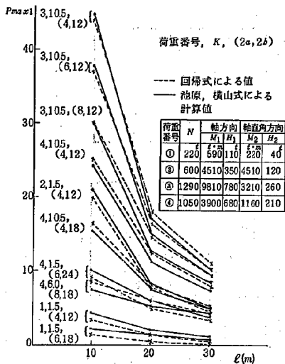
図-44 池原・横山式と回帰式による値の比較 ( P_{max1} )
