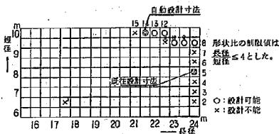
図-54 設計条件 (比較設計例 その1)
