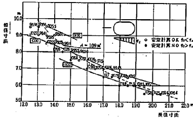
図-5 ケーソン形状と最大底面地盤反力度 (橋軸直角方向)
