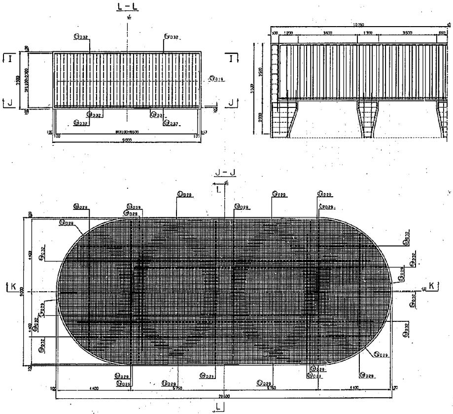
図-75-2 自動設計プログラムによる図化例（頂版配筋図）
