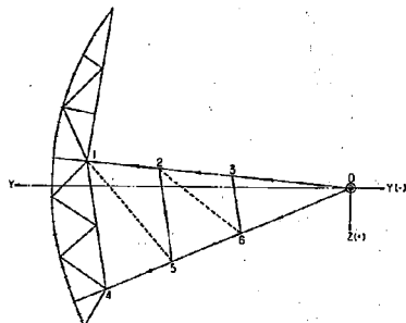
図 19 Dゲート脚柱の格点番号
