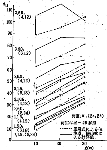
図-47 池原・横山式と回帰式による値の比較 ( q_{12} )
