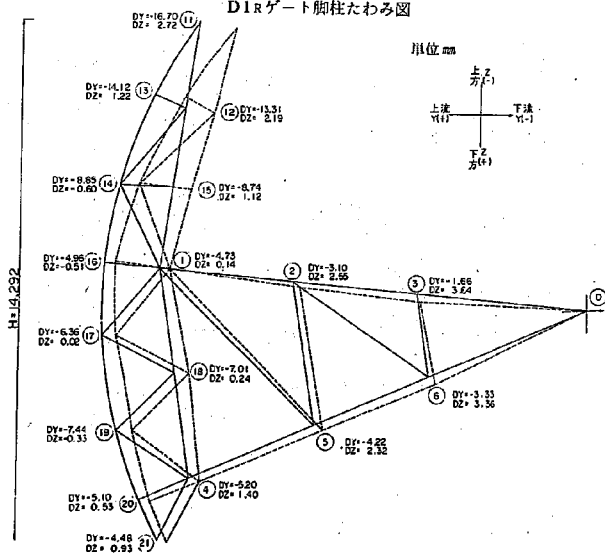
図-18 Dゲート脚柱たわみ図
