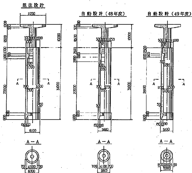
図-66 設計結果の比較 (比較設計例 その5)
