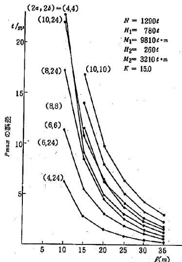
図-42 誤差とケーソン長さとの関係 (1)
