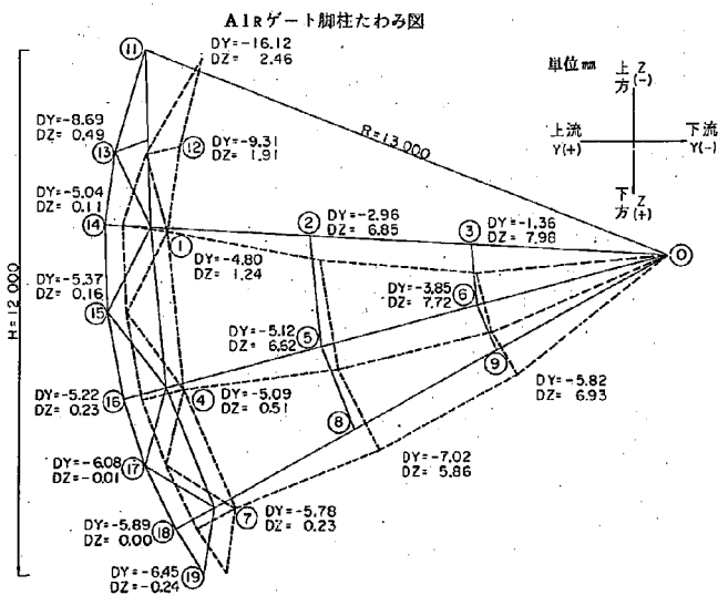
図 7-2 Aゲート脚柱たわみ図
