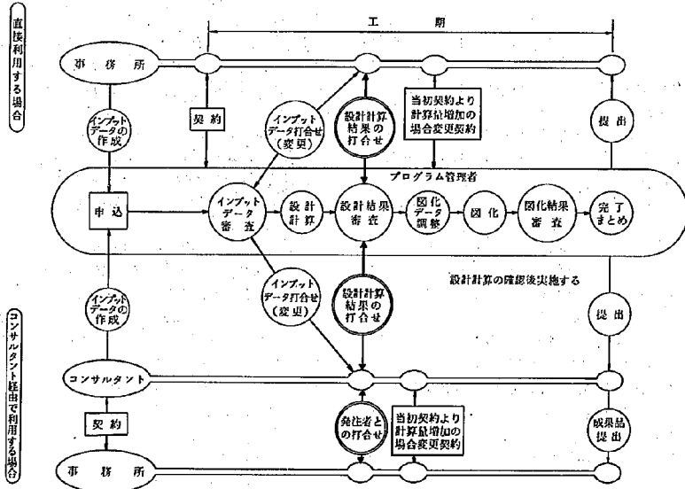
図-53 ケーソン自動設計プログラム利用の流れ
