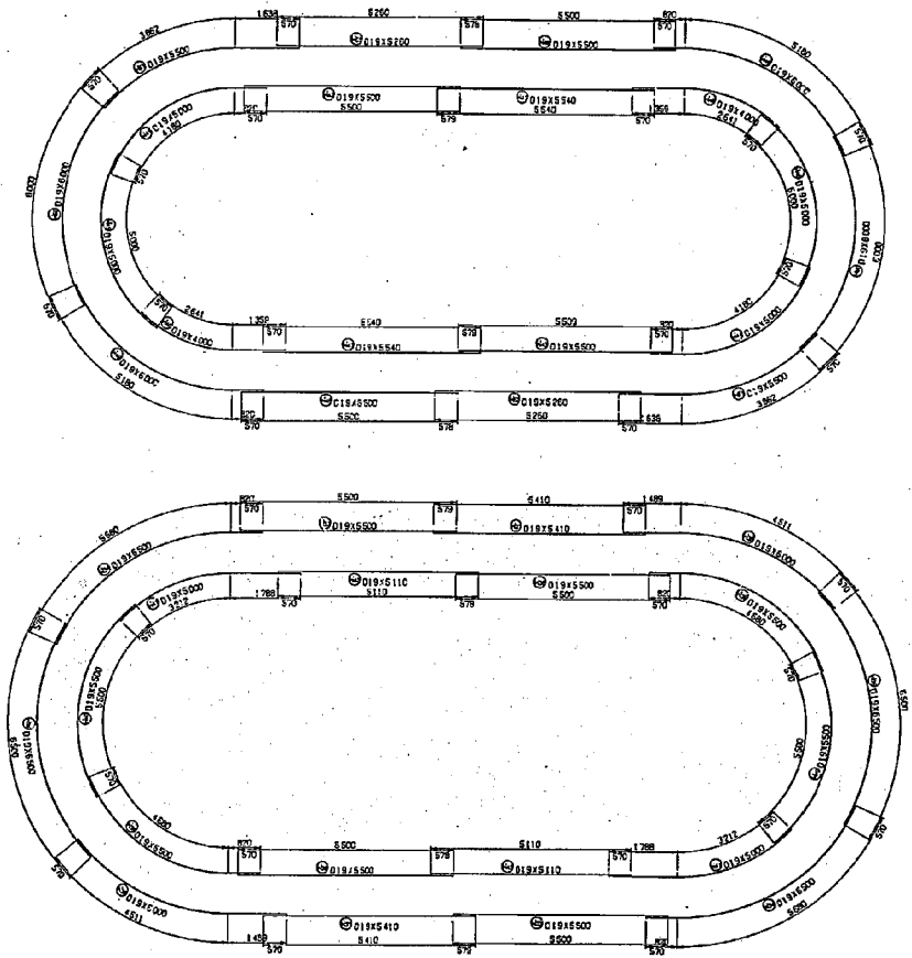
図-74-2 自動設計プログラムによる図化例（鉄筋加工図）
