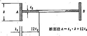
図-4 I 形断面のトラスへの置き換え
