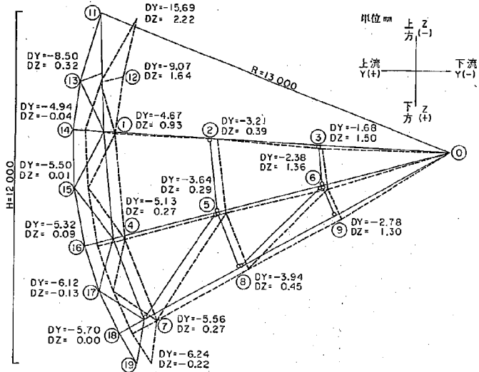
A3Rゲート脚柱たわみ図
