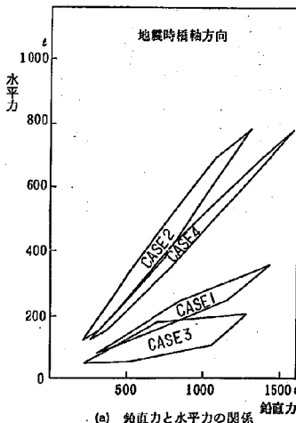
図-35 ケーソン天端に作用する外力の定式化
