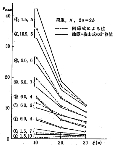
図-48 池原・横山式と回帰式による値の比較 ( P_{max} )
