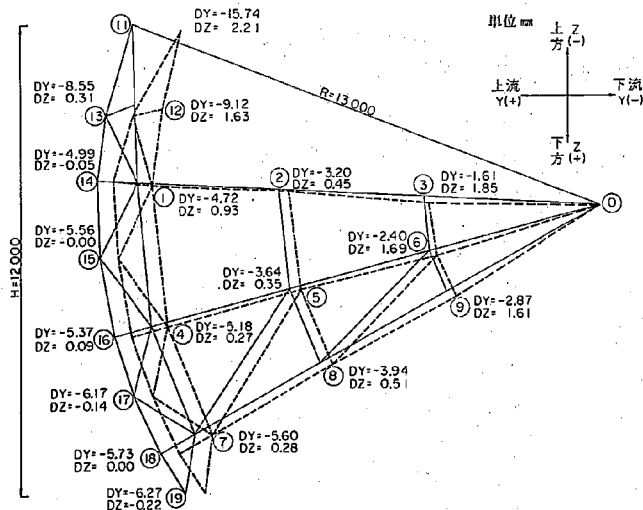
A2Fゲート脚柱たわみ図
