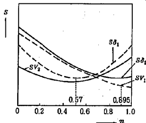
図-19 安全率 S とケーソン形状比 n との関係
