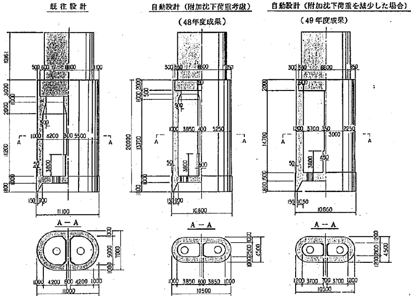
図-64 設計結果の比較（比較設計例 その3）
