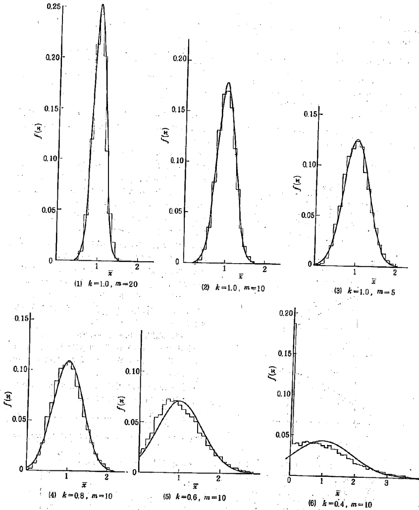
図-6 モデル降雨によるシミュレーションの結果(頻度分布)
