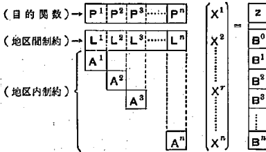
図-7 (31)式の行列表示
