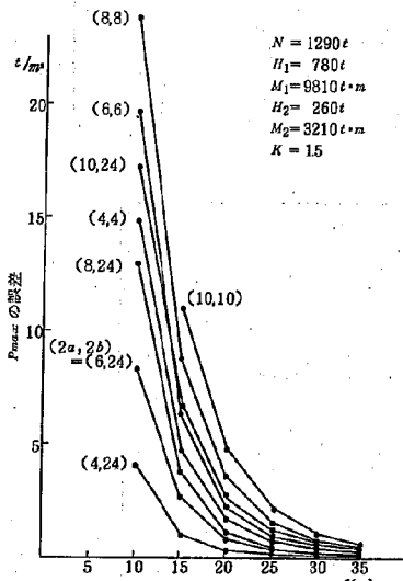
図-43 誤差とケーソン長さとの関係 (2)
