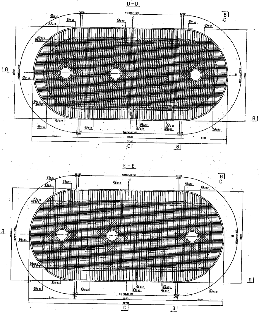
図-73 自動設計プログラムによる図化例（頂版配筋図）
