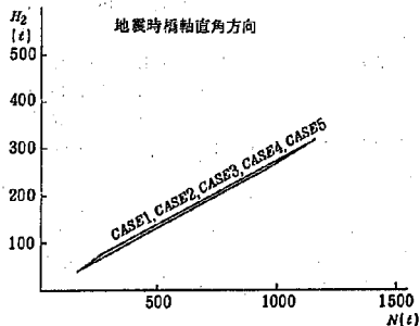
図-35(e) 鉛直力と水平力の関係
