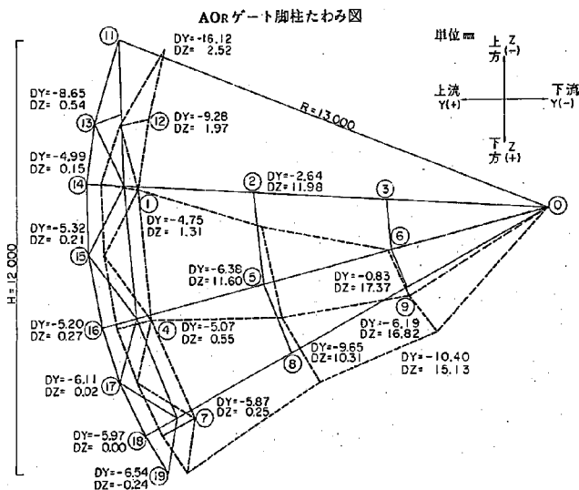
図 7-1-2 Aゲート脚柱たわみ図
