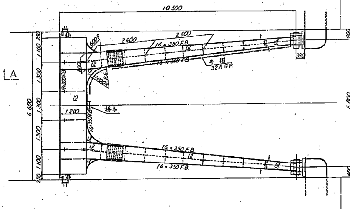
図-11 Bゲート一般図
