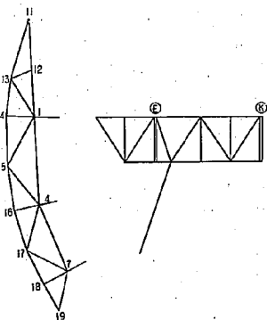
図-10 Aゲート縦トラスの格点番号
