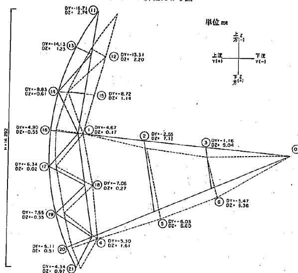
D1Rゲート脚柱たわみ図
