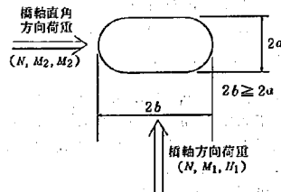
図-37 作用する荷重
