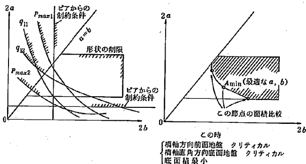
図-50 回帰式を用いた図式解法
