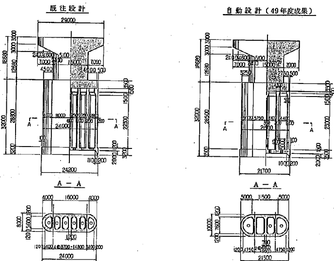
図-62 設計結果の比較 (比較設計例 その1)
