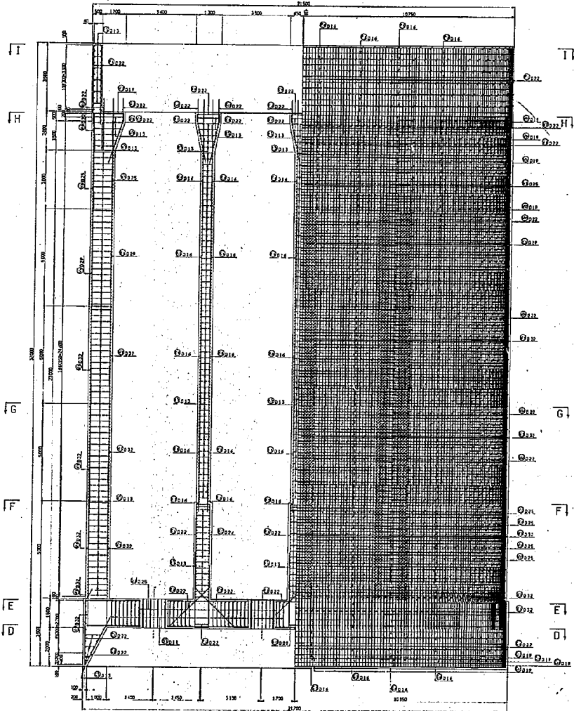
図-70 自動設計プログラムによる図化例（正面配筋図）
