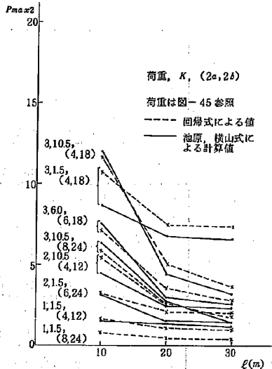
図-46 池原・横山式と回帰式による値の比較 ( P_{max2} )
