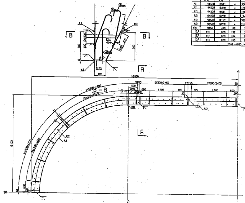
図-76 自動設計プログラムによる図化例 (刃口金物図)
