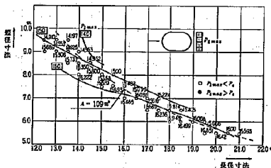
図-7 ケーソン形状と最大前面地盤反力度 (橋軸直角方向)
