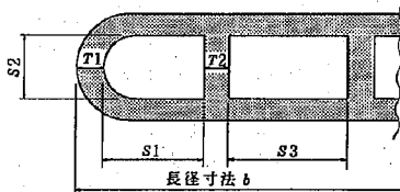
図-29 小判形の隔壁の位置
