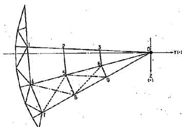
図-8 Aゲート脚柱の格点番号
