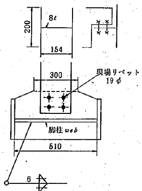
図-9 中間支持材の取付け
