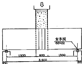
図-3.15 載荷方法
