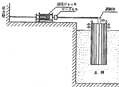
図-4.28 水平載荷試験例
