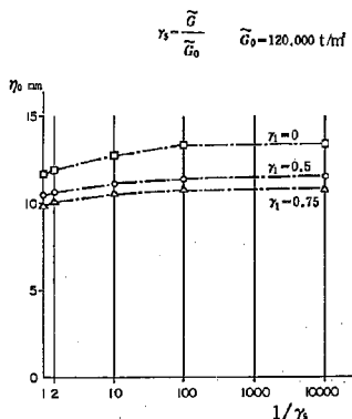
図-4.17 パラメータ \gamma_5 による影響
