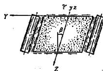
図-5.6 内部土のせん断抵抗
