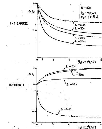
図-6.13 (3) 頂版の変位 (ケースG)
