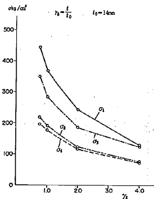
図-4.13 パラメータ \gamma_8 による影響
