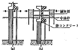
図-3.1 頂版構造 (群ぐい式)
