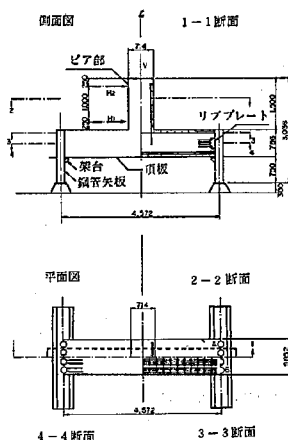
図-3.12 ラーメン型模型体
