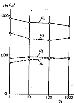
図-4.11 パラメータ \gamma_6 による影響
