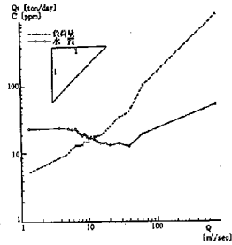
図-41 \text{KMnO}_4 消費量; Q_s , C \sim Q の関係 (河川④)
