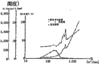
図-28 流量の発生頻度、平均水質・負荷量 (河川① KMnO 4 消費量)
