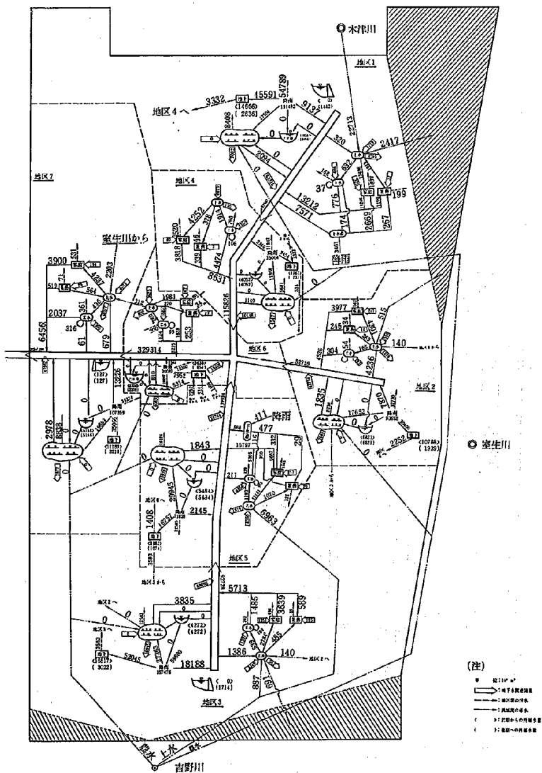
図-22(b) 大和川流域奈良盆地水利模式図 〔昭和47・9・15～昭和48・6・14 (非カンガイ期)〕
