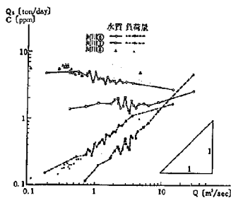
図-49 ケルゲール素; Q_s , C\sim Q の関係 (河川⑥～⑧)
