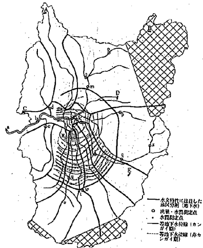
図-15(b) 水文図その2(等地下水水位線/カンガイ期・非カンガイ期)
