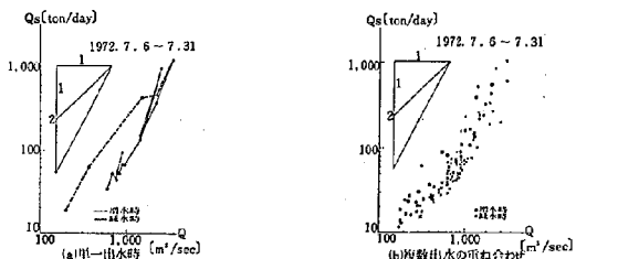
図-7 河川①のKMnO消費量・負荷量の出水時の特性
