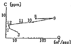
付図一19 河川④のDOの月変化
