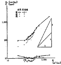
図-39 \text{KMnO}_4 消費量; Q_s , C \sim Q の関係 (河川④)
