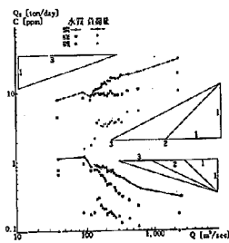
図-42 \text{NH}_4\text{-N} ; Q_s , C \sim Q の関係 (河川①)
