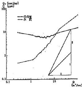
図-40 \text{KMnO}_4 消費量; Q_s , C \sim Q の関係 (河川②)
