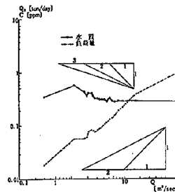
図-43 \text{NH}_4\text{-N} ; Q_s , C \sim Q の関係 (河川②)
