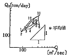
付図一16 (b) 河川④のECの月変化 (その2)
