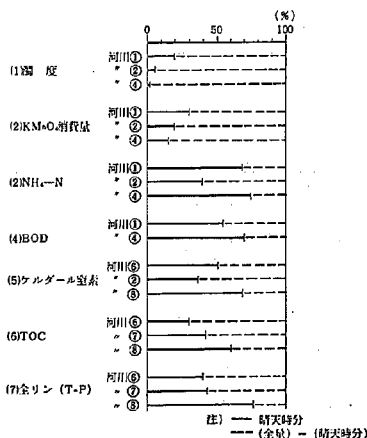
(a) 低水流量以下の流量における負荷量の平均値を晴天時分とした場合(ケース1)
