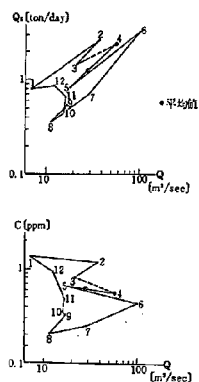
付図—10 河川⑩のHN 2 Nの月変化
