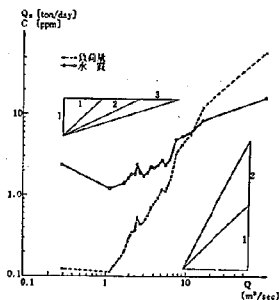
図-37 濁度; Q_s , C \sim Q の関係 (河川②)
