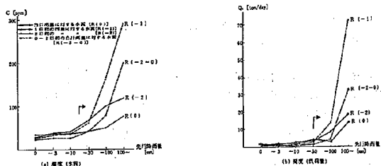
図-23 河川①における降雨に対する濁度の応答
