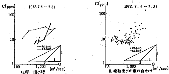
図-8 河川①のKMnO消費量・水質の出水時の特性
