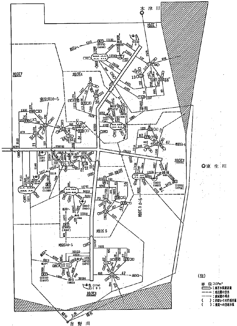
図-22(a) 大和川流域奈良盆地水利用模式図 (昭和47・6・15~昭和47・9・15(カンガイ期))
