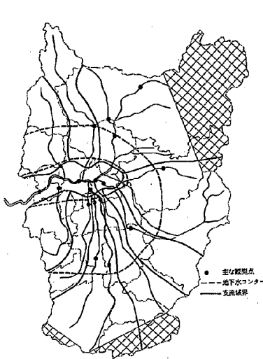
図-16(a) 水文特性に着目した地区分割
