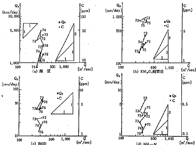
図-22 (a)~(d) 河川①の濁度・KMnO 4 消費量・BOD・NH 4 -Nの経年変化(平均値)
