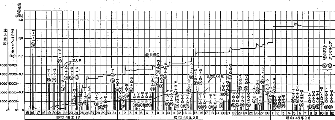
図-3.3.6 C-gam 注入と地表浮き上り
