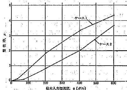
図-2.42 加速度と塑性率との関係 ( H=7\text{m} )
