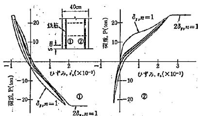
図-2-14 軸方向鉄筋のひずみ (供試体 C, \delta_y 載荷時)
