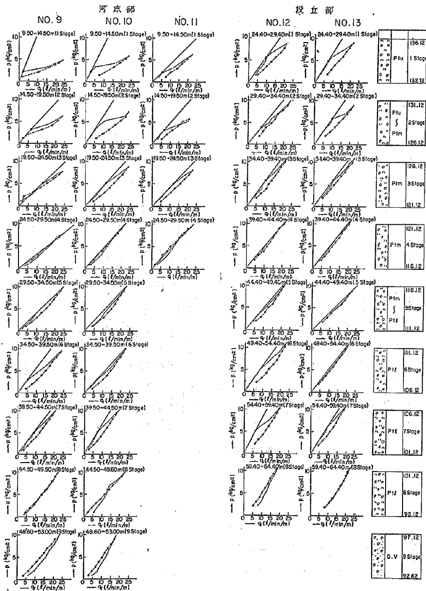
図-3-5.6 Eダム PI 層の p - q 曲線
