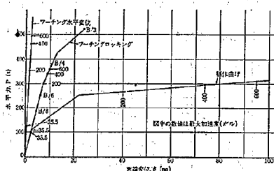
図-2.41(a) 水平力と天端変位との関係 ( H=7\text{m} , ケース 1, フーチング: 8 \times 9\text{m} )
