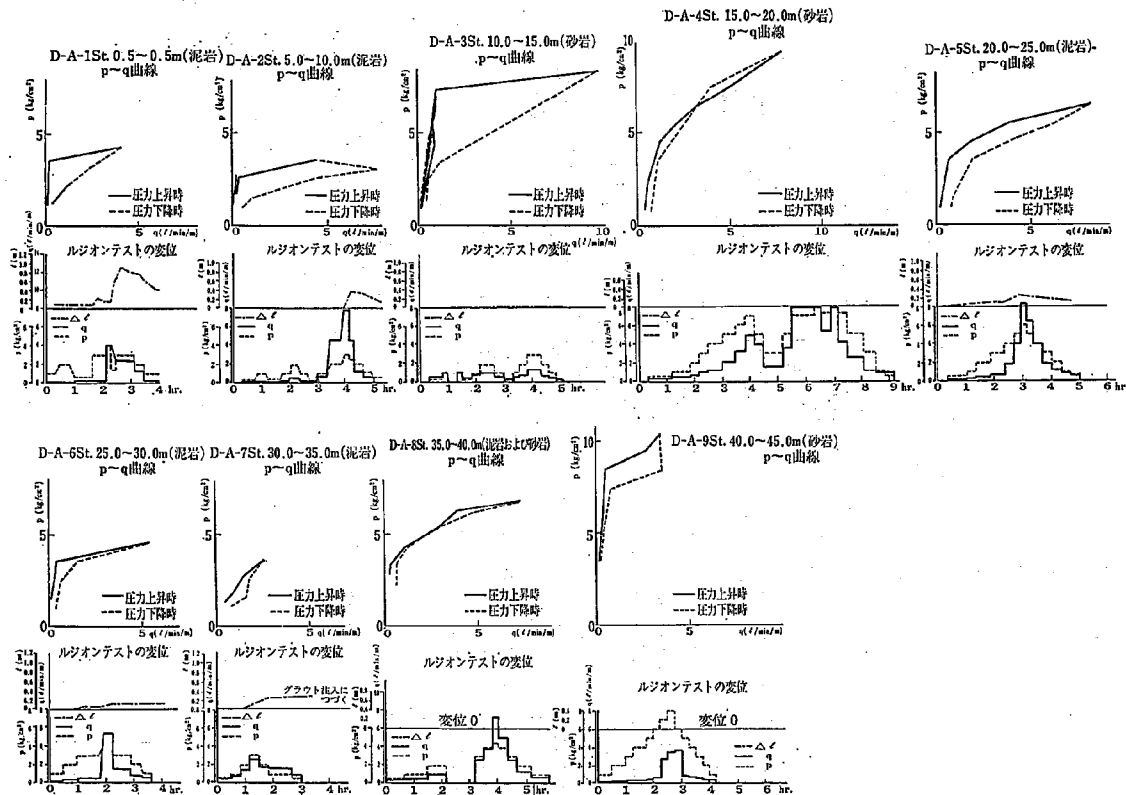
図-3.1.6 A・B・C 各地帯の p-q 曲線および変位量
