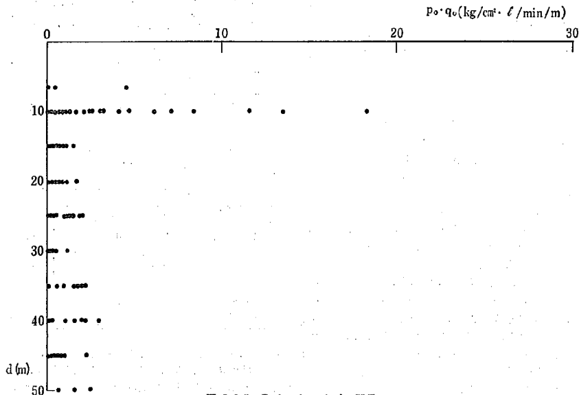
図-3.2.5 Bダム p_0 q_0 と d の関係
