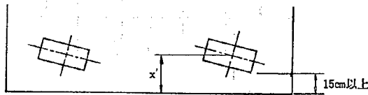
図-1.7.4 斜角筋の巻の配置
