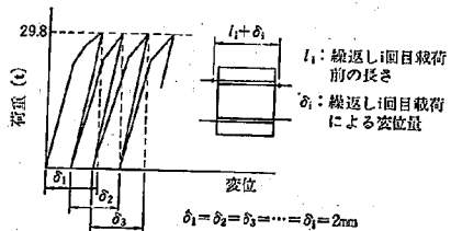
図-3.17 変位制御による荷重の履歴〔シリーズ (II-1)〕
