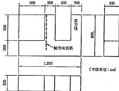
図-3.35 供試体の形状寸法 (シリーズB)
