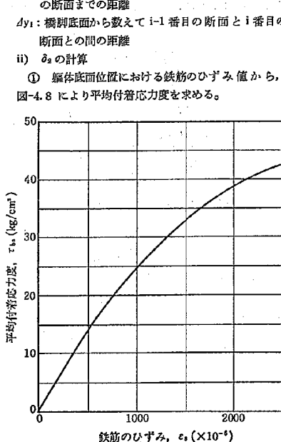
図-4.8 平均付着応力度
