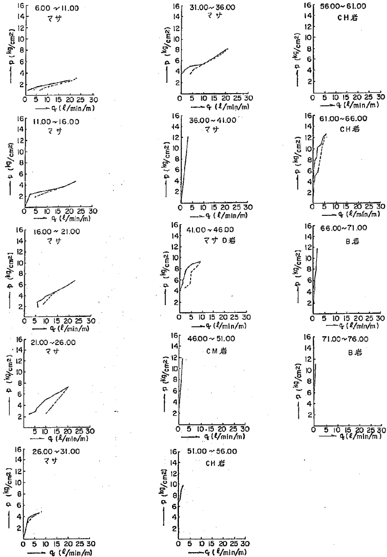
図-3.8.3 H 2 M p~q 曲線
