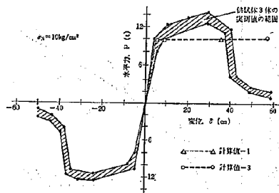
図-2.23 西山らの実験 10, 60) における p- \theta 曲線の包絡線
