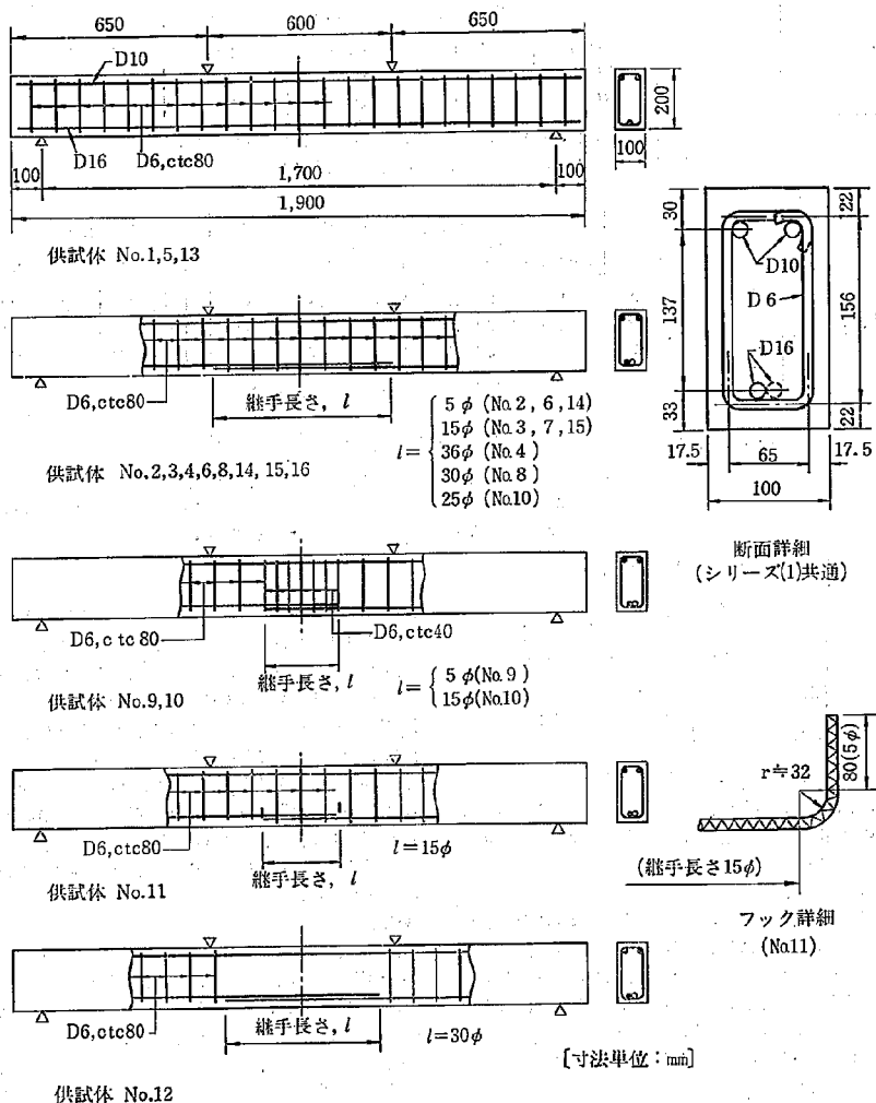
図-3.1 供試体の構造概要〔シリーズ(I-I)〕
