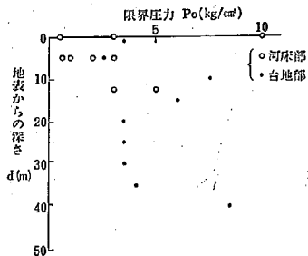
図-3.1.8 Aダム p_0 と d の関係
