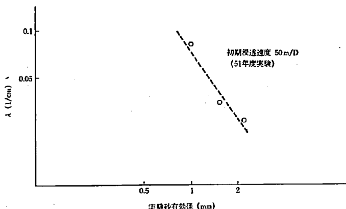
図-31 実験砂有効径と \lambda
