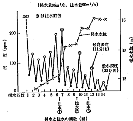
図-46 妻沼での再揚水時の注入の効果 11) (濁度と再揚水時水位) (水井・村下原因)
