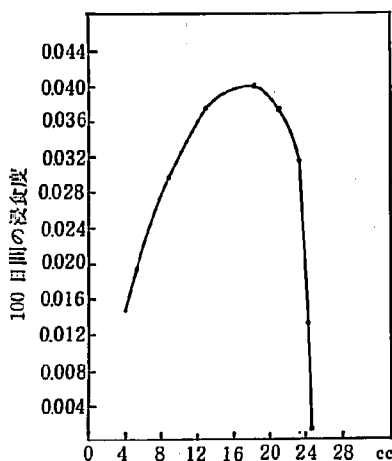
図-15 鉄鋼の腐食に及ぼす水中の溶解鉄量の影響 (清水他原図) (10)
