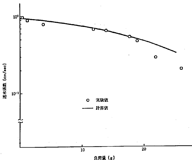
図-29 全層での透水系数の変化、実験値との比較
