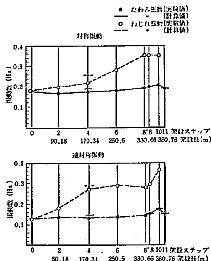
図-16 架設時固有振動数の変化 (1)
