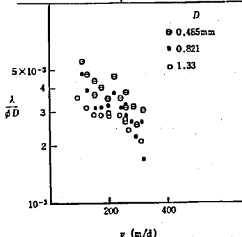
図-32 透過速度 ( q ) と \lambda/qD (藤田原因 13) ) ここに、 D はろ過砂の平均径 \phi は形状係数
