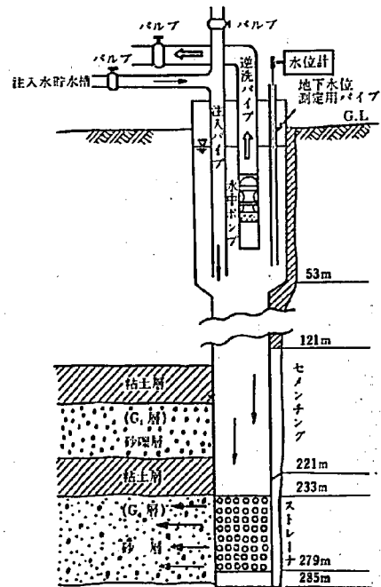
図-8 注入井の構造例図 10)
