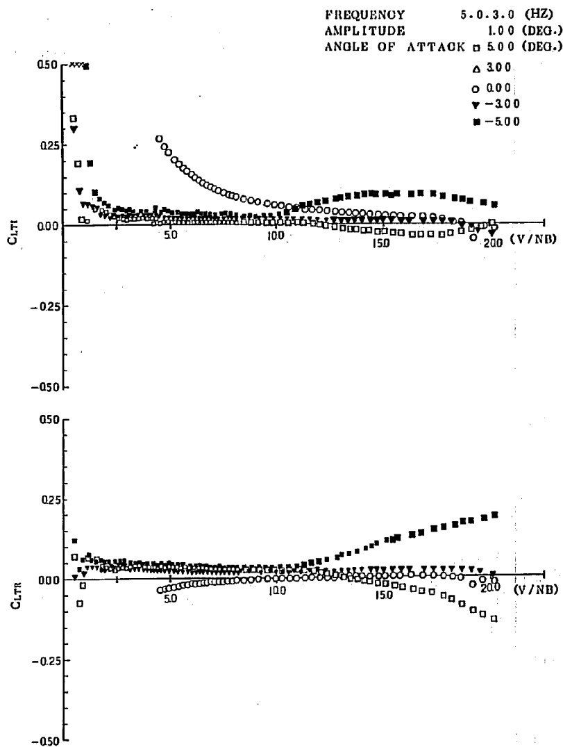
図-21.2 非定常空気力係数 C_{LRT} , C_{LRI} (第1案)
