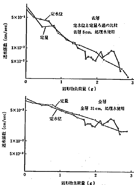
図-33 定量浸透と定水位浸透における透水係数の変化係数 11) (室内実験)
