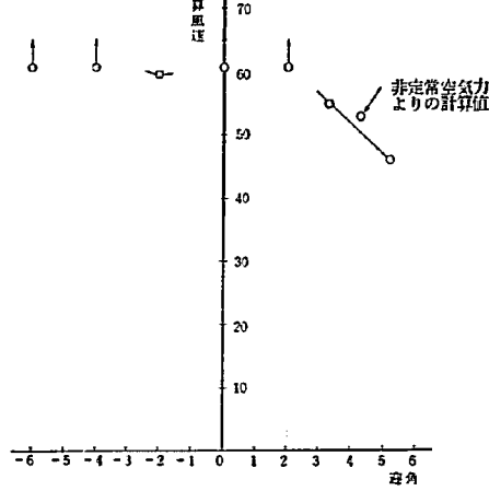
図-25.2 V_{eff} \sim \alpha 曲線 (第Ⅲ案13ステップ)
