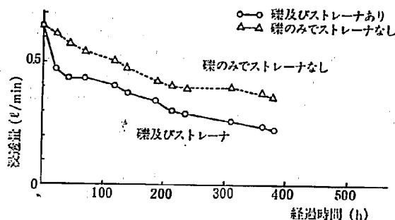
図-16 直カラムによる目詰り実験・流量変動図 (13) (ストレーナの影響) (室内実験)
