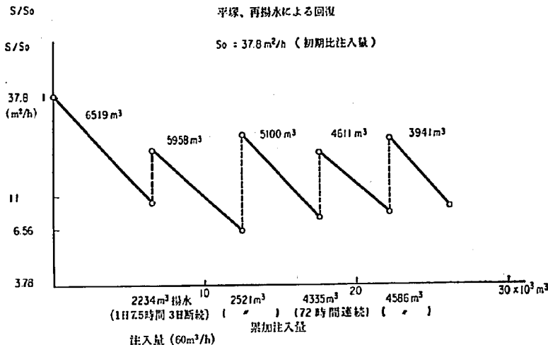
図-44 平塚市における再揚水による比注入量の回復 (注入量の 52%)
