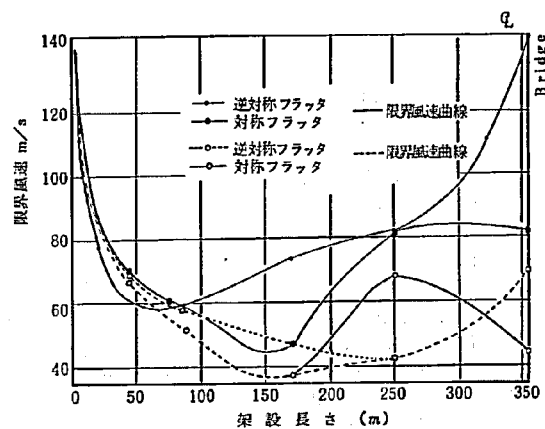
図-13 関門橋架設時フラッタ発生風速 (1)
