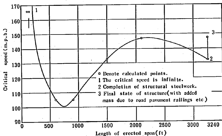
図-5 セミコン橋架設時フラッタ発振風速 1)
