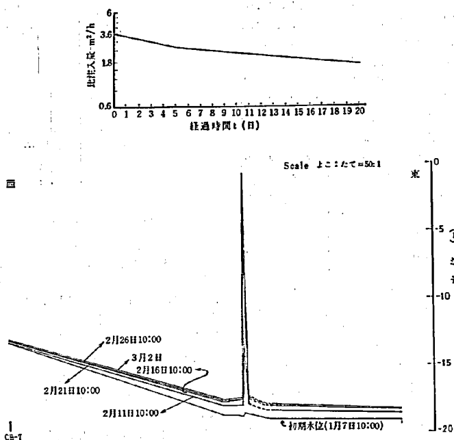
図-11 大阪鶴見区における注入実験での帯水層の水位変化と比注入量
