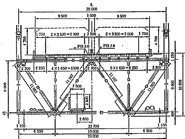
図-15 本州四国連絡橋断面図 (1)
