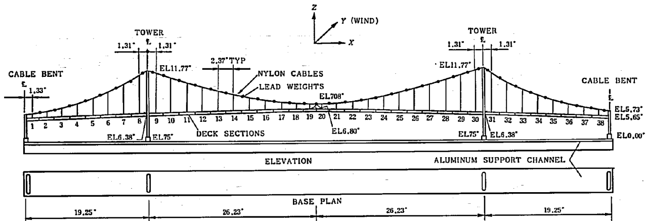
図-6 ナローズ橋模型図 (10)
