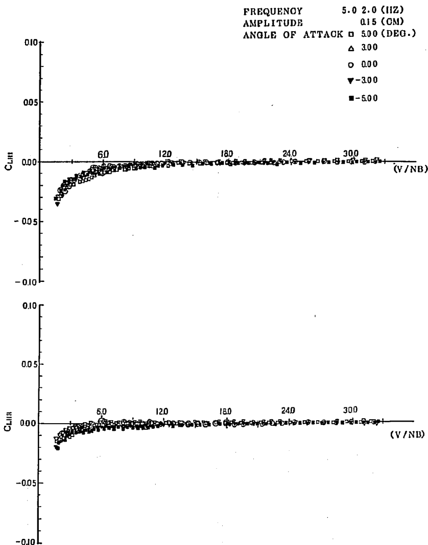
図-27.1 非定常空気力係数 C_{LNF} , C_{LNI} (第1案)
