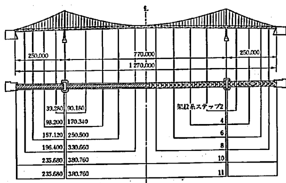
図-14 本州四国連絡橋架設順序 (1)
