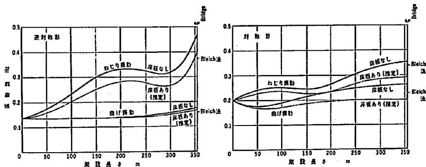
図-12 関門橋架設時固有振動数の変化 (1)
