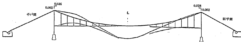
図-22.11 梁橋振動モード図(第11ステップ曲げ対称1次 f=0.3719 Hz)
