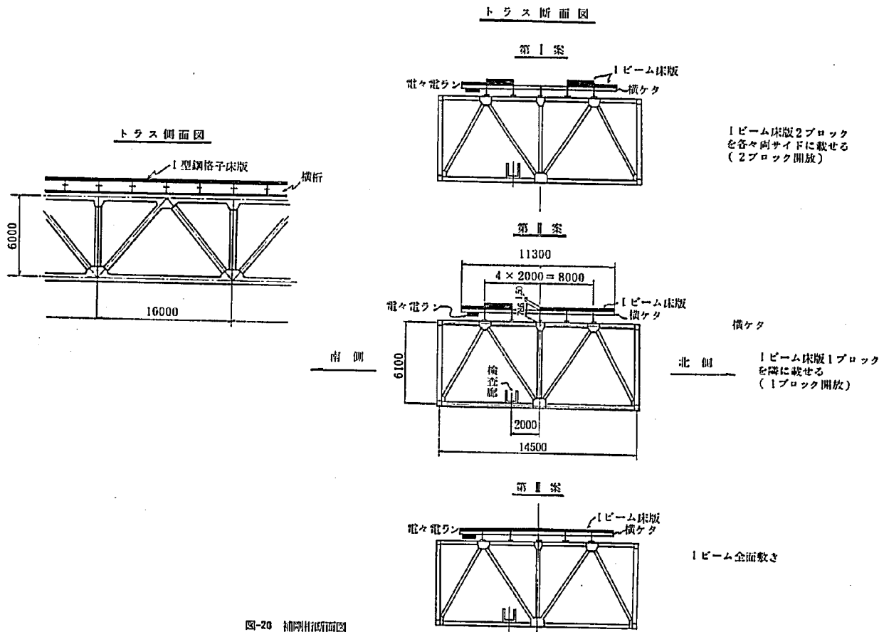
図-20 補剛断面図
