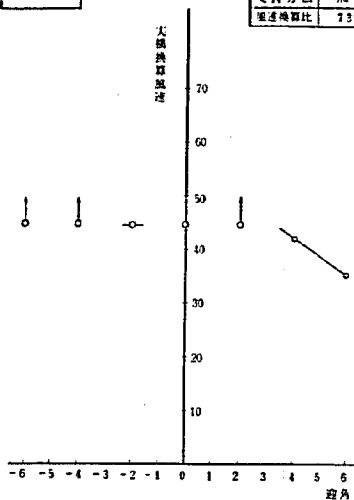
圖-25.4 V_{cr} \sim \alpha 曲線 (第四案 N\alpha/N_T=1.65 )
