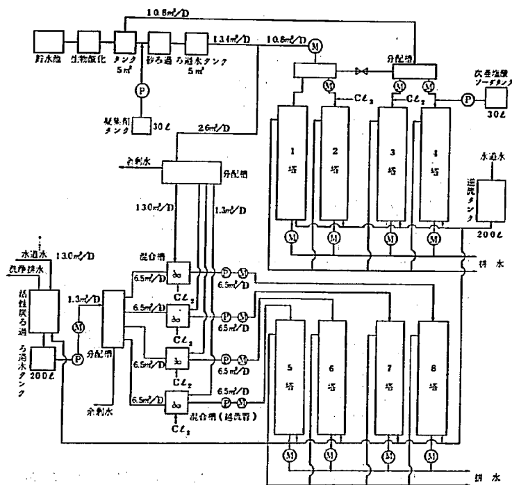
図-20 実験水フローシート
