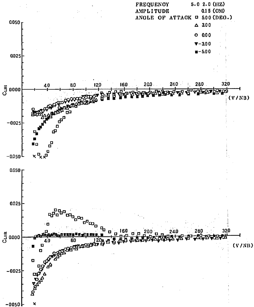
図-21.4 非定常空気力係数 C_{LH1} , C_{LH2} (第Ⅲ案)
