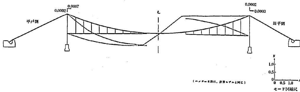
図-22.10 梁橋時振動モード図(第11ステップ曲げ対称1次 f=0.1934 Hz)
