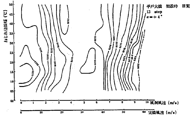
図-26.13 V \sim A \sim \delta 曲線
