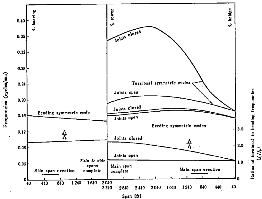
図-4 セミコン橋架設時固有振動数の変化 1)
