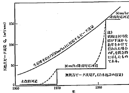
図-36 N地点ピーク流量の経年変化と河川改修による対応
