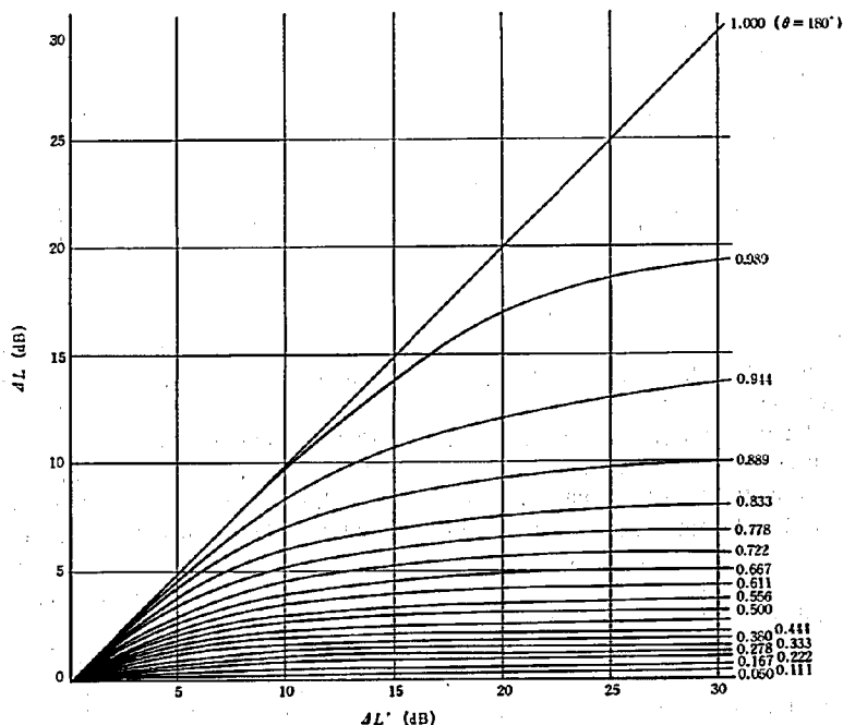
図-4.13 壁による減衰計算図表 (壁の長さによる補正)
