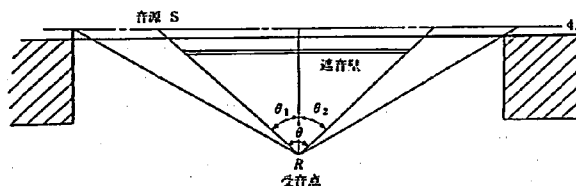
図-4.12 音源および遮音壁の見込み角
