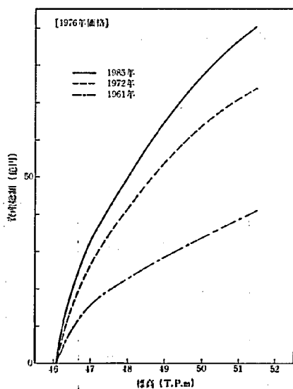
図-22 標高～資産額曲線の例示 (N地点近傍約 0.57 km² について)
