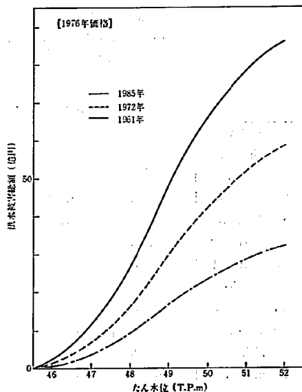
図-23 たん水位～被害額曲線の例示 (N地点の近傍約 0.57 km² について)
