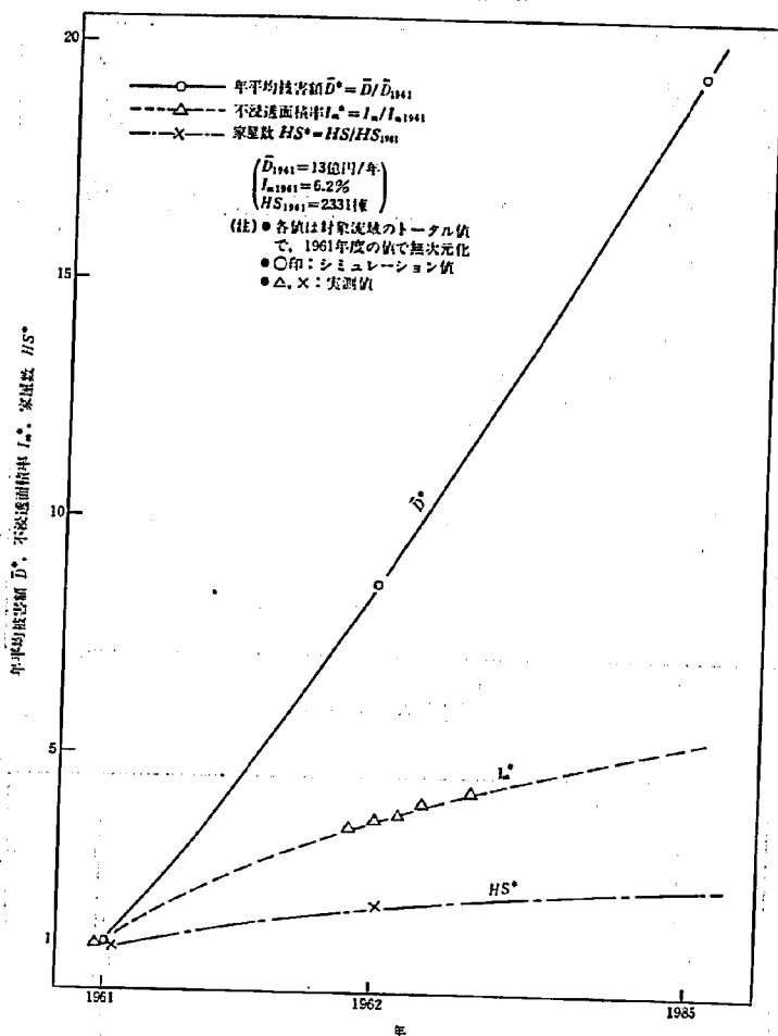
図-32 治水対策なしに都市化が進行した場合の洪水被害の増大 (不透透面積率, 家屋数を併記)
