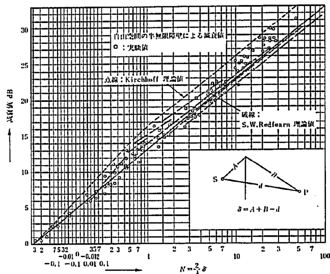
図-4.2 半無限障壁の減衰実験曲線(実線)。○点: 短音による実験値
