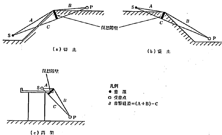
図-4.10 這へい物による音響経路差の計算
