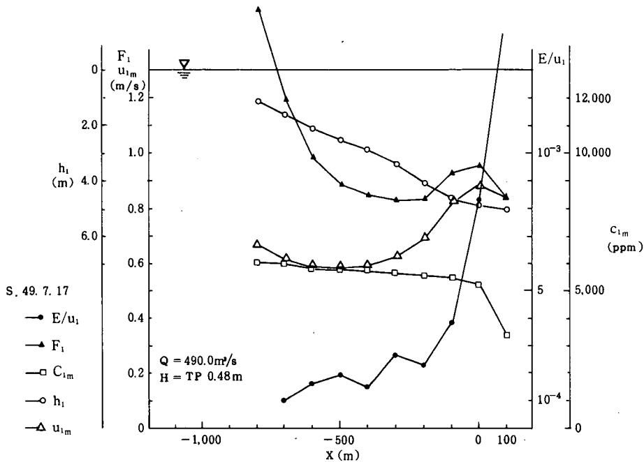
図-1-11 水利諸量縦断変化図 (最上川)
