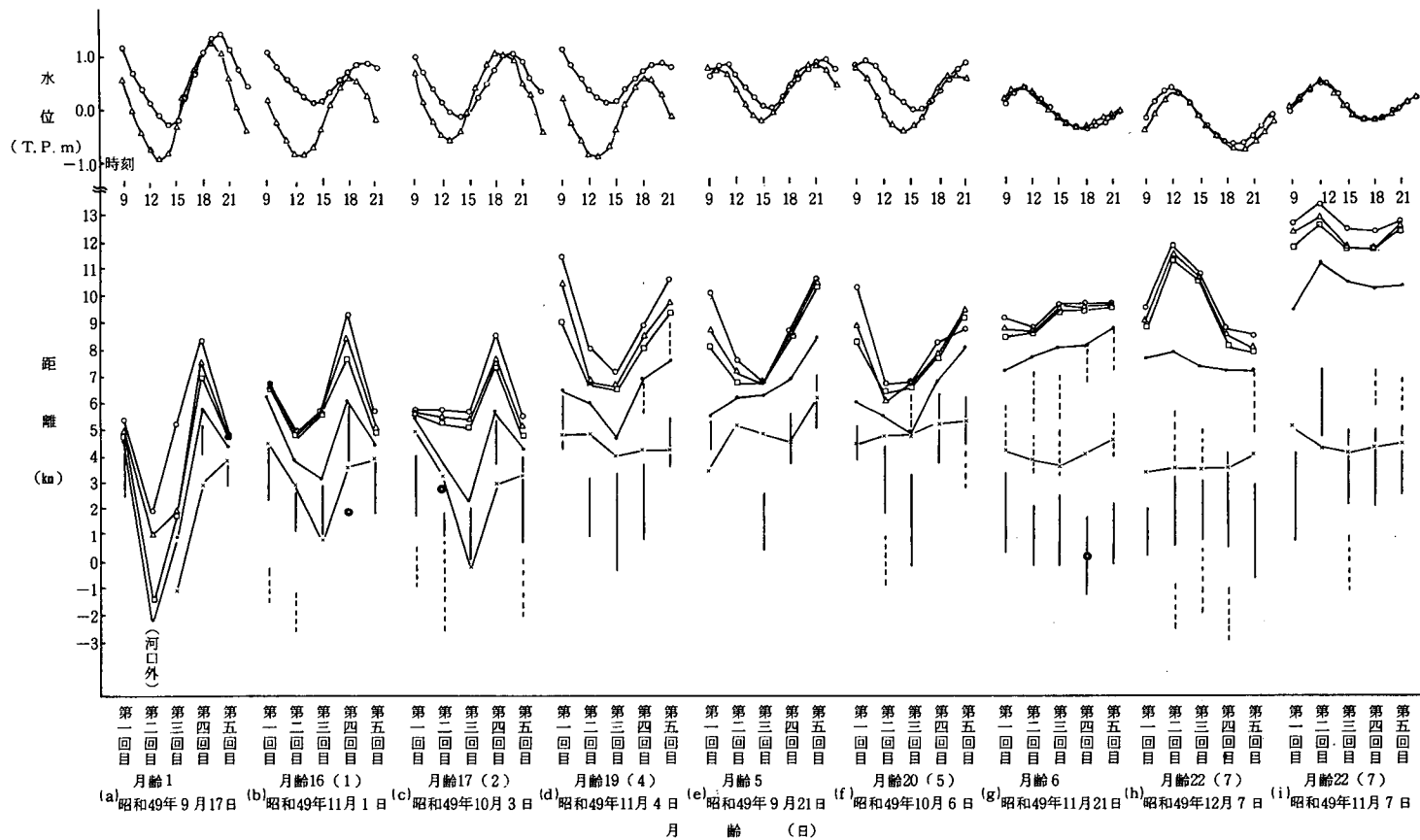
図-1・18(a) 内部渦の範囲とその移動状況、及び濃度分布と水位変化の関係(長良川)
