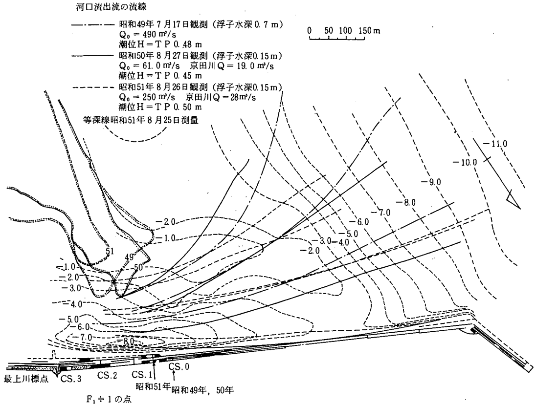
図-1.3 最上川の河口流出流
