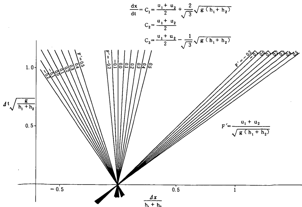
図-3・2 特性曲線の勾配
