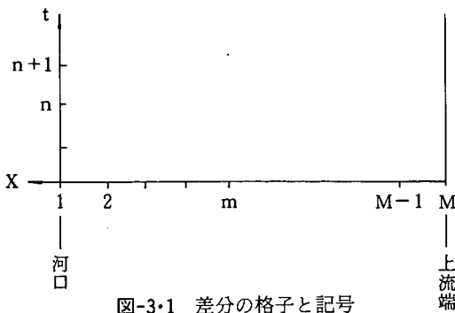
図-3・1 差分の格子と記号
