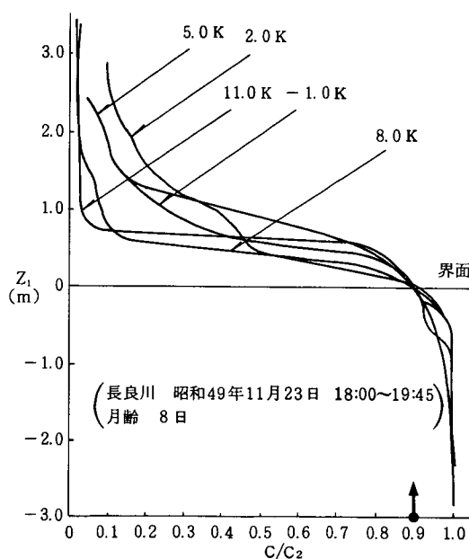
図-2・2 Z = Z_{c=0.9c_2} を界面としたときの濃度分布曲線
