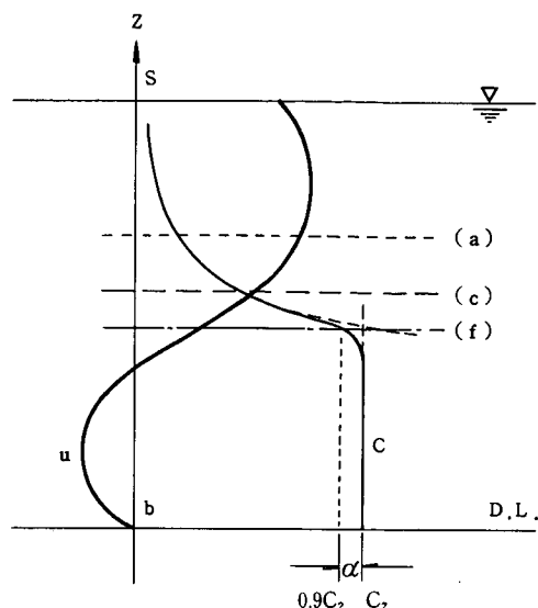
図-2.1 内部境界面位置の定義
