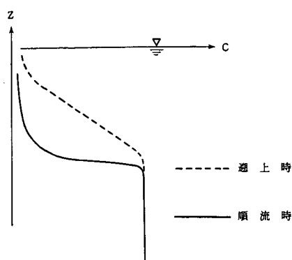
図-4-22 濃度分布形状のパターン
