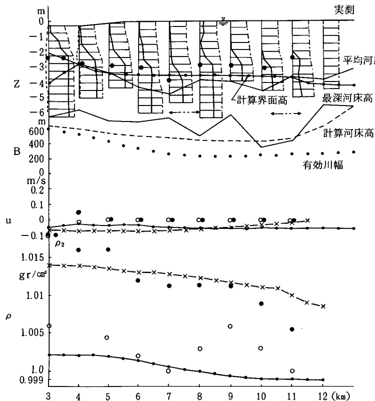
図 3-16 (a) 長良川成層流の数値計算結果 (縦断変化量, 11月23日)
