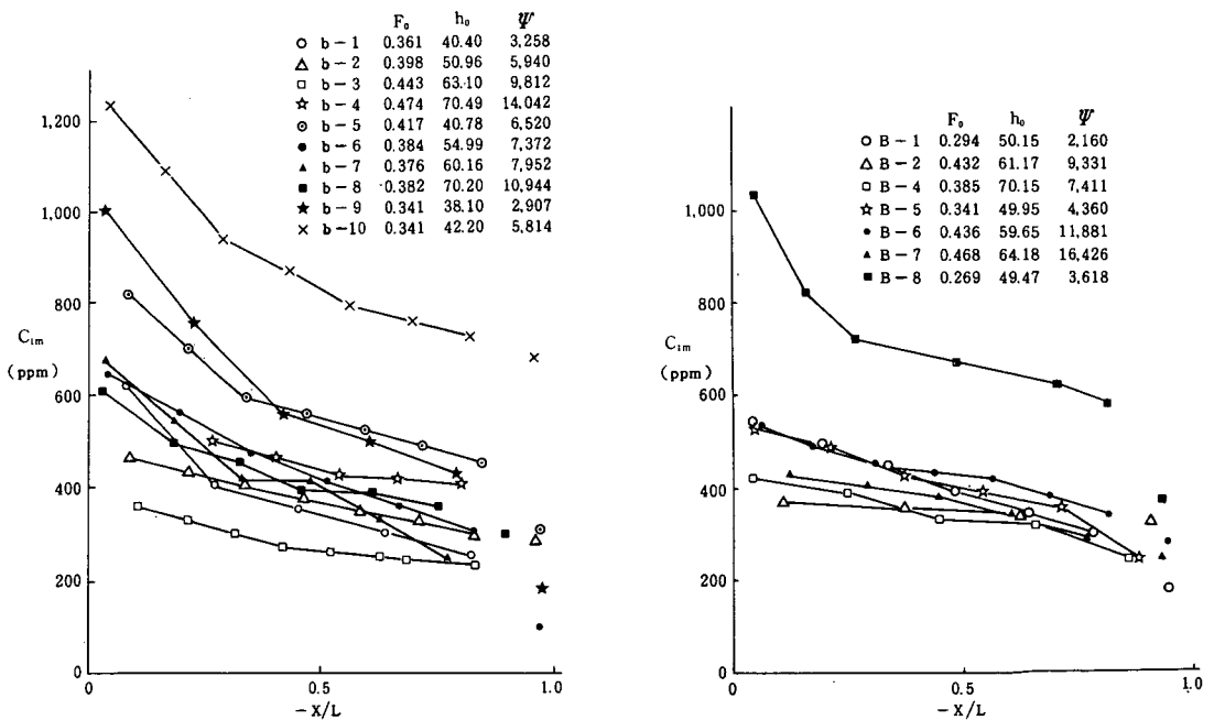
図-1-25(a) 層の塩素イオン濃度の縦断変化 (実験水路, 定常状態)
