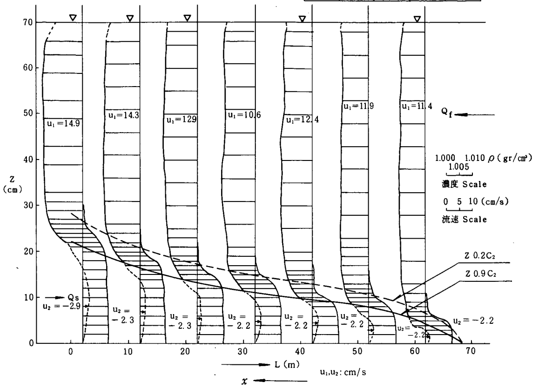
図-2・3 100m水路における塩水くさび
