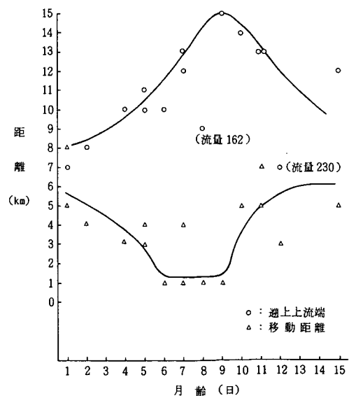
図-4.13 最長遡上距離と変動距離の月齢変化 (長良川)
