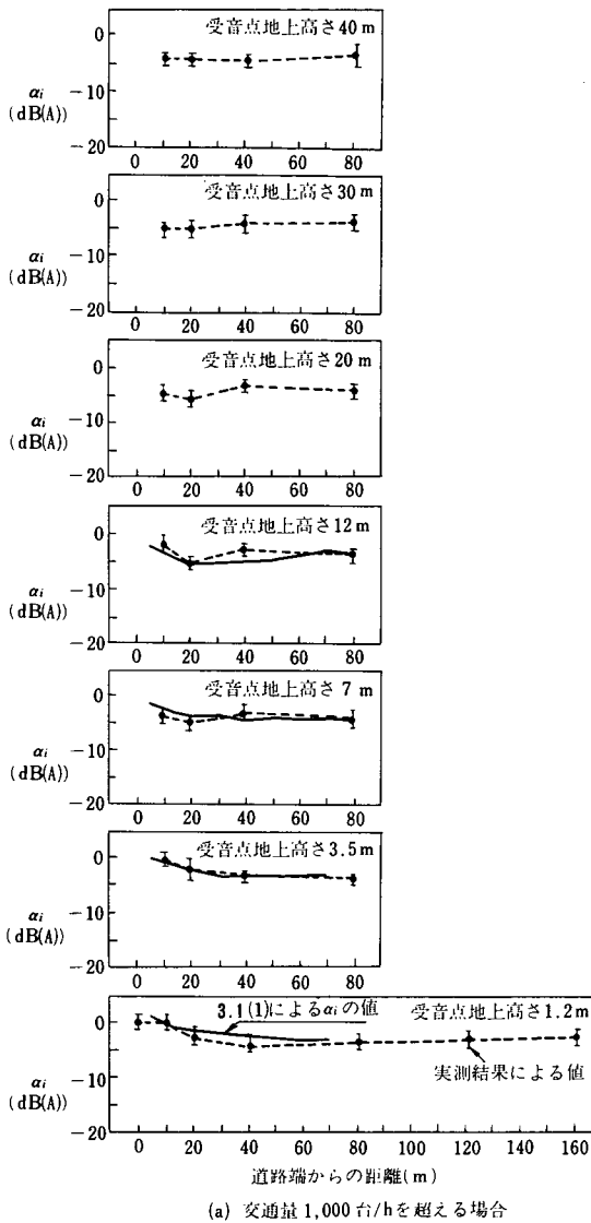
図-3-20 道路端から距離方向への \alpha_i (高架構造)
