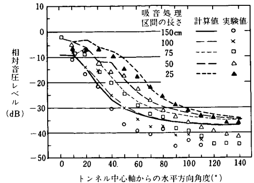
図-5-13 吸音処理区間を含むトンネル坑口からの放射指向性状 (音源: 16kHz オクターブバンドノイズ, 音源位置: 坑口より150cm)
