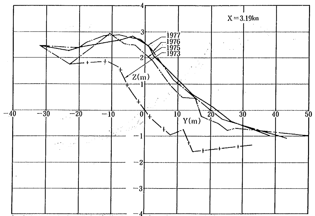
図-2.18 Sanur 海岸の X = 3.19\text{km} 地点における海浜断面形の変化 (Tsuchiya, 1978)
