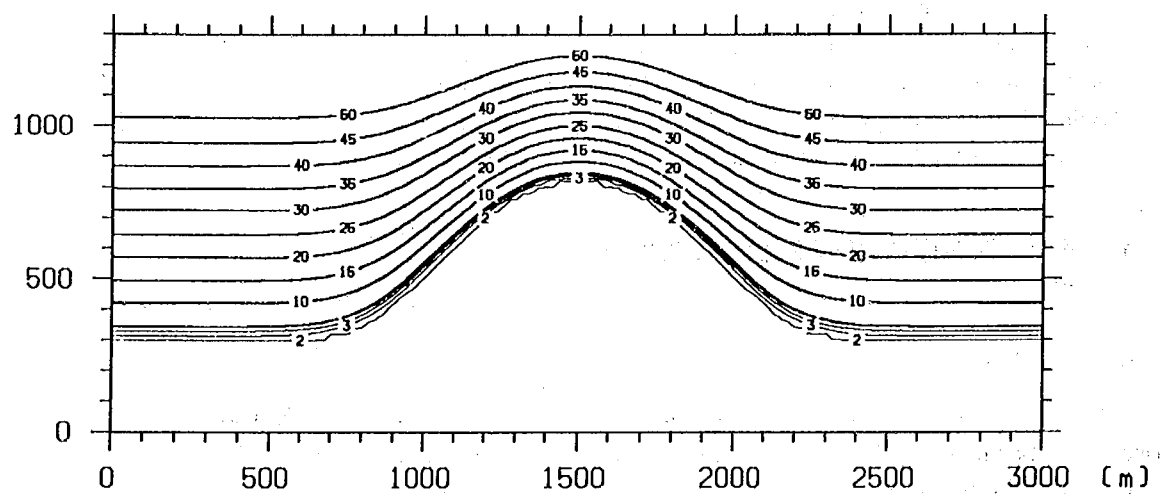
図-5.2 幅広いリーフのモデル地形
