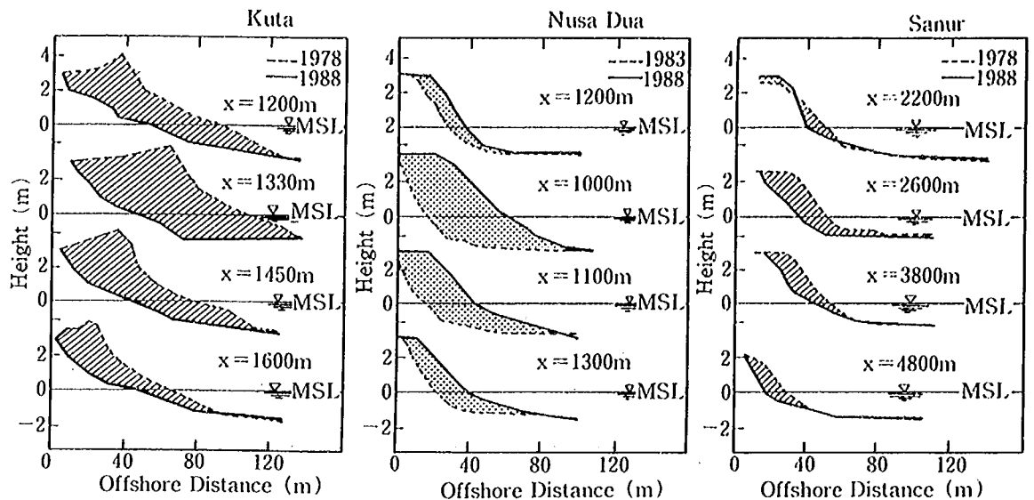
図-2.10 海浜断面形の変化 (Kuta, Nusa, Dua, Sanur 海岸)
