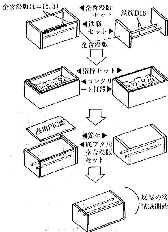
図-5・2 ポリマー含浸防食試験体の製作手順
