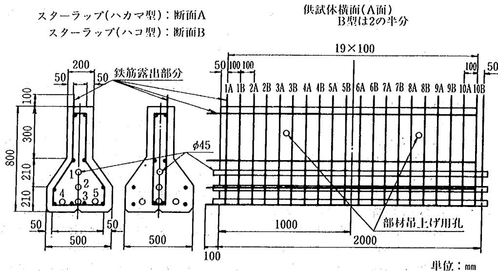
図-6・8 電位分布および電流密度測定用供試体の形状
