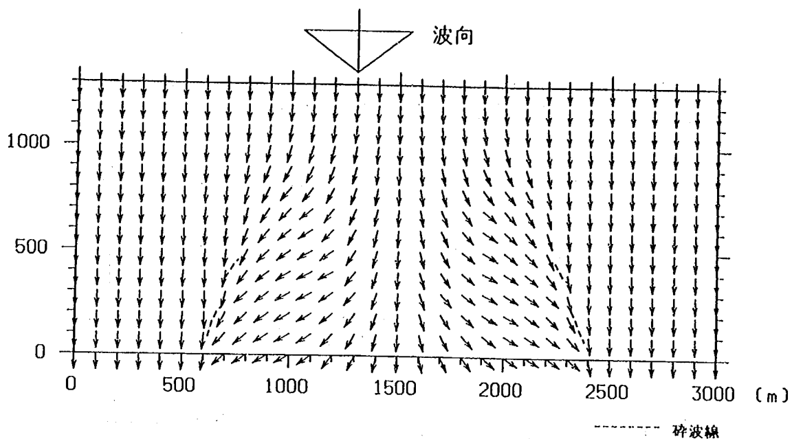
図-5.3 リーフギャップ周りでの波向分布
