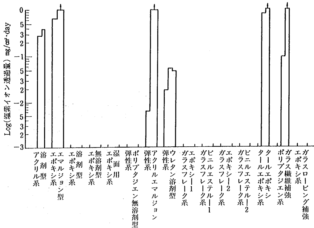
図-4・1 塗膜の塩素イオン透過量試験結果
