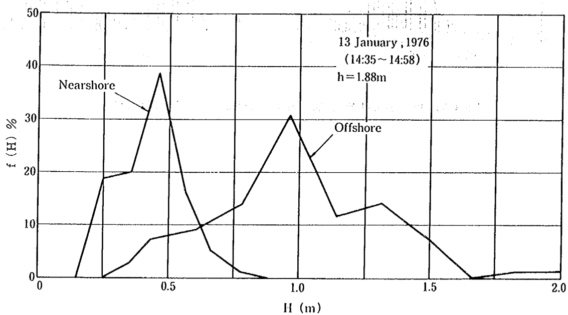
図-3.35 Kuta 海岸におけるリーフ内外の有義波高・周期の分布 (その2) (Tsuchiya et al., 1976)
