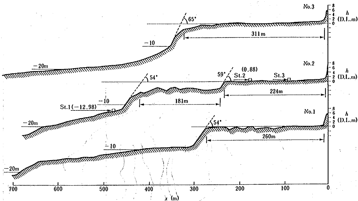
図-2.5 大宜味地区におけるリーフの断面形と観測計器の設置地点の高さ
