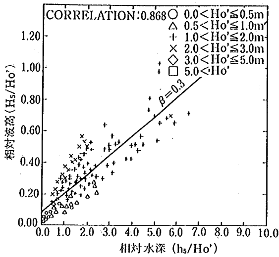
図-3.52 相対波高 ( H_s/H_o' ) と相対水深 ( h_s/H_o' ) の関係
