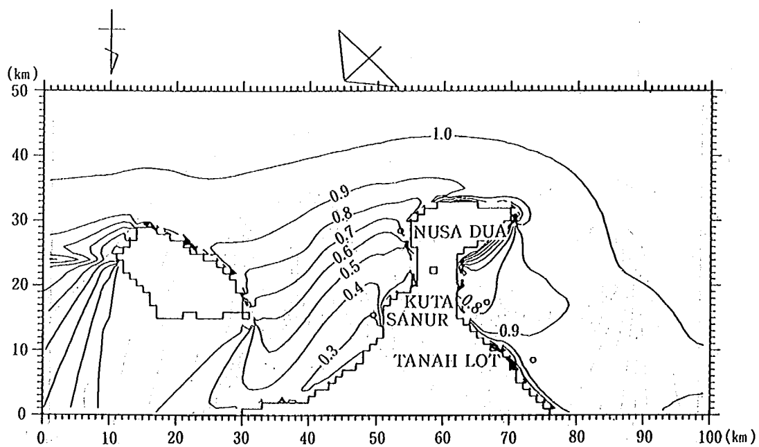
図-3.24 バリ島南部海岸沖での波高分布（入射方向 S W）
