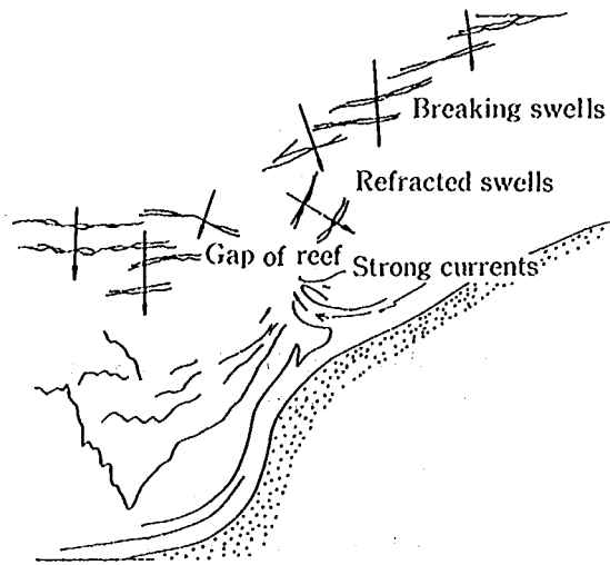
図-4.9 Nusa Dua 海岸のリーフギャップ付近の流れのパターン (Tsuchiya, 1987)
