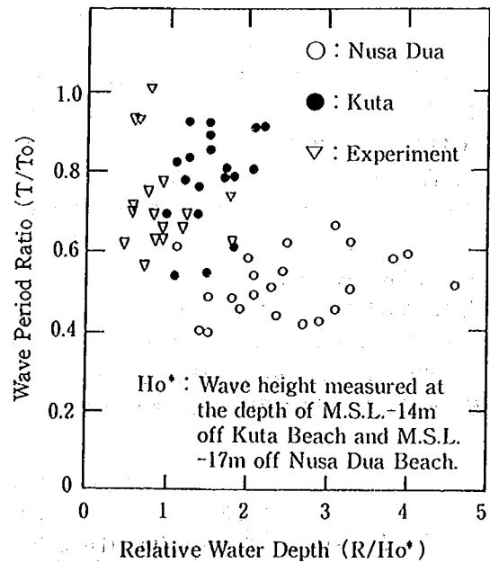
図-3.42 リーフ内外の周期比と相対水深との関係
