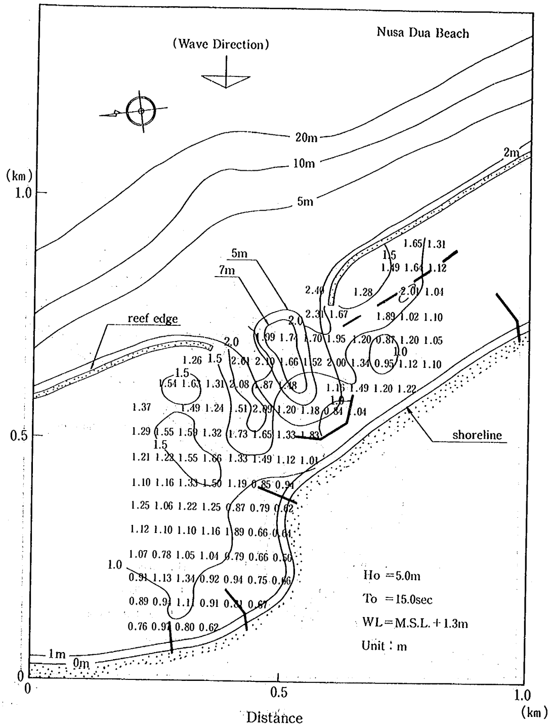
図-4.15 波高の平面分布 (Nusa Dua 海岸)
