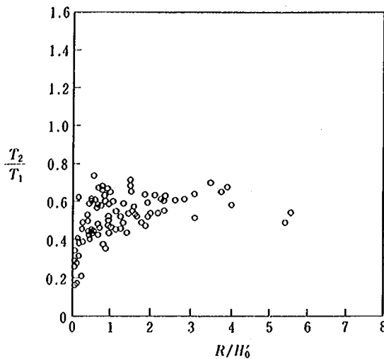
図-3.15 周期比と波高リーフ上水深比の関係 (St. 2)
