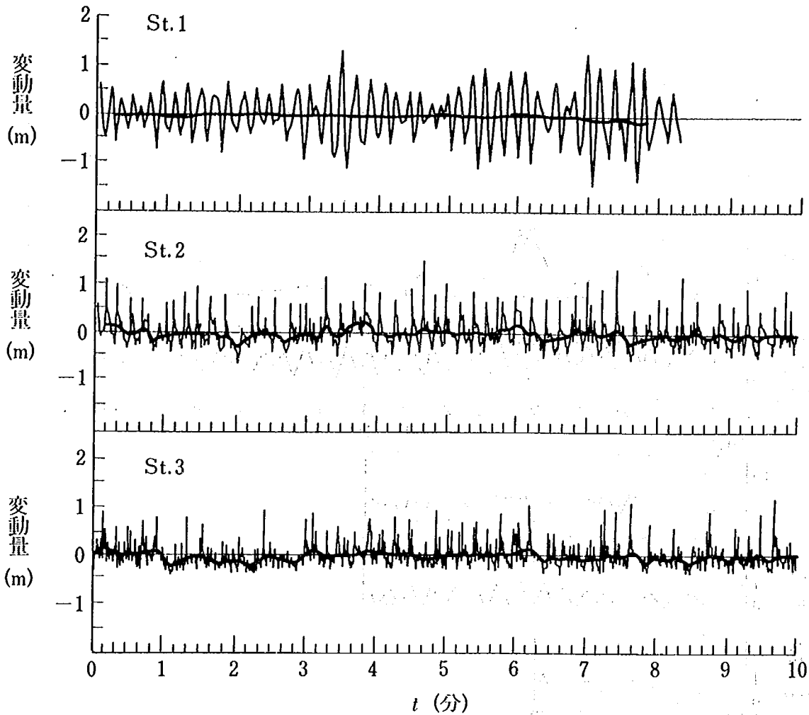
図-3.9 St. 2 における水面波形記録の 1 例 (1987年 2 月 28 日 8 時測定)
