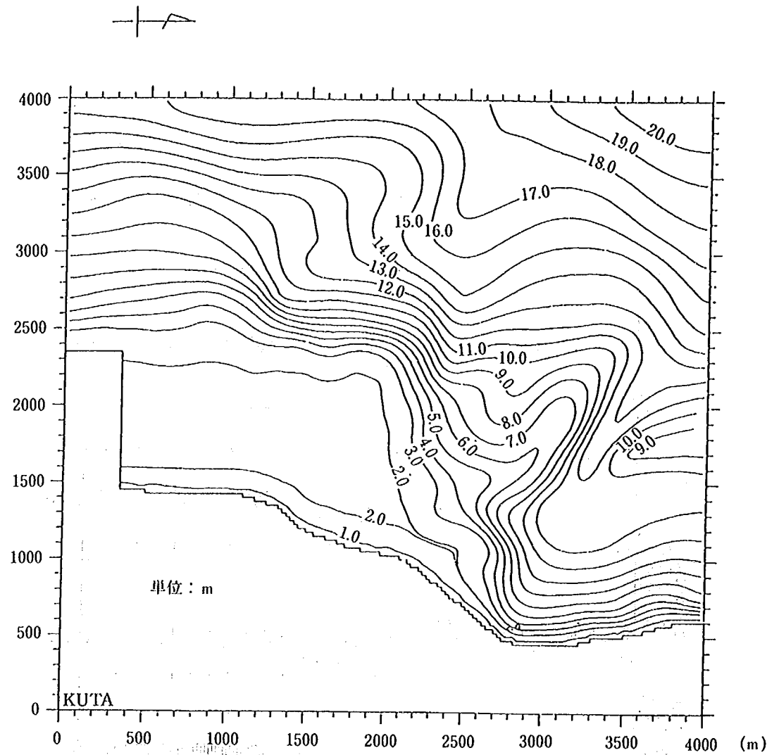
図-5.8 Kuta 海岸の深淺図
