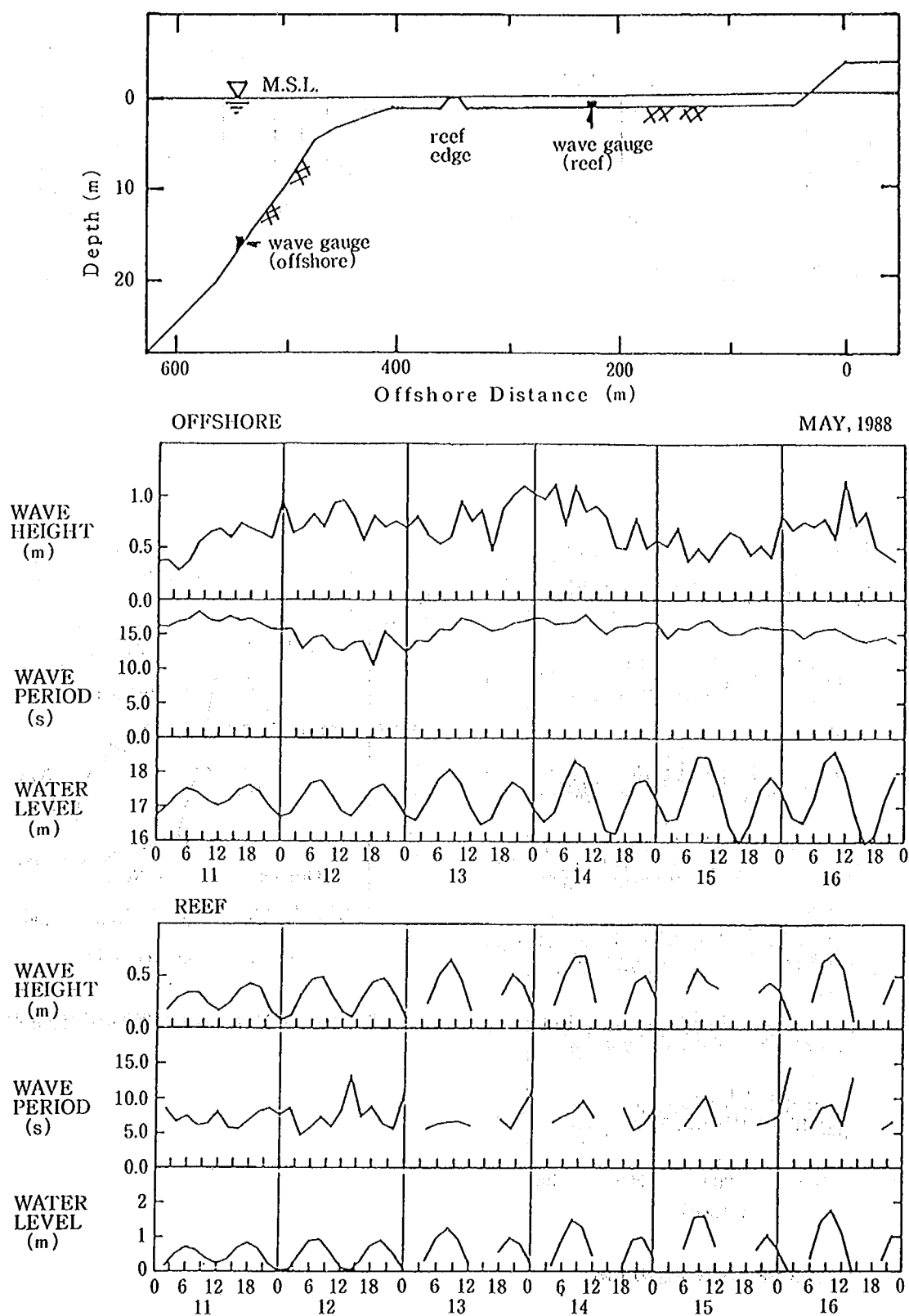
図-3.36 Nusa Dua 海岸におけるリーフ内外の有義波高・周期の経時変化
