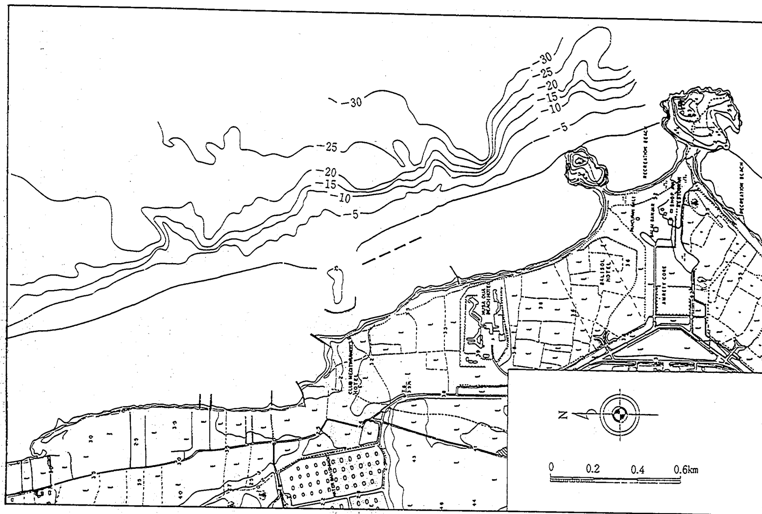
図-2.11 Nusa Dua 海岸の深浅図
