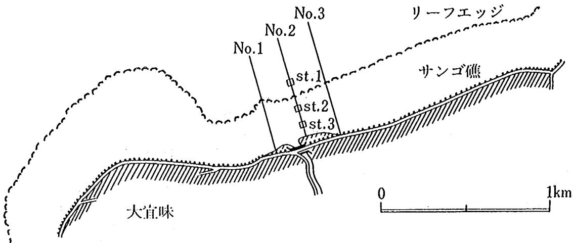
図-2.4 大宜味地区における深浅測量の測線位置と観測計器の配置
