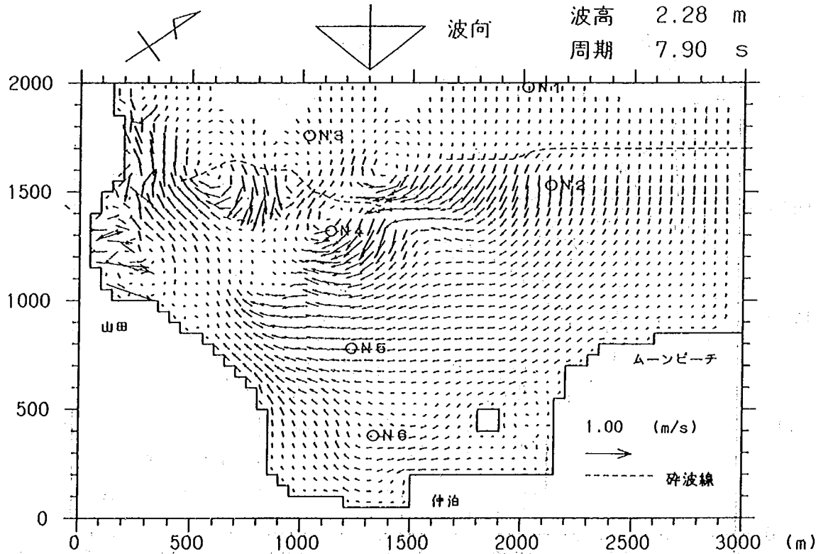
図-4.24 海浜流の流況 (ケース 4, H_1=2.28\text{ m} , T_1=7.9\text{ s} )
