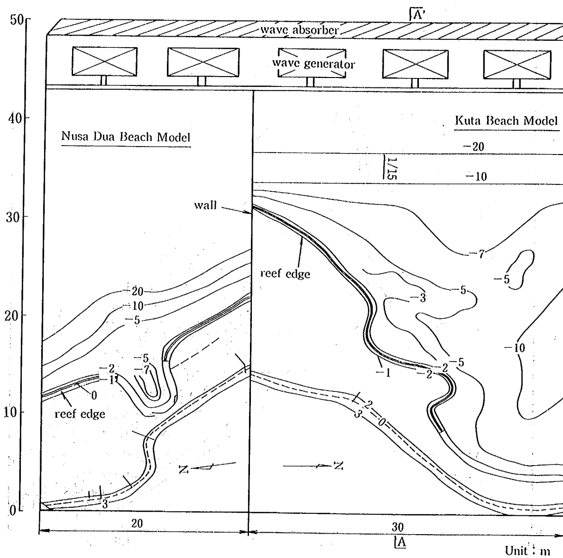
図-4.11 Kuta および Nusa Dua 海岸の模型形状
