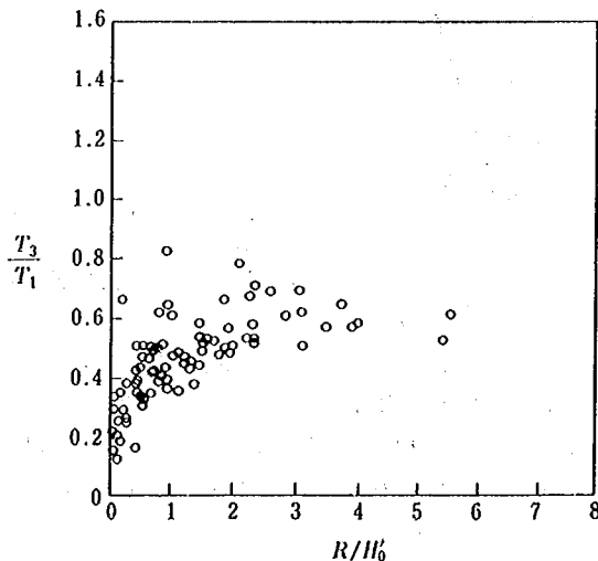
図-3.16 周期比と波高リーフ上水深比の関係 (St. 3)
