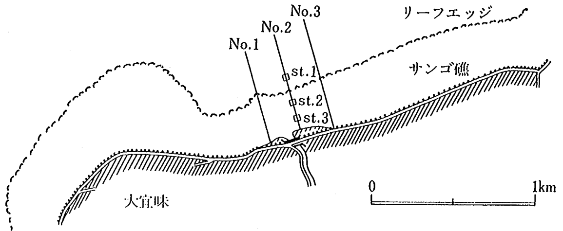
図-3.8 大宜味地区における測線配置
