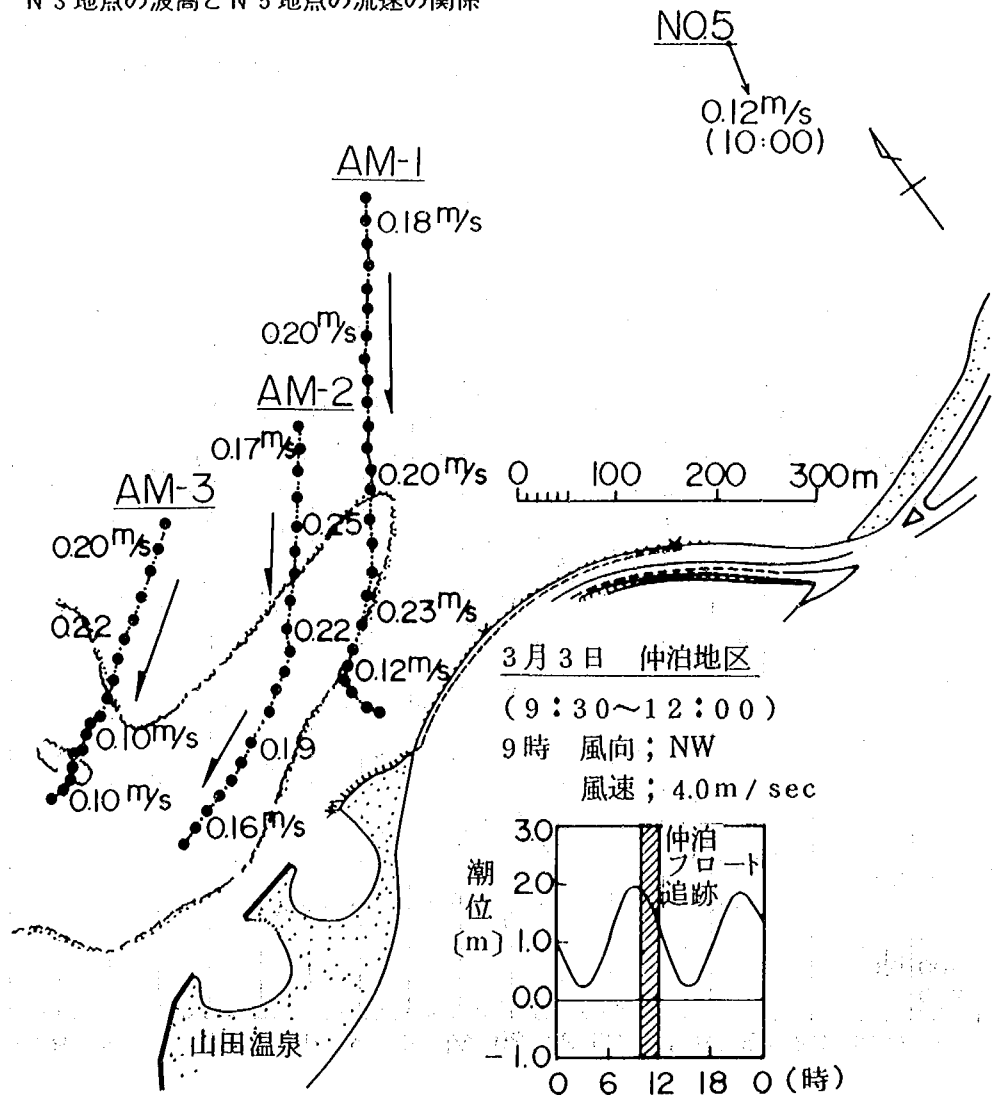
図-4.4 フロート追跡による流速測定(山田温泉沖)
