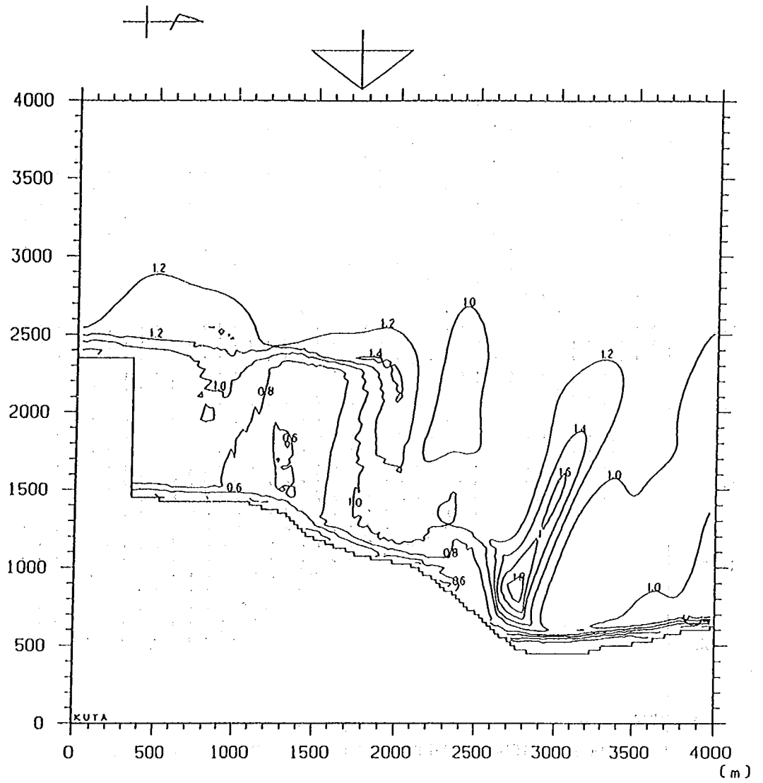
図-5.10 Kuta 海岸の波高分布 (入射方向W)
