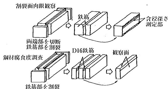
図-5・3 ポリマー含浸試験体の測定方法
