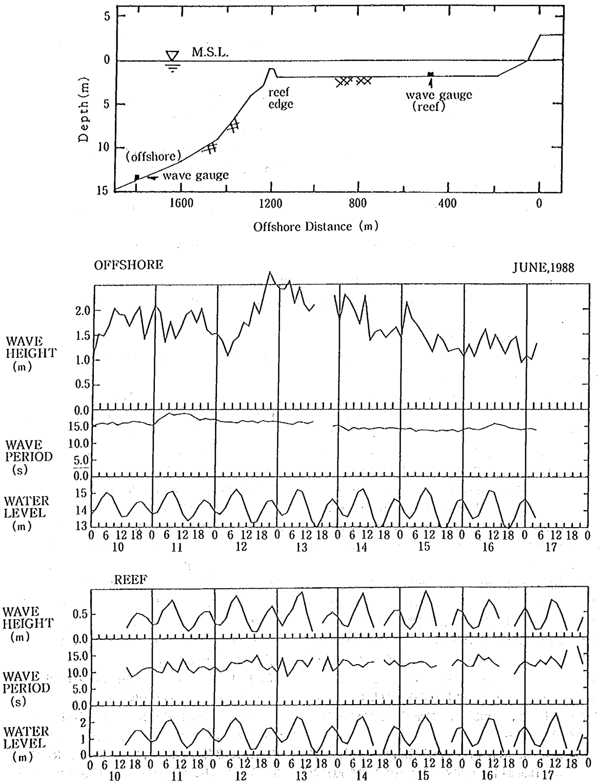
図-3.32 Kuta 海岸におけるリーフ内外の有義波高・周期の経時変化
