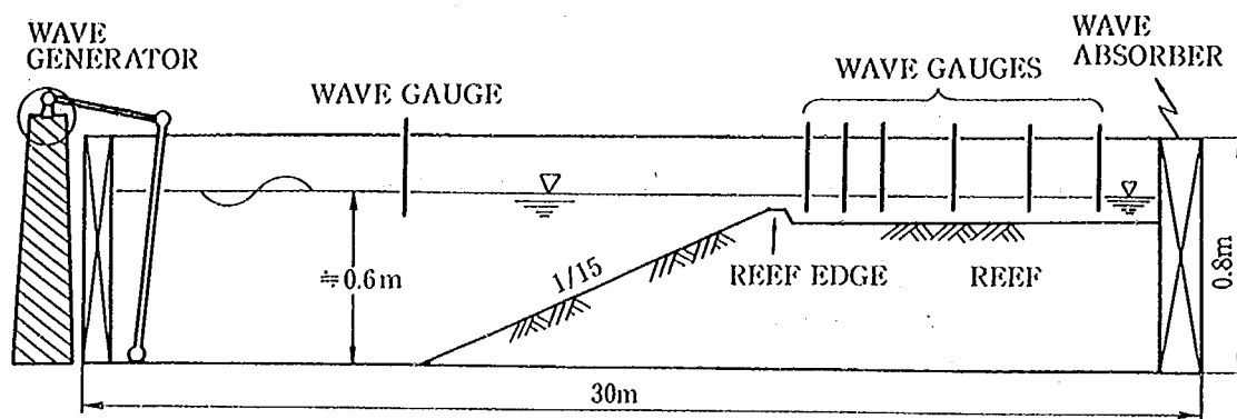
図-3.37 2次元造波水槽とリーフ模型
