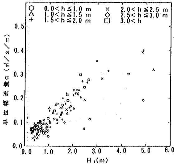
図-4.19 リーフ内の流量と入射波高の関係
