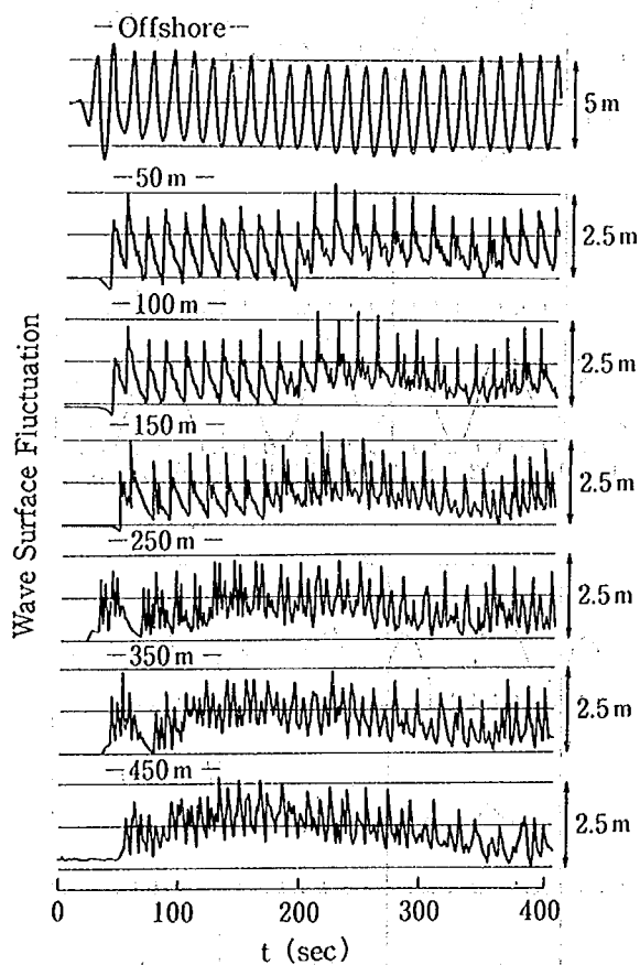
図-3.38 実験波形の一例
