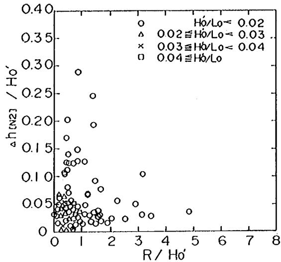
図-3.7 相対 wave set-up 量と R/H_0 の関係
