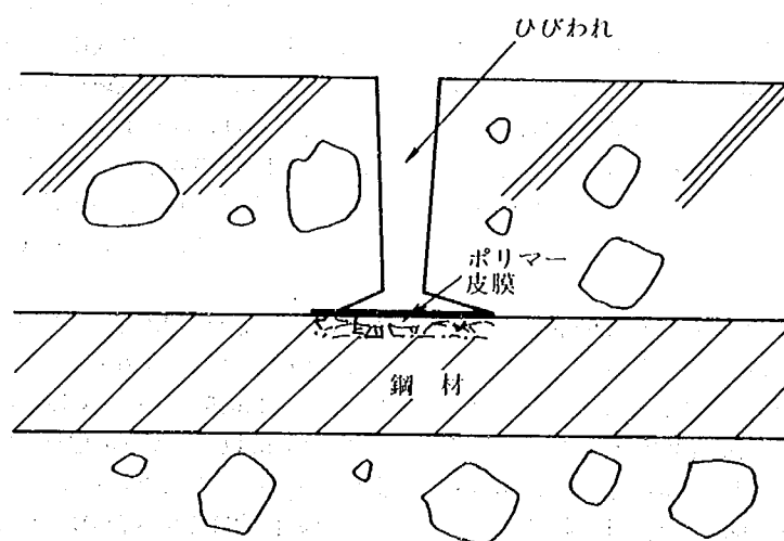
図-5・5 ひびわれ部分のポリマーの形態 (拡大模式図)
