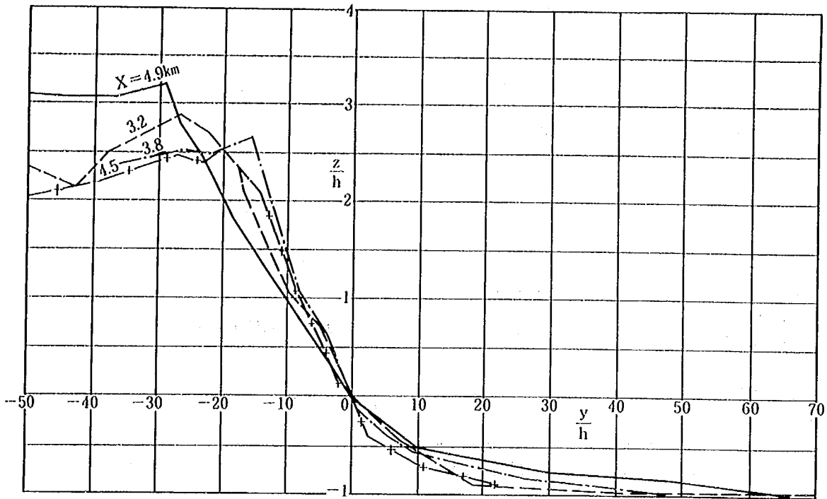
図-2.19 海浜断面形の無次元表示 (Tsuchiya, 1978)
