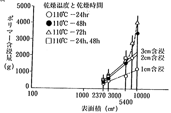
図-5.8 乾燥時間とモノマー置換率との関係
