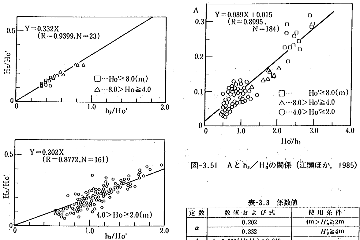
図-3.50 H_3/H_o' と h_2/H_o' の関係 (江頭ほか, 1985)
