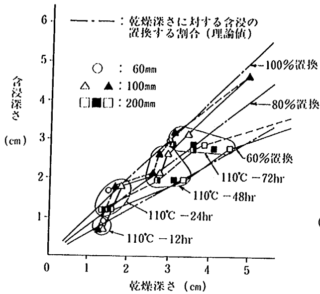
図-5.7 コンクリートの乾燥深さと含浸深さとの関係
