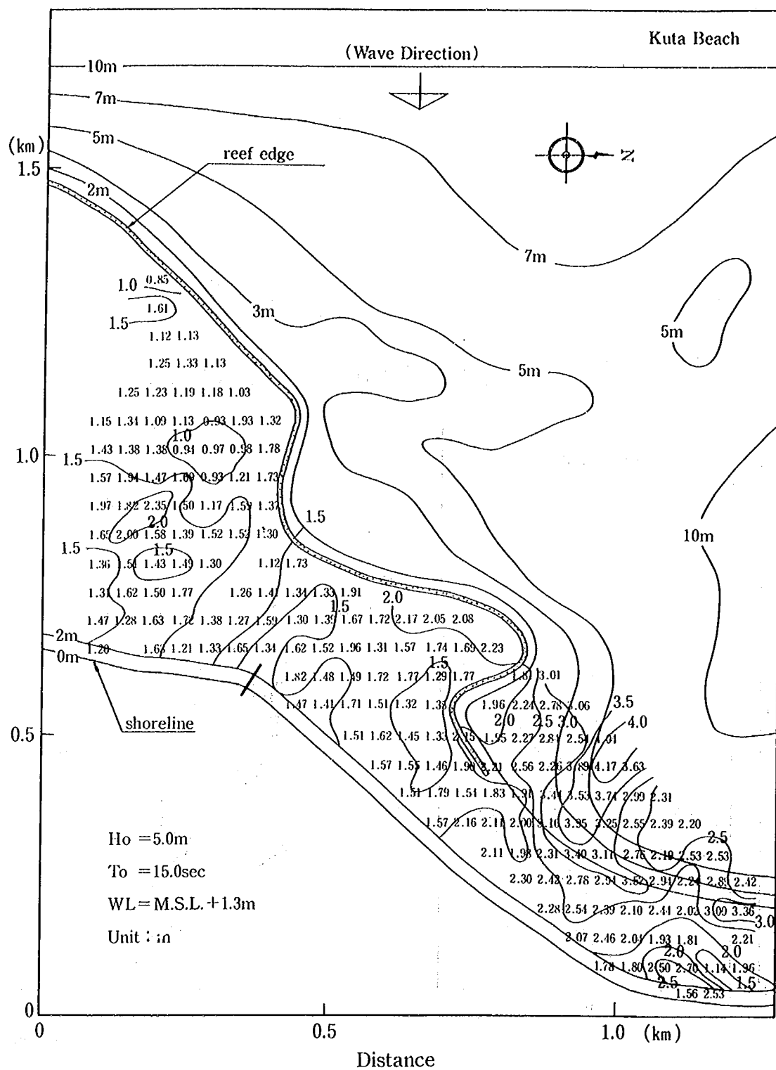
図-4.12 波高の平面分布 (Kuta 海岸)
