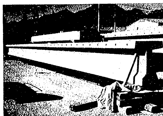
写真-4・4 コンクリート塗装桁部材（プレキャスト塗装方式）
