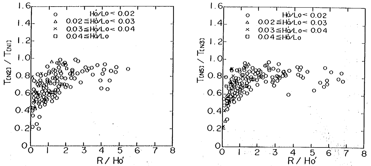
図-3.5 周期比と R/H_0' の関係
