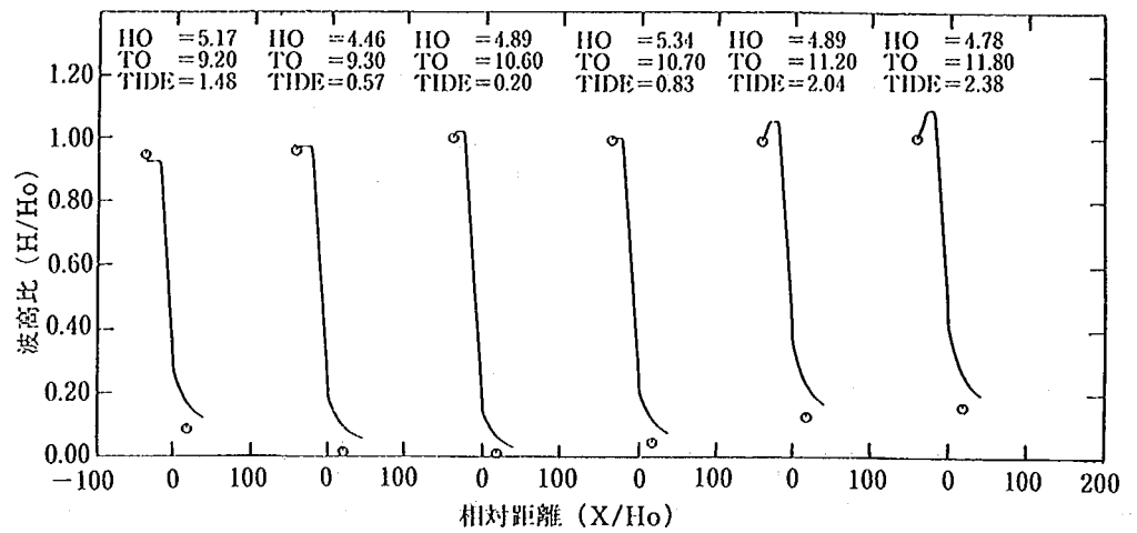
図-3.44 仲泊地区の北側線上における波高変化の比較
