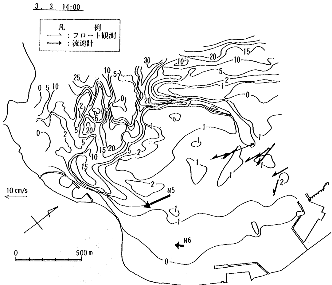
図-4.26 流速計およびフロートを用いた観測によって得られた流況 (1987年3月3日, 14:00観測)
