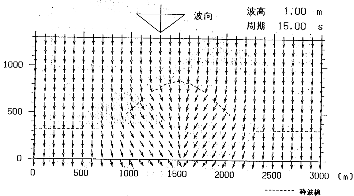
図-5.4 幅広いリーフの周りでの波向分布
