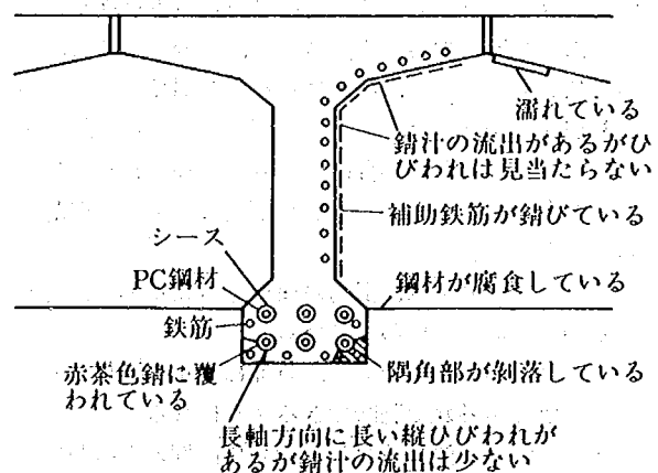
図-3・3 コンクリート桁の損傷状況別
