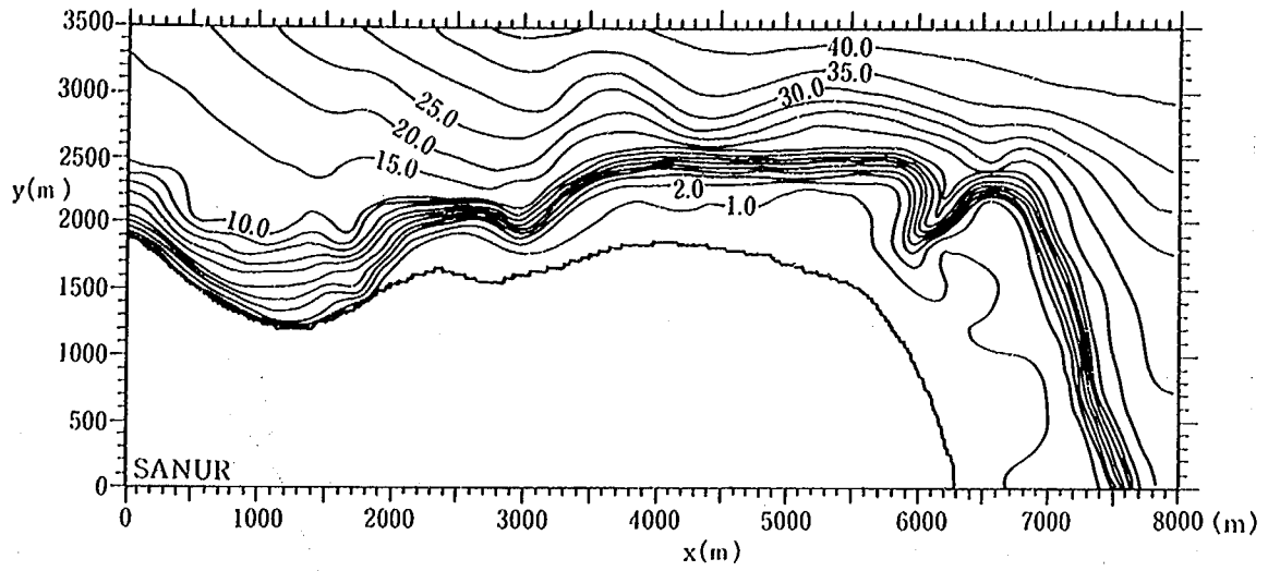
図-3.29 Sanur 海岸の海底地形
