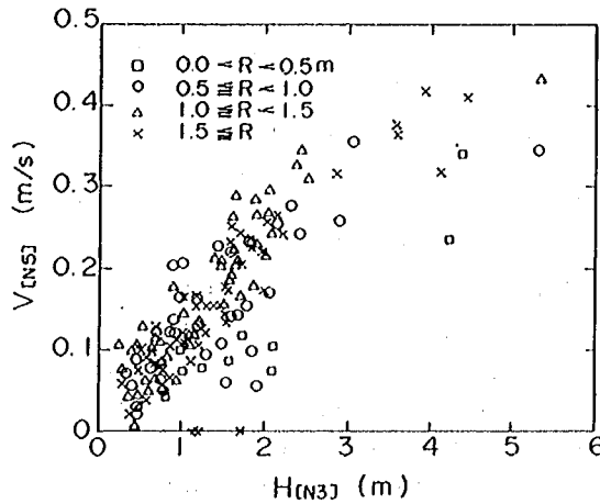
図-4.3 N 3 地点の波高と N 5 地点の流速の関係
