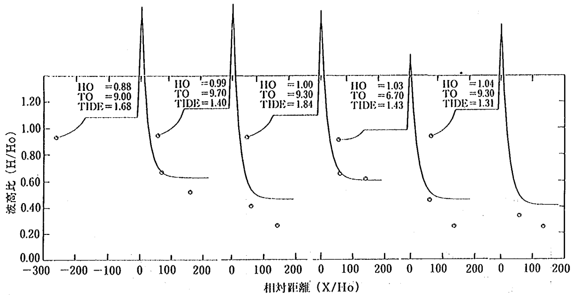
図-3.47 大宜地区の測線上における波高変化の比較(1)
