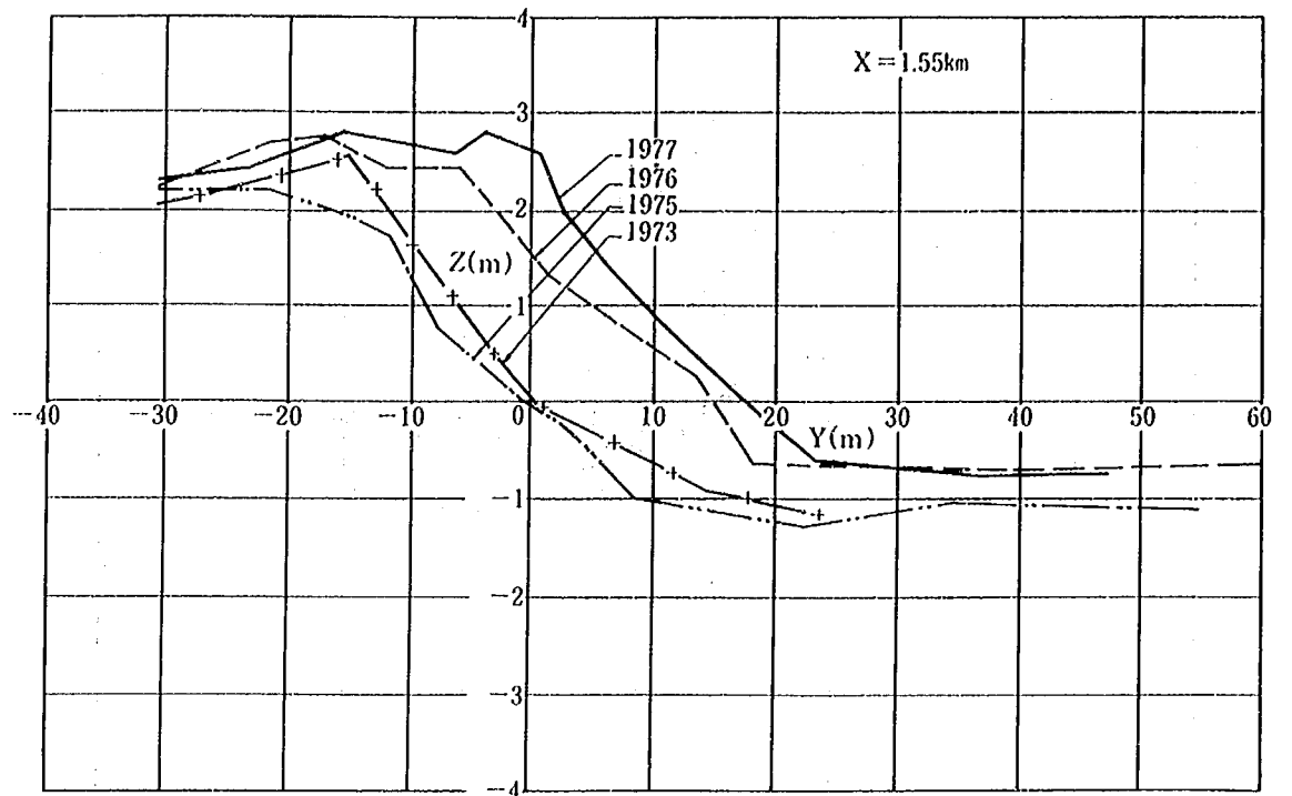
図-2.17 Sanur 海岸の X = 1.55\text{ km} 地点における海浜断面形の変化 (Tsuchiya, 1978)
