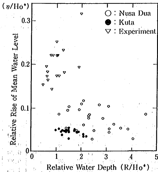
図-3.41 リーフ上の相対水位上昇量と相対水深との関係
