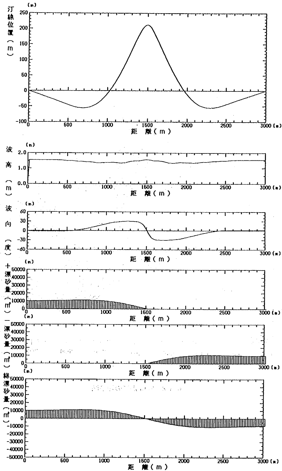
図-5.7 鰐広いリーフの周りでの汀線変化 (12か月後)
