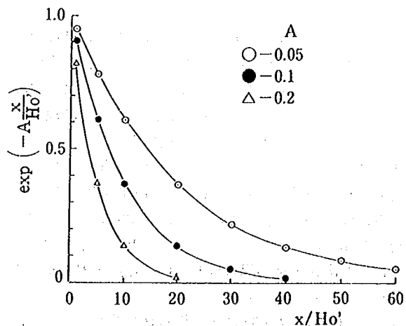
図-3.55 A の値による波高減衰割合の変化
