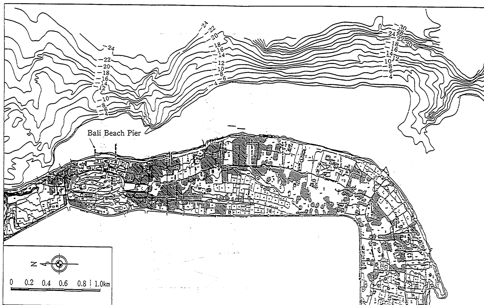
図-2.13 Sanur 海岸の深浅図
