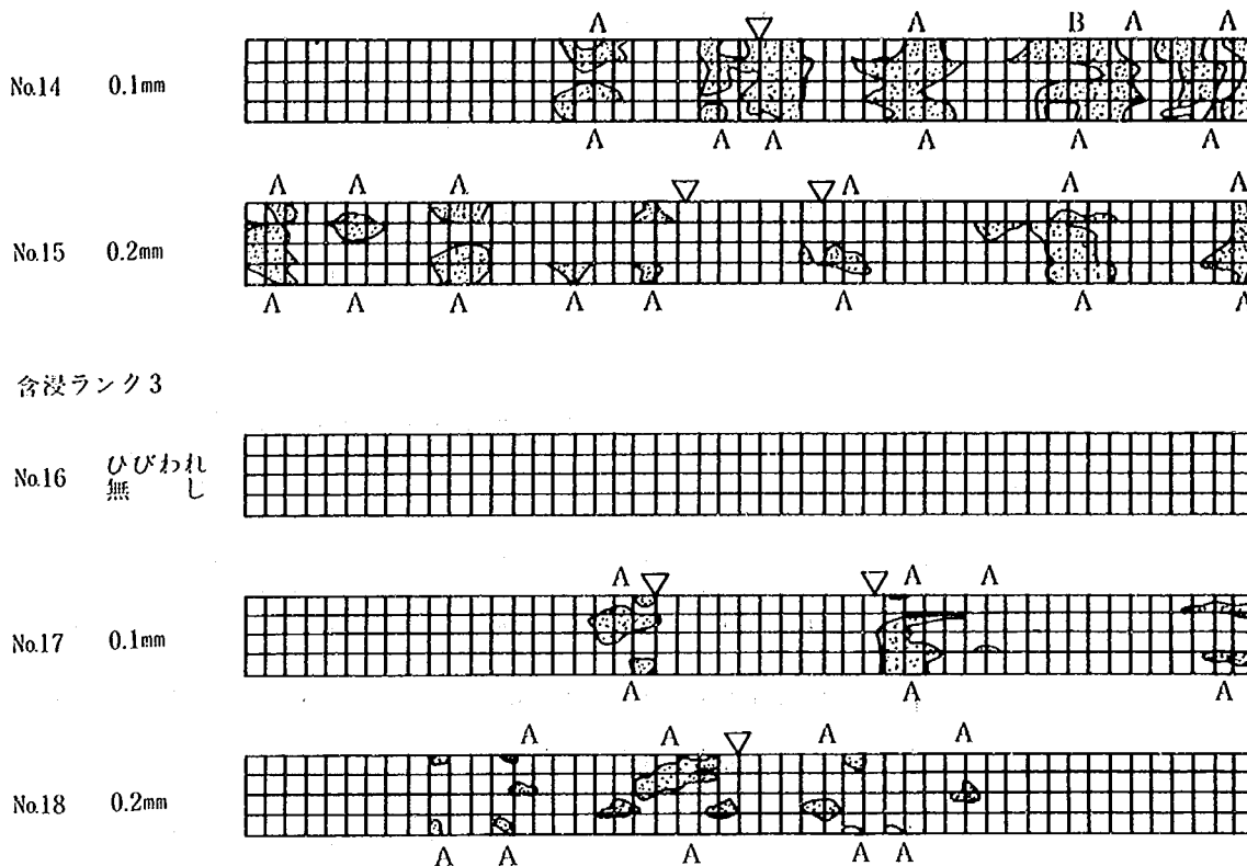
図-5.4 内部鋼材の腐食詳細状況
