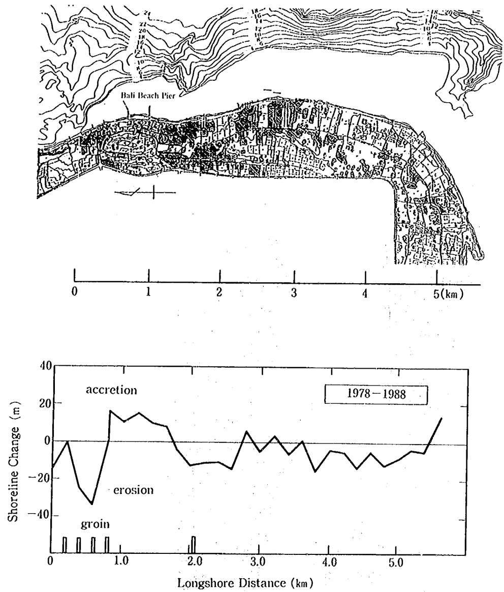
図-2.14 Sanur 海岸における汀線変化
