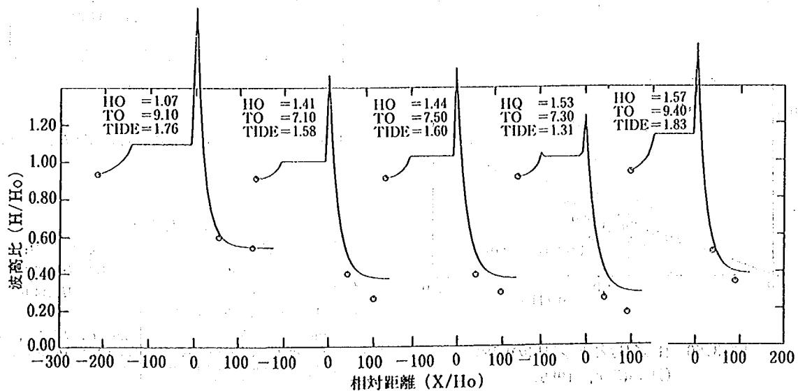
図-3.48 大宜味地区の測線上における波高変化の比較(2)
