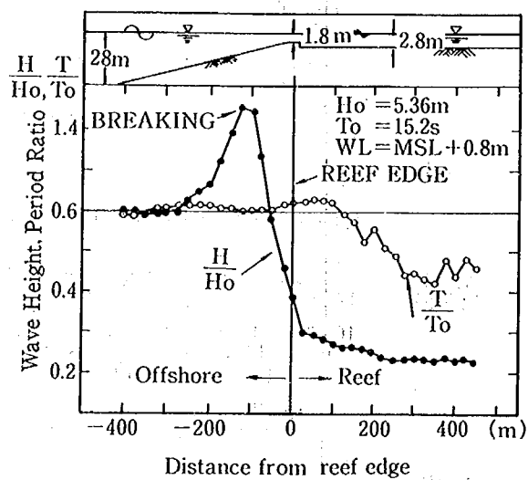
図-3.39 有義波高および周期の岸沖分布
