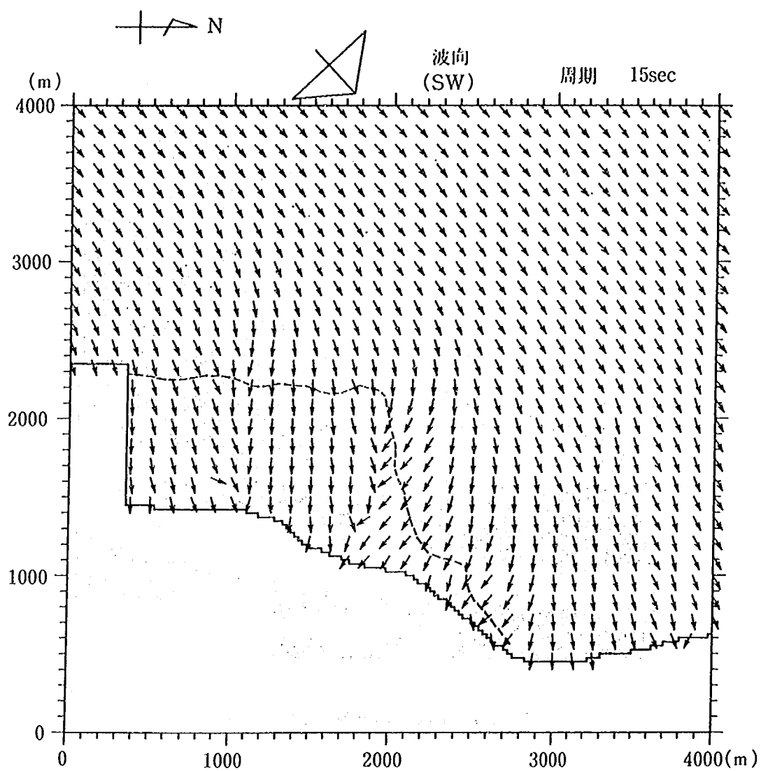
図-3.26 Kuta 海岸の屈折図
