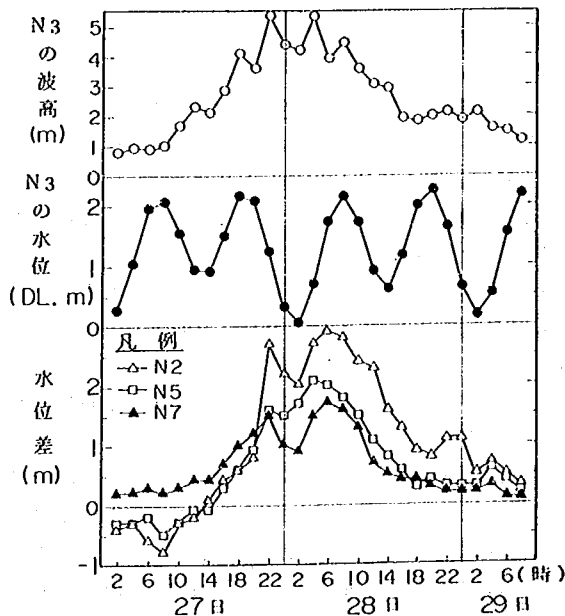
図-3.6 N 3 の波高、水位と外海との水位差の経時変化
