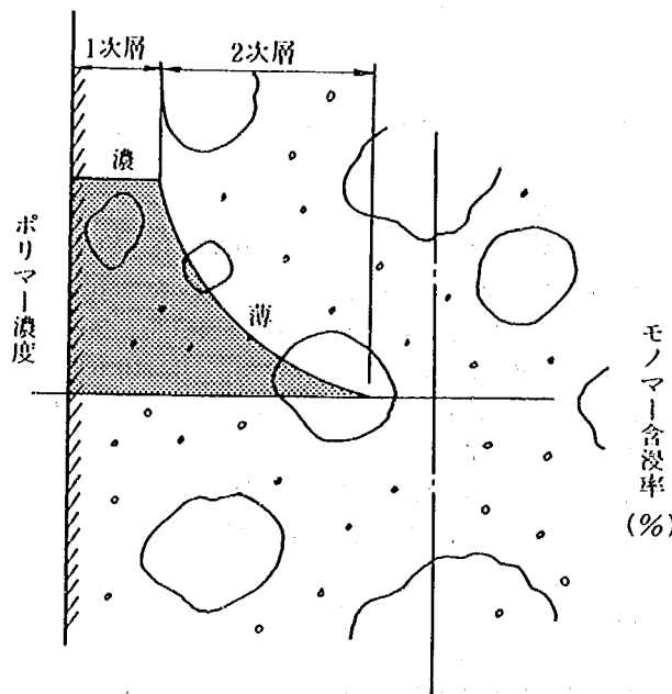
図-5.9 ポリマー含浸後のポリマー濃度分布
