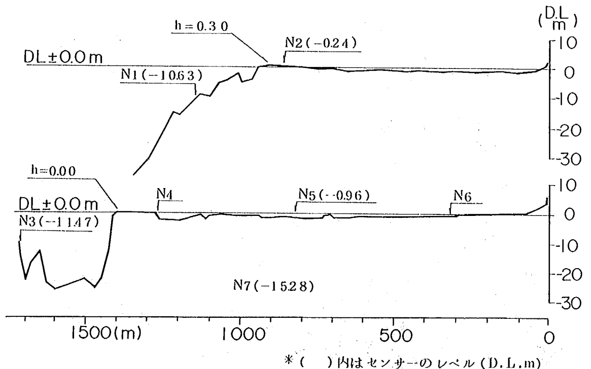
図-2.3 仲泊地区のリーフの断面形状
