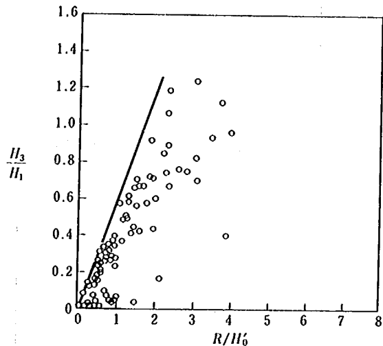
図-3.14 波高伝達率と波高リーフ上水深比の関係 (St. 3)
