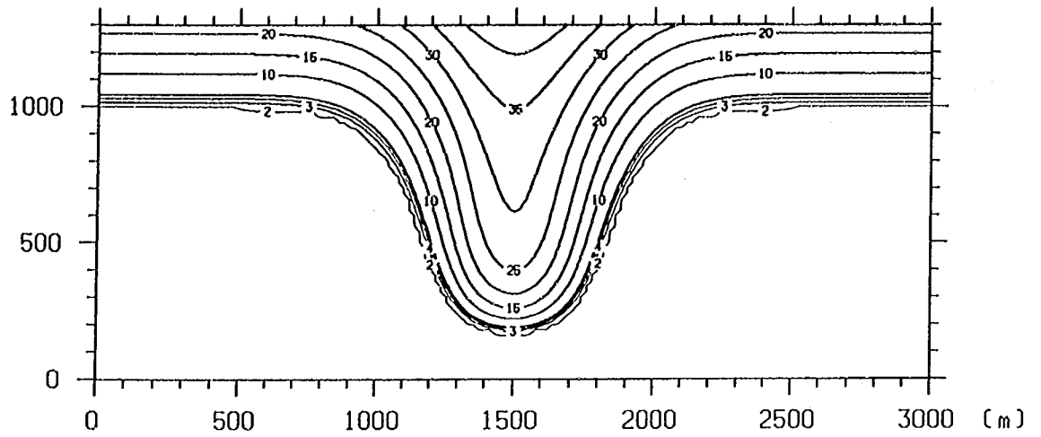
図-5.1 リーフギャップのモデル地形
