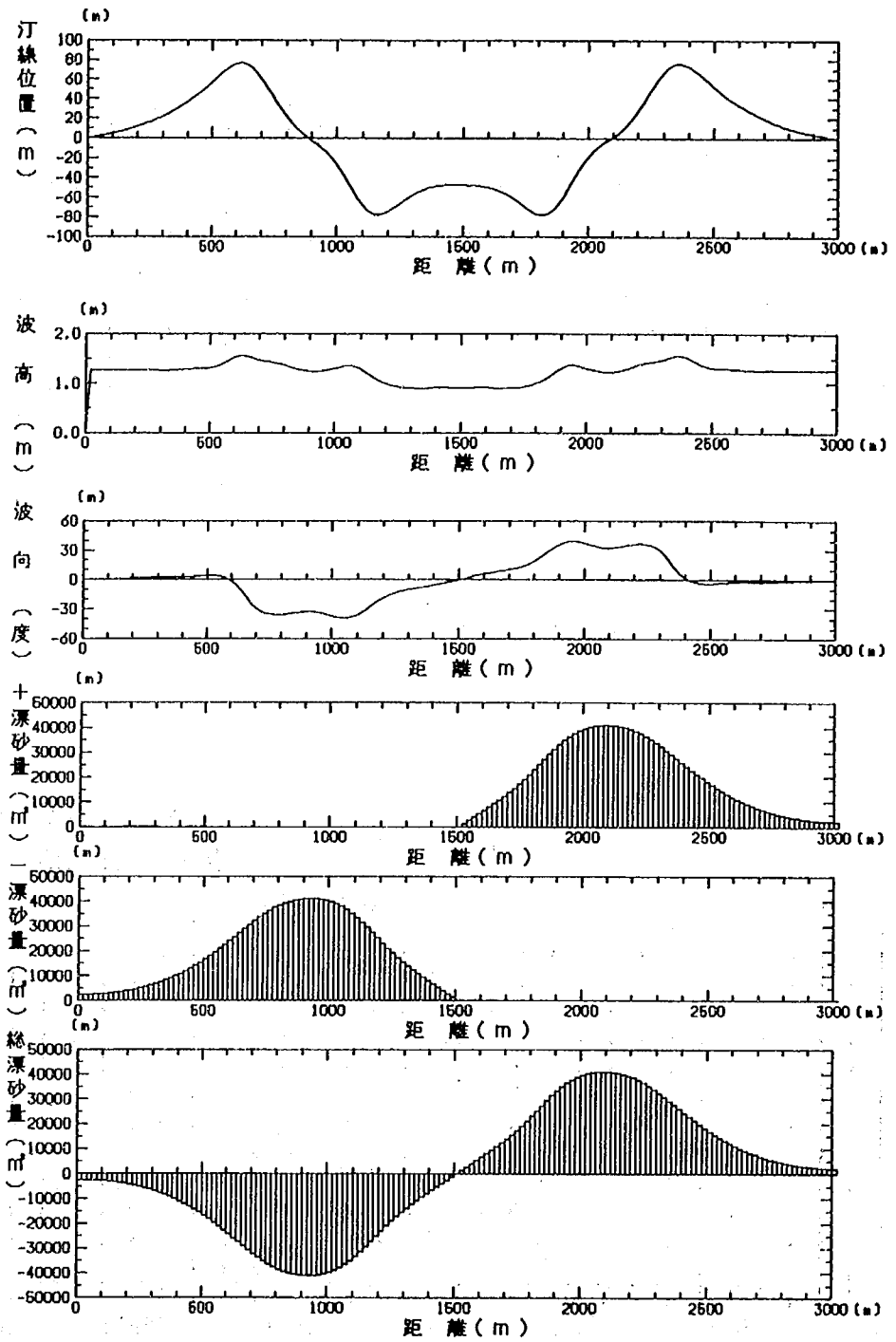
図-5.5 リーフギャップ周りでの汀線変化 (3か月後)
