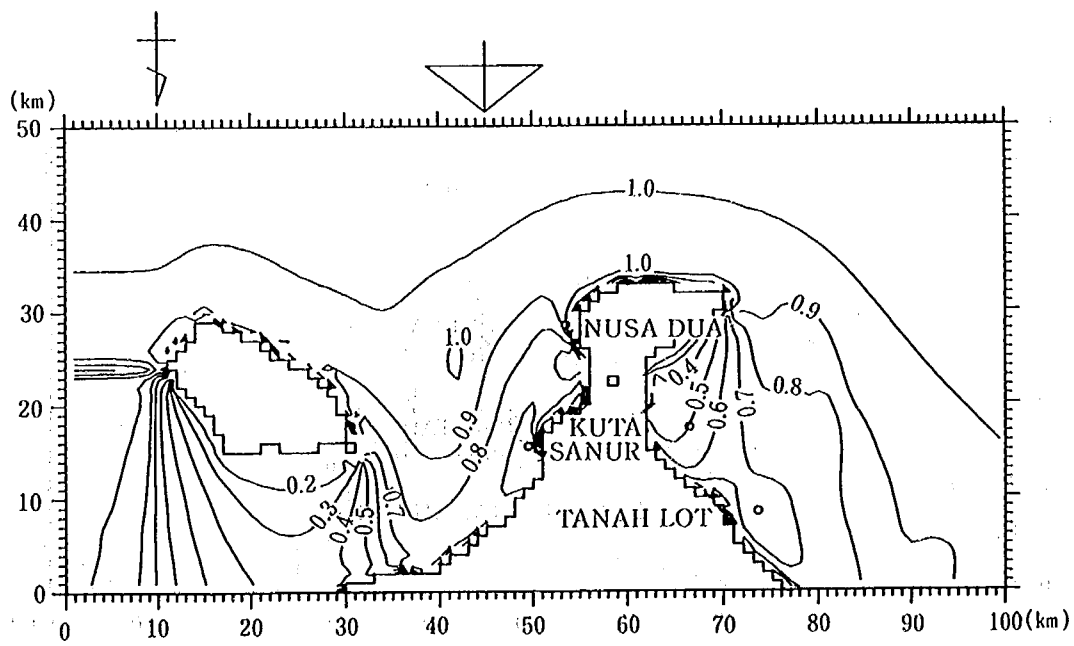
図-3.22 バリ島南部海岸沖での波高分布 (入射方向 S)
