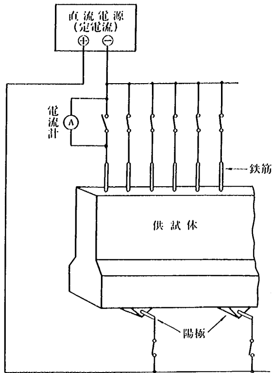
図-6・9 電位分布測定用供試体への電気防食の方法
