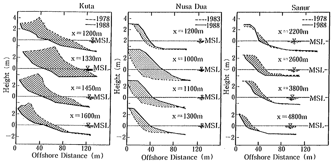
図-2.10 海浜断面形の変化 (Kuta, Nusa, Dua, Sanur 海岸)
