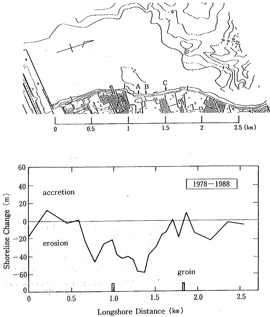
図-2.9 Kuta 海岸における汀線変化
