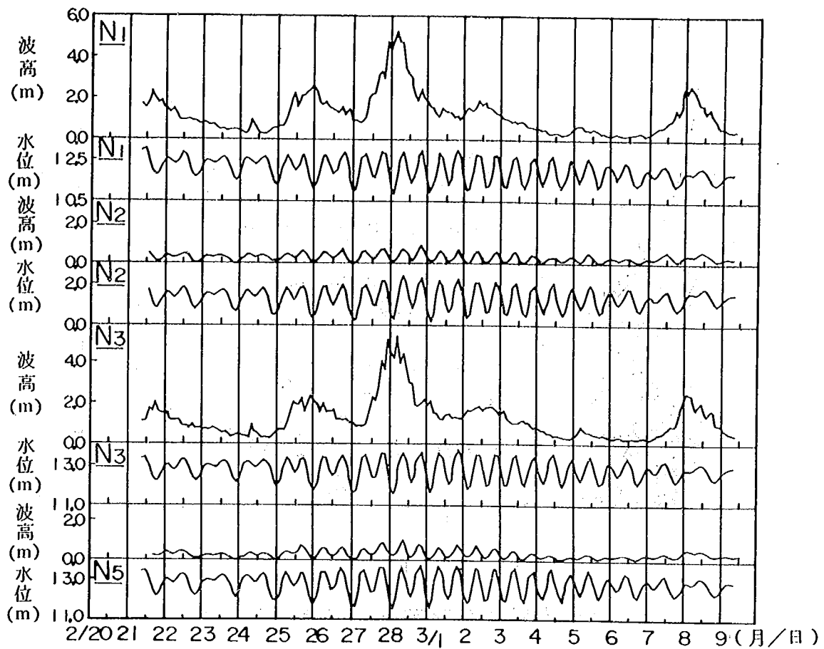
図-3.2 N1, N2, N3, N5地点の波高と水位の経時変化
