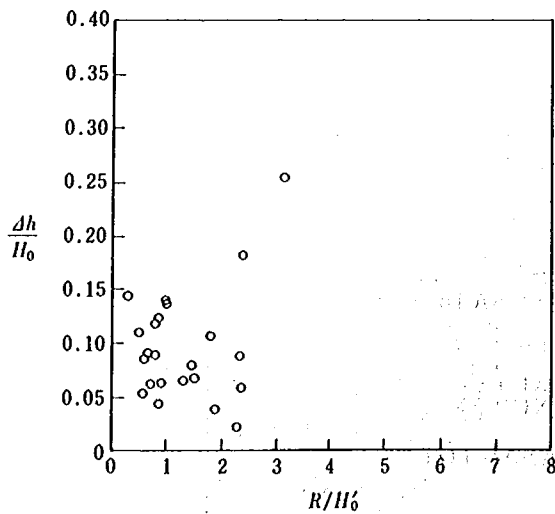
図-3.18 Wave Set-up と波高リーフ上水深比の関係
