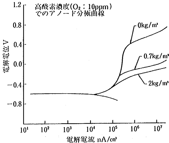
図-6・3 鉄筋のアノード分極特性測定結果 (高酸素濃度の場合)
