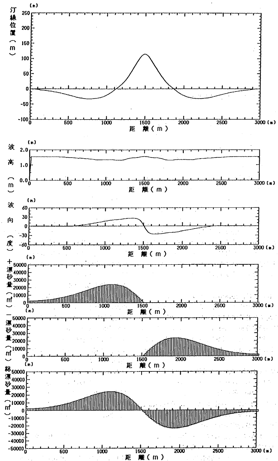
図-5.6 幅広いリーフの周りでの汀線変化 (3か月後)
