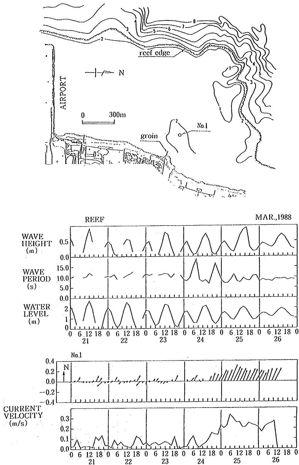
図-4.7 Kuta 海岸における流速の経時変化
