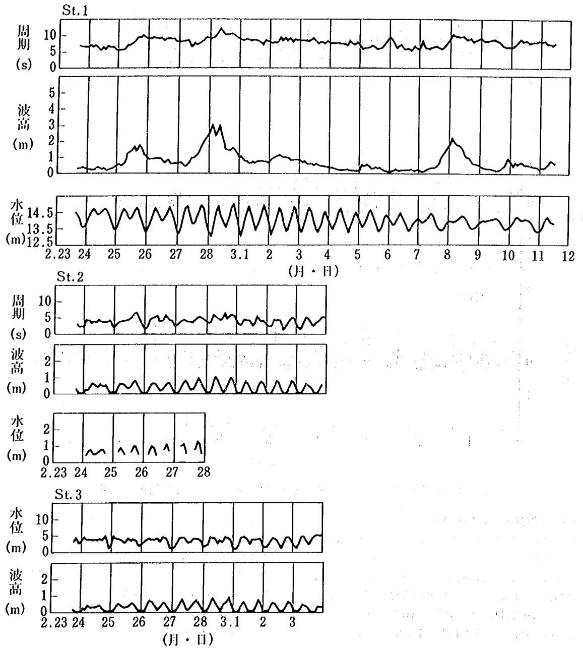
図-3.10 St. 1, 2, 3における周期, 波高, 水位の時間的変化
