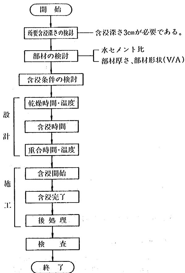
図-5・11 ポリマー含浸防食の設計・施工手順
