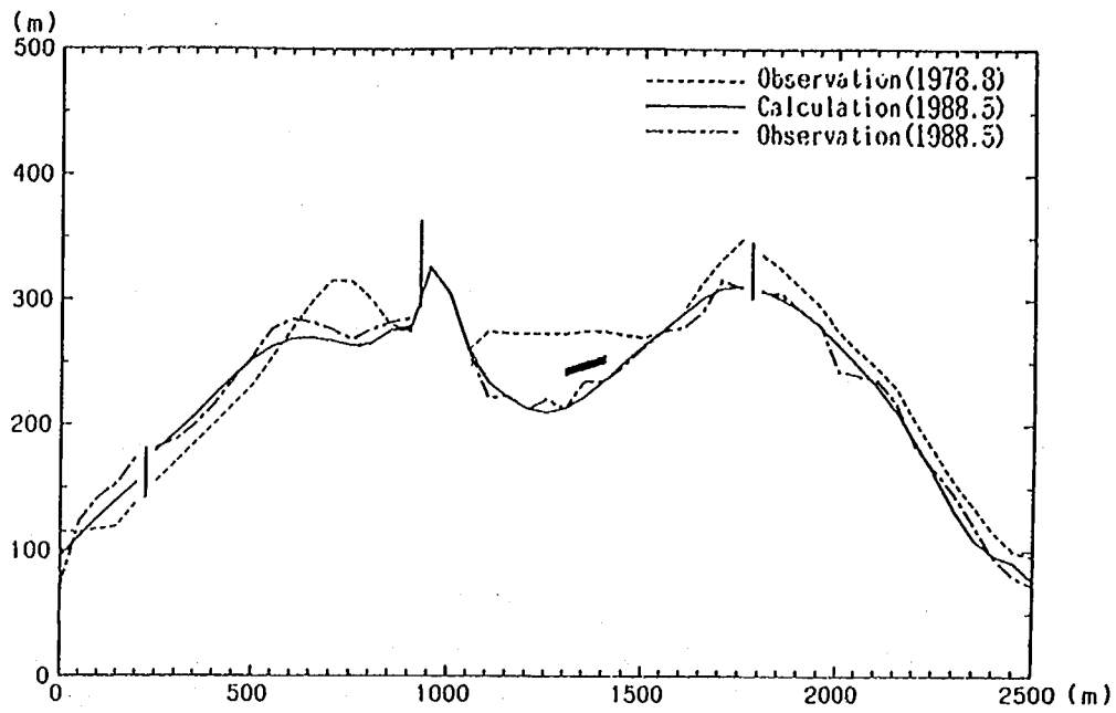
図-5.11 実測と計算による汀線形の比較
