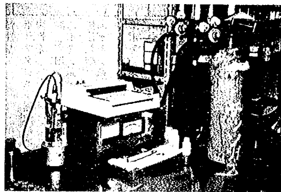
写真-4・2 塗膜の酸素透過量試験方法
