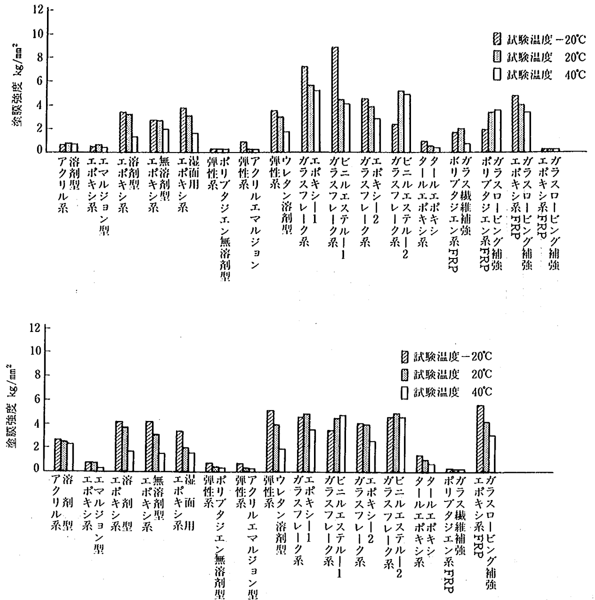
図-4.3 塗膜の強度試験結果
