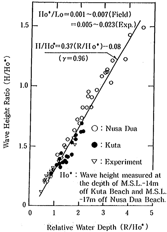
図-3.40 リーフ内外の波高変化と相対水深との関係
