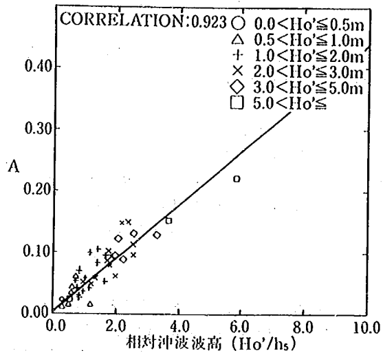
図-3.54 A と相対沖波波高 ( H_o'/h_s ) の関係
