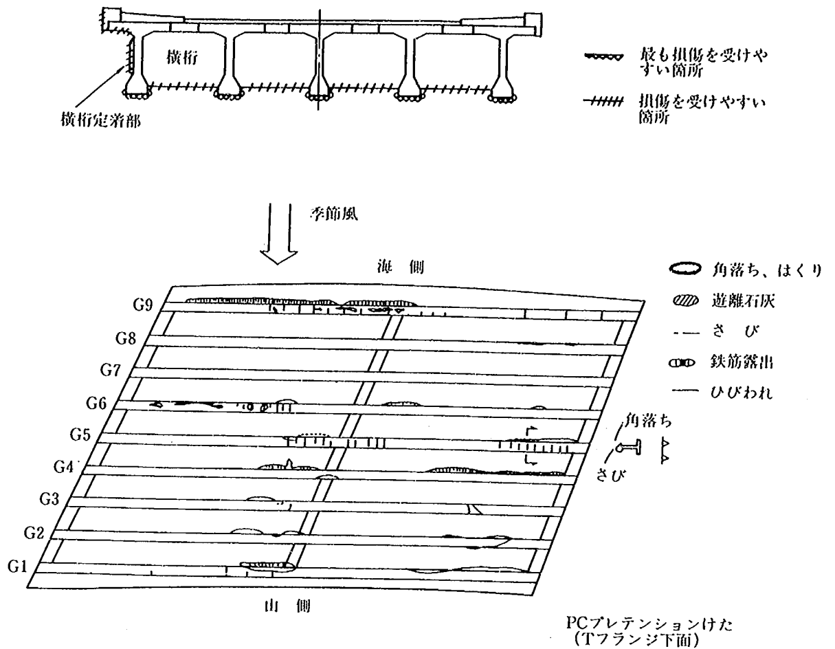
図-3-1 塩害によるコンクリート橋の損傷例
