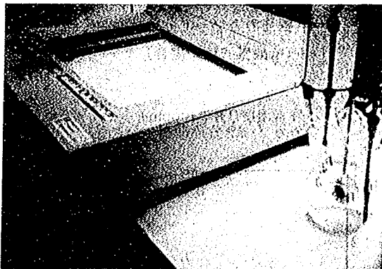
写真-6・1 コンクリート中鉄筋の分極特性測定方法
