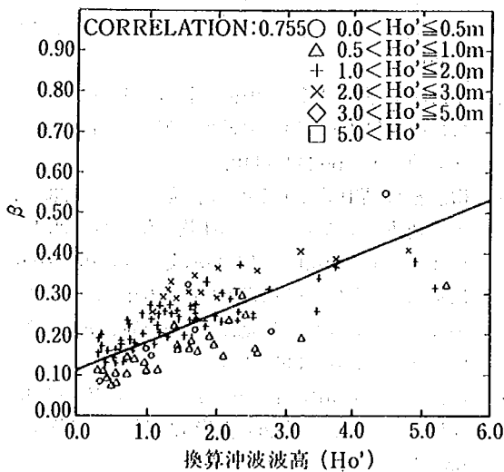
図-3.53 \beta と換算沖波波高 ( H_o' ) の関係
