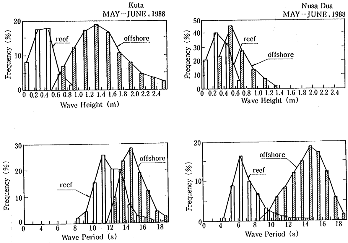
図-3.33 Kuta および Nusa Dua 海岸における有義波高・周期の分布
