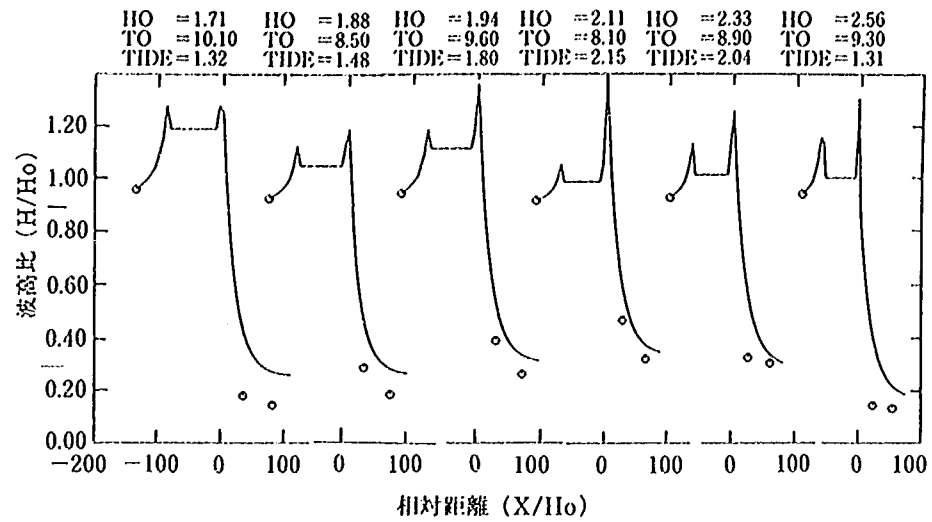
図-3.49 大宜味地区の測線上における波高変化の比較(3)
