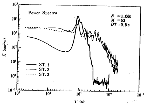
図-3.12 波形のパワースペクトル(1987年2月28日8時)
