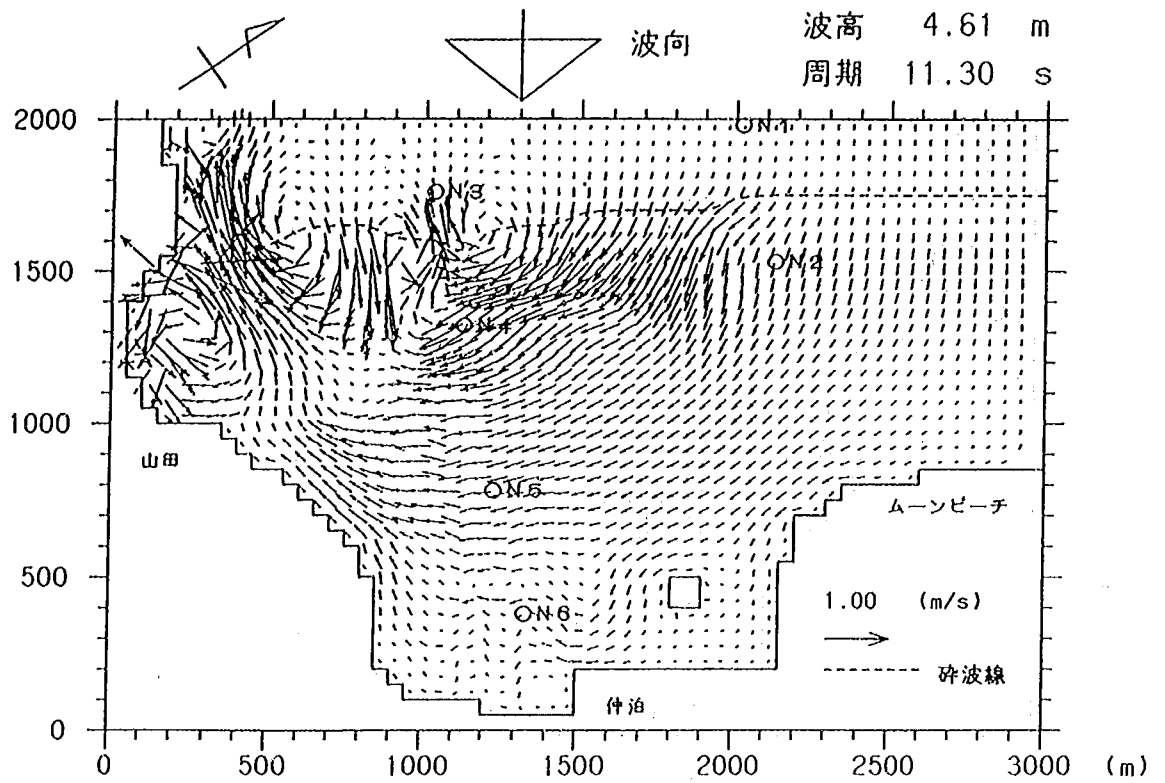
図-4.23 海浜流の流況 (ケース 1, H_1=4.61\text{ m} , T_1=11.3\text{ s} )
