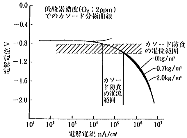
図-6・4 鉄筋のカソード分極特性測定結果 (低酸素濃度の場合)
