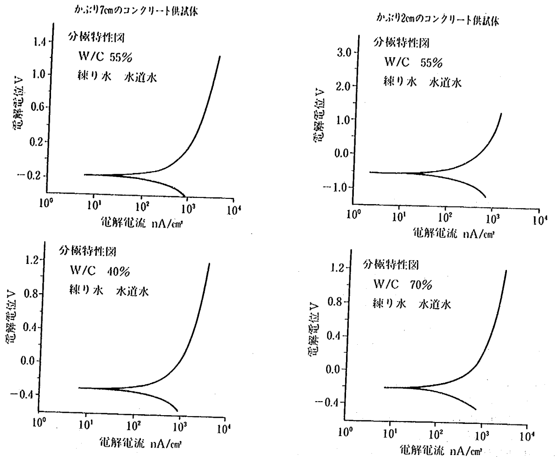
図-6.6 コンクリート中鉄筋の分極特性測定結果
