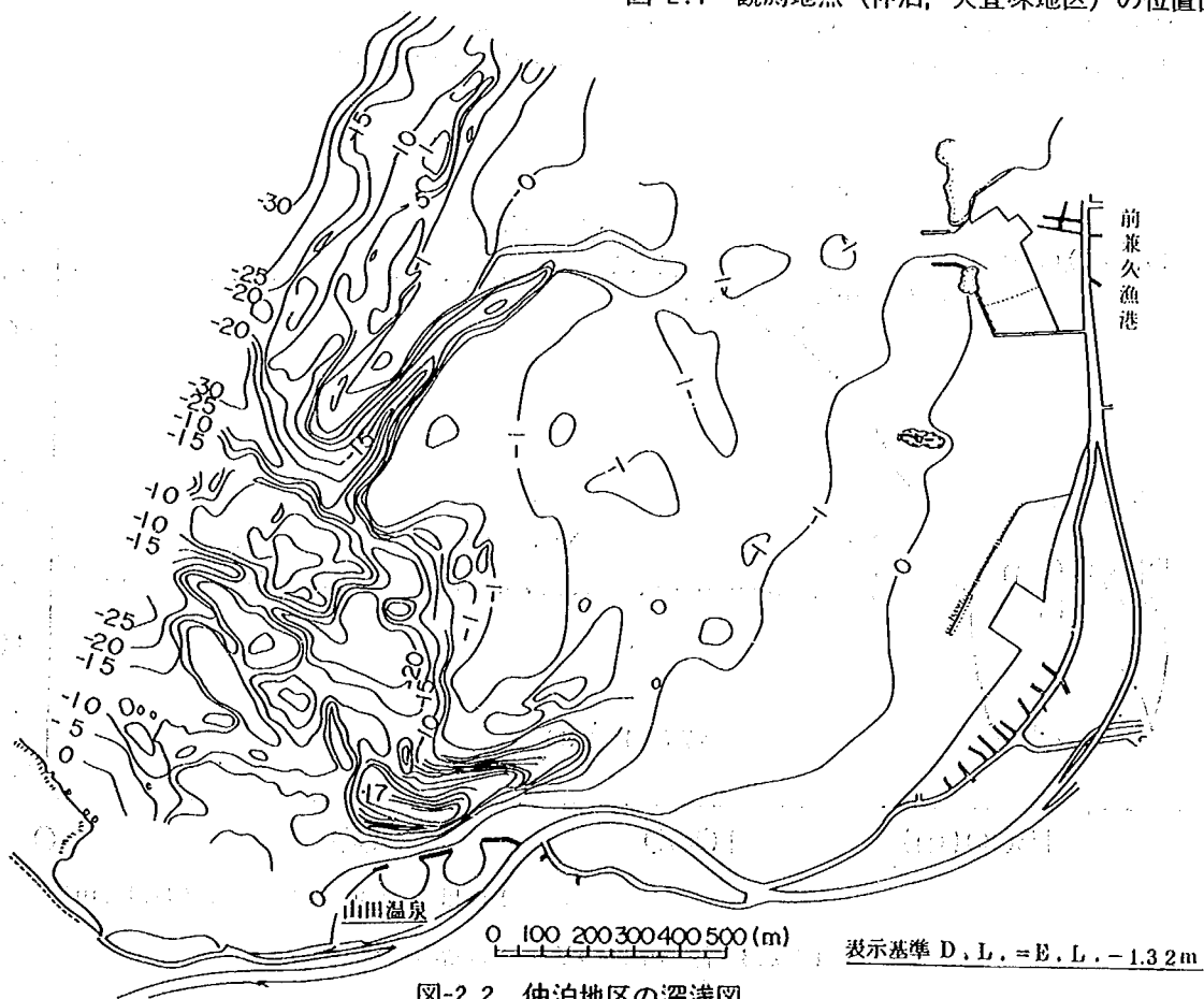
図-2.2 仲泊地区の深浅図
