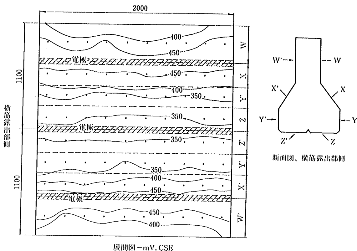
図-6・11 コンクリート供試体の電位分布測定結果 (その2)
