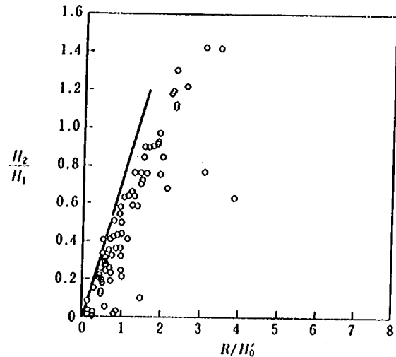
図-3.13 波高伝達率と波高リーフ上水深比の関係 (St. 2)
