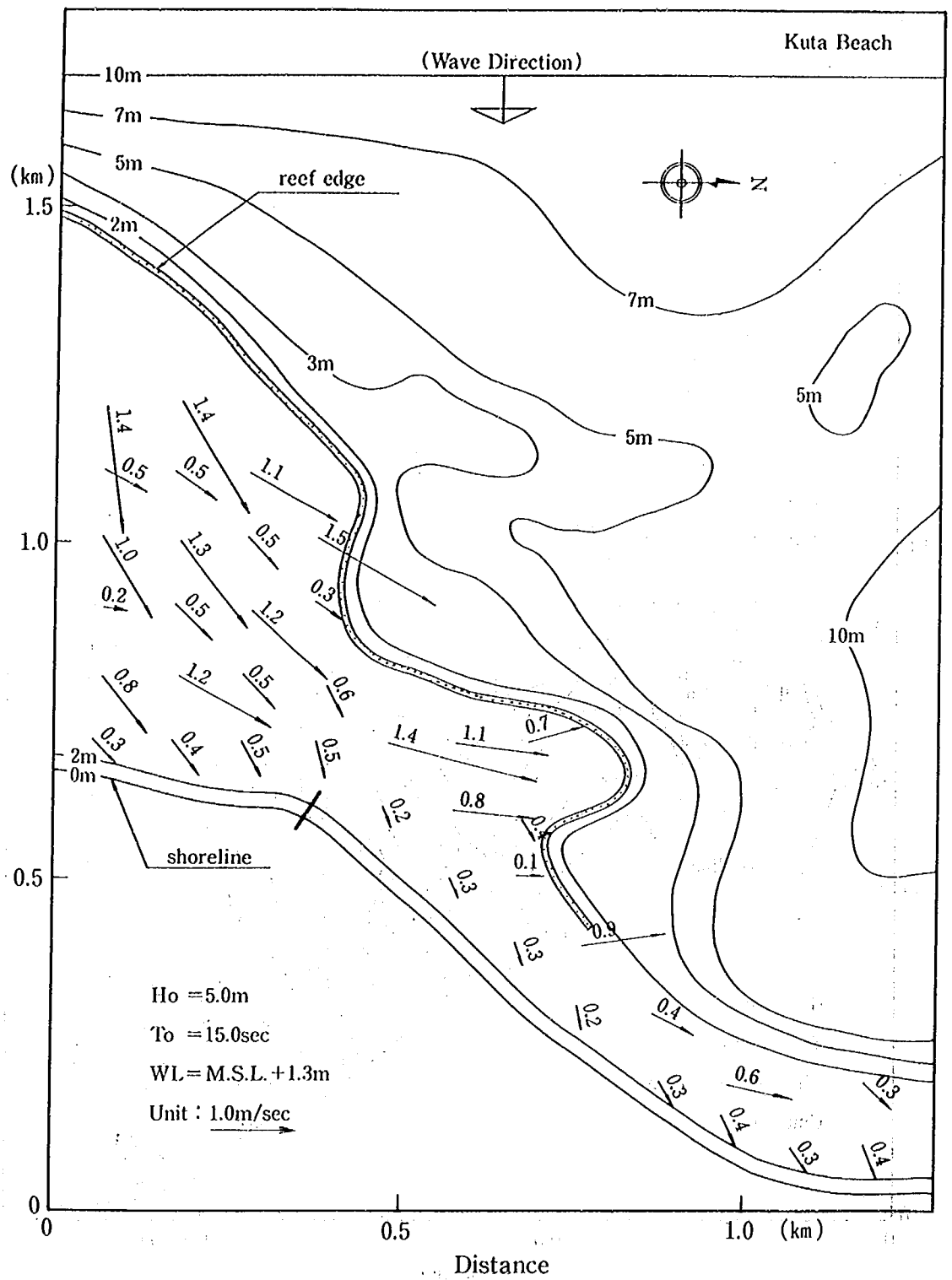
図-4.14 海浜流の流況 (Kuta 海岸)
