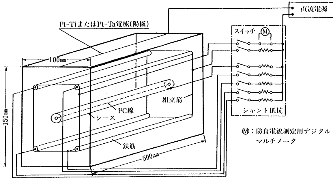
図-6・7 電気防食の効果に関する実験方法
