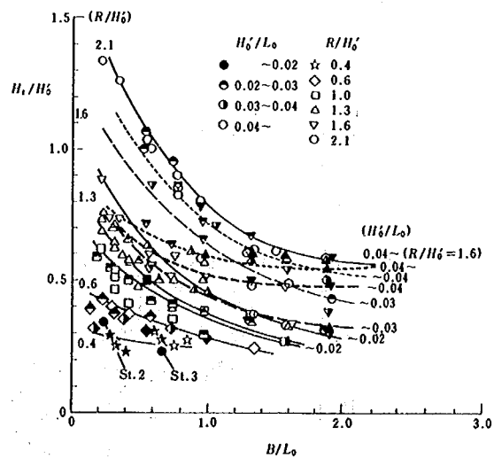
図-3.19 人工リーフの波高低減率と天然リーフ上での実測値との比較
