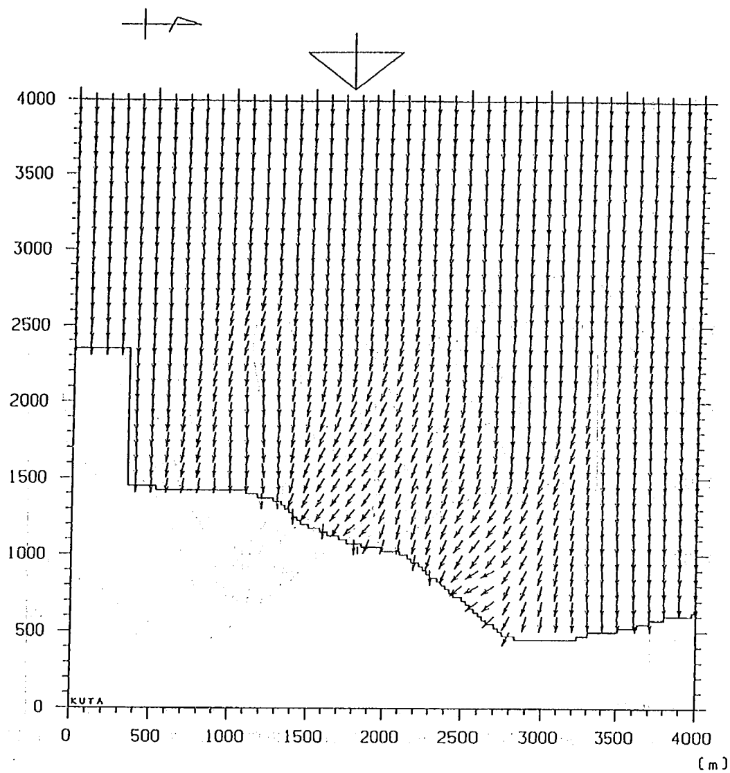
図-5.9 Kuta 海岸の波向分布 (入射方向W)
