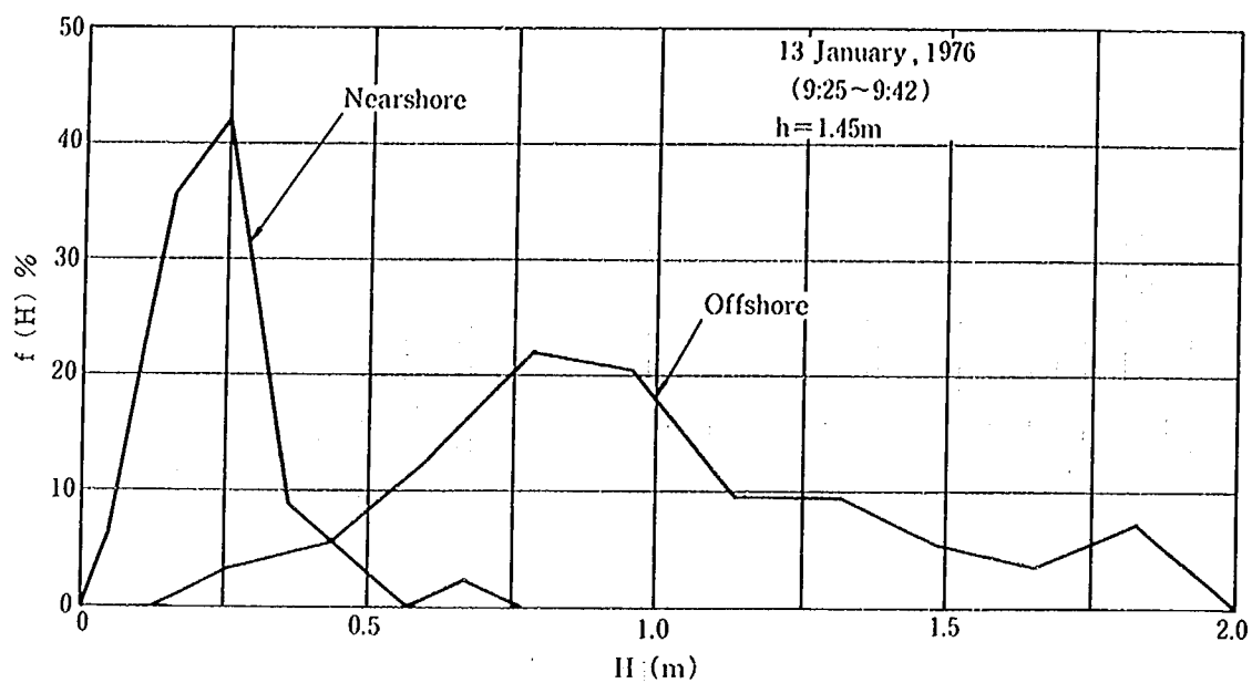
図-3.34 Kuta 海岸におけるリーフ内外の有義波高・周期の分布 (その1) (Tsuchiya et al., 1976)
