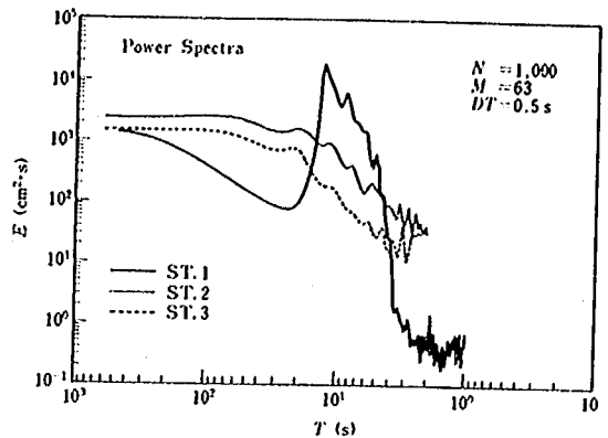
図-3.11 波形のパワースペクトル(1987年2月28日4時)
