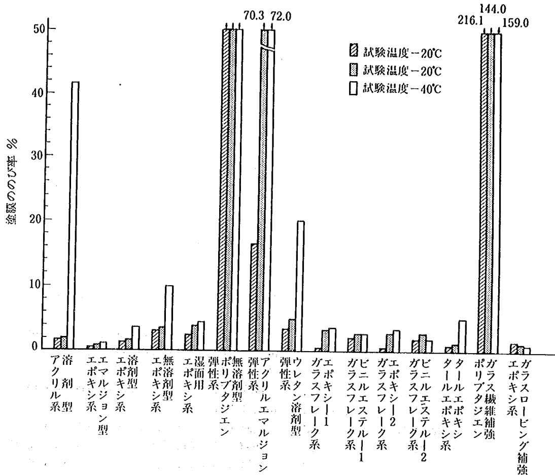
図-4.4 塗膜の伸び率試験結果
