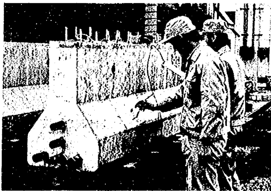
写真-6・2 コンクリート供試体の電位分布及び電流密度の測定
