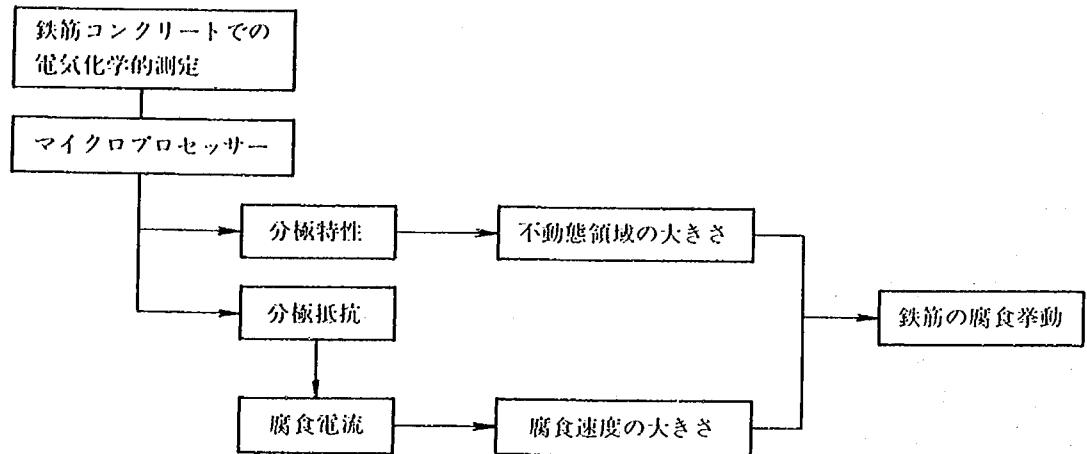
図-6・1 鉄筋の腐食挙動を知るための電気化学的測定方法
