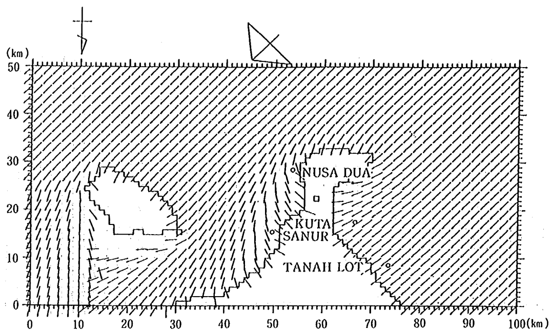
図-2.23 バリ島海岸の屈折図（入射方向 SW）
