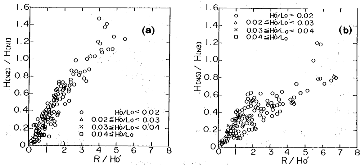
図-3.3 波高伝達率と R/H_0 の関係
