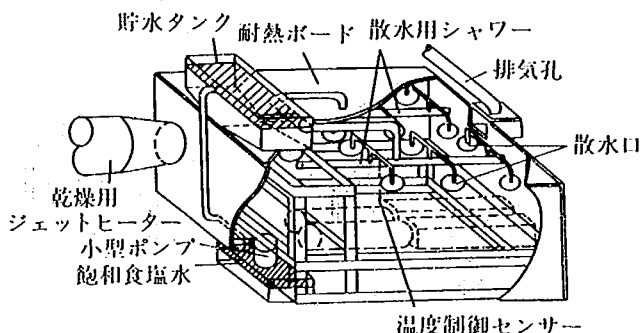
図-5・1 乾燥・湿潤繰り返し腐食促進試験装置
