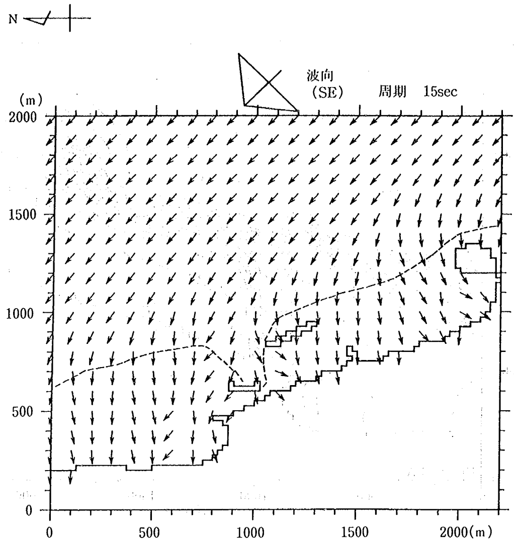
図-3.28 Nusa Dua 海岸の屈折図
