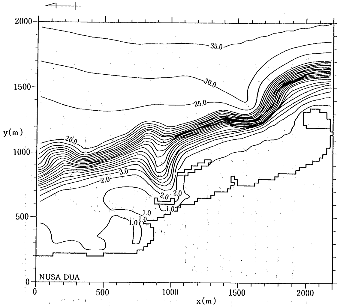
図-3.27 Nusa Dua 海岸の海底地形
