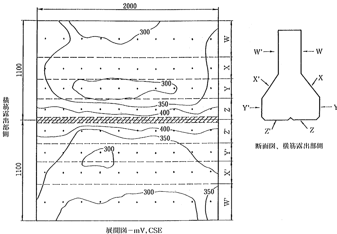
図-6・13 コンクリート供試体の電位分布測定結果 (その4)
