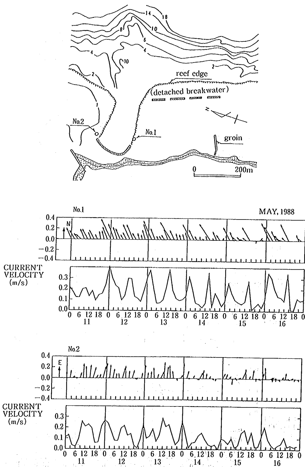
図-4.8 Nusa Dua 海岸における流速の経時変化
