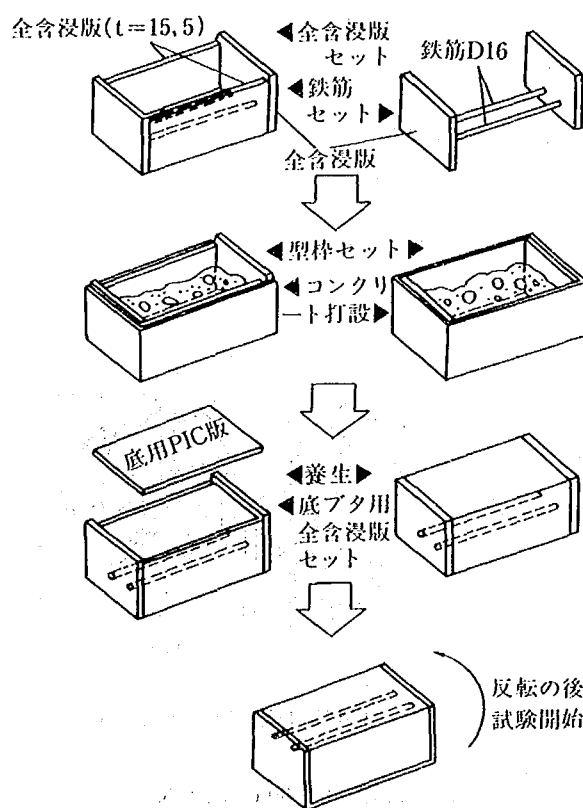
図-5・2 ポリマー含浸防食試験体の製作手順
