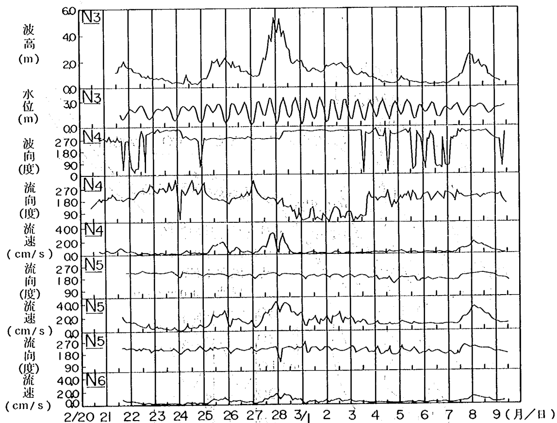
図-4.2 N3~N6地点の波高、波向、流速の経時変化
