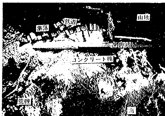
写真-3・2 塩害を受けた構造部材例
