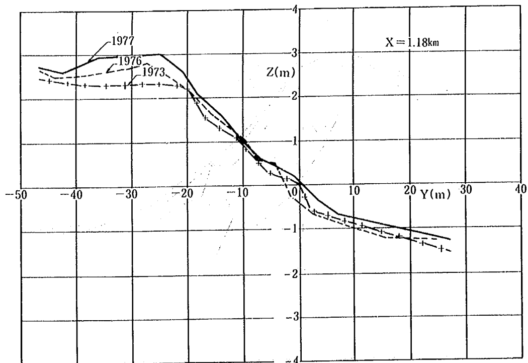
図-2.16 Sanur 海岸の X = 1.18\text{km} 地点における海浜断面形の変化 (Tsuchiya, 1978)
