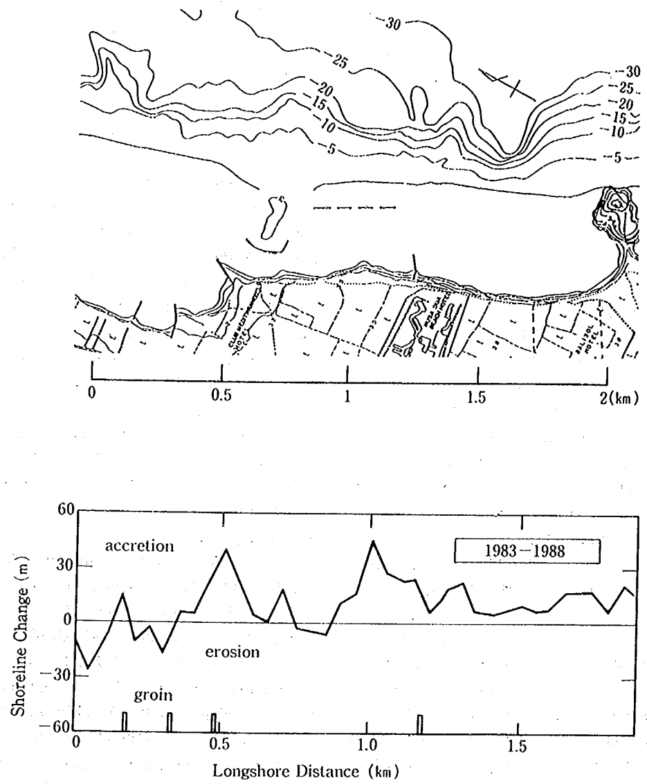
図-2.12 Nusa Dua 海岸における汀線変化
