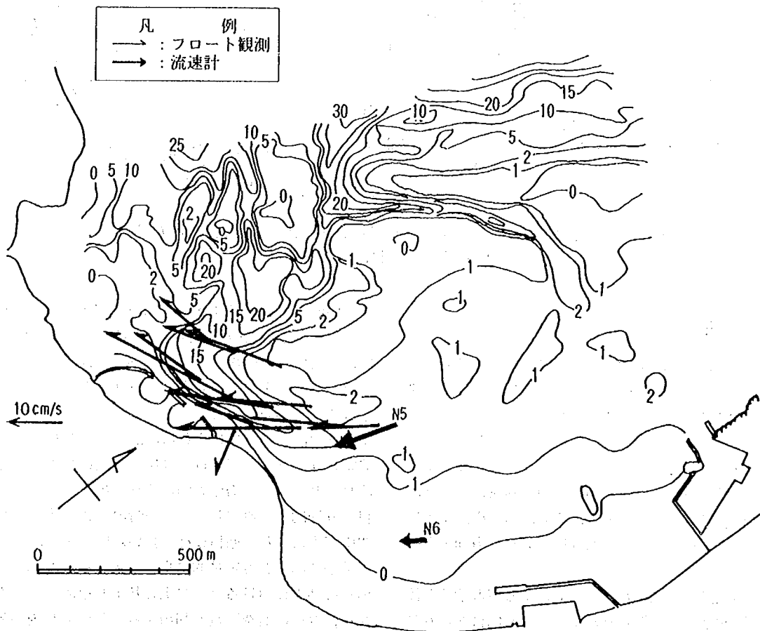
図-4.25 流速計およびフロートを用いた観測によって得られた流況 (1987年3月3日, 10:00観測)
