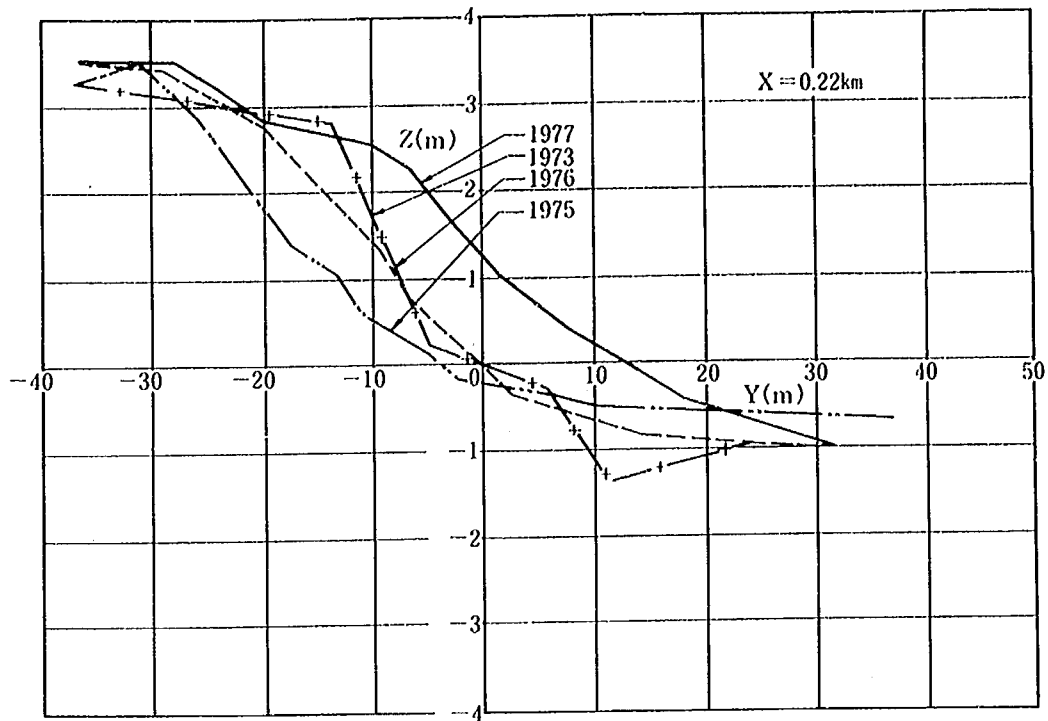
図-2.15 Sanur 海岸の X = 0.22\text{km} 地点における海浜断面形の変化 (Tsuchiya, 1978)
