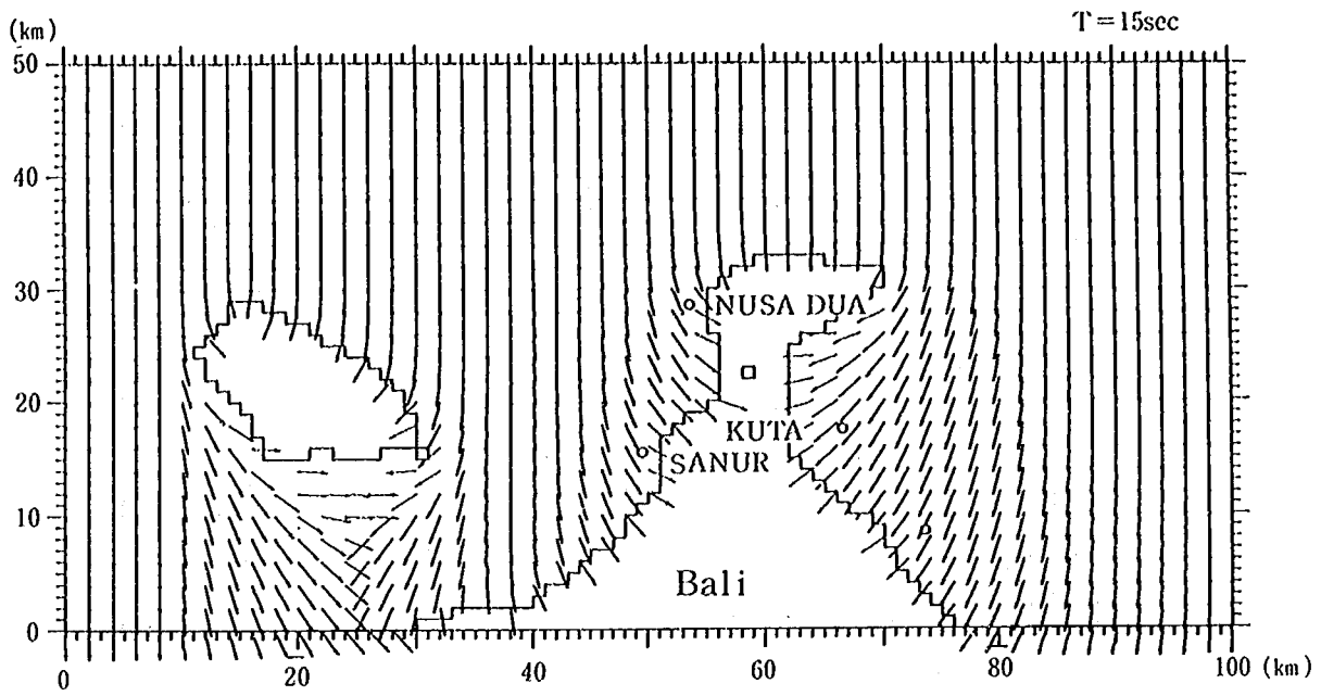
図-3.21 バリ島海岸の屈折図 (入射方向 S)
