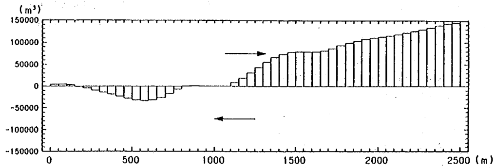
図-5.12 1978年～1988年の総沿岸漂砂量の沿岸分布
