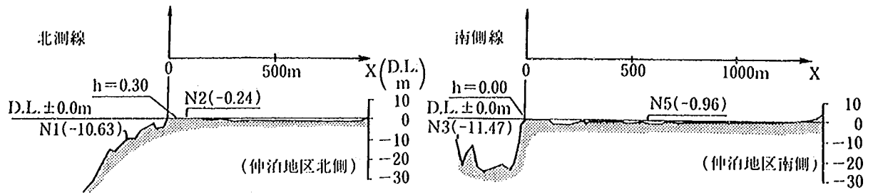
図-3.43 仲泊地区の南北測線上での座標軸の設定
