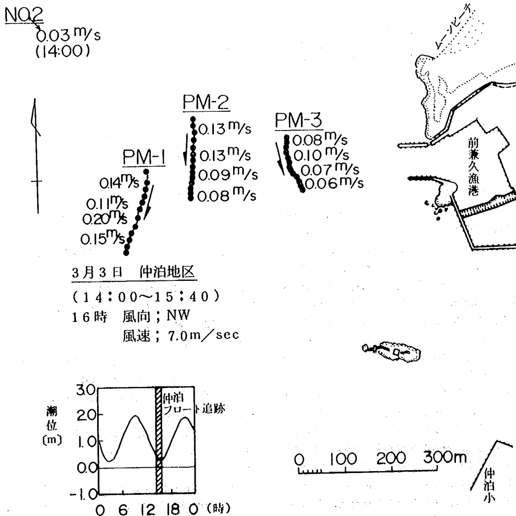
図-4.5 フロート追跡による流速測定 (前兼久漁港沖)
