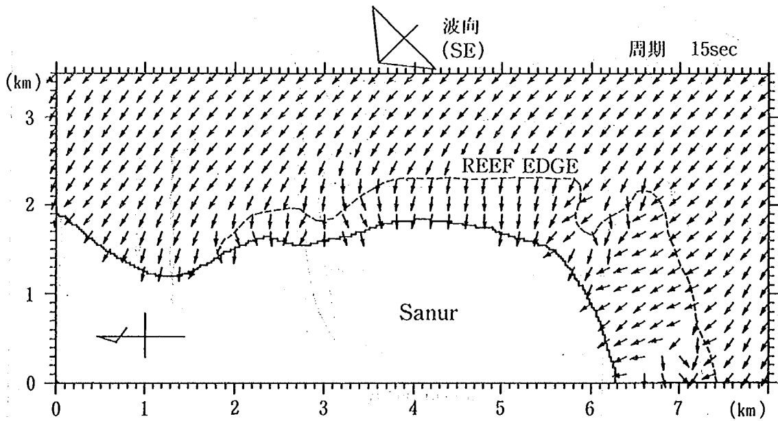
図-3.30 Sanur 海岸の屈折図
