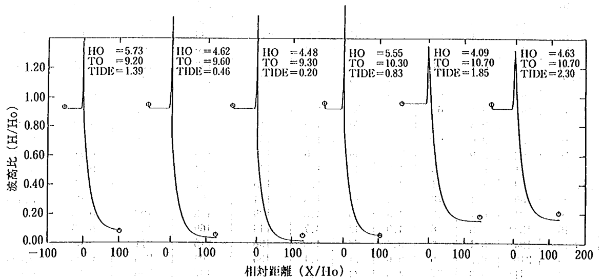
図-3.45 仲泊地区の南測線上における波高変化の比較
