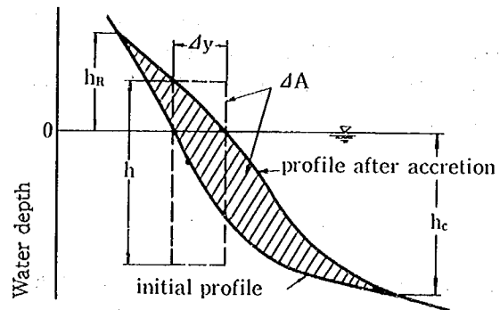
図-2.21 漂砂の移動高の定義図
