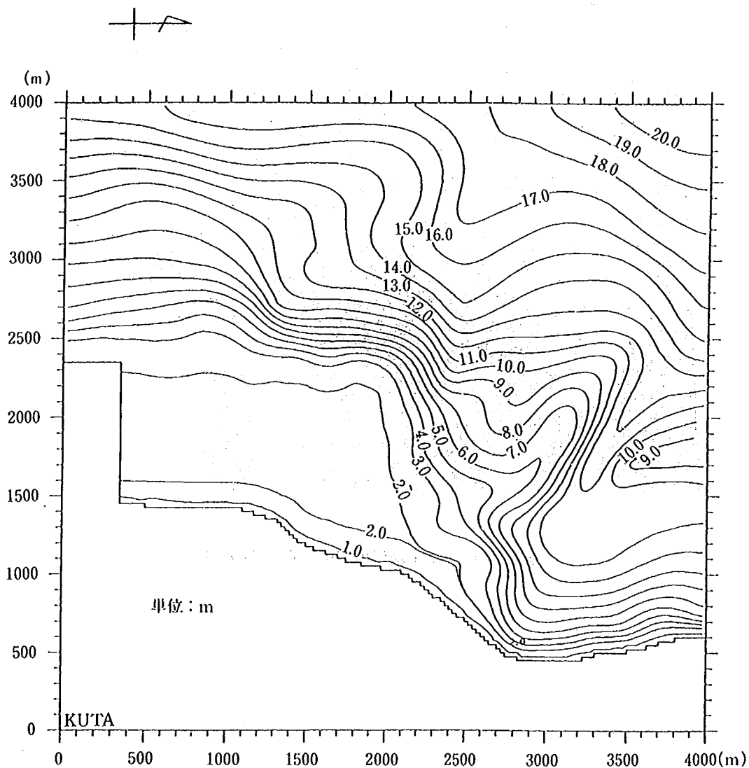
図-3.25 Kuta 海岸の海底地形
