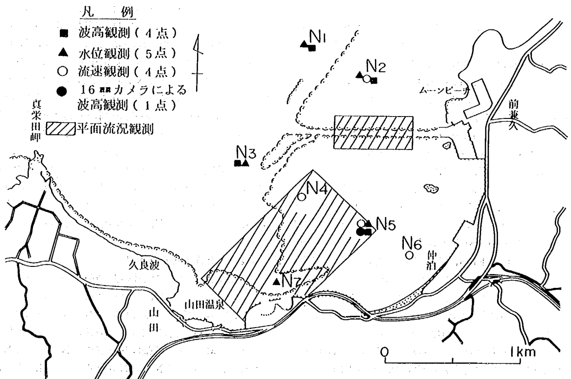
図-3.1 仲泊地区における観測点の配置
