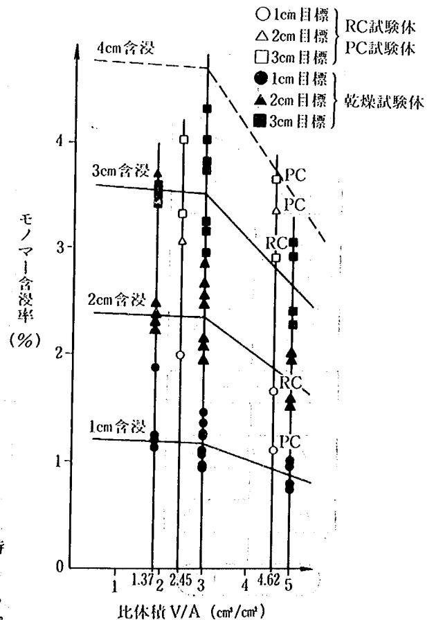
図-5.10 モノマー含浸率と比表面積との関係
