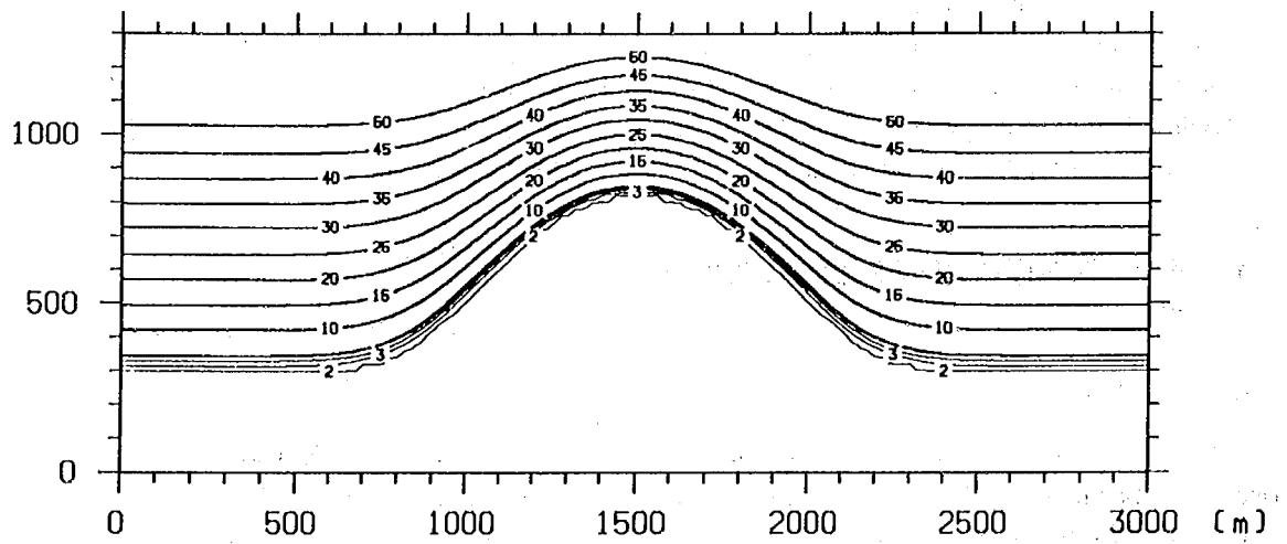
図-5.2 幅広いリーフのモデル地形
