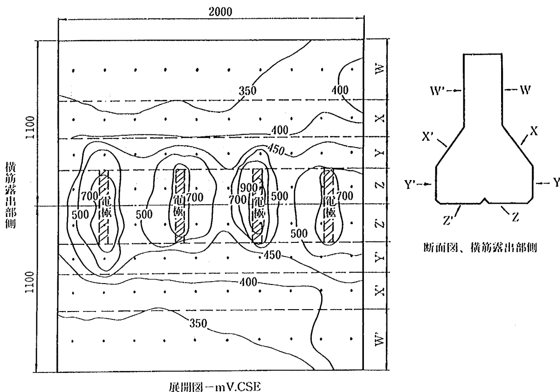
図-6-12 コンクリート供試体の電位分布測定結果 (その3)
