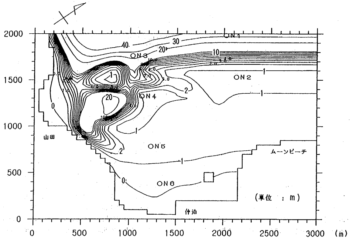
図-4.20 計算に用いたリーフ周辺の海底地形
