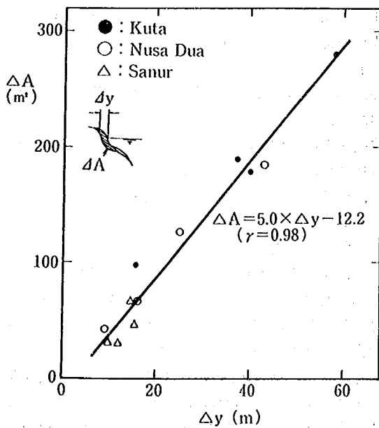
図-2.20 断面積変化量と汀線変化量との関係
