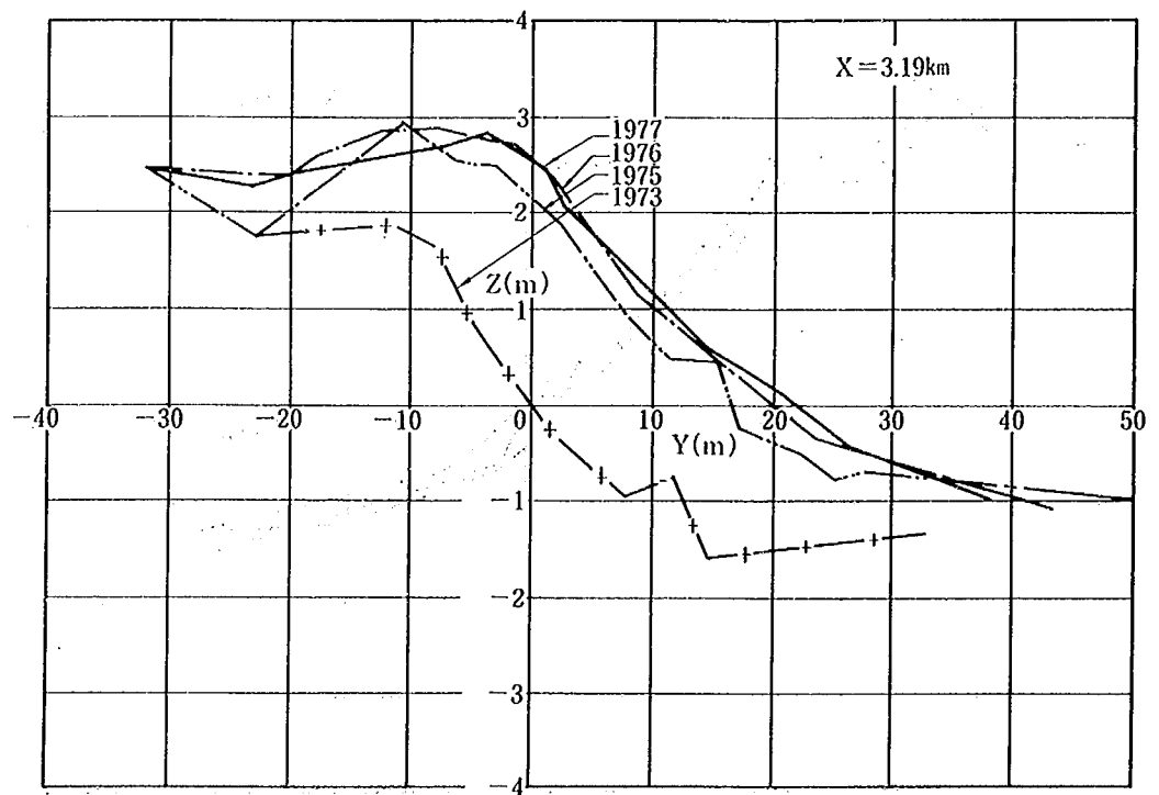
図-2.18 Sanur 海岸の X = 3.18\text{ km} 地点における海浜断面形の変化 (Tsuchiya, 1978)
