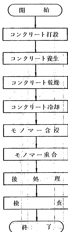
図-5・6 ポリマー含浸コンクリート試験体の製作手順
