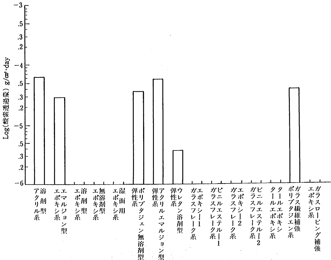
図-4.2 塗膜の酸素量透過量試験結果
