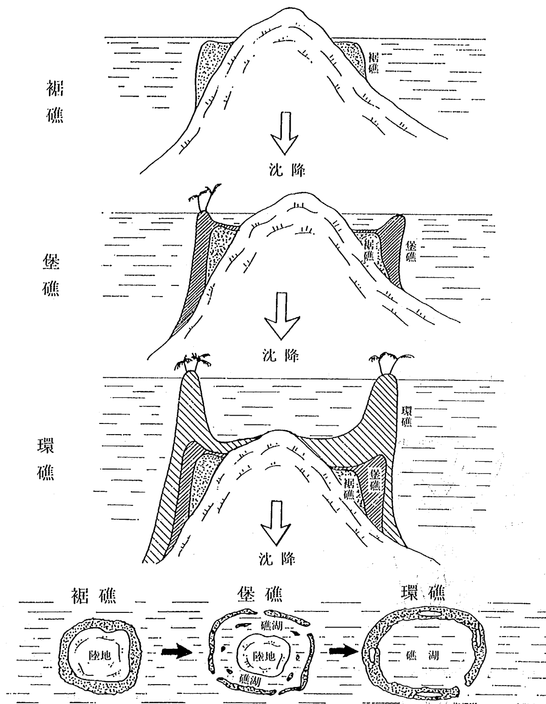
図-1.2 サンゴ礁の形と成因 (白井・佐野, 1985)
