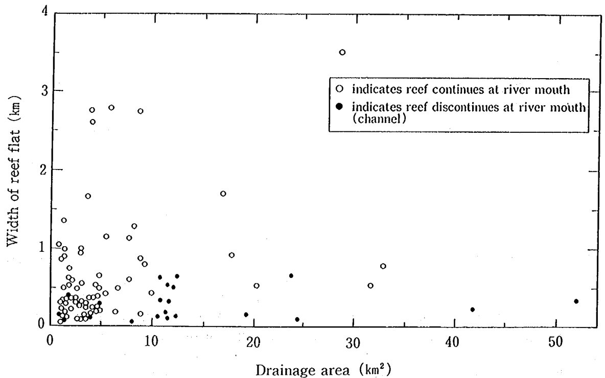
図-1.6 河川流域面積と礁原幅との関係（目崎ほか，1977）
