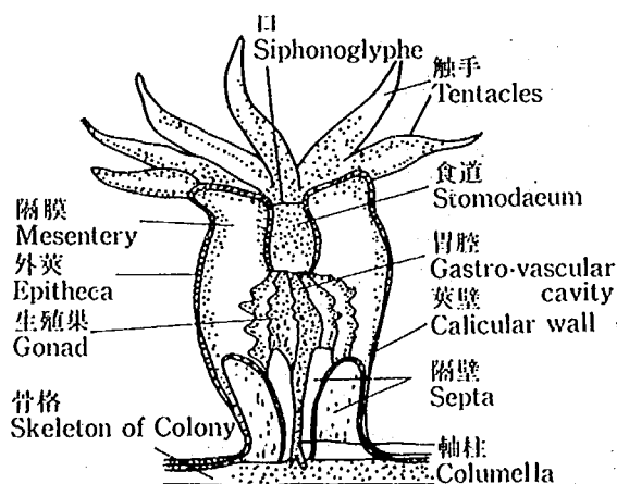
図-1.1 サンゴ虫の構造 (白井・佐野, 1985)
