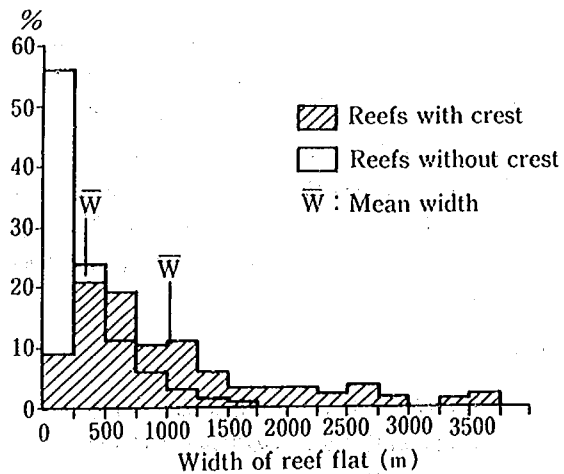
図-1.5 crestの有無とリーフ幅の関係(目崎ほか, 1977)
