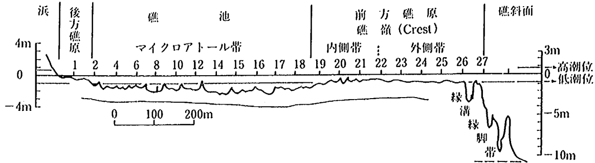
図-1.3 石垣島川平のサンゴ礁断面と地形区分 (高橋, 1988)
