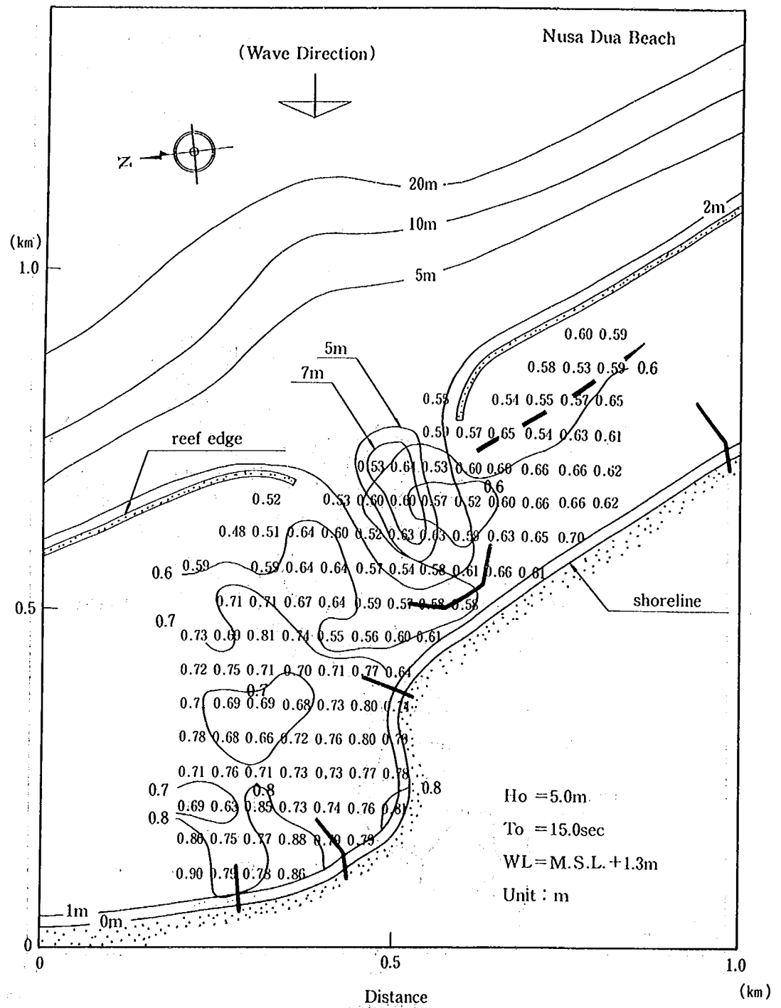
図-4.16 平均水位の平面分布 (Nusa Dua 海岸)
