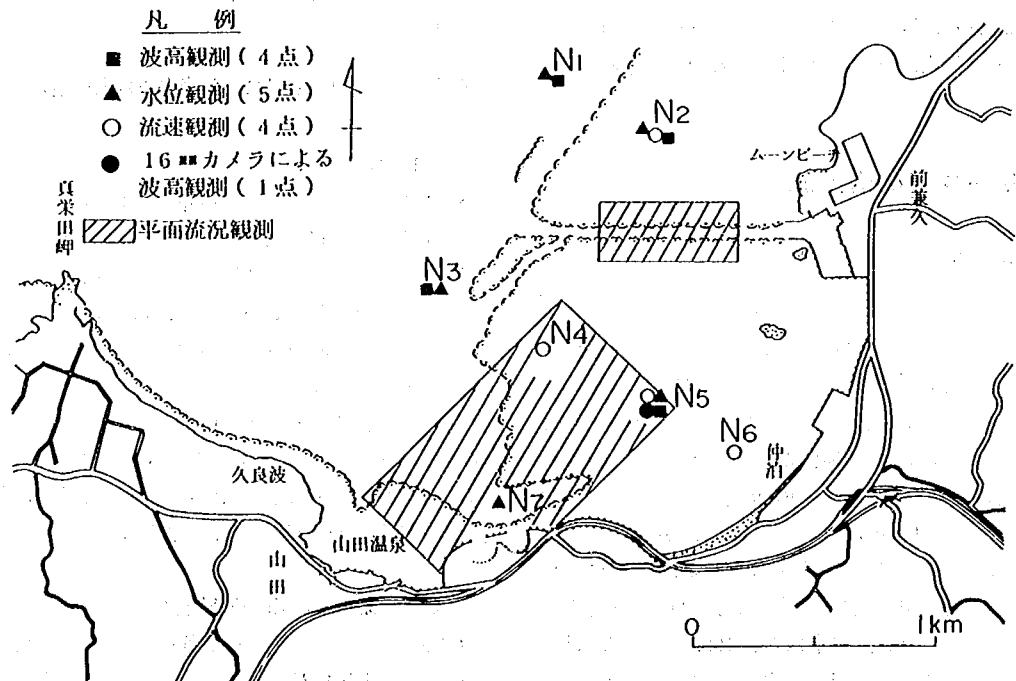
図-4.1 仲泊地区における波高、水位、流速の観測点の配置
