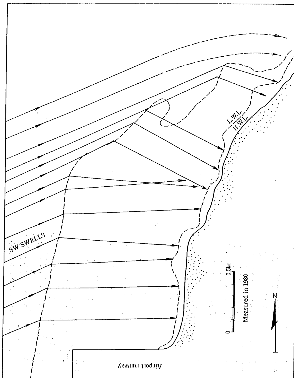
図-3.31 Kuta 海岸の屈折図 (Tsuchiya, 1987)
