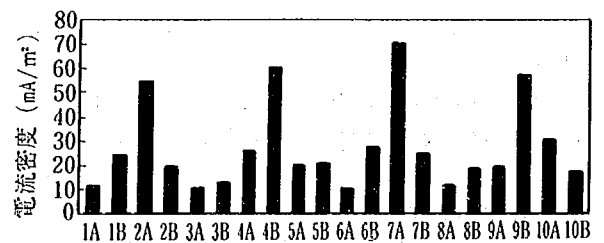
図-6・15 コンクリート供試体の電流密度測定結果
