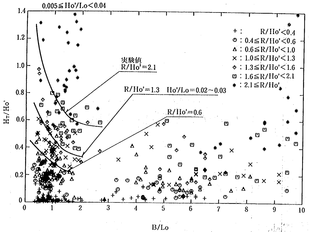
図-3.4 人工リーフの波高伝達率と現地データとの比較
