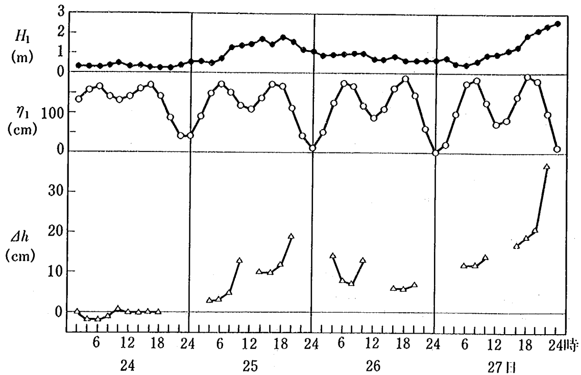
図-3.17 St. 1 の早位を基準とした水位差の変動
