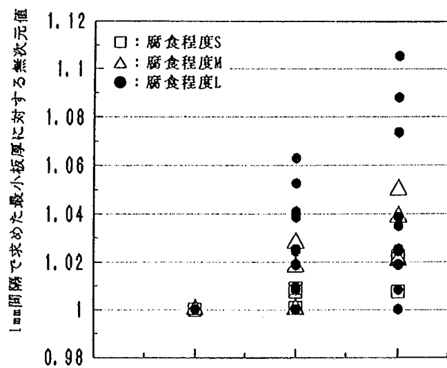
(c) 最小板厚
