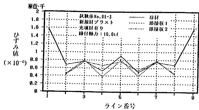
試験体 No.D1-3 (39.9tf 時)
