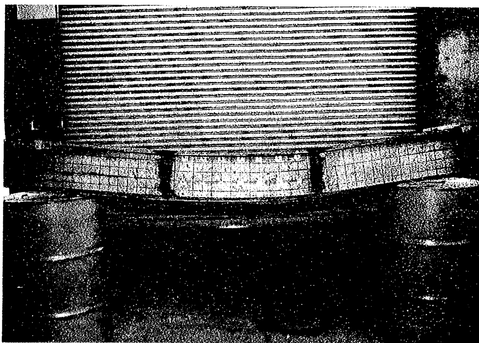
写真-1.3.5(d) 試験後の状況 (試験体No.5)
