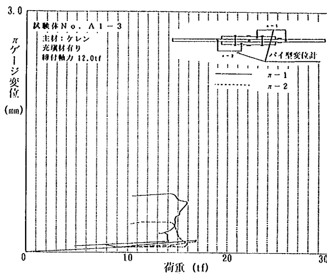
試験体 No. A1-3
