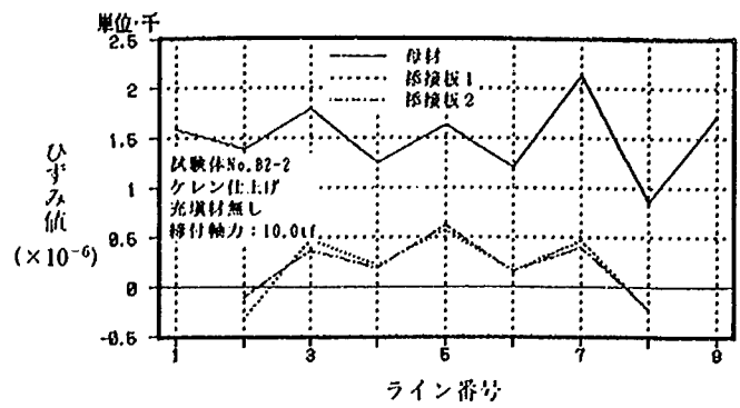
試験体 No. B2-2 (39.9tf 時)
