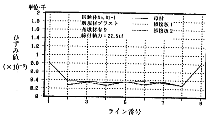
試験体 No. D1-1 (20.1tf 時)
