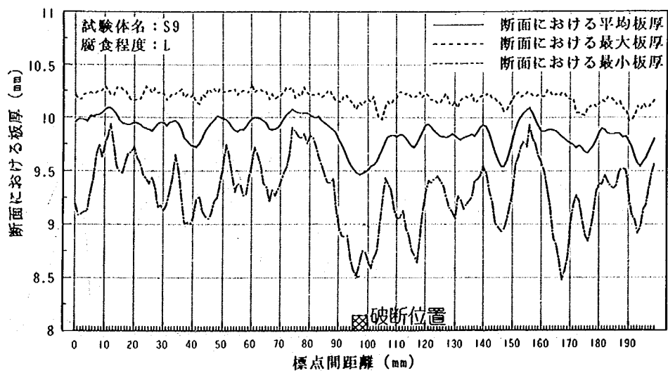
図-1.2.6(c) 板厚測定結果と破断位置の関係
