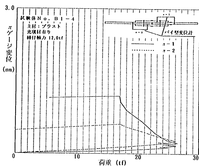
試験体 No. B1-4
