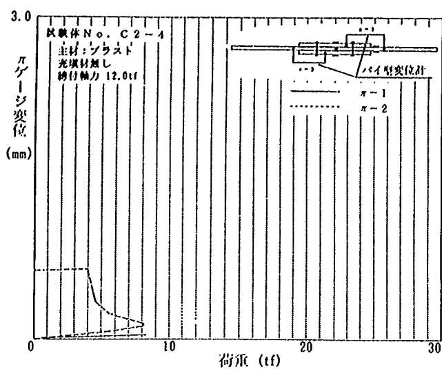
試験体 No. C2-4
