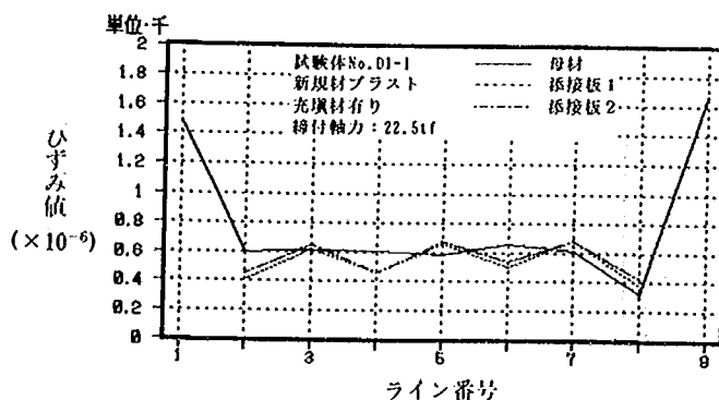
試験体 No. D1-1 (33.1tf 時)
