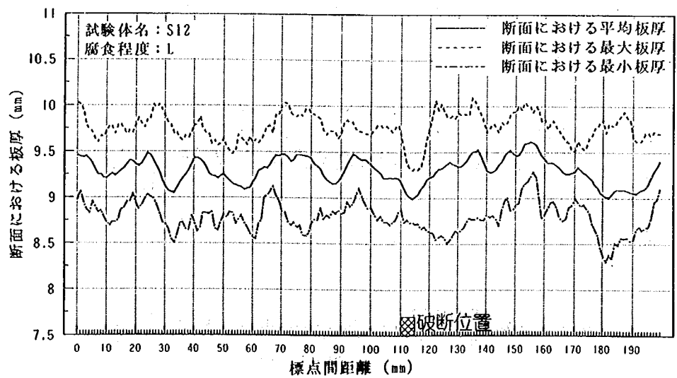
図-1.2.6 (d) 板厚測定結果と破断位置の関係
