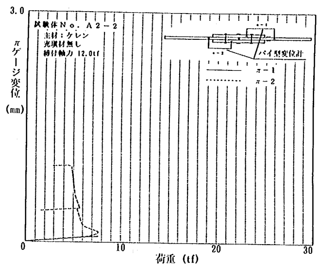
試験体 No. A2-2
