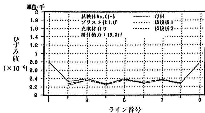
試験体 No.C1-5(20.1tf 時)
