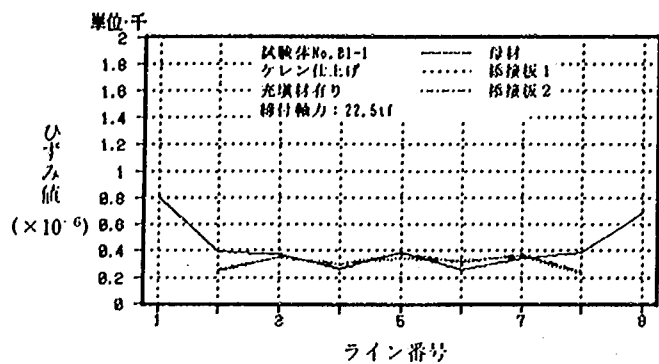
試験体 No.B1-1 (20.0tf 時)
