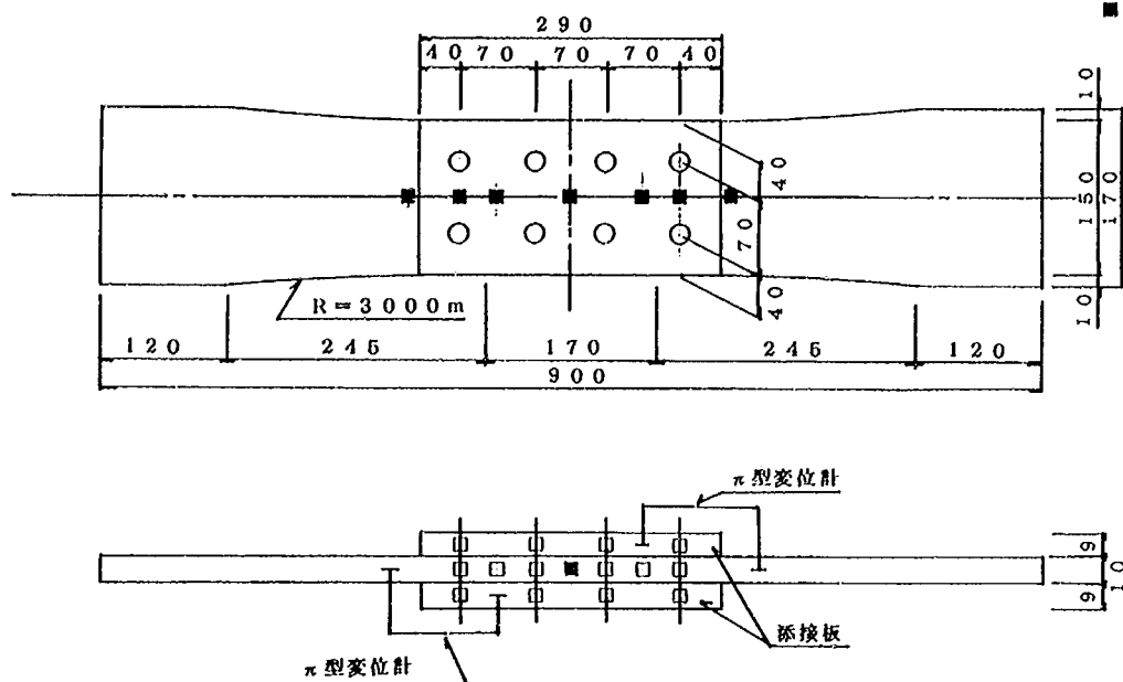
図-2.3.1 試験体の寸法形状およびひずみゲージ測定位置
