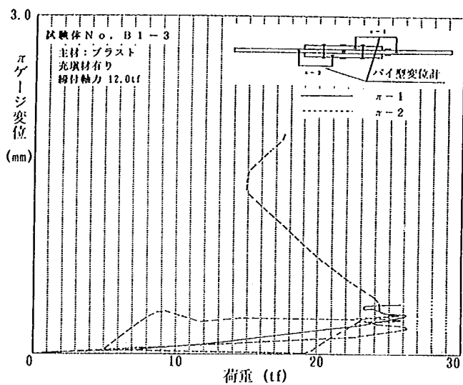
試験体 No. B1-3
