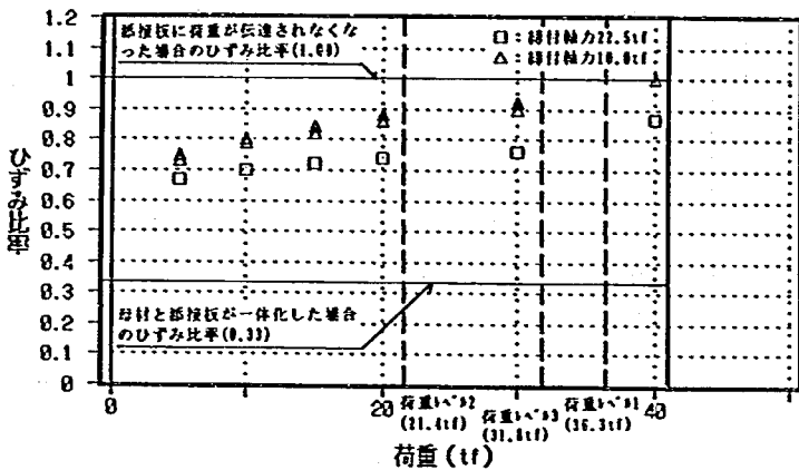
条件：ケレン、充填材無し
