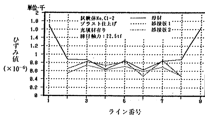
試験体 No. C1-2 (40.1tf 時)
