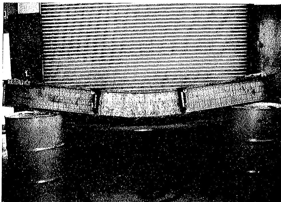
写真-1.3.5(a) 試験後の状況(試験体No.1)
