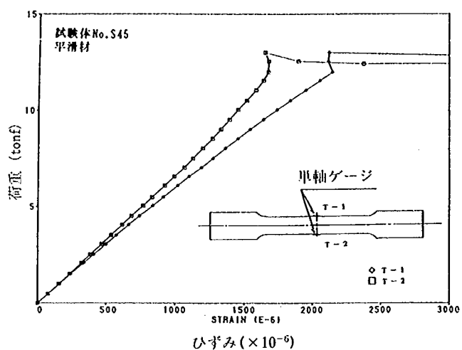
図-1.2.7(e) 板タイプ試験体の荷重-ひずみの関係
