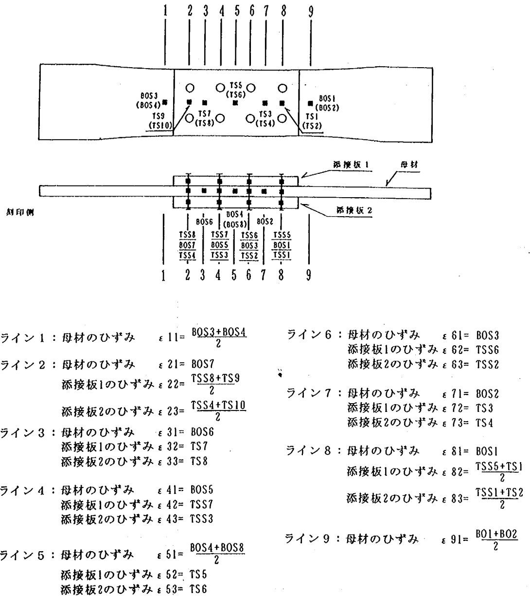
図-2.3.2 各断面のひずみの計算方法
