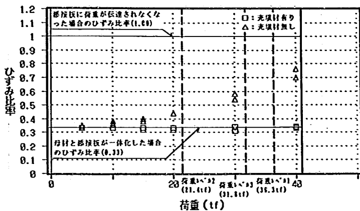
条件：ケレン、締付軸力 10.0tf
