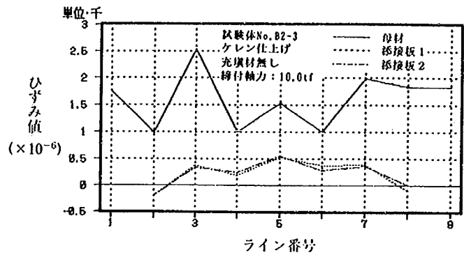
試験体 No. B2-3 (39.0tf 時)
