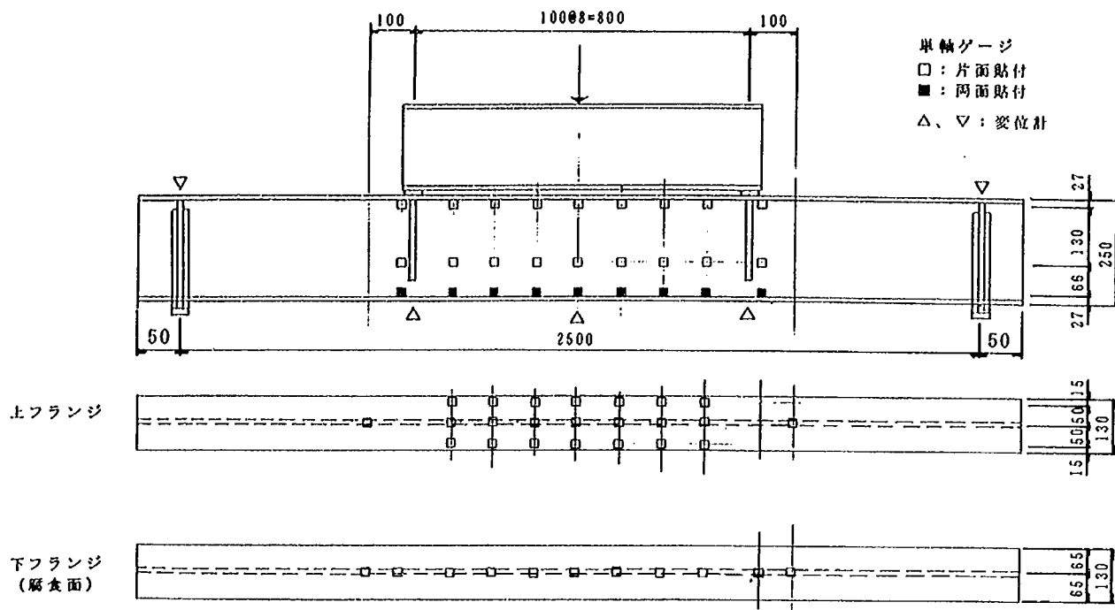
図-1.3.1 桁タイプ試験体の寸法形状、ひずみゲージおよび変位測定位置
