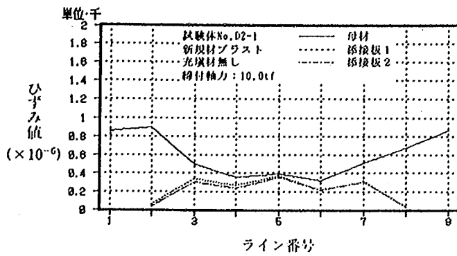
試験体 No.D2-1 (20.0tf 時)
