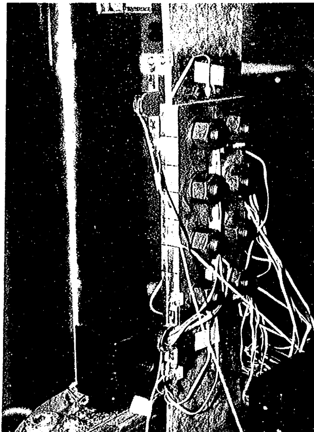
写真-2.3.1 添接板補強試験体の引張試験の状況
