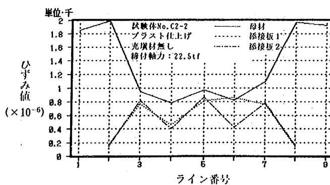
試験体 No.C2-2 (39.9tf 時)
