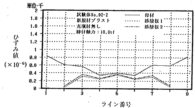
試験体 No.D2-2 (26.9tf 時)
