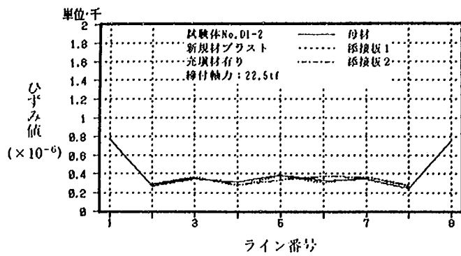
試験体 No.D1-2(20.1tf 時)
