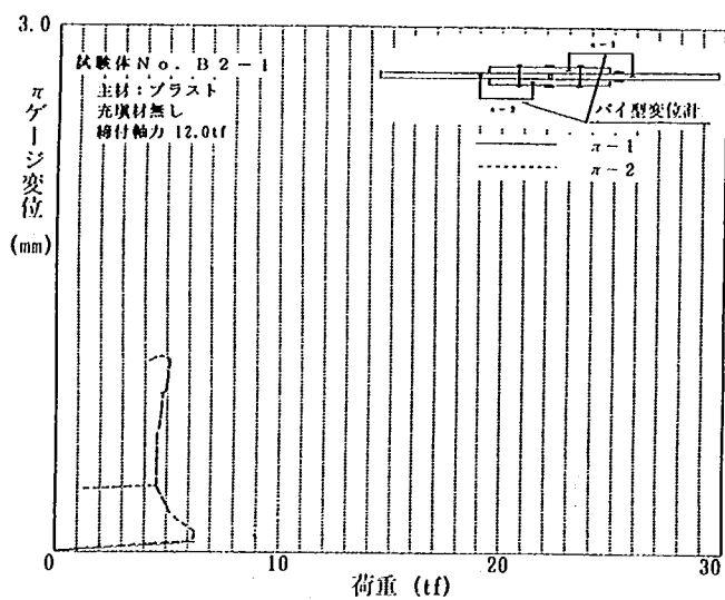
試験体 No. B2-1
