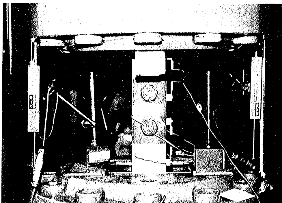
写真-2.2.1 板タイプ試験体のすべり試験の状況
