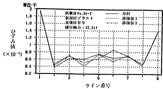
試験体 No.D1-2 (35.1tf 時)
