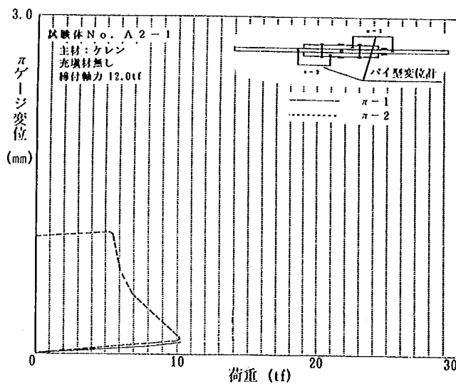
試験体 No. A2-1
