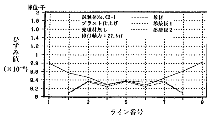
試験体 No.C2-1 (19.8tf 時)
