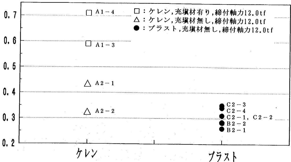
図-2.2.4 接合条件とすべり係数との関係
