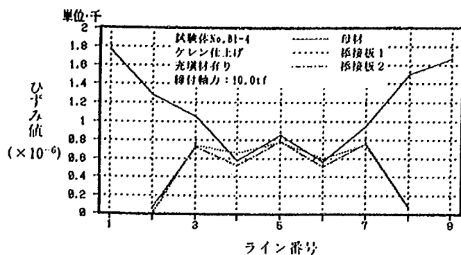
試験体 No. B1-4 (39.9tf 時)
