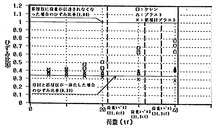
条件：充填材有り、締付軸力 22.5tf
