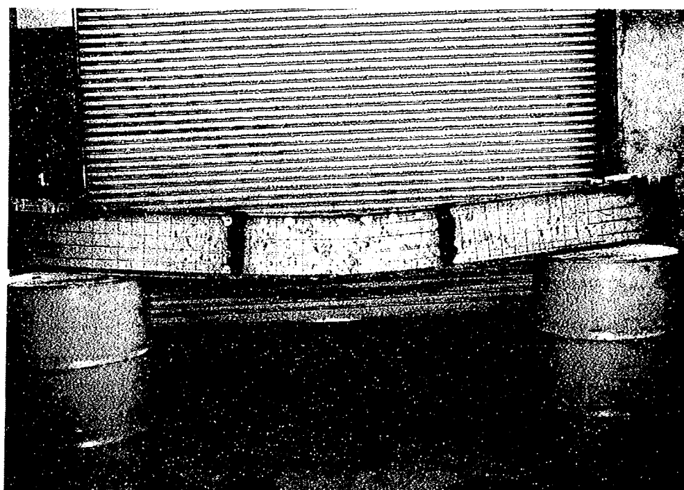
写真-1.3, 5(c) 試験後の状況 (試験体No.4)
