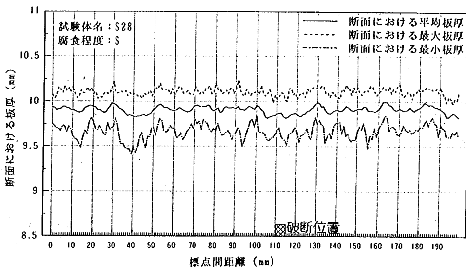
図-1.2.6(f) 板厚測定結果と破断位置の関係
