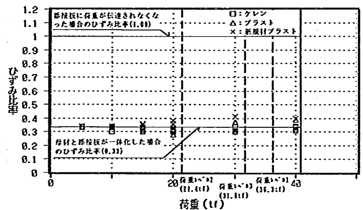
条件：充填材有り、締付軸力 22.5tf
