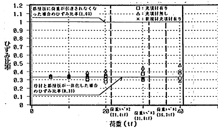
条件：プラスト、締付軸力 22.5tf
