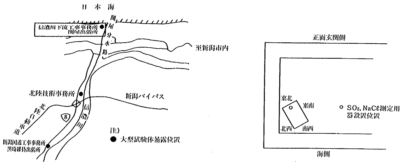
図-1.2.2 耐候性銅箱型暴露試験体の暴露位置
