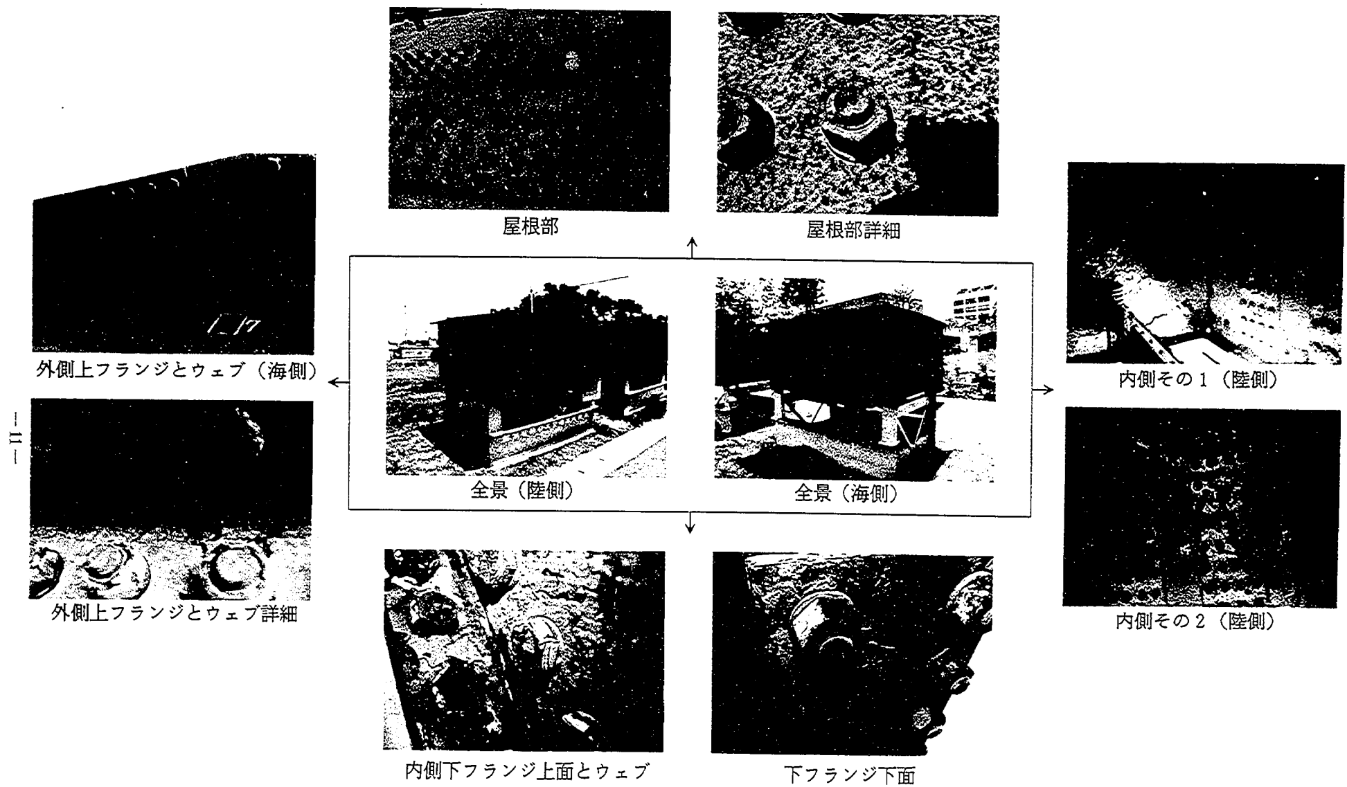
写真-1.2.1(b) 耐候性鋼箱型曝露試験体の腐食状況
