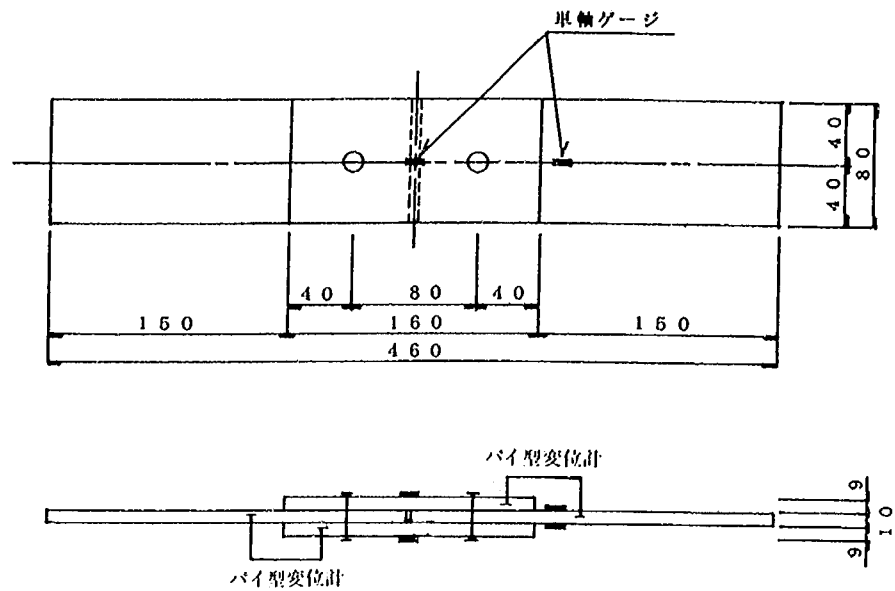
図-2.2.1 すべり試験体の寸法形状・ひずみゲージおよび変位測定位置
