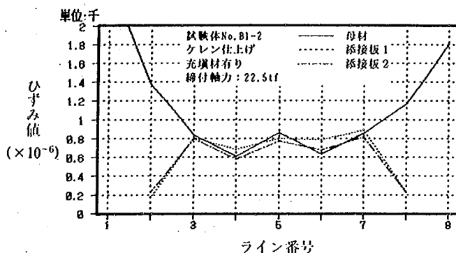
試験体 No.B1-2 (40.0tf 時)
