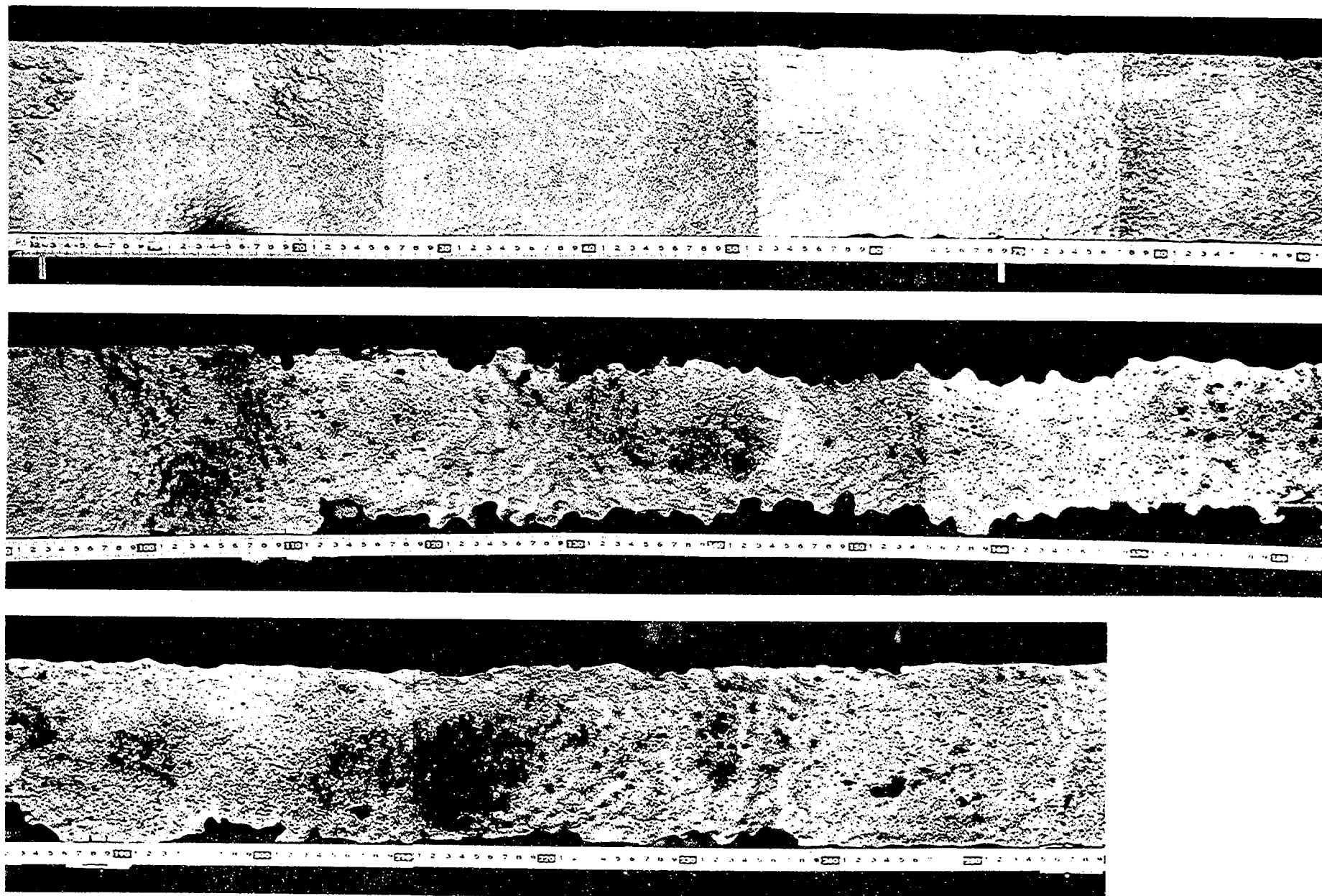
写真-1.3.2(b) 上フランジ腐食状況（試験体No.3）
