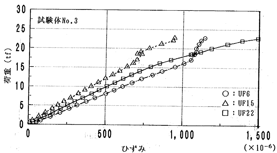
図-1.3.11 (a) 支間中央上フランジにおける荷重-ひずみの関係
