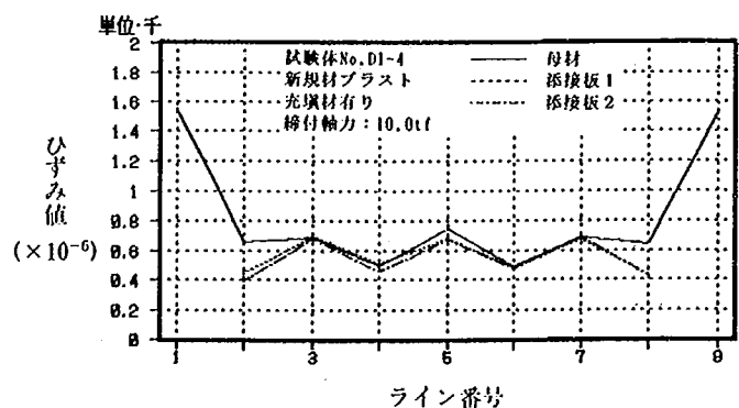
試験体 No.D1-4 (40.1tf 時)
