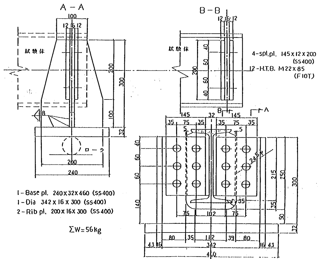
図-1.3.3 載荷ばりの寸法形状
