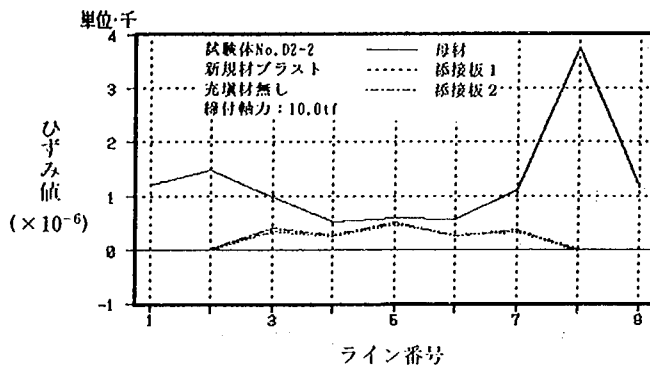
試験体 No.D2-2 (20.0tf 時)
