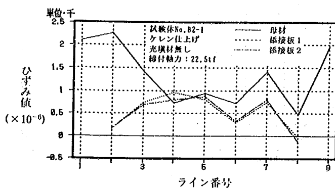
試験体 No. B2-1 (40.3tf 時)
