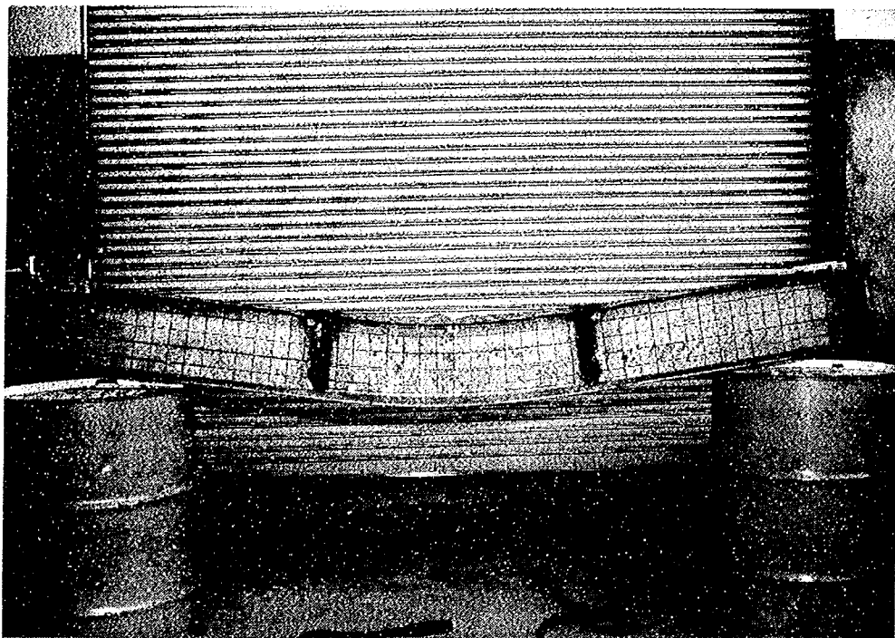
写真-1.3.5(c) 試験後の状況(試験体No.6)
