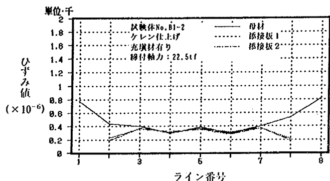
試験体 No.B1-2 (19.9tf 時)
