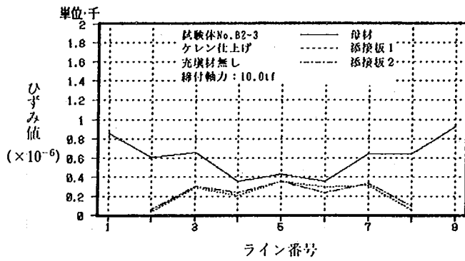
試験体 No. B2-3 (20.0tf 時)
