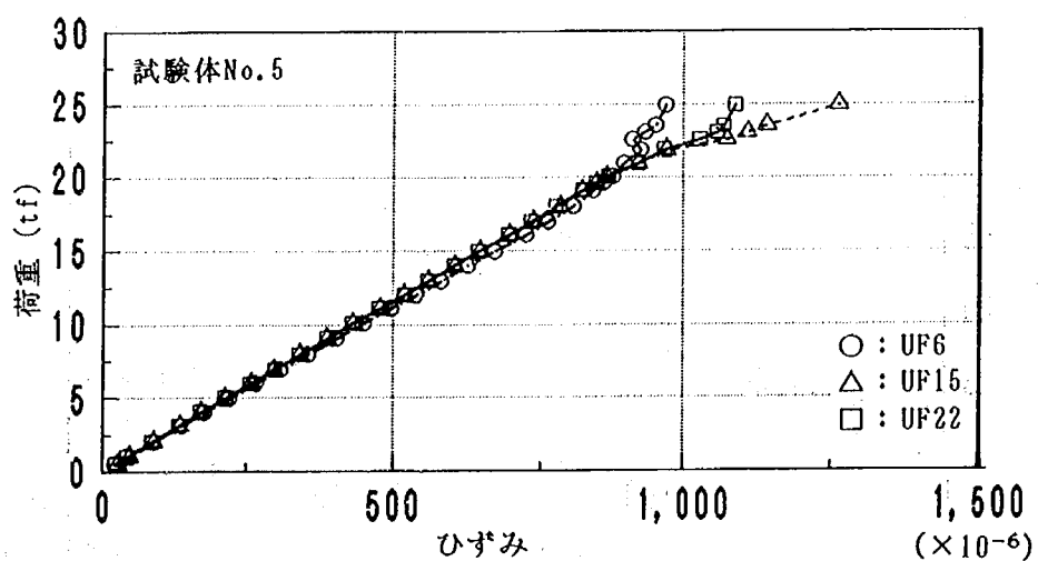
図-1.3.11 (b) 支間中央上フランジにおける荷重-ひずみの関係
