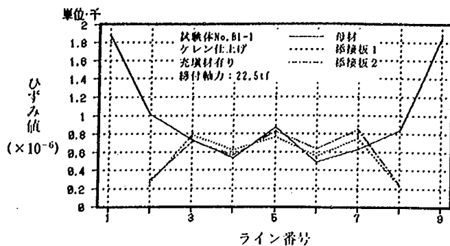
試験体 No.B1-1 (39.9tf 時)
