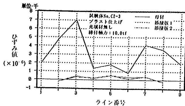
試験体 No. C2-3 (40.3tf 時)
