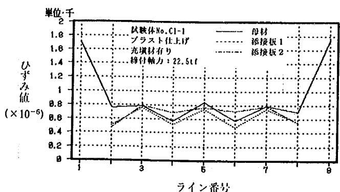
試験体 No. C1-1 (39.8tf 時)
