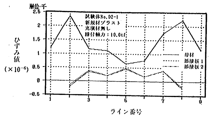
試験体 No.D2-1 (26.9tf 時)
