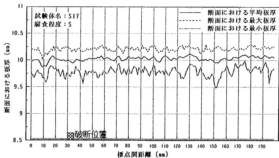
図-1.2.6(e) 板厚測定結果と破断位置の関係
