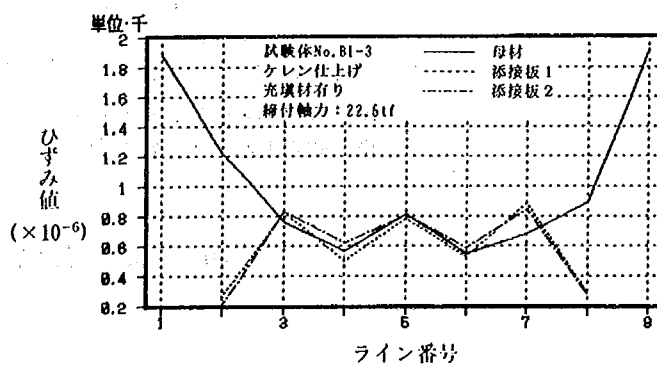
試験体 No.B1-3 (39.8tf 時)
