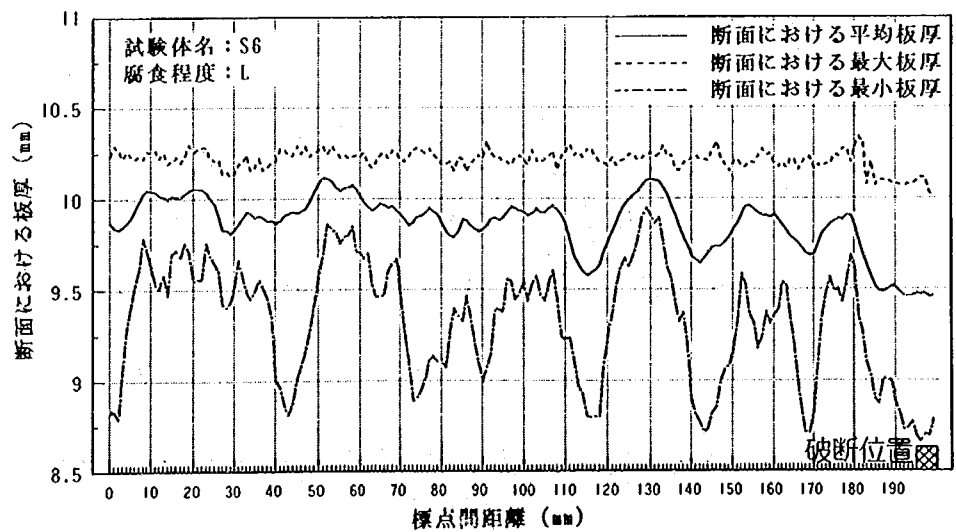
図-1.2.6 (b) 板厚測定結果と破断位置の関係
