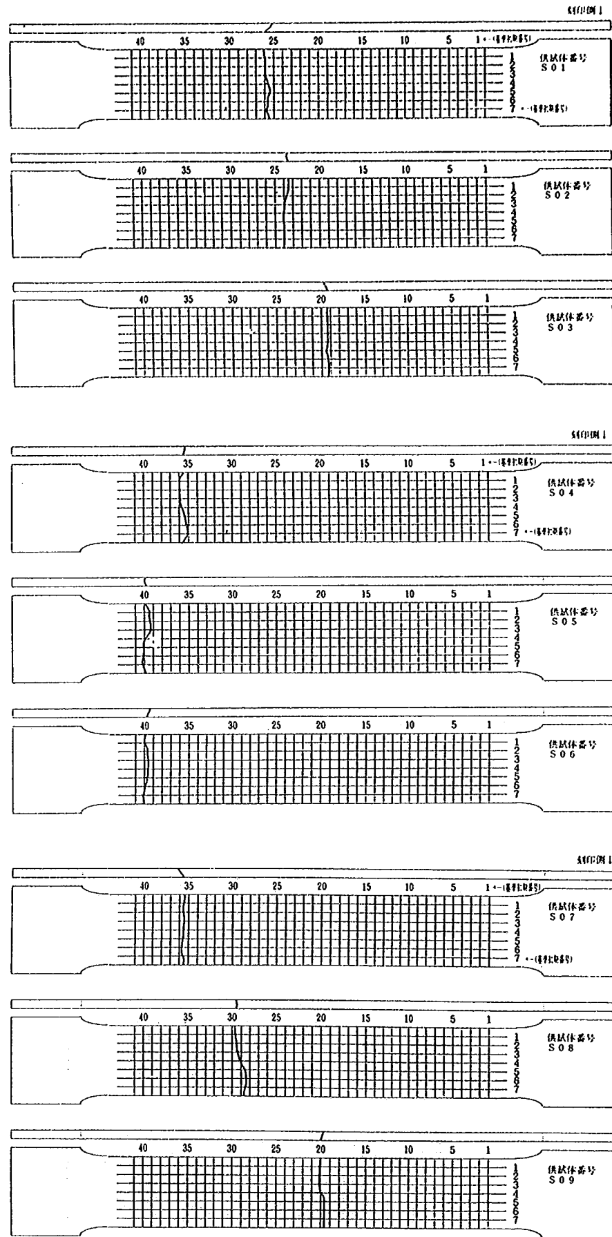
図-1.2.5(a) 板タイプ試験体の破断位置
