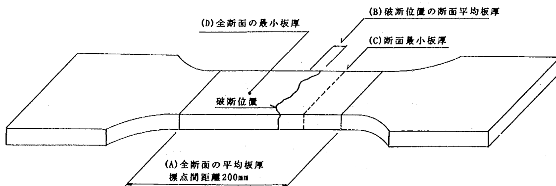
図-1.2.4 板厚測定結果の整理方法
