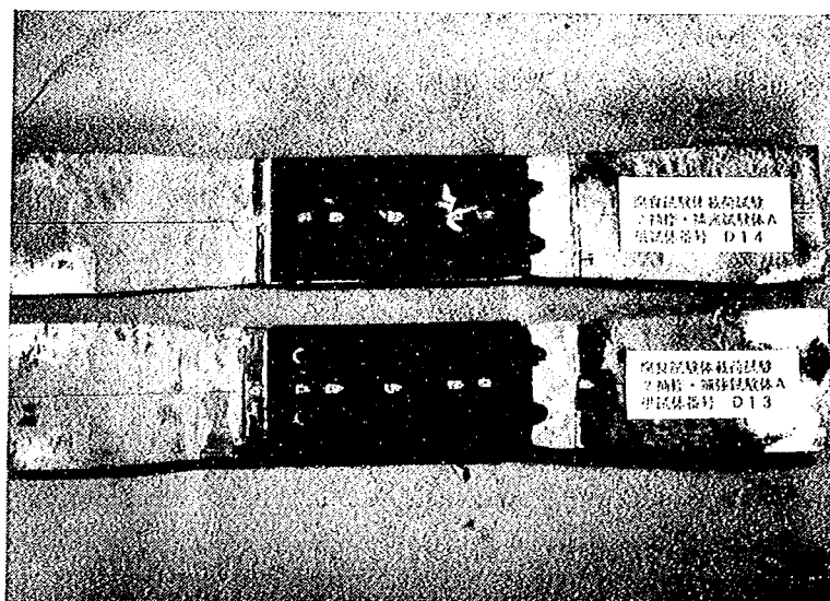
写真-2.3.2 試験体の破断状況
