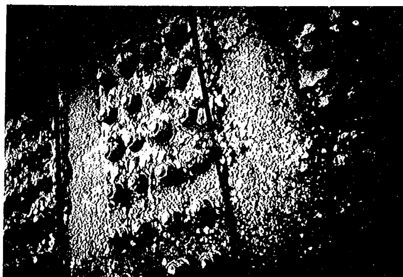
写真-1.2.1(a) 耐候性鋼箱型曝露試験体の腐食状況
