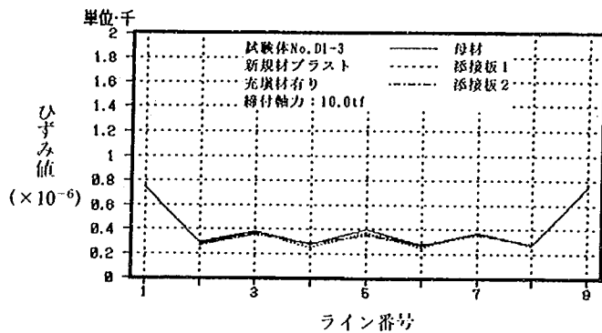
試験体 No.D1-3 (20.1tf 時)
