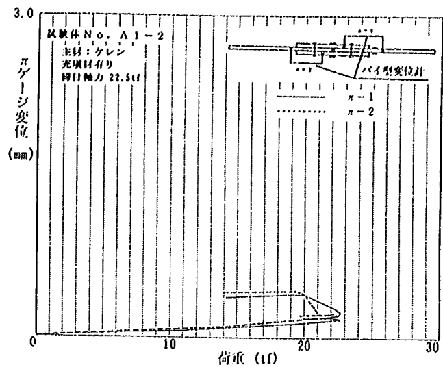
試験体 No. A1-2
