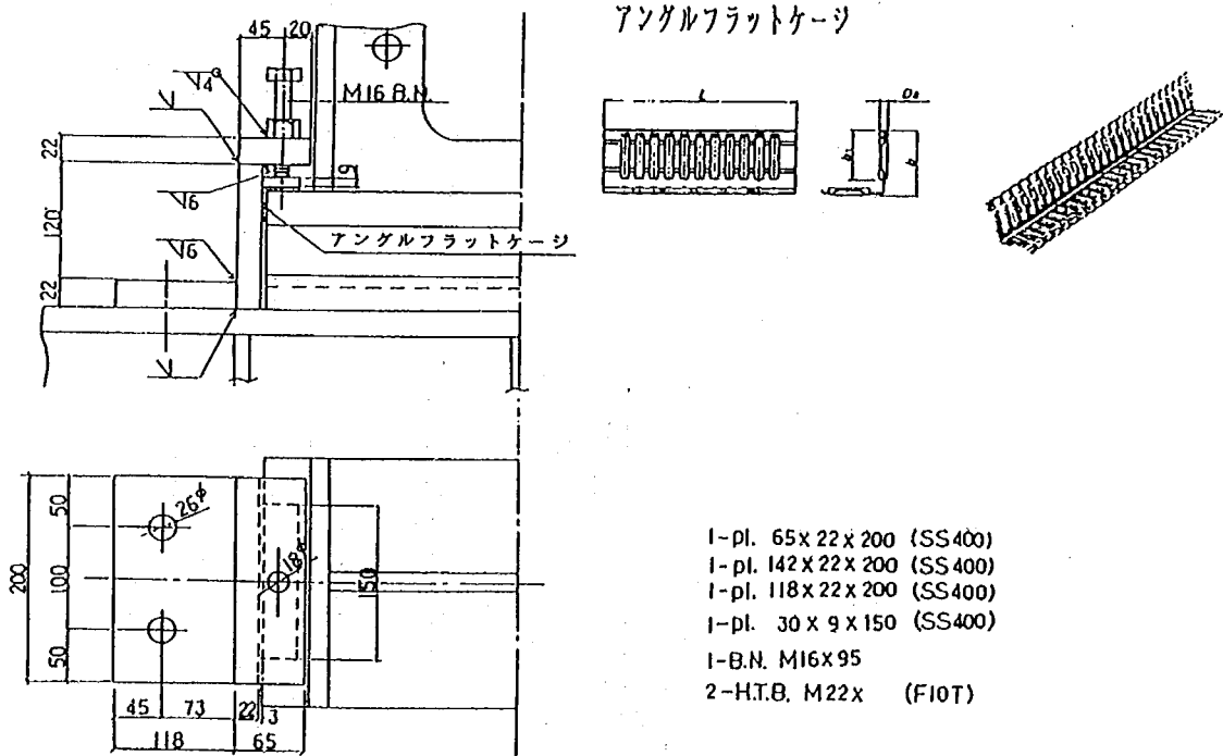
図-1.3.5 横倒れ防止治具の寸法形状
