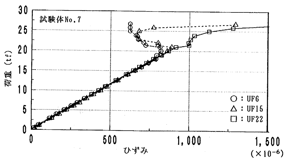
図-1.3.11 (c) 支間中央上フランジにおける荷重-ひずみの関係
