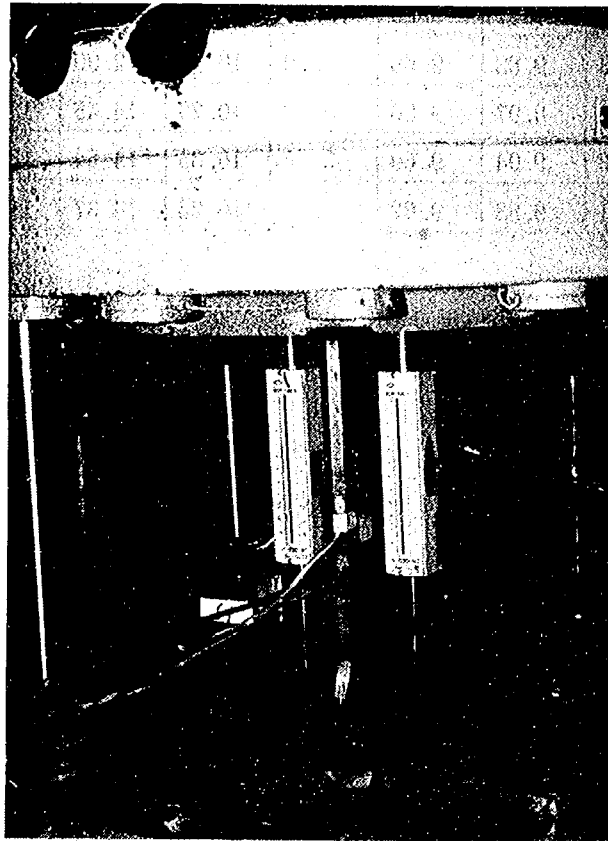
(b) 試験体および変位計の設置状況
