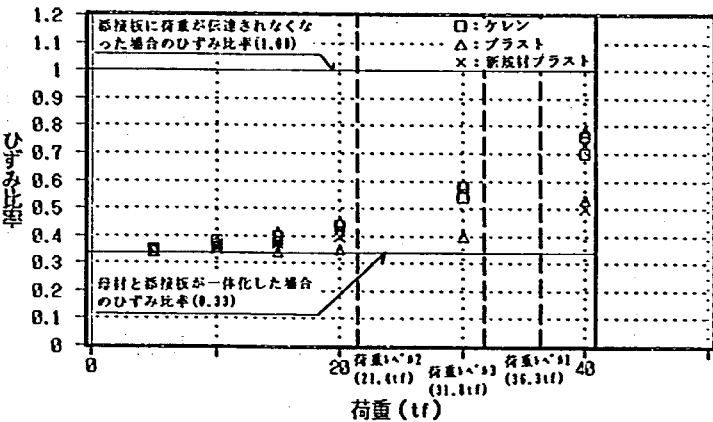
条件：充填材無し、締付軸力 10.0tf
