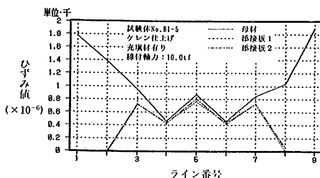
試験体 No. B1-5 (40.0tf 時)
