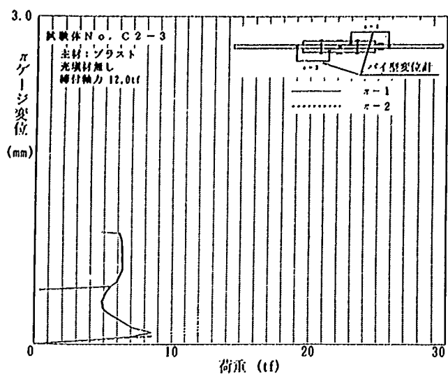
試験体 No. C2-3
