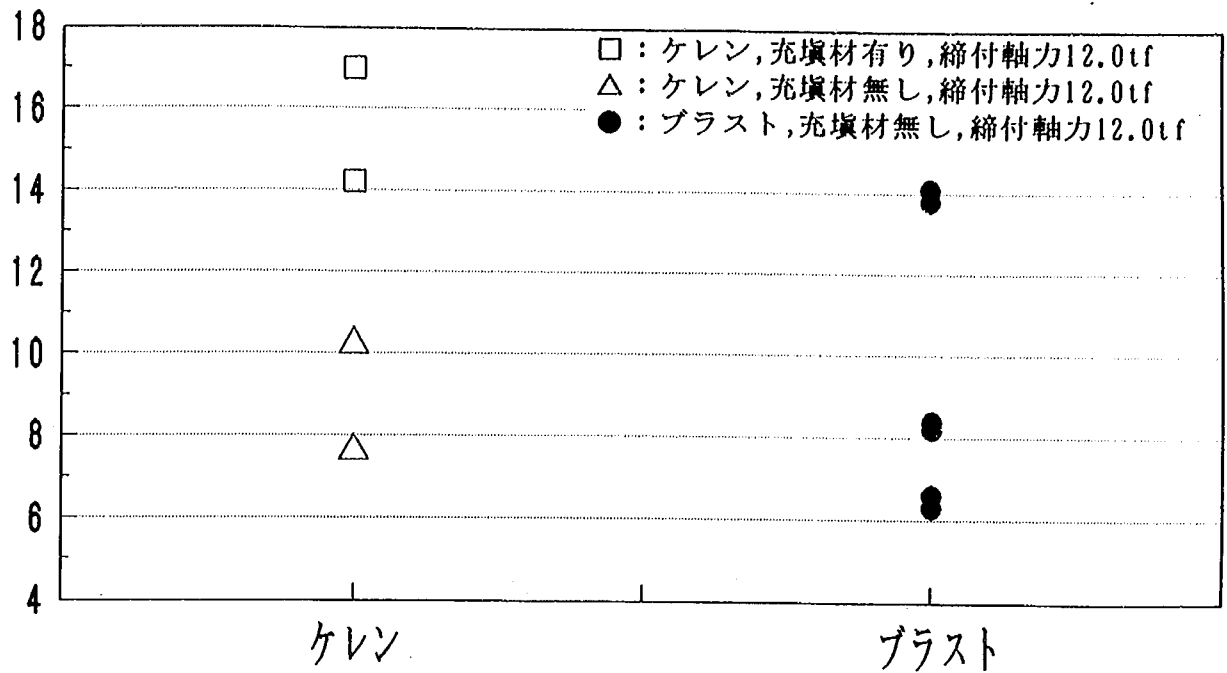
図-2.2.3 接合条件とすべり荷重との関係
