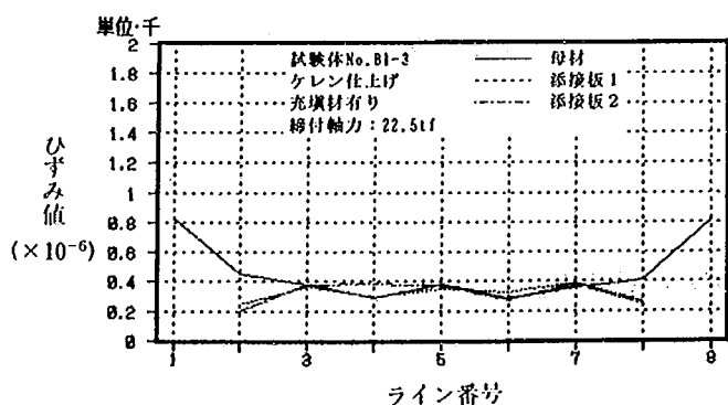
試験体 No.B1-3 (20.0tf 時)
