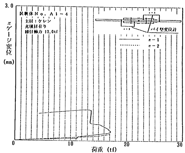
試験体 No. A1-4
