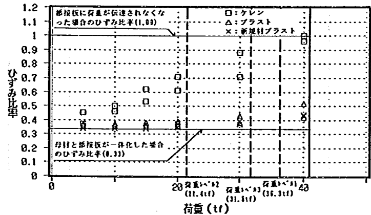
条件：充填材有り、締付軸力 10.0tf
