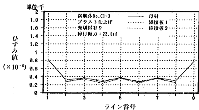
試験体 No. C1-3 (19.8tf 時)
