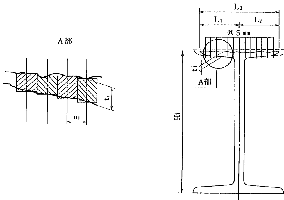
図-1.3.2 断面欠損したフランジ部の板厚測定方法
