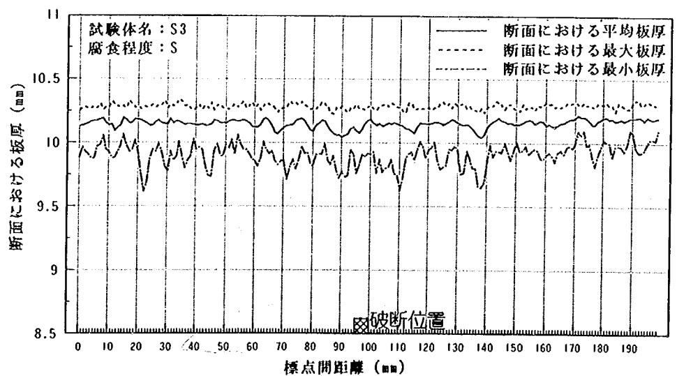
図-1.2.6(a) 板厚測定結果と破断位置の関係
