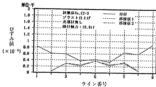
試験体 No. C2-3 (20.1tf 時)
