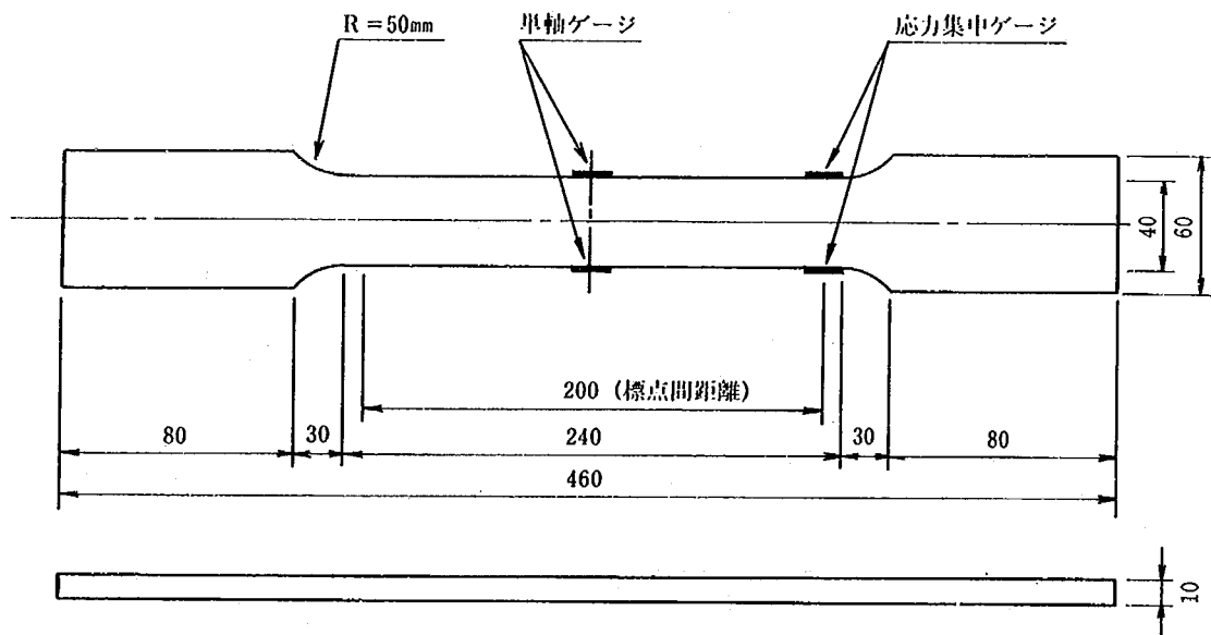
図-1.2.3 板タイプ試験体の寸法形状、ひずみゲージ添付位置
