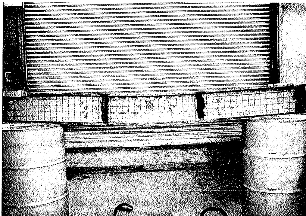
写真-1.3.5(f) 試験後の状況（試験体No.7）
