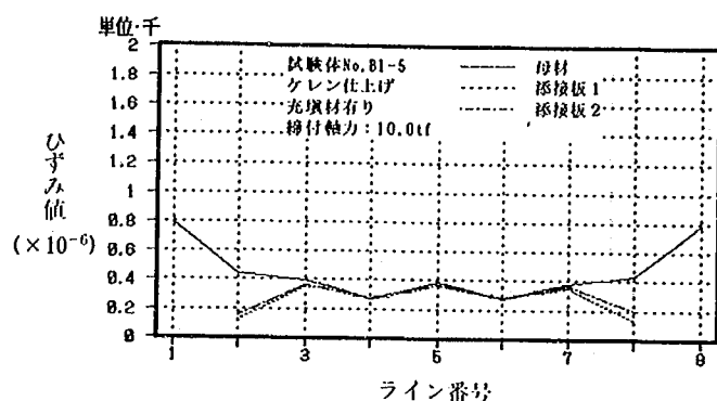
試験体 No. B1-5 (20.1tf 時)
