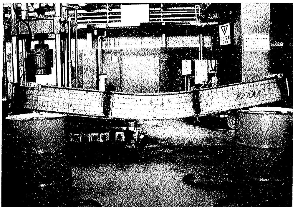
写真-1.3.5(b) 試験後の状況（試験体No.3）
