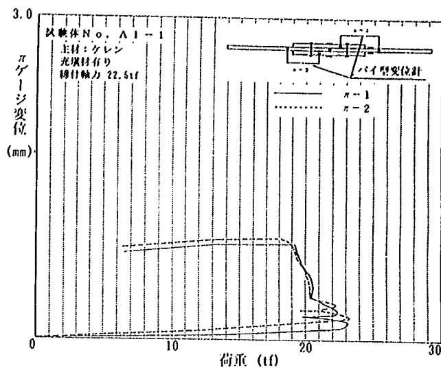
試験体 No. A1-1
