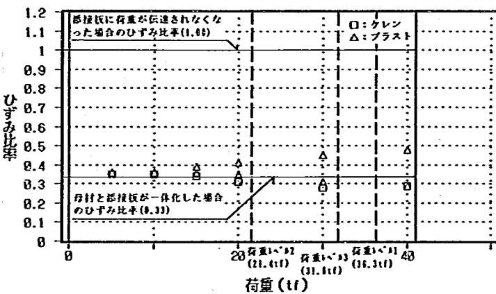
条件：充填材無し、締付軸力 22.5tf
