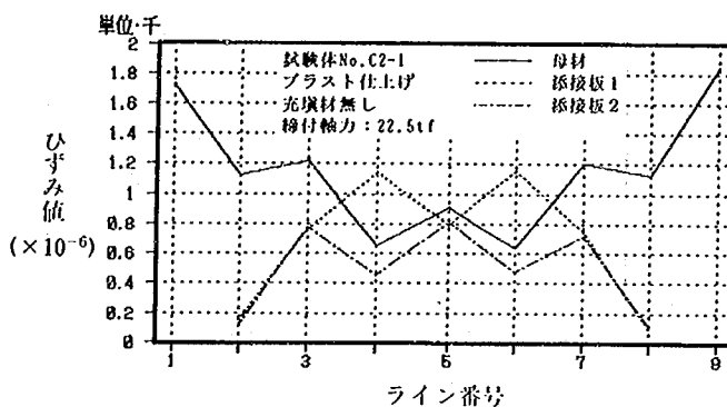
試験体 No.C2-1 (39.9tf 時)
