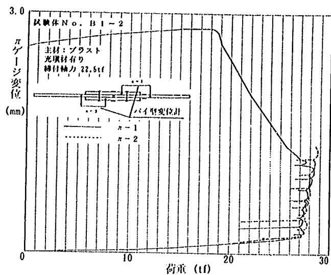
試験体 No. B1-2
