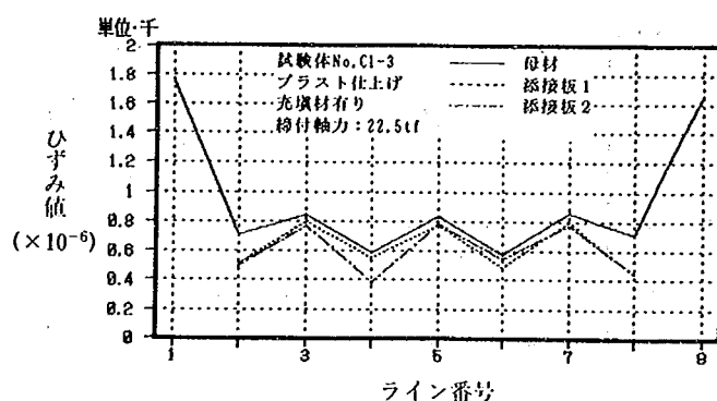
試験体 No. C1-3 (39.9tf 時)
