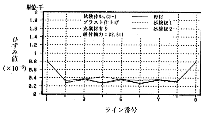
試験体 No. C1-1 (19.8tf 時)
