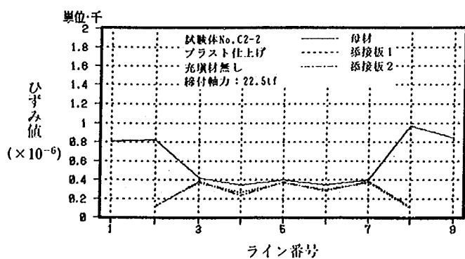
試験体 No.C2-2 (19.9tf 時)
