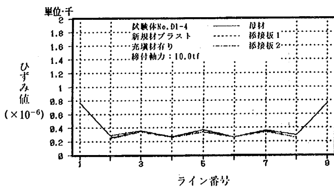
試験体 No.D1-4 (20.2tf 時)
