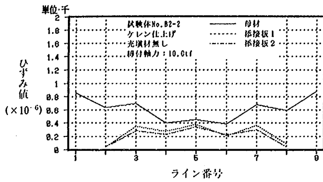
試験体 No. B2-2 (20.2tf 時)
