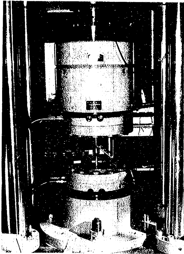
(a) 60/90 tf 疲労試験機
