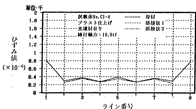
試験体 No. C1-4 (20.1tf 時)
