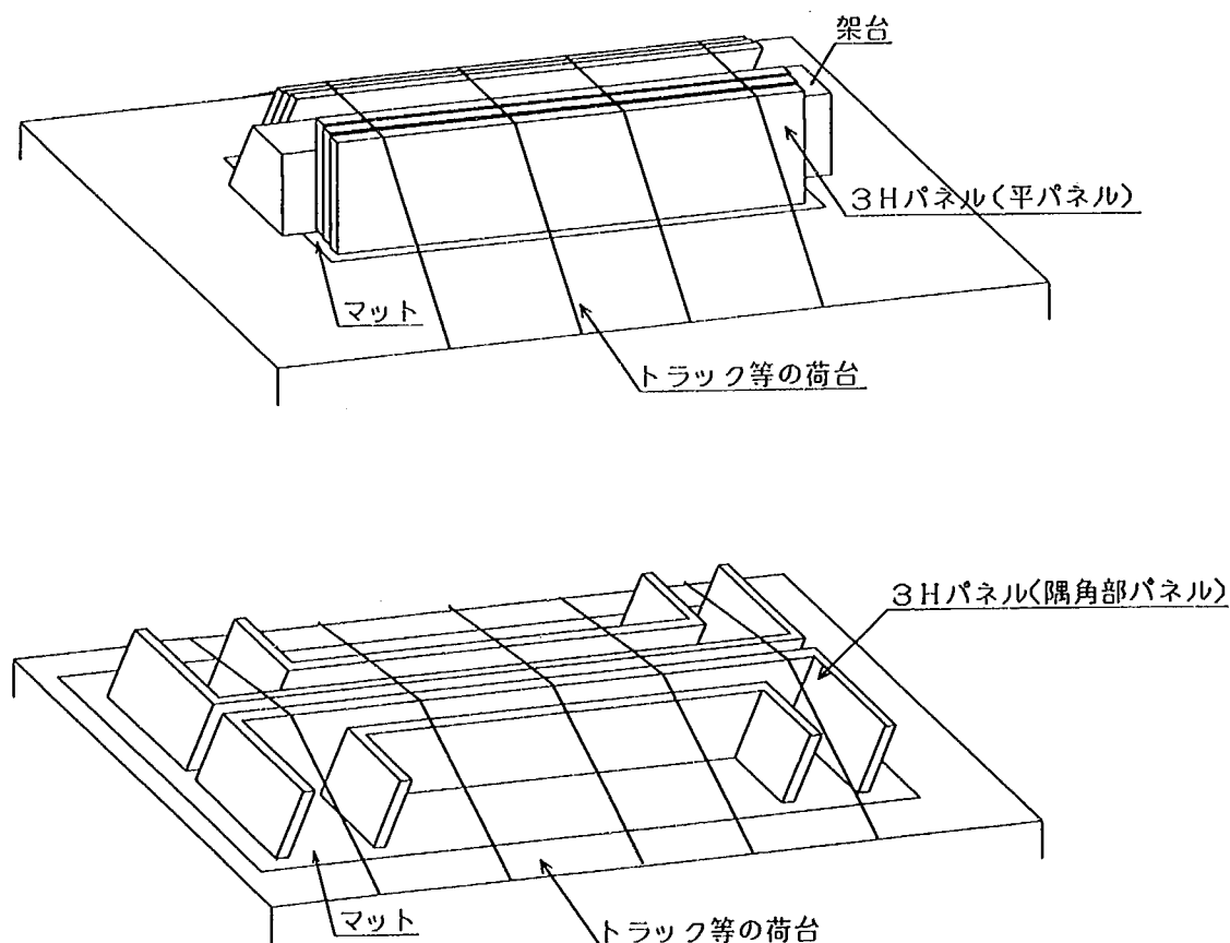
図-解 7.3.1 3Hパネルの運搬状況
