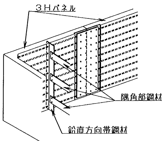
図-解 12.3.1 隅角部鋼材の接合構造
