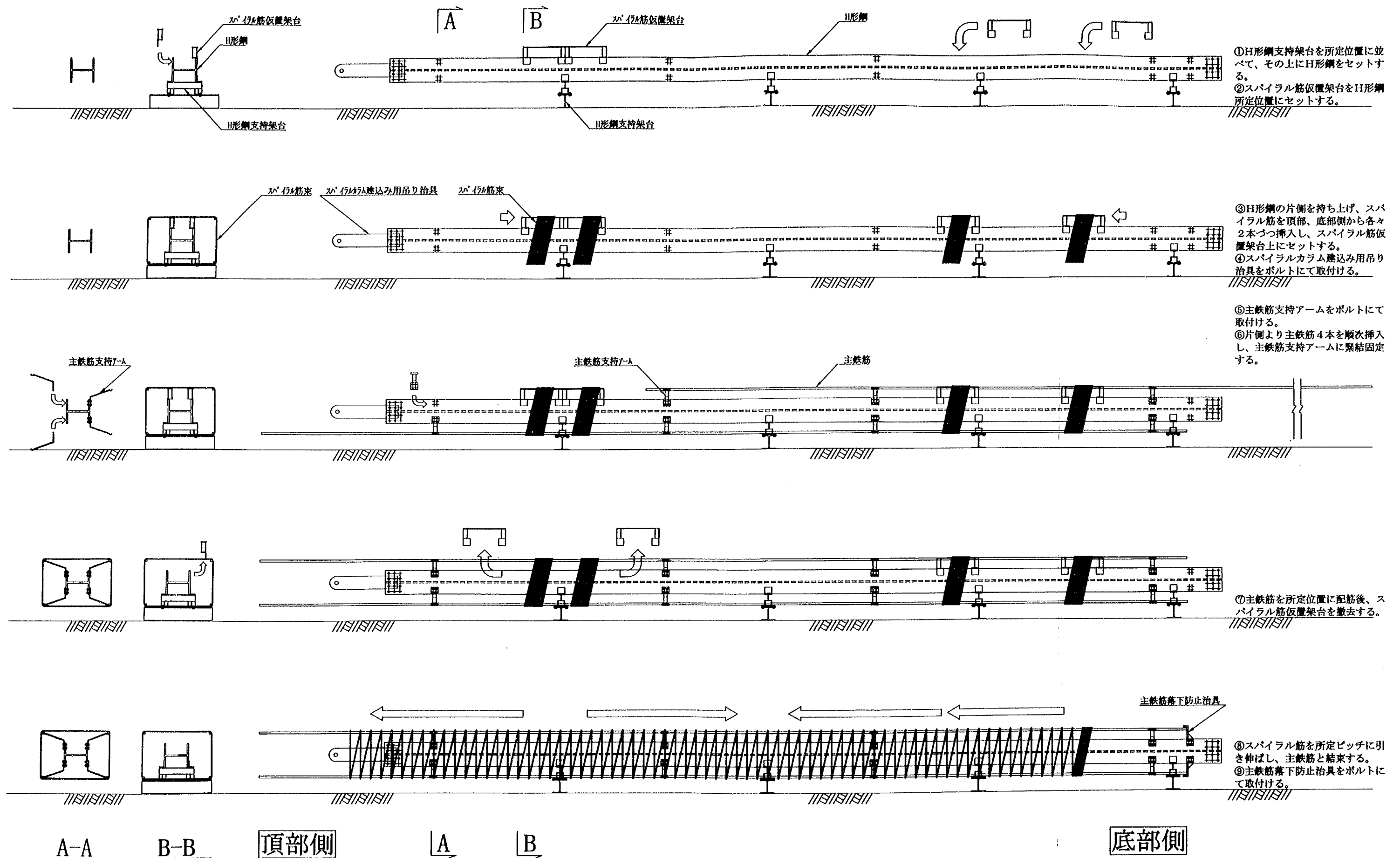
図-解 11.2.1 スパイラルカラムの地組み順序の一例
