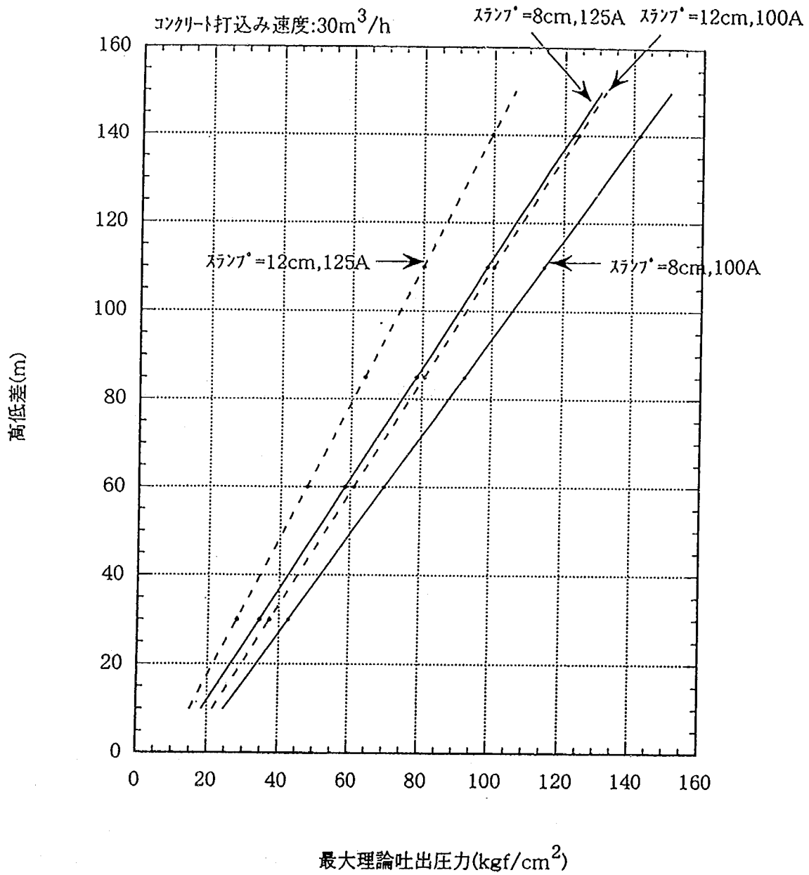
図-解 14. 1. 1 最大理論吐出圧力と高低差の関係
