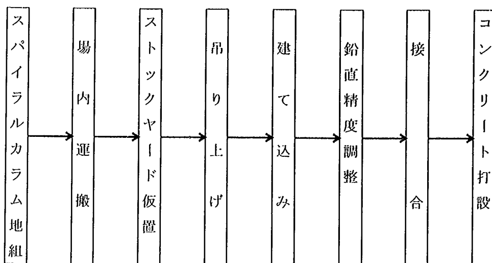
図-解 11.2.2 スパイラルカラムの施工ステップ
