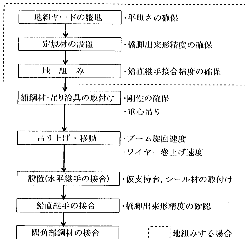
図-解 12.1.1 3Hパネルの組立手順
