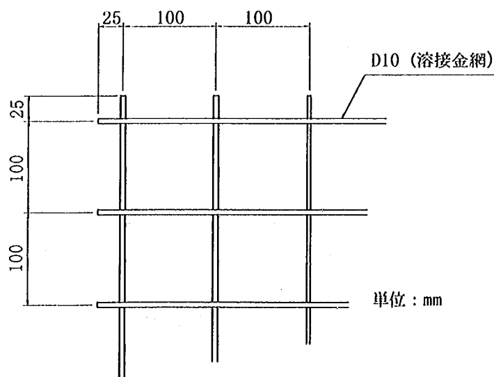
図-解 5.1.1 ひび割れ制御筋の一例
