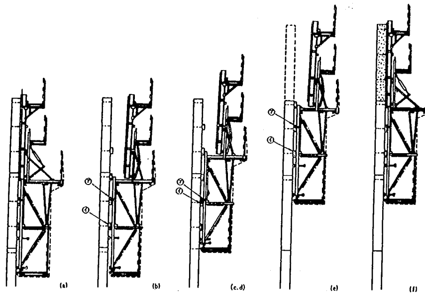
図-解 13.1.4クライミングフォーム工法
