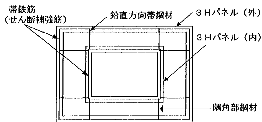
図-解 5.4.1 3Hパネル，鉛直方向帯鋼材，隅各角鋼材の配置例
