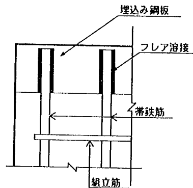
図-解 7.2.3 埋込み鋼板と帯鉄筋の溶接方法の例
