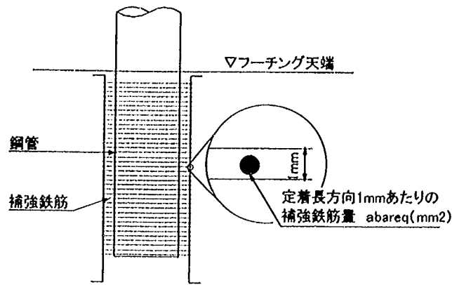
図-解 5.2.5 補強鉄筋量
