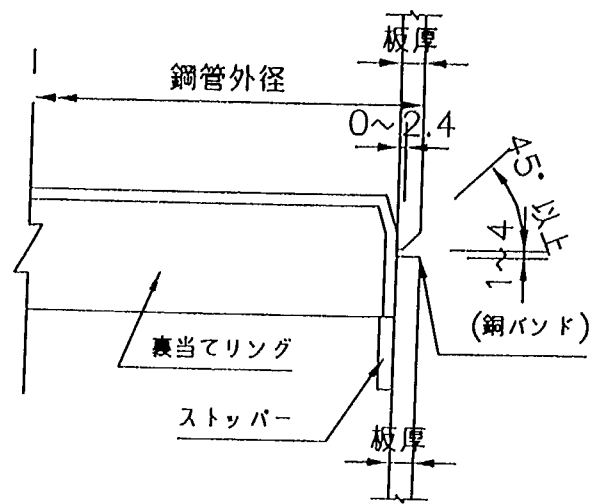
図-解 8.3.1 現場溶接継手の構造（鋼管）
