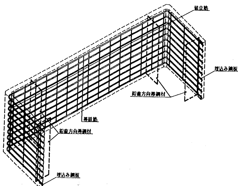
図-解 7.2.1 3 Hパネルの鉄筋・鋼材配置例
