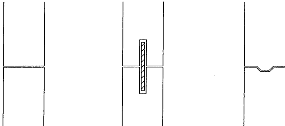
図-解 12.2.2 3Hパネルの水平継手構造の例
