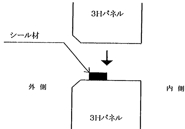
図-解 12.2.1 3H工法の継目処理
