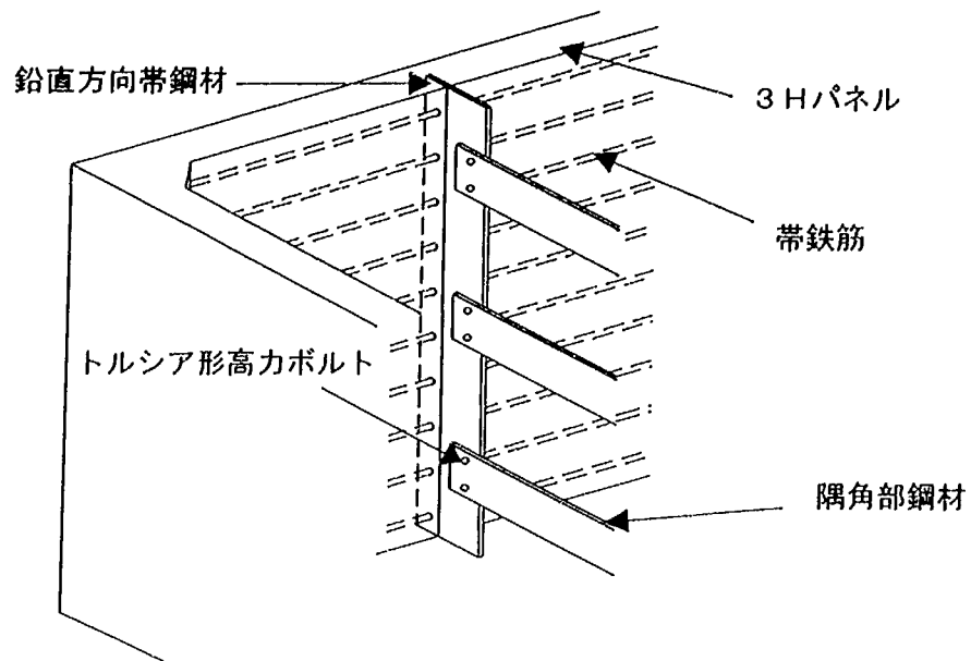
図-解 5.4.3 鉛直方向帯鋼材，隅角部鋼材の配置例
