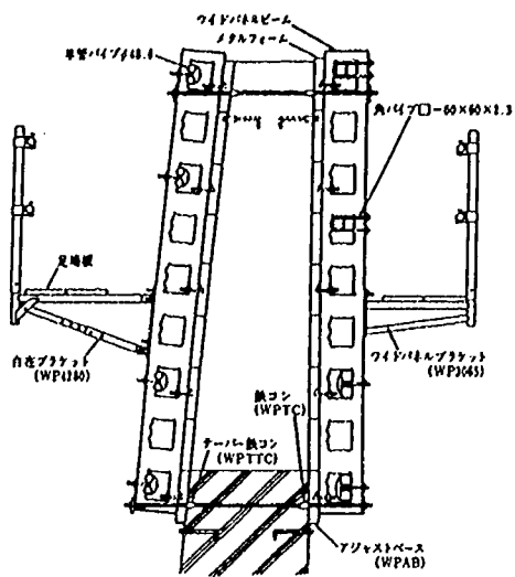
図-解13.1.1 大型パネル型枠工法
