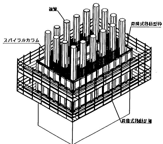
図-解 1.1.2 3Hパネルによる高橋脚の施工 図-解 1.1.3 昇降式移動型枠による高橋脚の施工
