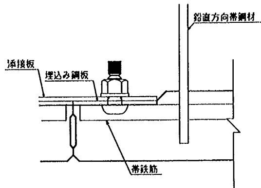
図-解 7.2.2 埋込み鋼板と添接板のボルトによる連結
