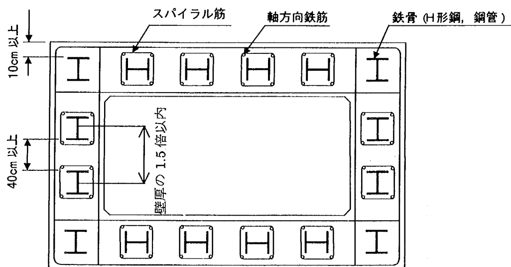
図-解 5.2.1 軸方向鋼材の配置例
