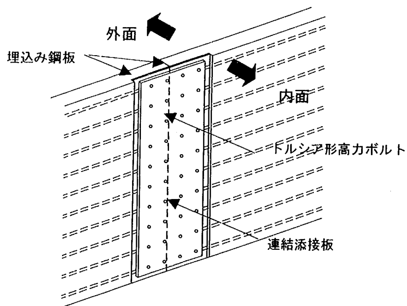
図-解 5.4.2 鉛直継手構造
