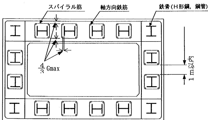
図-解 5.3.1 スパイラル筋配置例
