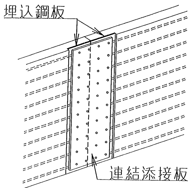
図-解 1.4.4 埋込み鋼板および連結添接板
