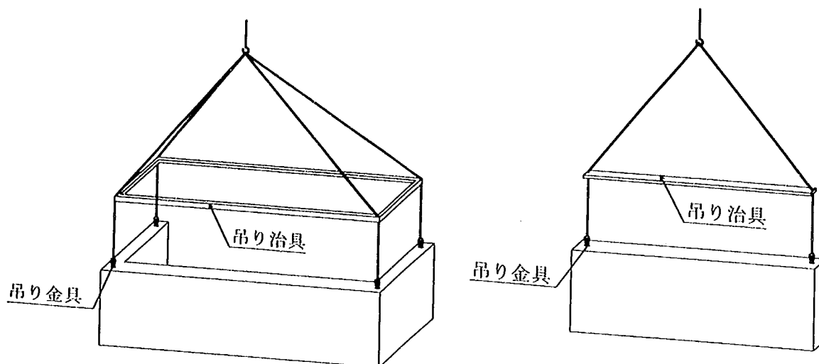
図-解 7.2.4 3 H パネルの吊り状況の例
