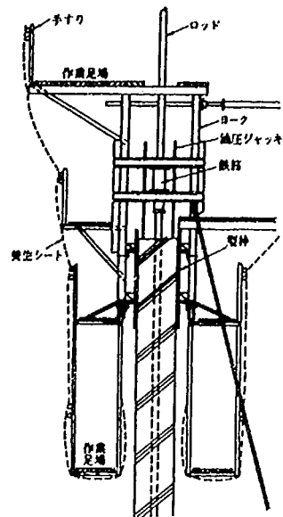
図-解13.1.2 スリップフォーム工法
