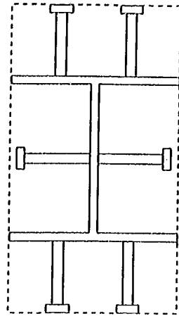
図-解 5.2.2 スタッドを取り囲む鉄骨周囲のせん断抵抗面
