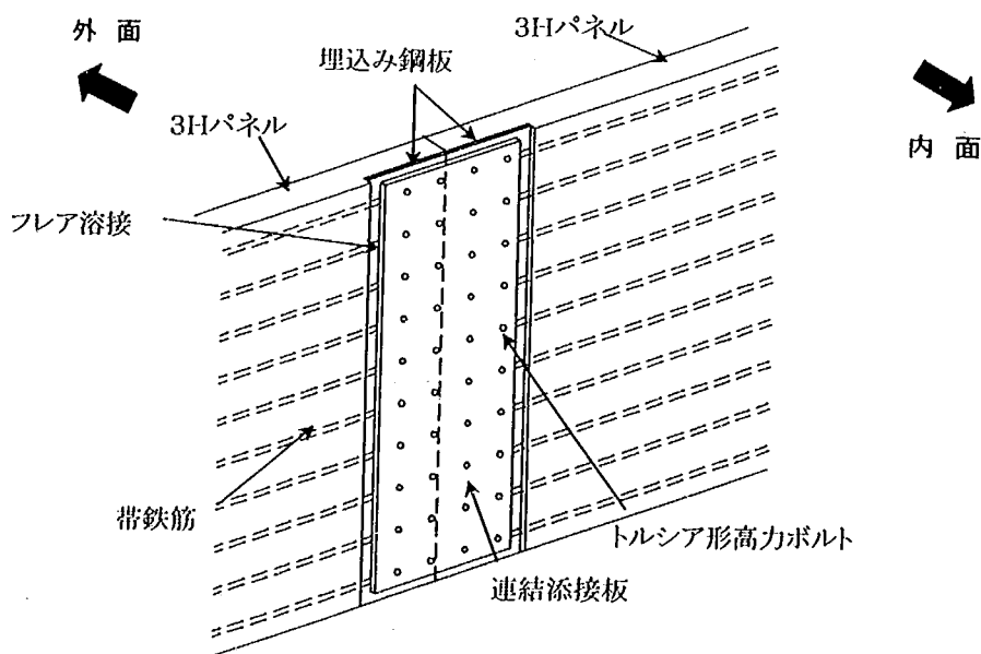
図-解 12.2.4 3Hパネルの鉛直継手構造
