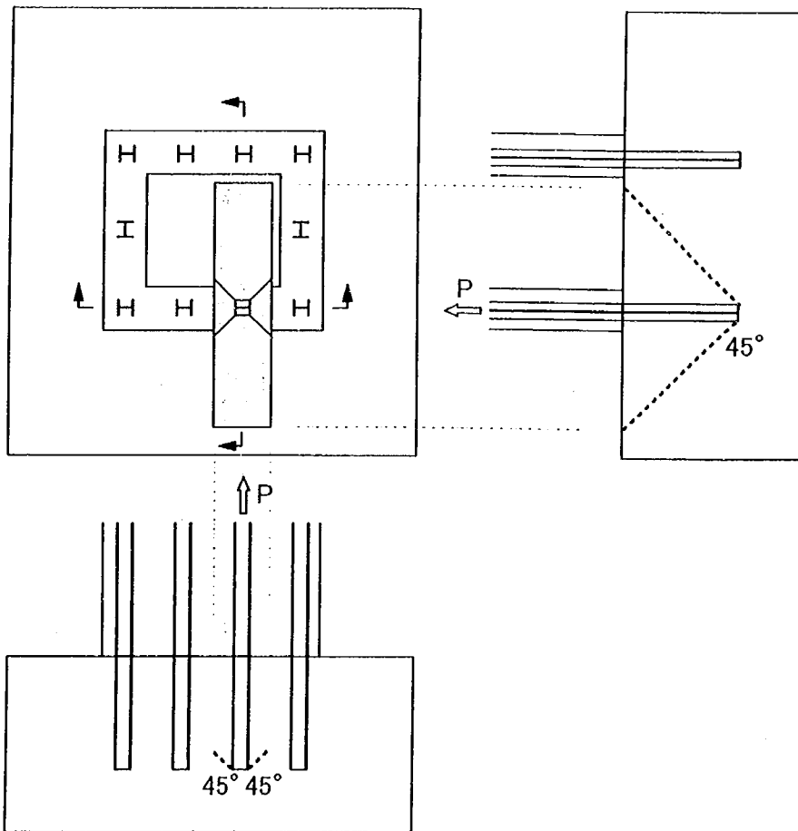
図-解 5.2.3 鉄骨下端から45° のせん断抵抗面
