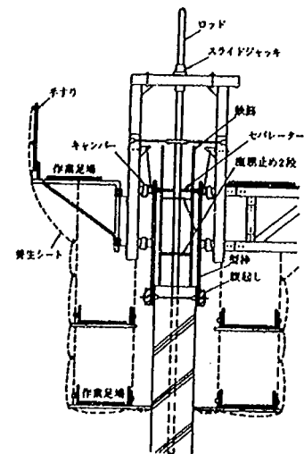
図-解13.1.3 ジャンピングフォーム工法
