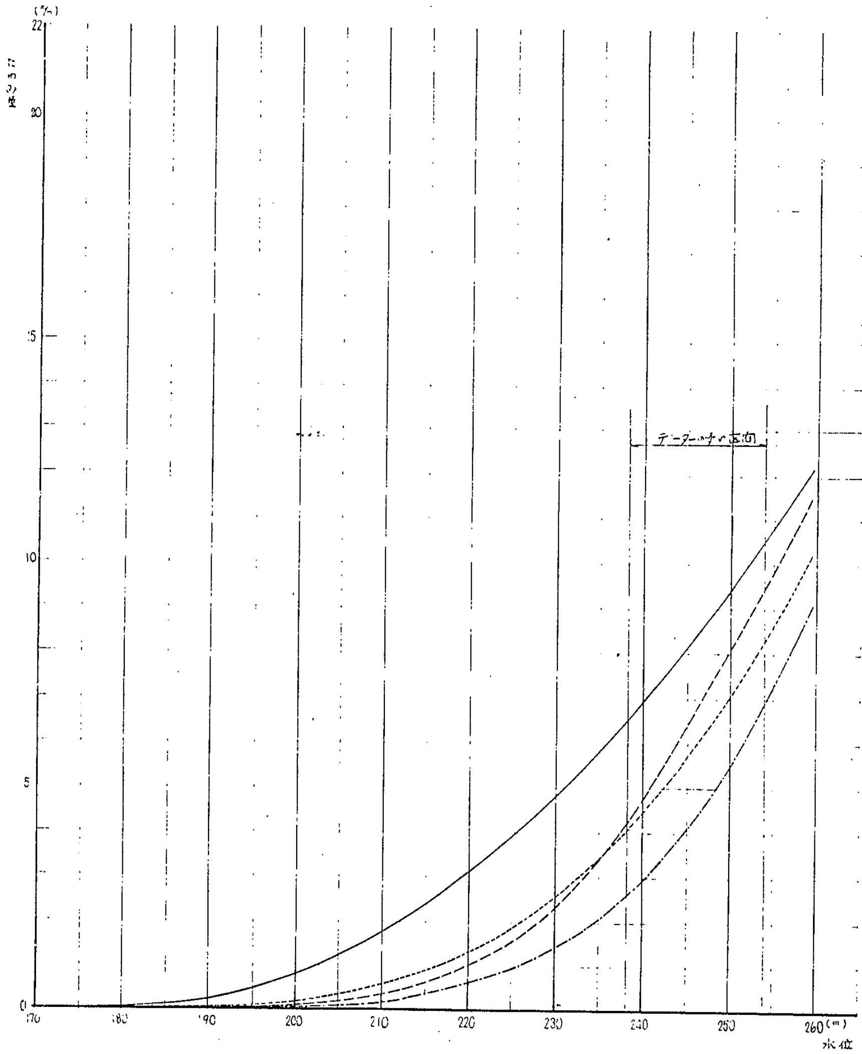
図-5 鳴子ダム水位たわみ曲線
