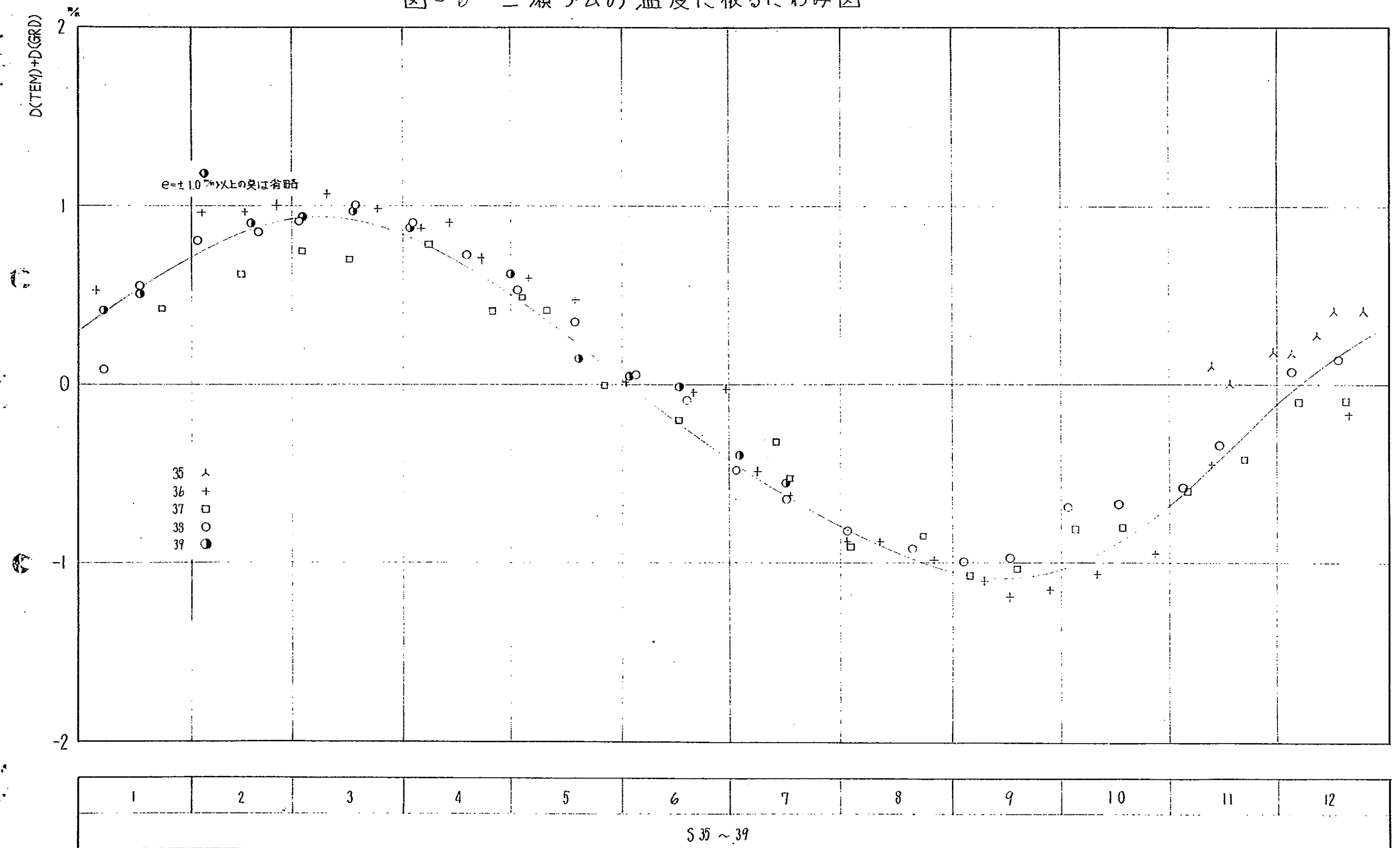
図-6 二瀬タムの温度に依るにわみ図
