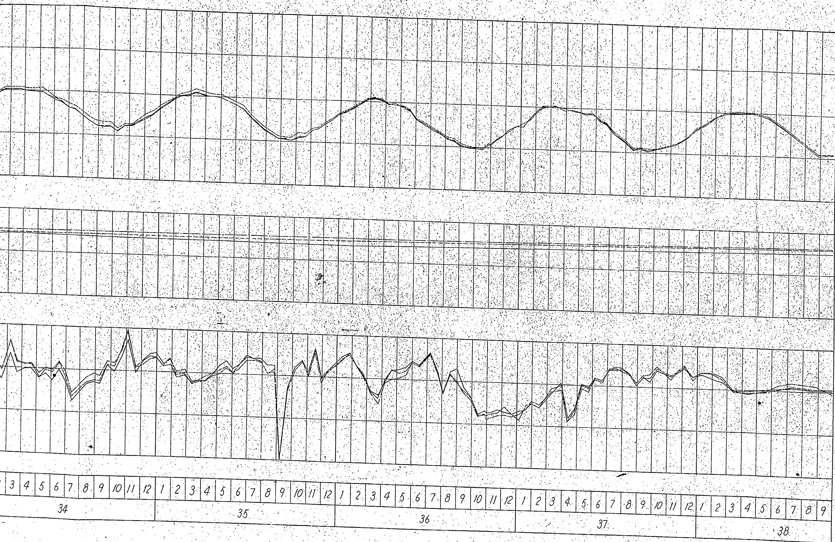
図-2 鳴子ダム撓み重回帰分析比較図
