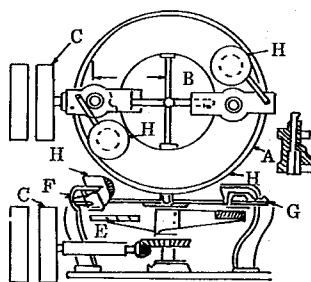
ドリー すりへり摩耗試験機
