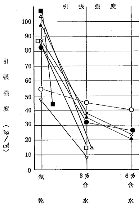
図-16 引張強度
