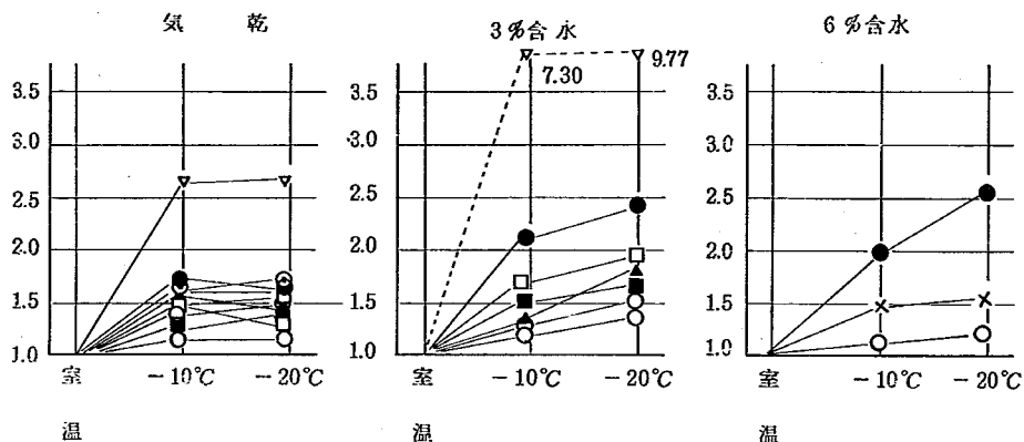
図-15 低温状態の違いによる圧縮強度比(室温状態を1とした場合)
