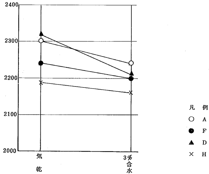
図-36 骨材の含水状態とコンクリートの単位体積重量の関係
