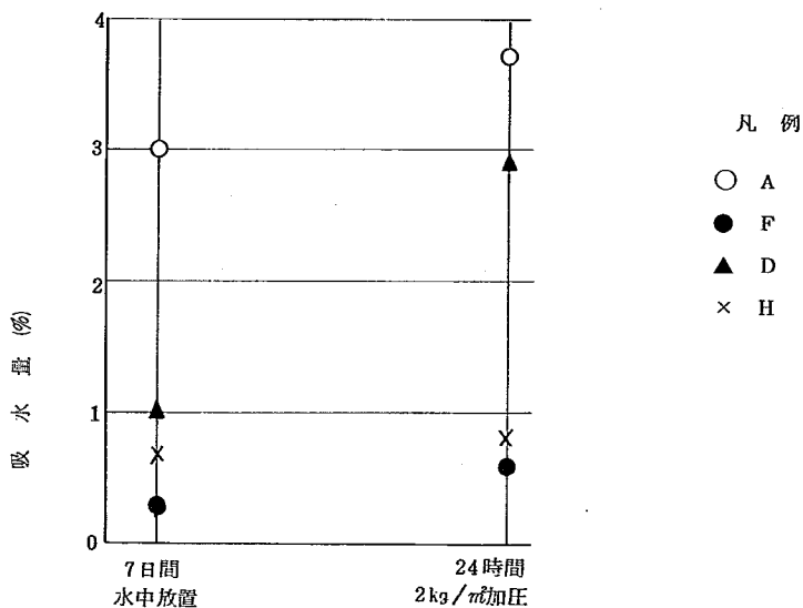
図-37 吸水量試験結果
