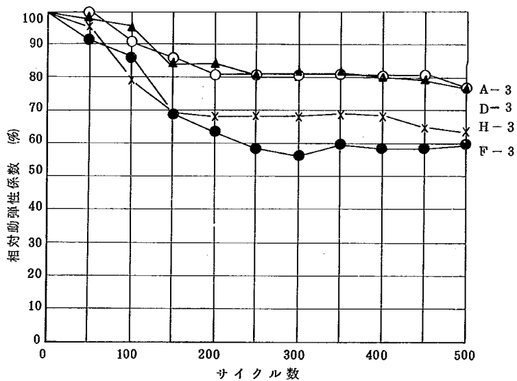
図-38 単体供試体の相対動弾性係数の変化
