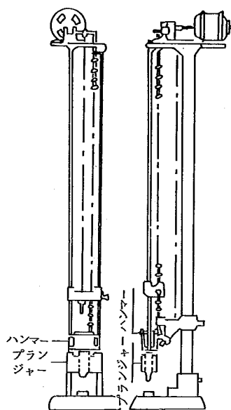
ペー ジ 衝撃試験機
