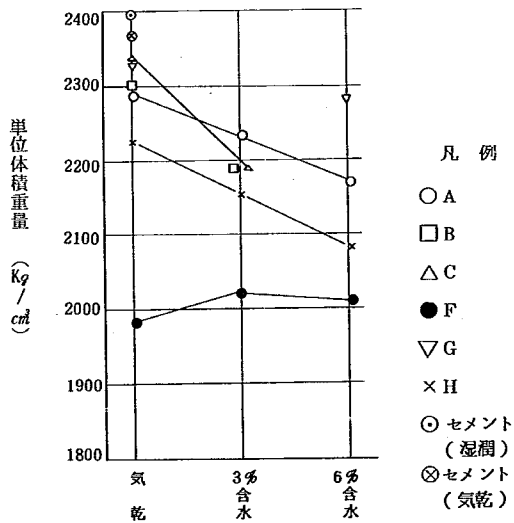
図-21 コンクリートの単位体積重量
