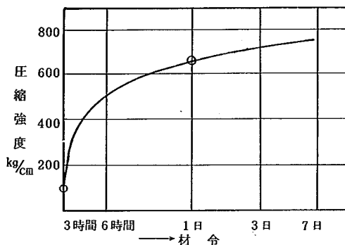
図-5 ポリクリートの材令と強度
