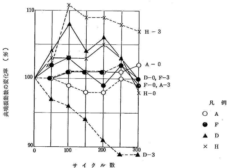
図-44 張り合せ供試体の共鳴振動数の変化
