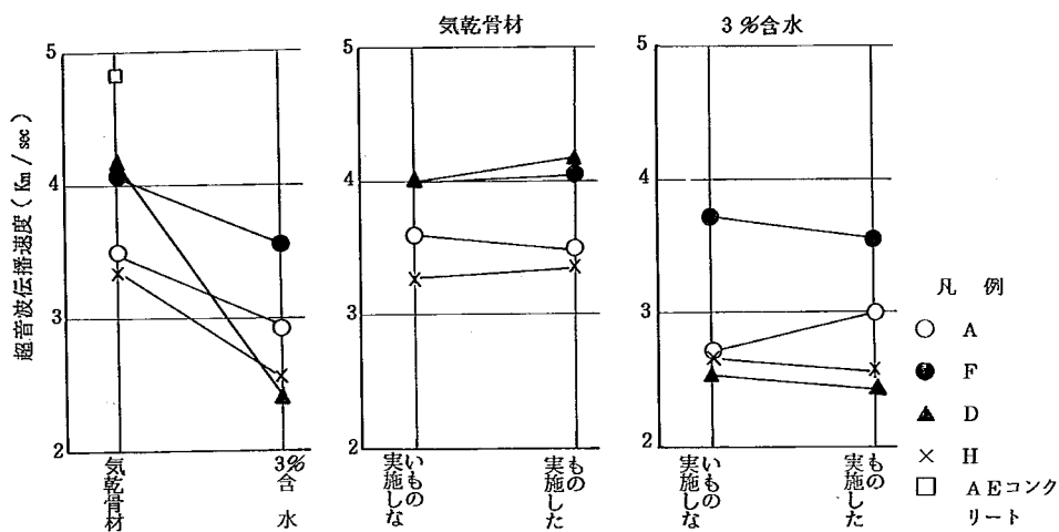
図-43 張合せ供試体の超音波伝播速度 (レジコンクリートのみ)
