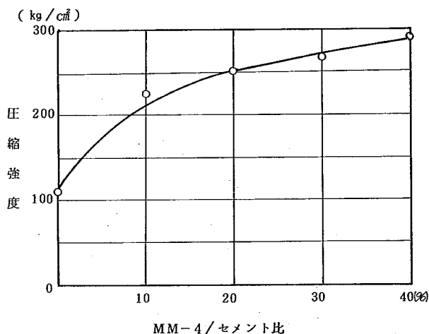
図-6 圧縮強度とMM-4 / セメントの関係
