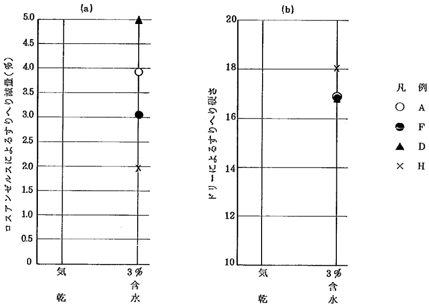
図-35 摩耗(すりへり減量, すりへり硬さ)試験結果
