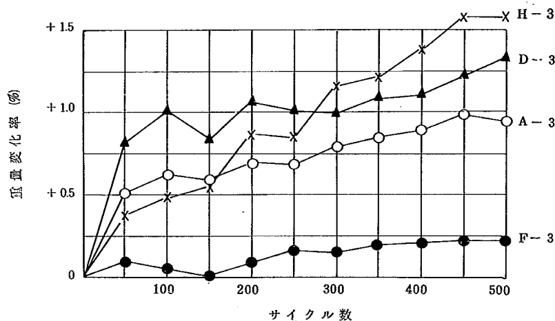
図-39 単体供試体の重量変化
