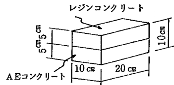
張り合せ供試体 (B)
