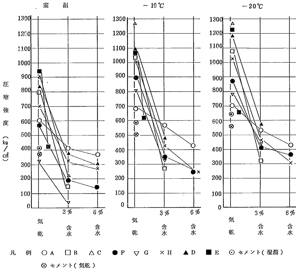
図-12 骨材の含水状態と圧縮強度との関係
