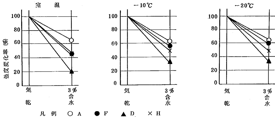
図-29 含水状態の違いによる圧縮強度比
