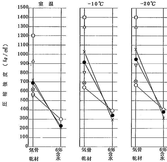
図-45 一年暴露供試体の骨材含水状態と圧縮強度の関係
