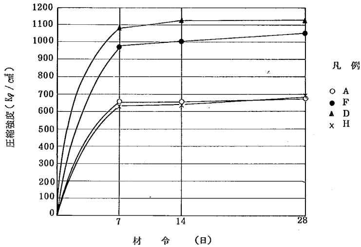
図-27 気乾骨材を用いた各レジンコンクリートの材令と強度の関係
