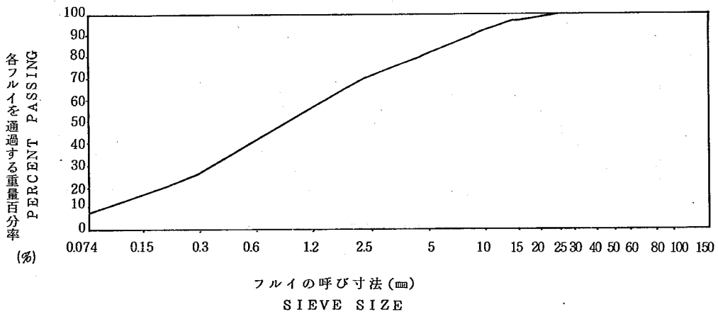
図 - 8 現地骨材の粒度分布
