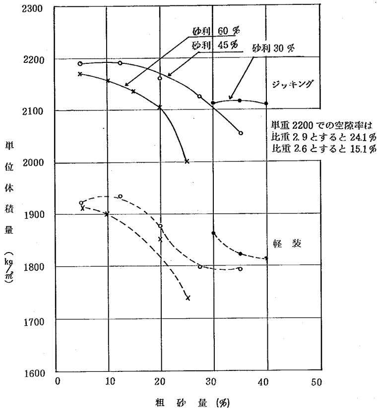
図 - 10 骨材の最大密度の検討
