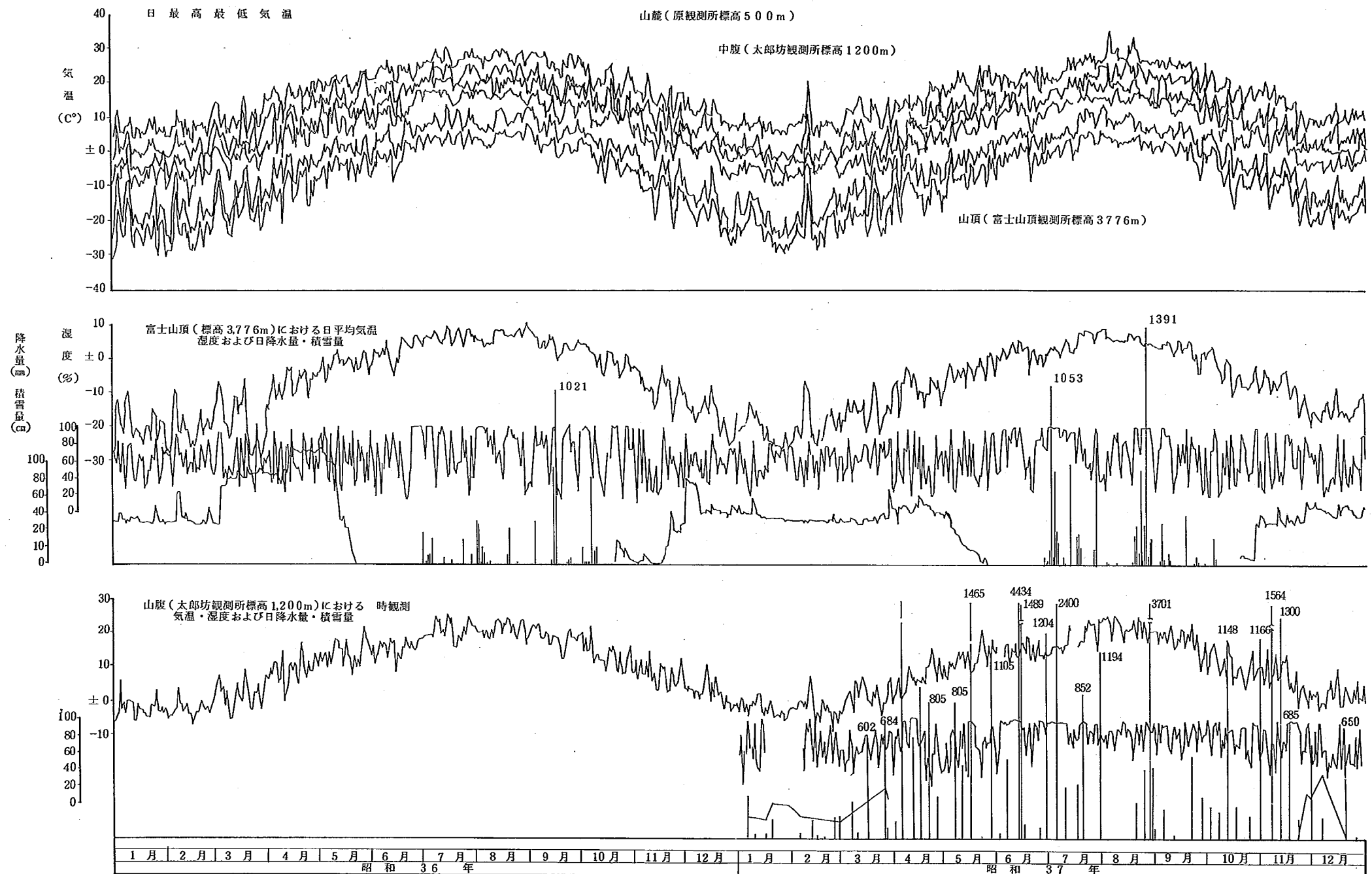
図 - 1 気象記録
