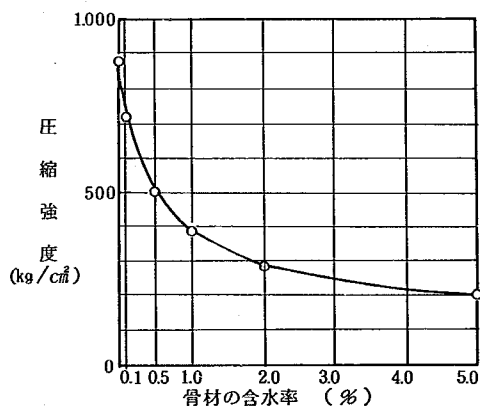
図-7 強度と骨材含水率の関係
