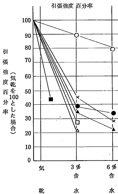
図-17 引張強度百分率
