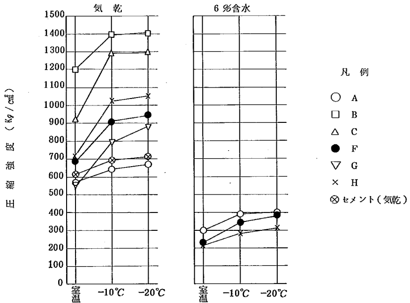
図-46 試験時の温度と圧縮強度の関係
