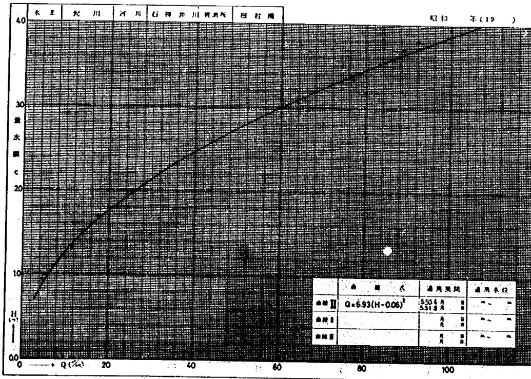
水位流量曲线图 II
