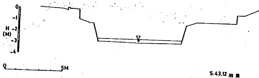
图3 上石神井観測所河川断面 (同観測上流 5 m 地点)
