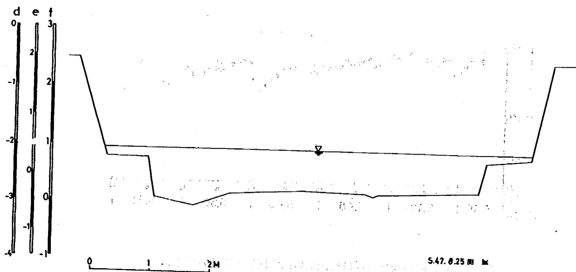
图4 上石神井観測所断面
