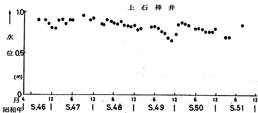
図5 低水位の経年変化（根村橋流量観測所は量水標Cの読み、 上石神井流量観測所は量水標hの読みに換算した値）
