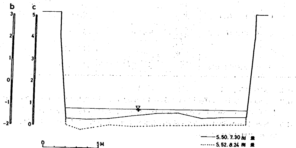
図2 根村橋観測所河川断面
