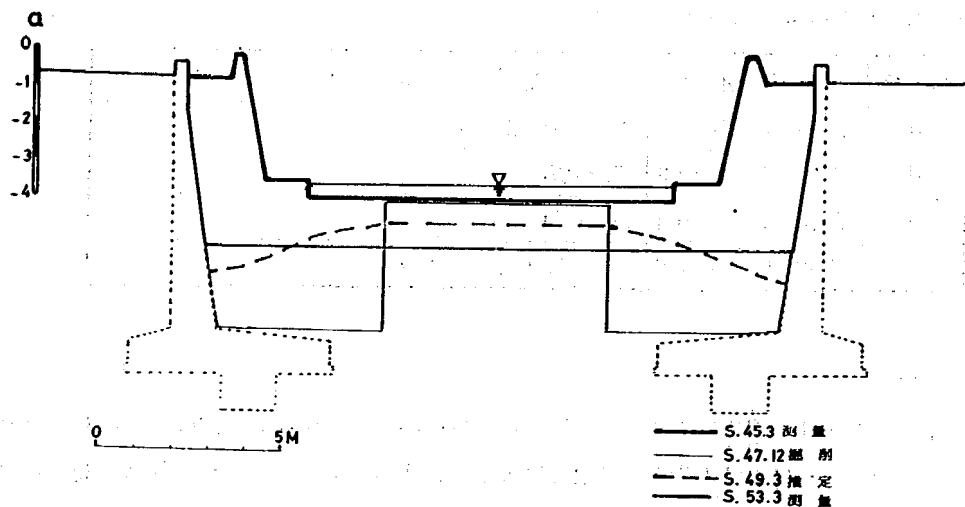
図1 根村橋観測所河川断面（同観測所上流8m地点）
