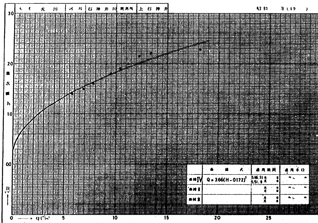
水位流量曲线图 IV
