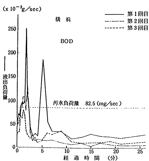
図4-7 BOD 流出負荷量
