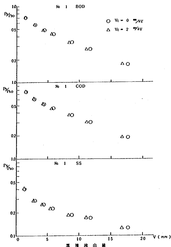
図 2-11 P_s/P_{so} と累積流出量の関係
