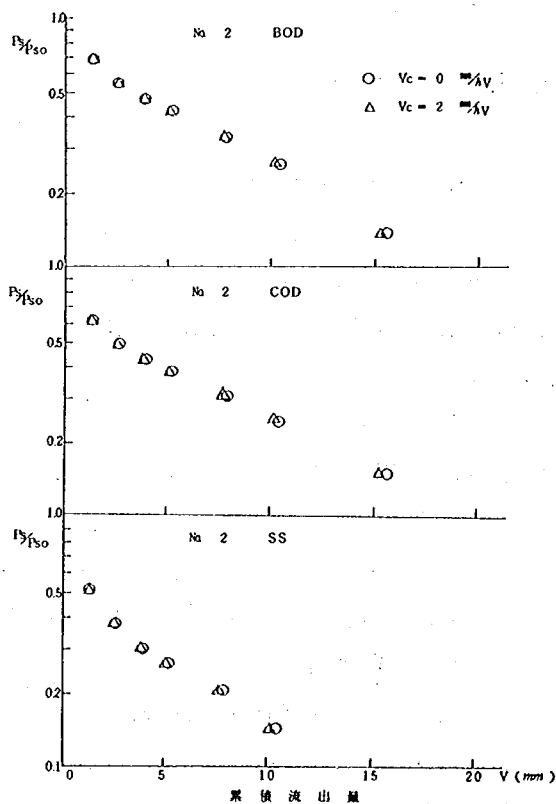
図 2-12 P_s/P_{so} と累積流出量の関係
