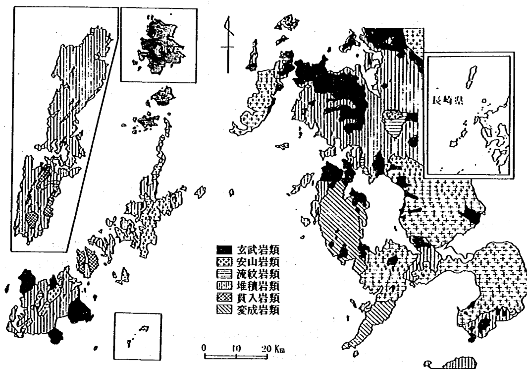
図2-2 長崎県の地質図
