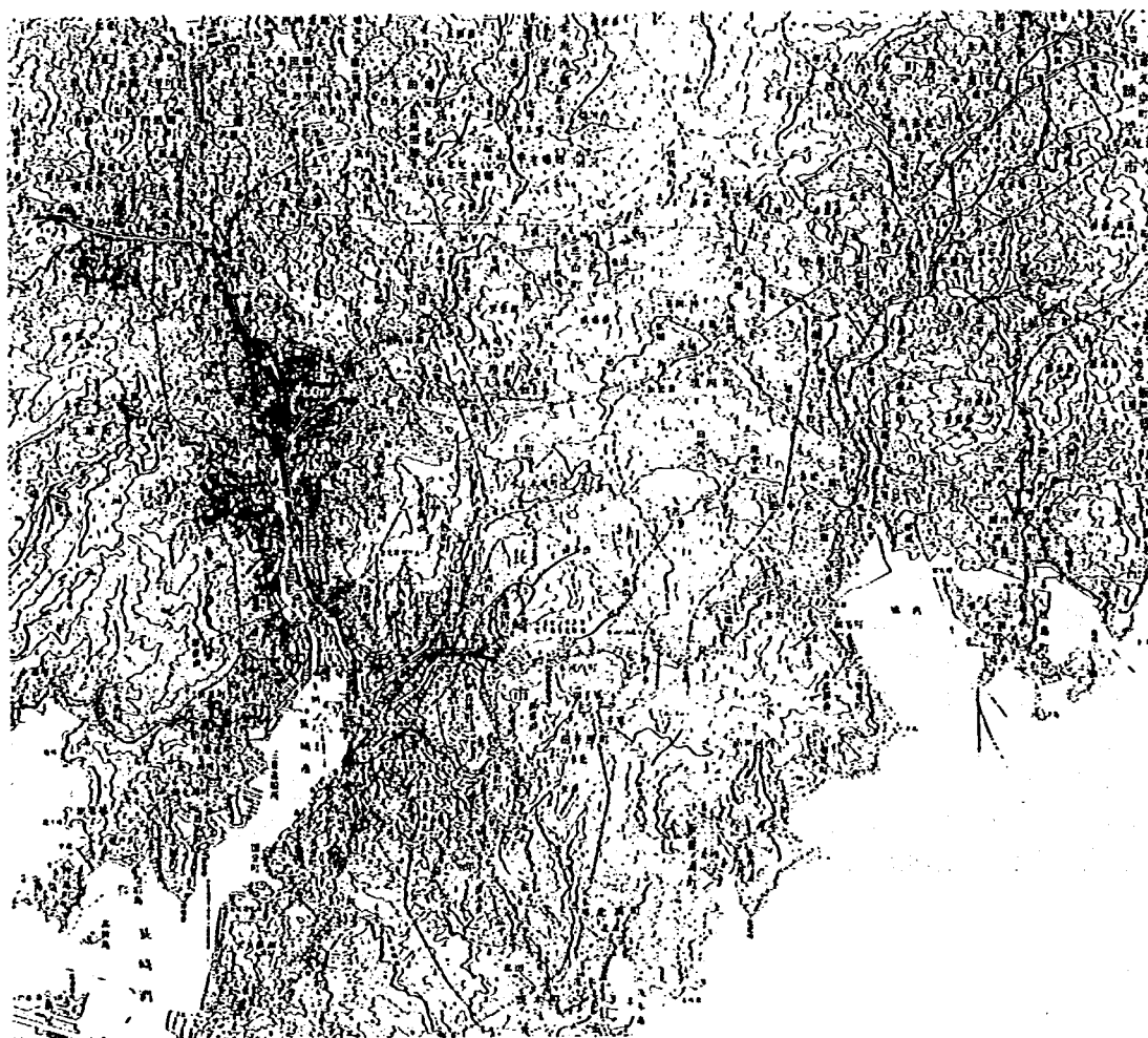
図2-1 長崎地区の地形
