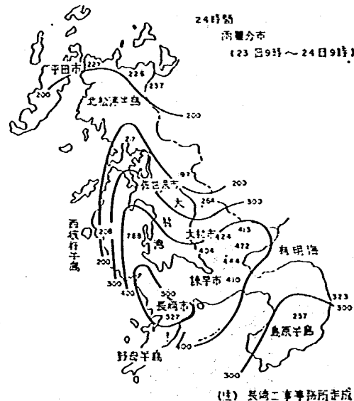
図2-3 長崎市の位置と本豪雨の雨量分布図(4)
