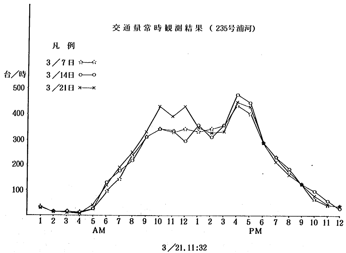
図-3.8 交通量の時間変化
