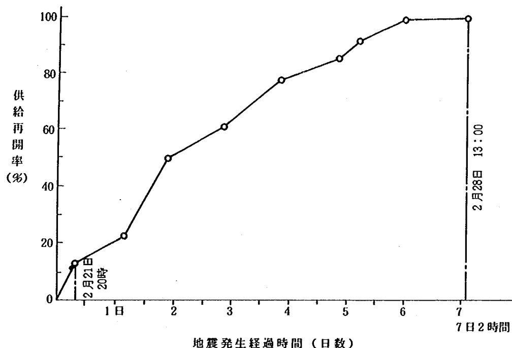
図-4.3 浦河町上水道の復旧経過
