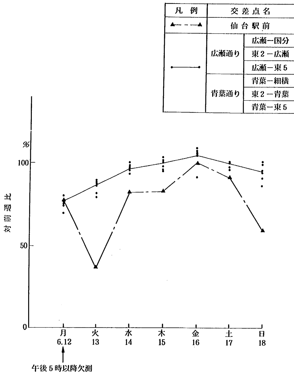
図－3.6 仙台市内主要交差点流入交通量変化（宮城県沖地震）
