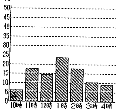
% 冒険コース
