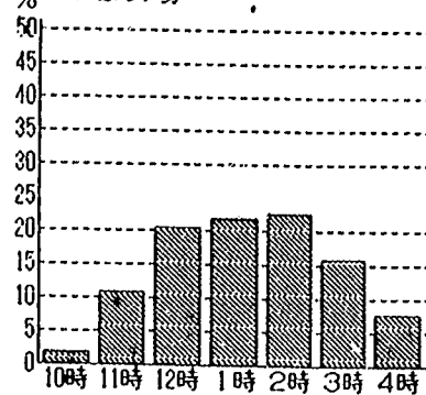
% 記念広場
