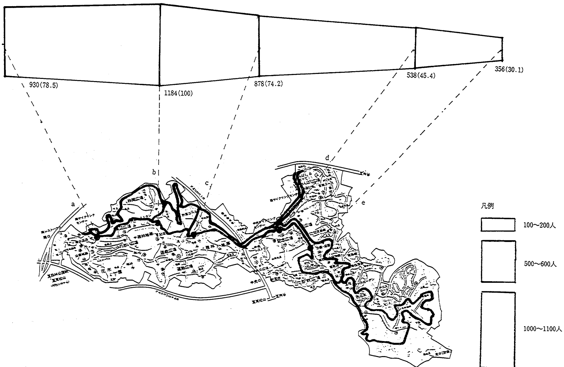
付図-21-② 12時
