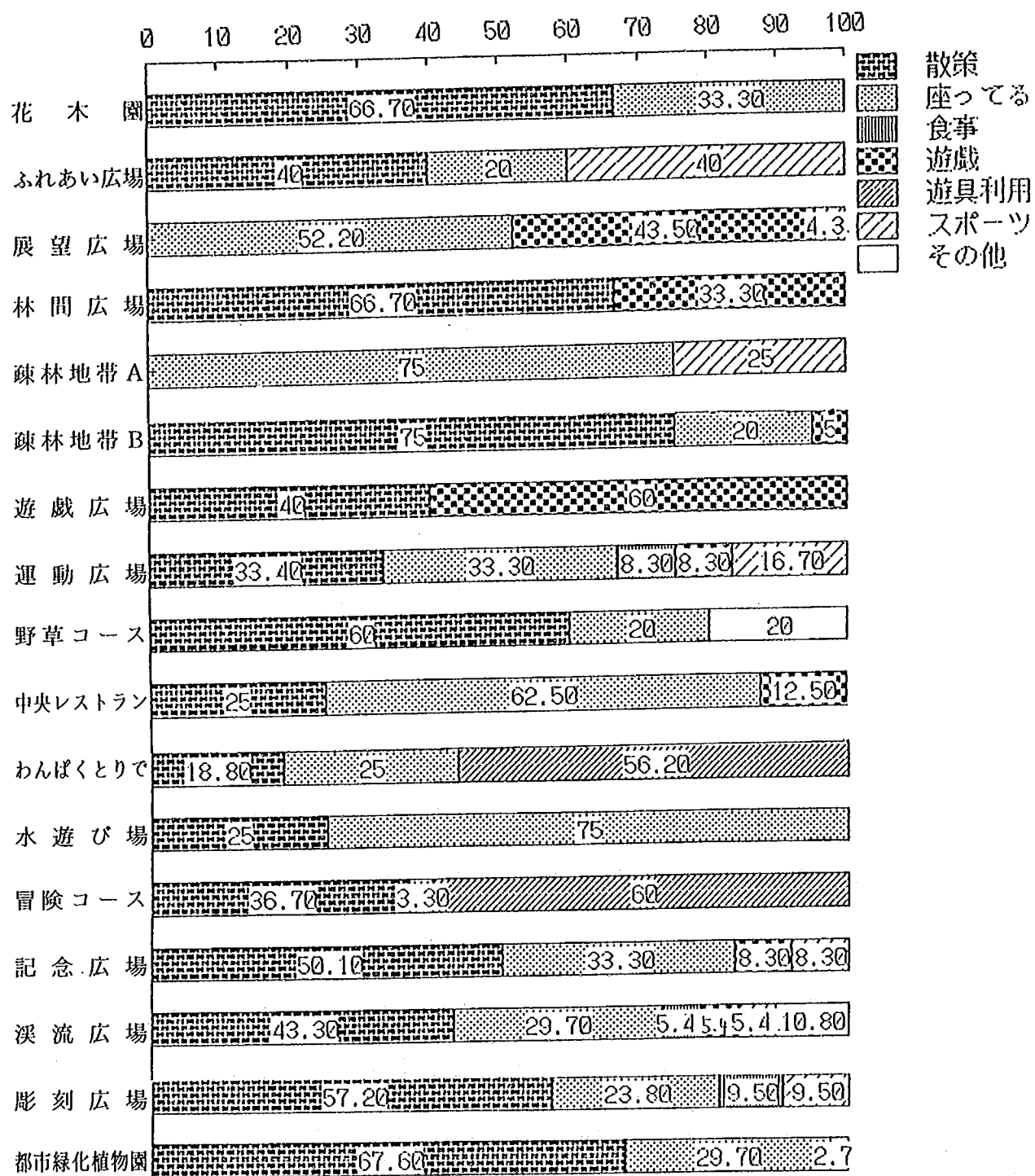
付図-18-④ 16:00
