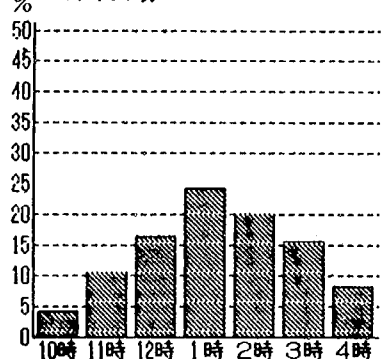
% 彫刻広場
