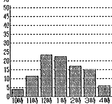
% 溪流広場
