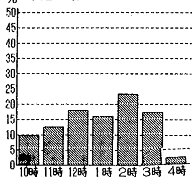
% 水遊び場
