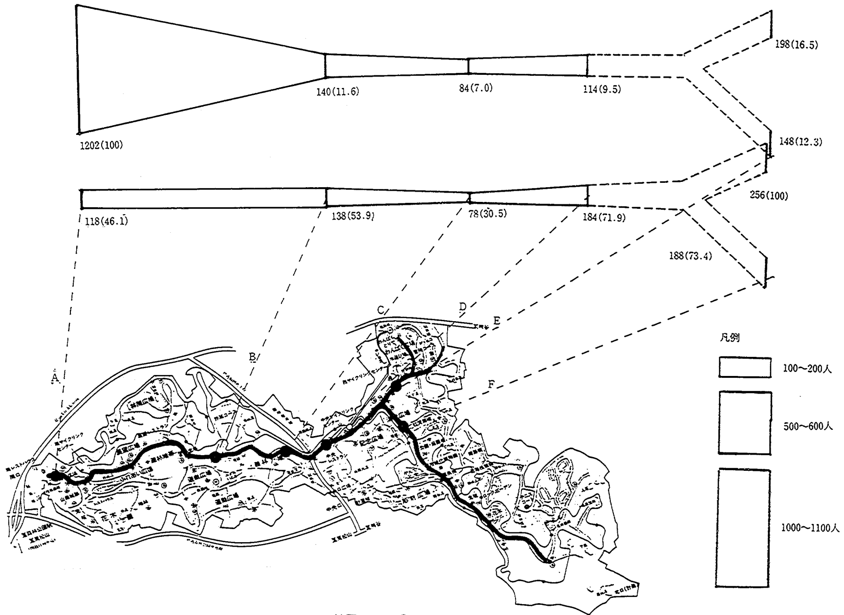
付図-20-② 12時
