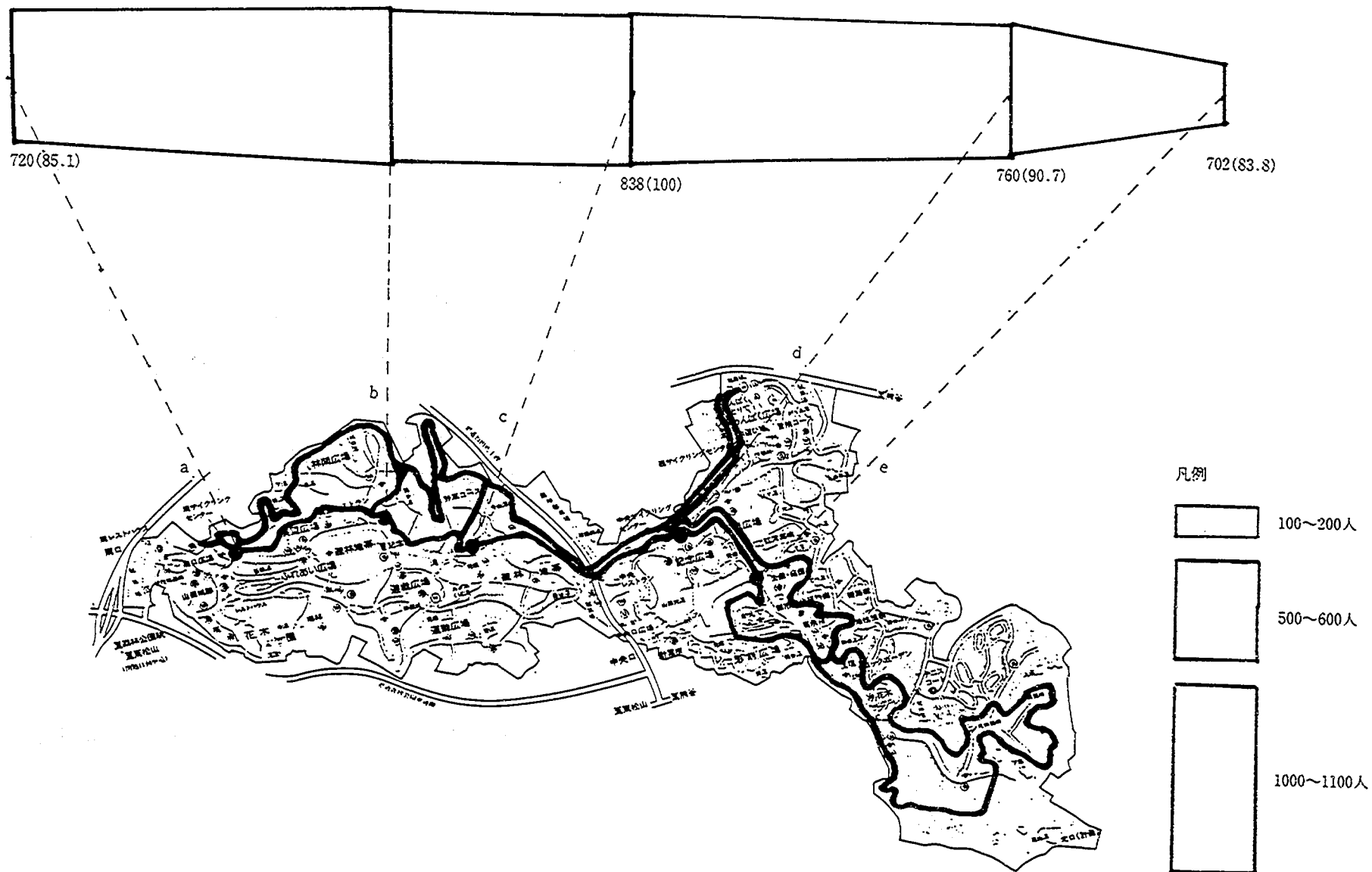
付図-21-③ 14時
