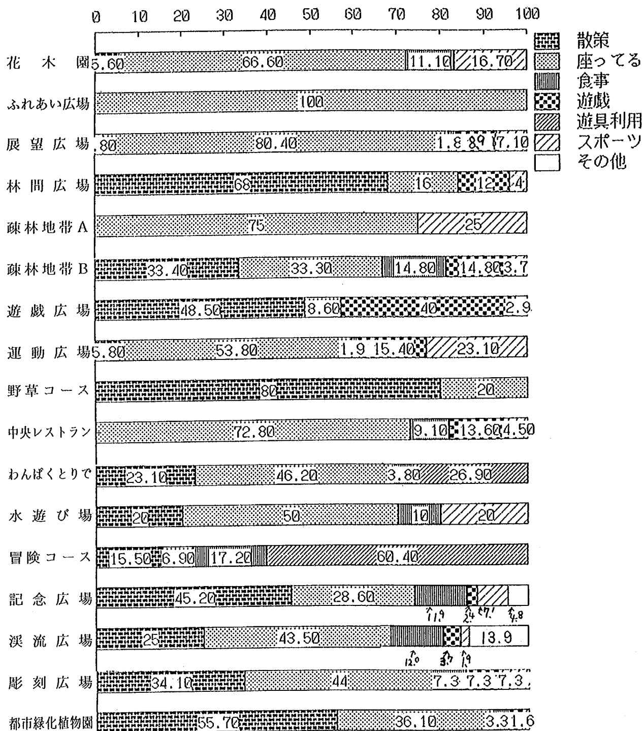
付図-18-③ 14:00
