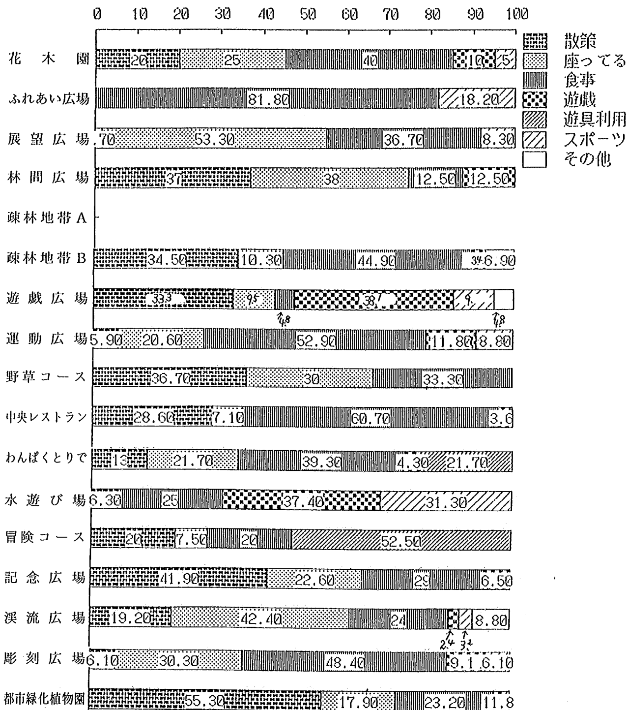
付図-18-② 12:00
