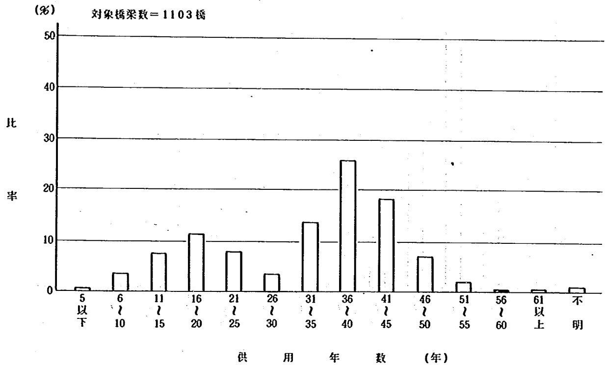
図-1-1 RC橋の供用年数
