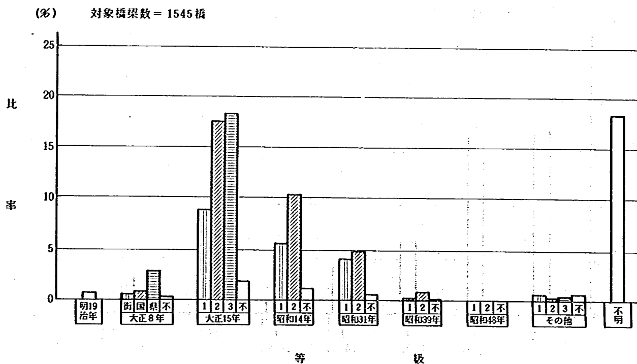
図-5-4 全橋の等級(示方書別)
