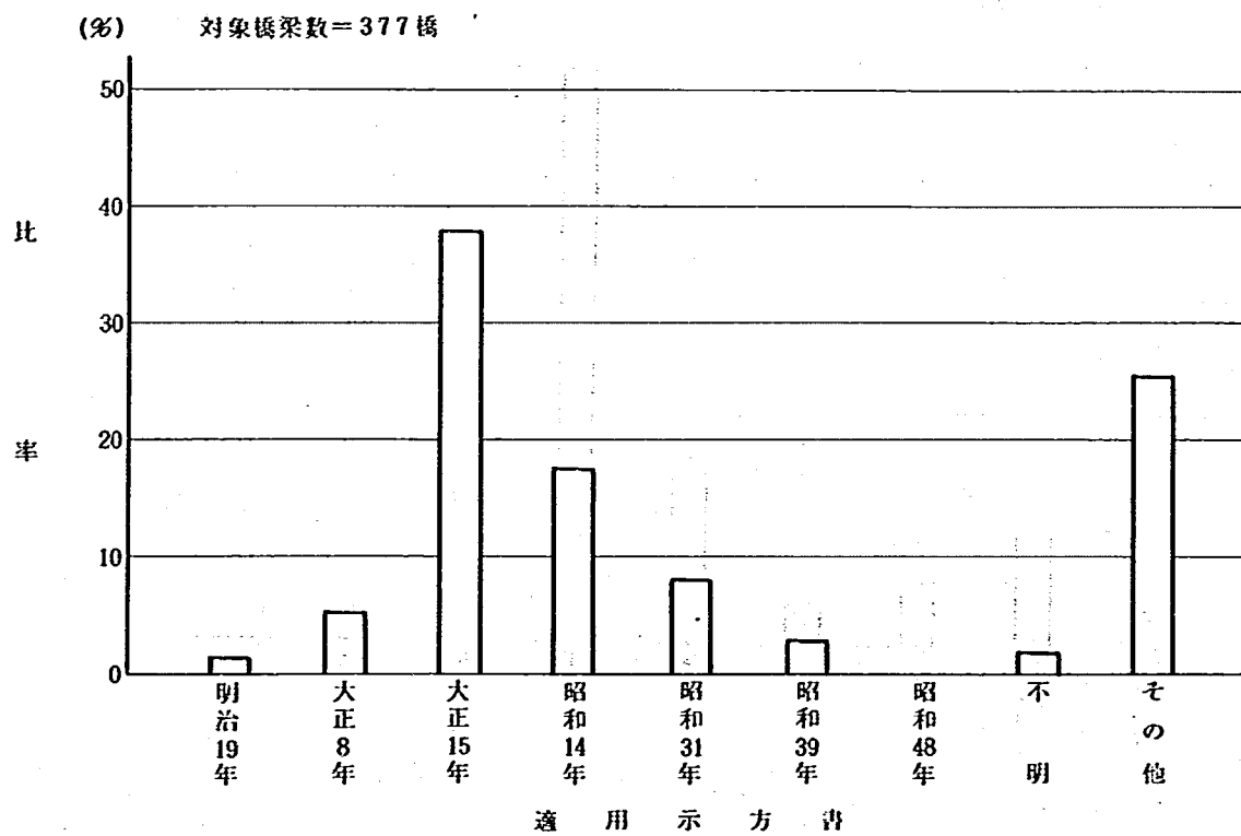
図-4-2 鋼橋の適用示方書
