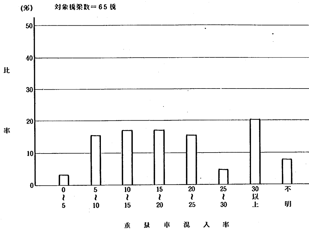
図-7-3 PC橋の重量車混入率
