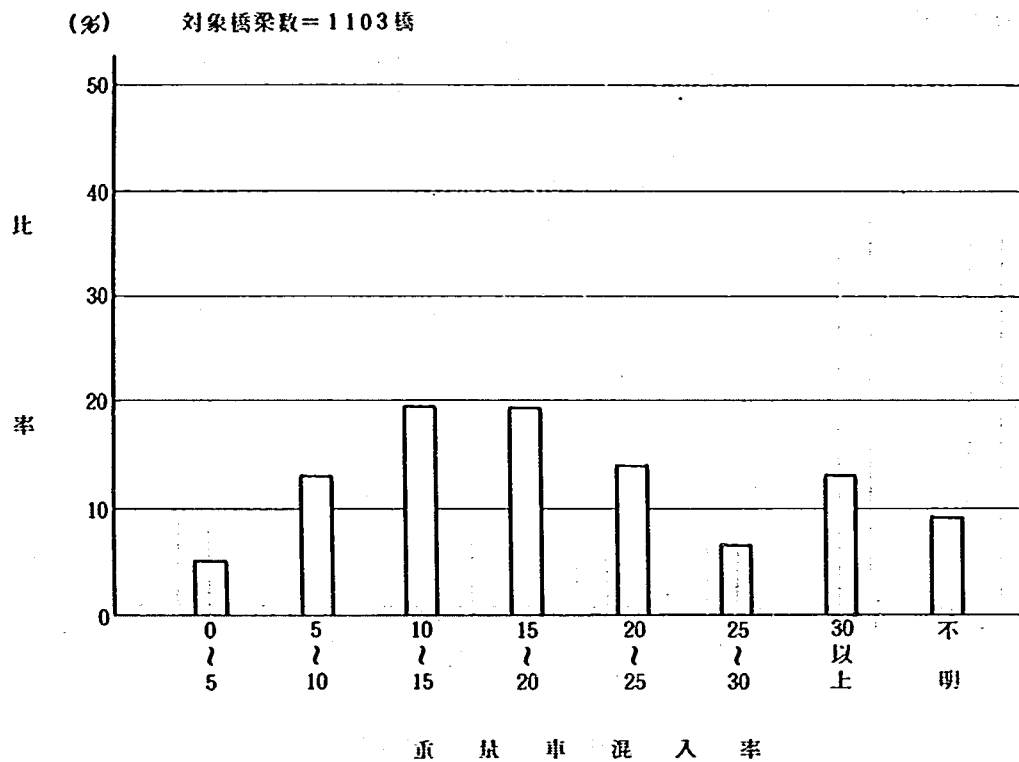
図-7-1 RC橋の重量車混入率
