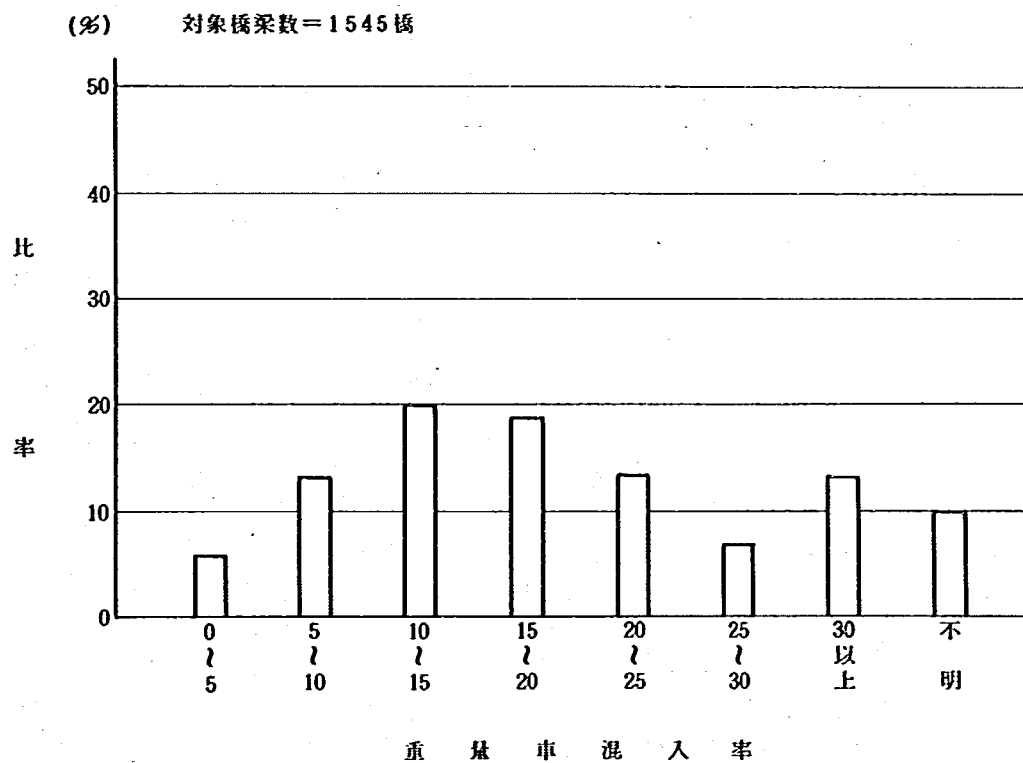
図-7-4 全橋の重量車混入率
