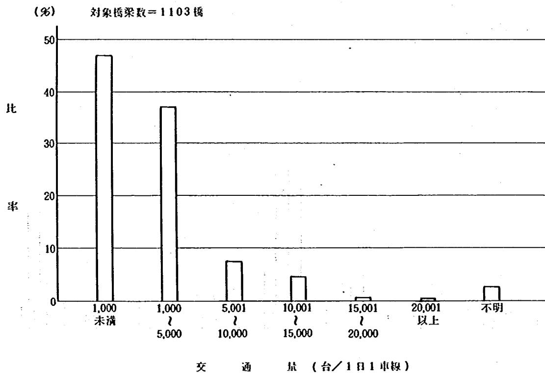
図-6-1 RC橋の交通量
