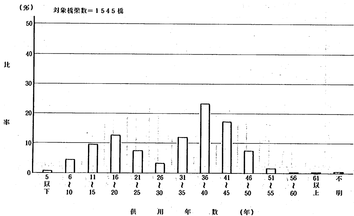
図-1-4 全橋の供用年数
