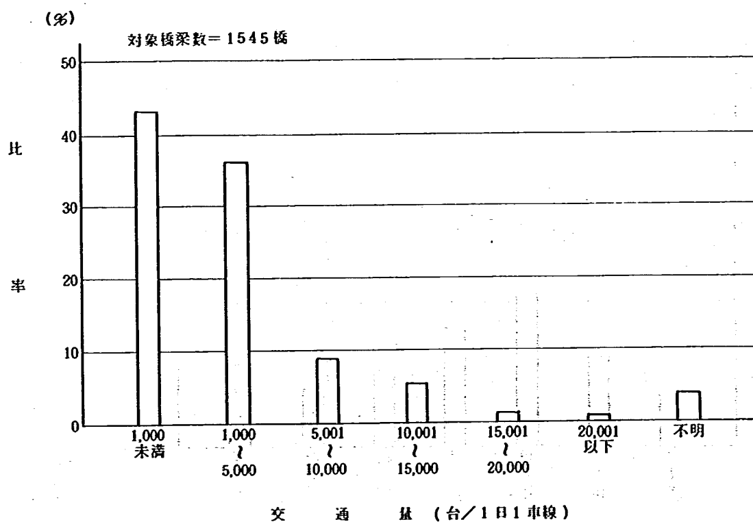
図-6-4 全橋の交通量
