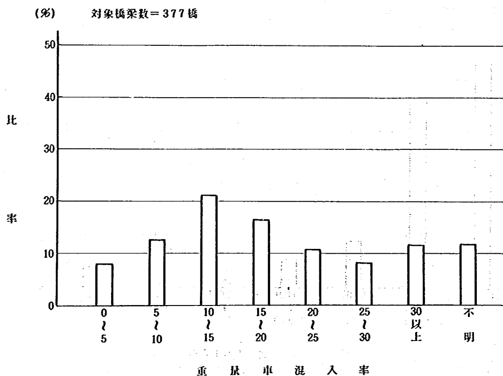
図-7-2 鋼橋の重量車混入率
