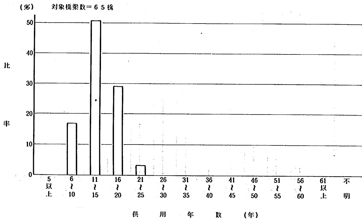
図-1-3 PC橋の供用年数
