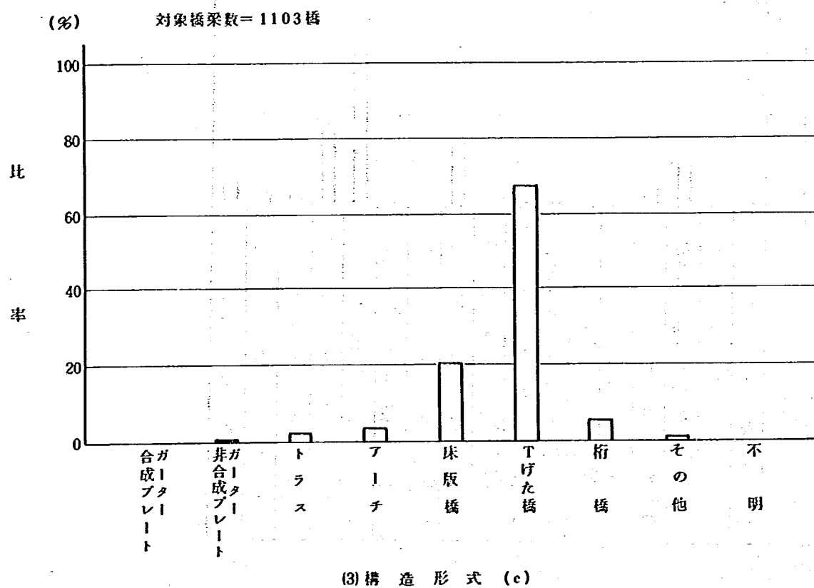
図-3-1 RC橋の構造形式
