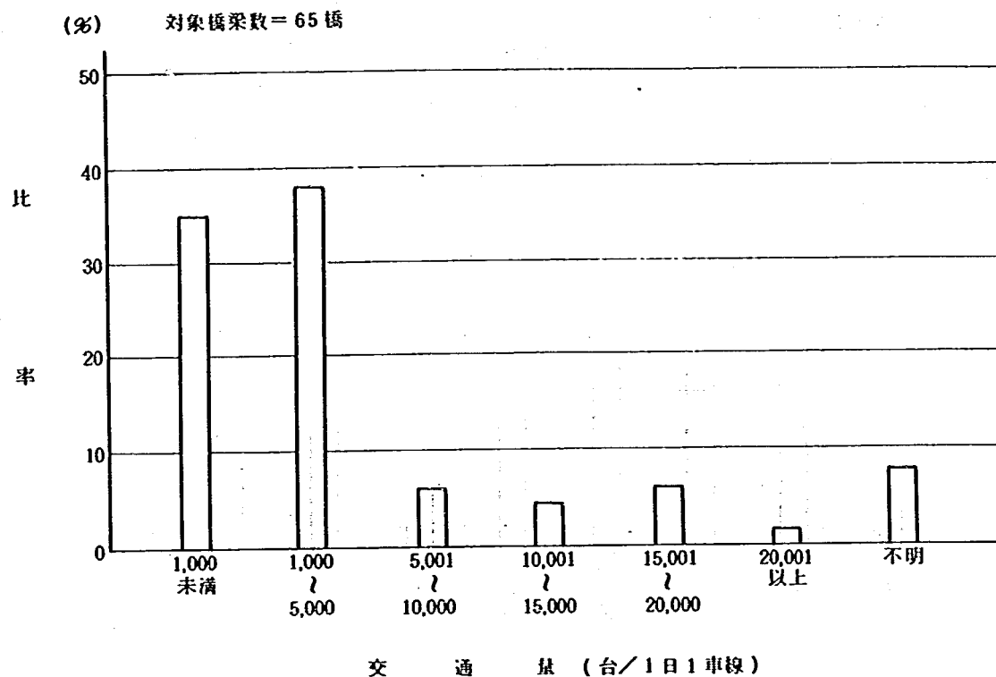
図-6-3 PC橋の交通量
