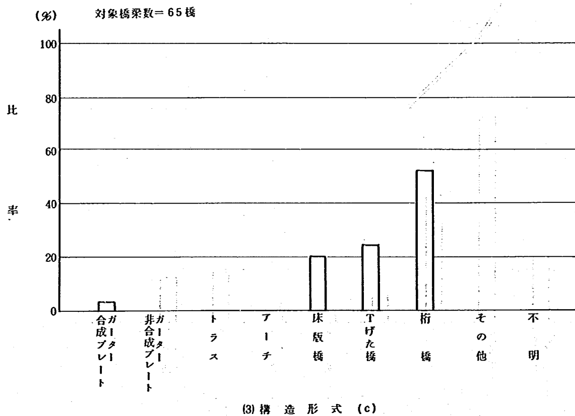
図-3-3 PC橋の構造形式
