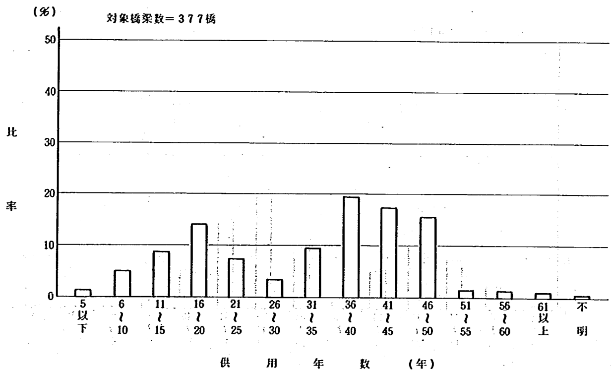
図-1-2 鋼橋の供用年数
