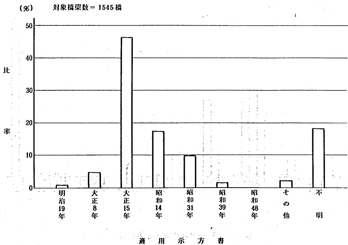
図-4-4 全橋の適用示方書
