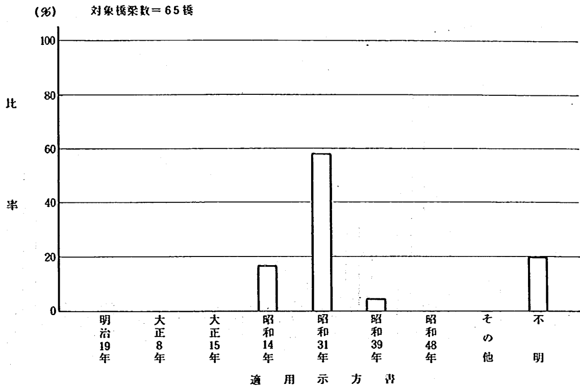
図-4-3 PC橋の適用示方書
