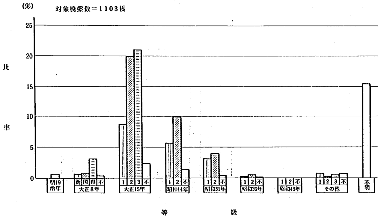
図-5-1 RC橋の等級(示方書別)
