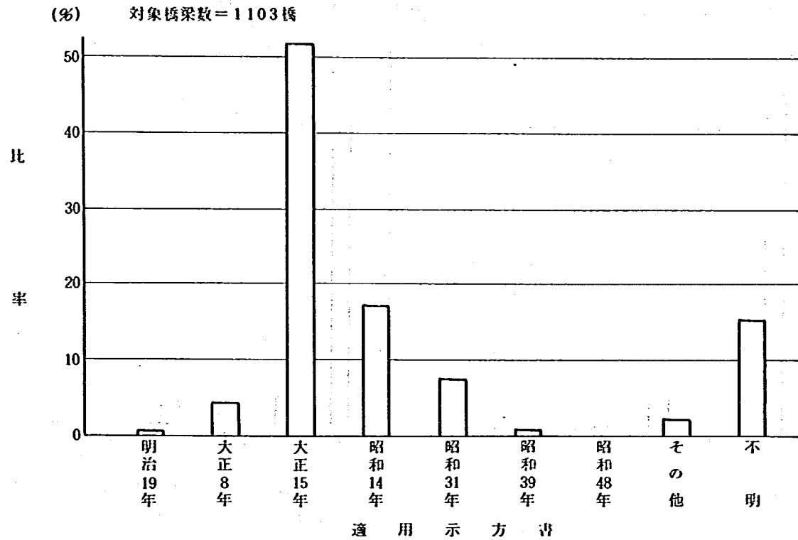
図-4-1 RC橋の適用示方書
