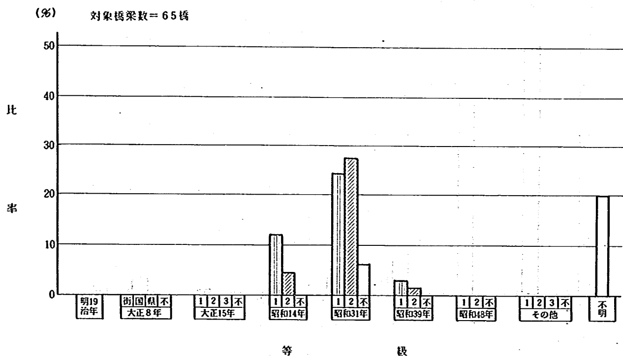
図-5-3 PC橋の等級(示方書別)
