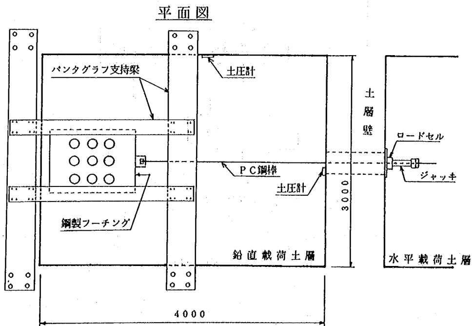
図-2.1.2 実験概要図
