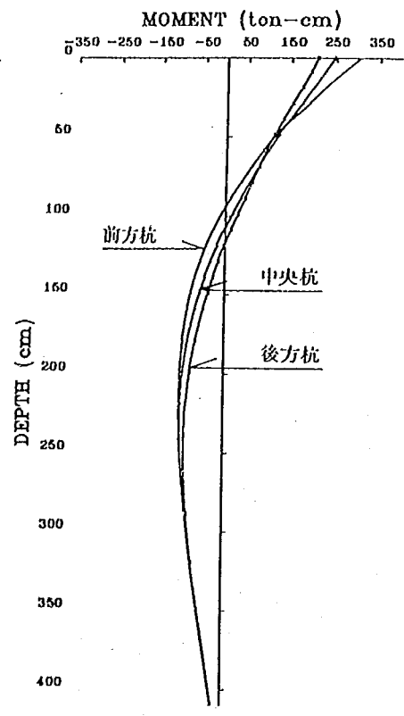
図-3.2.6 曲げモーメント分布図 (9本組杭・中央杭)
