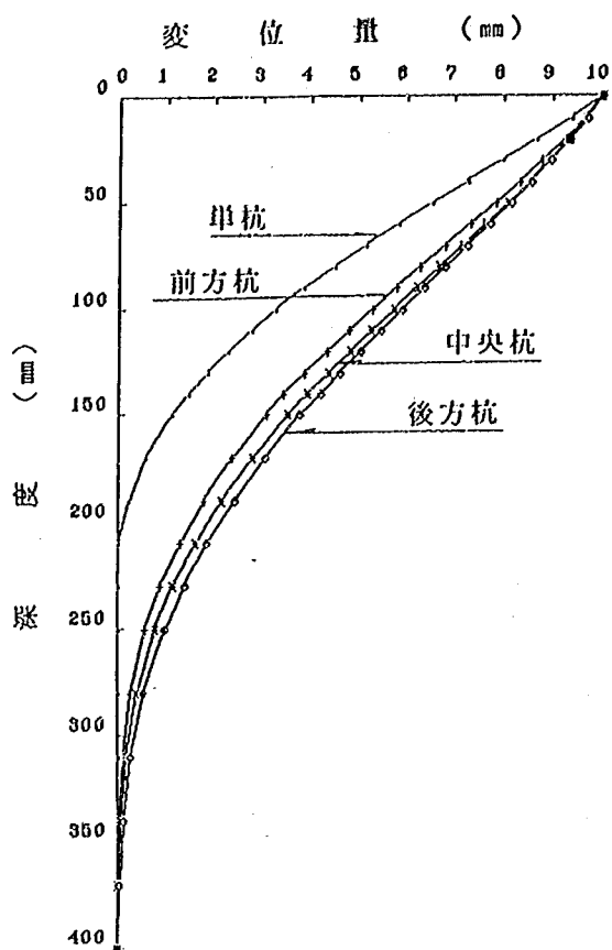
図一3.3.5 杭体変位の比較 (9本組杭・中央列) 【地表面変位量 10mm時】
