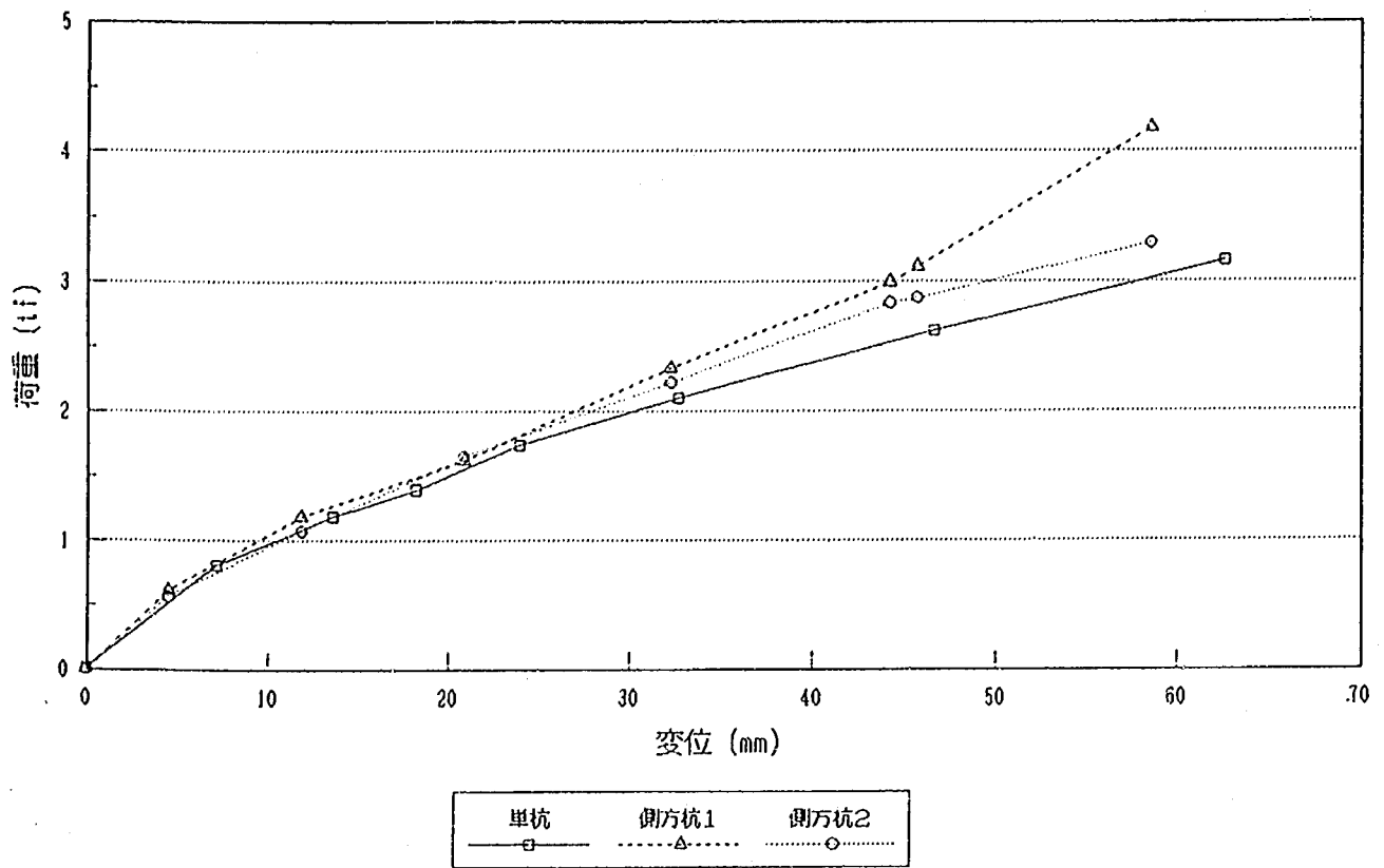
图—3.1.8 杭頭荷重—變位量曲線（2本並列杭）
