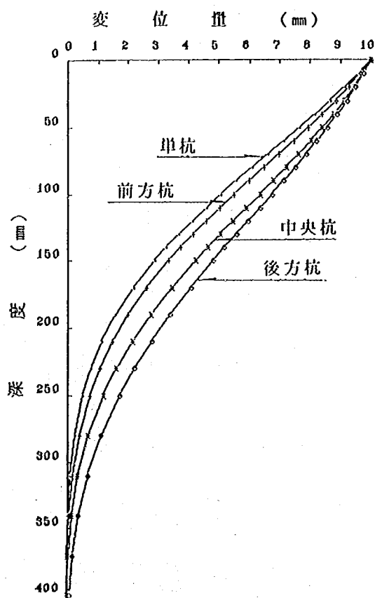
図一 3.3.3 杭体変位の比較 (3本直列杭) 【地表面変位量 10mm時】
