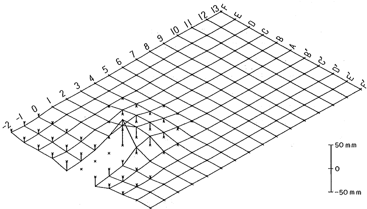
圖—3.6.2 地表面變位觀察圖（3本直列杭）
