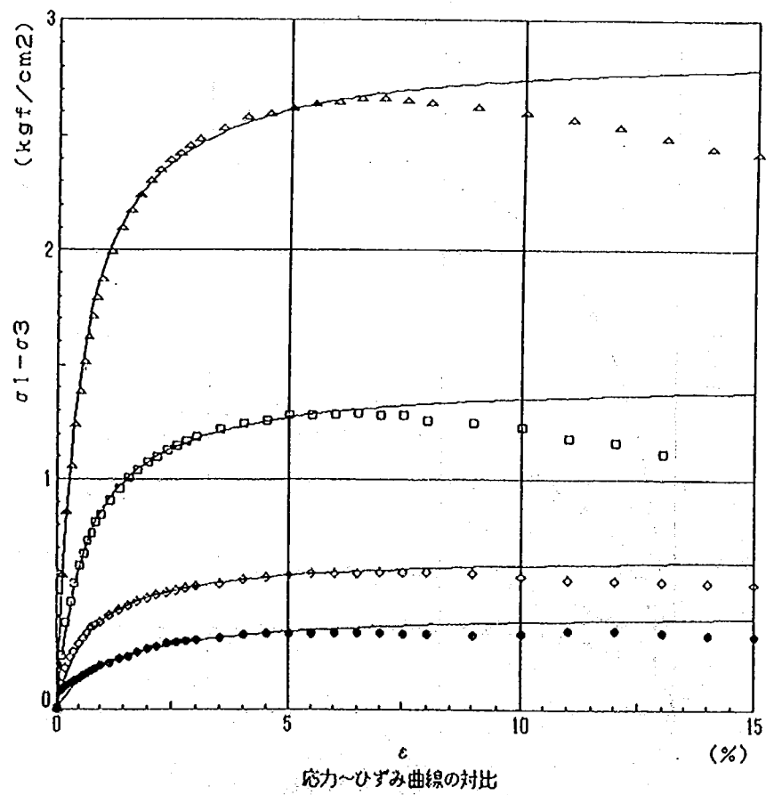
図一参一2.2 三軸圧縮試験の双曲線近似 (CASE1 0.5 m)
