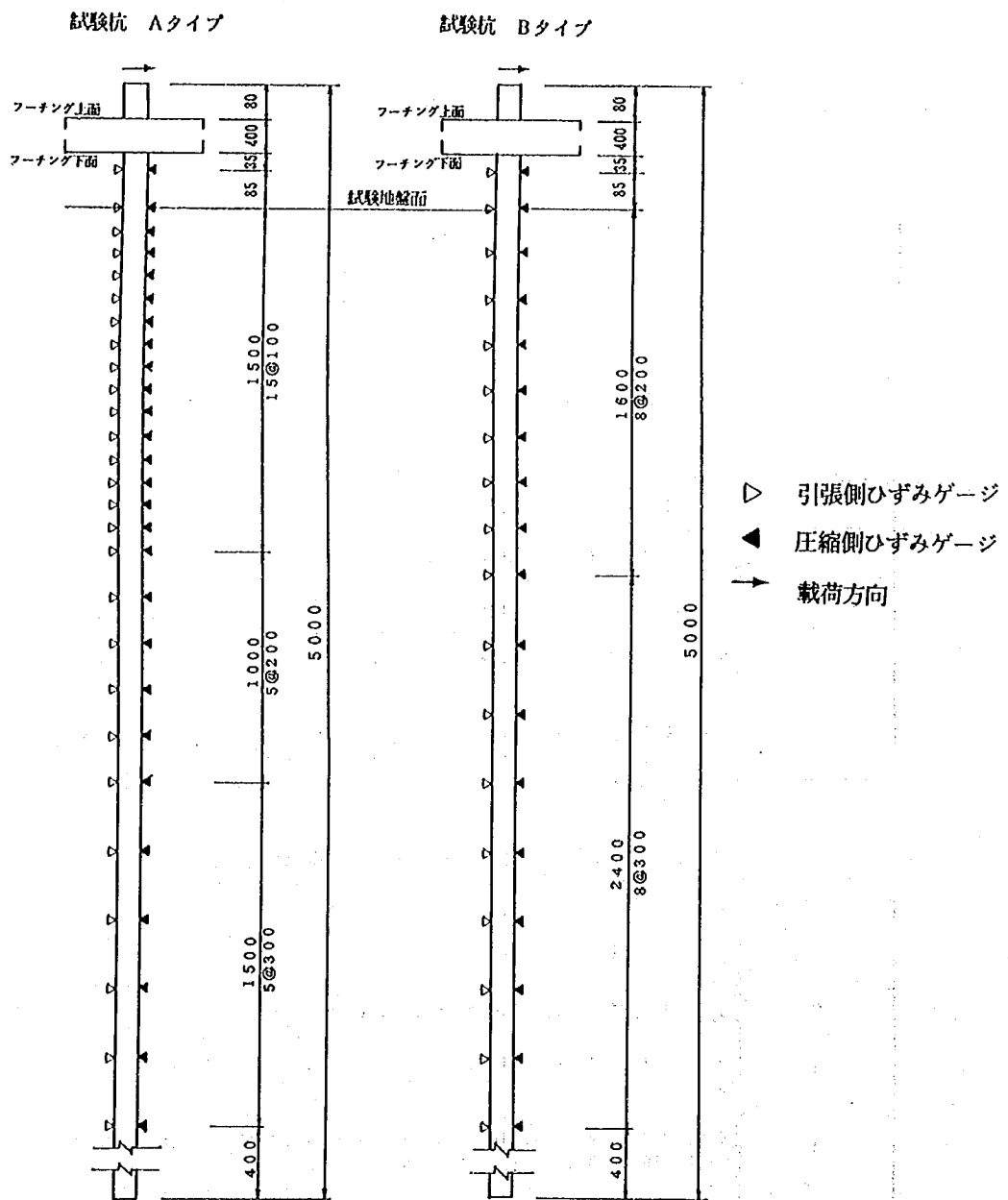
図-2.7.1 杭体ひずみの計測位置
