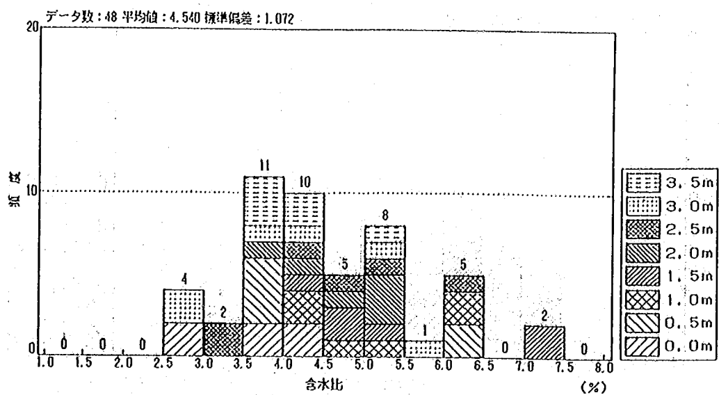
図一参-2.21 三軸圧縮試験 \sigma_t , \rho_d W の頻度分布図 (CASE 2)
