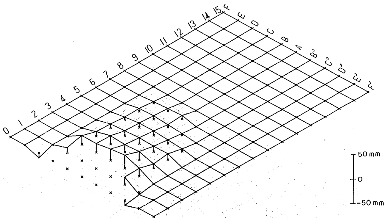
図-3.6.1 地表面変化観察図（3本並列杭）
