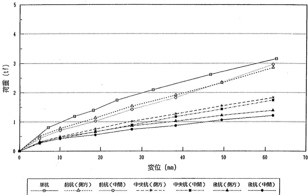
図—3. 1.12 杭頭荷重—変位置曲線（9本組杭）
