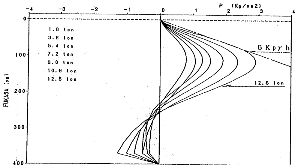
図一 3.4.12 地盤反力度分布 (3本並列・中央杭)
