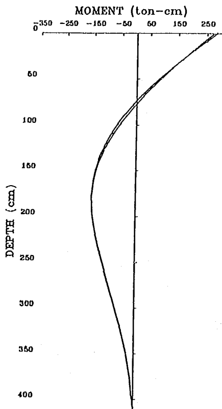
図-3.2.4 曲げモーメント分布図 (3本並列杭)
