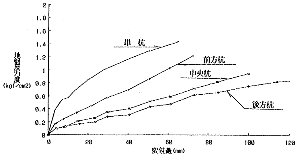
図一 3.4.28 地盤のP～y曲線比較 (9本組杭・中央列) 【深度GL-0.5 m】
