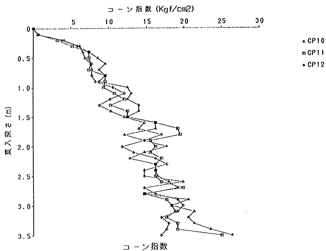
図一参一 2.30 コーン指数 (CP10~12)
