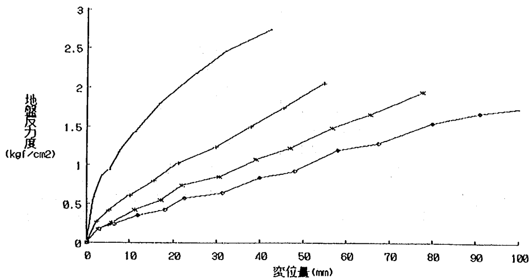
図一 3.4.29 地盤のP～y曲線比較 (9本組杭・中央列) 【深度GL-1.0 m】
