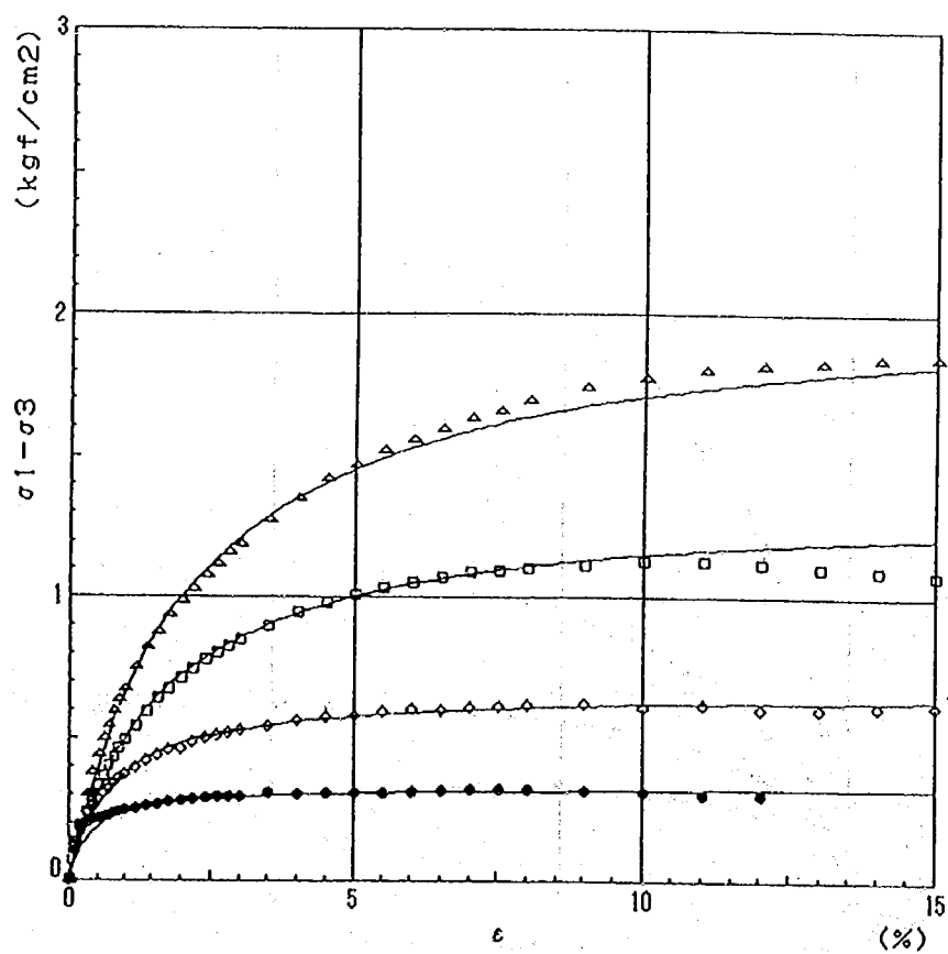
図一参一 2.10 三軸圧縮試験の双曲線近似 (CASE 5 0.5 m)
