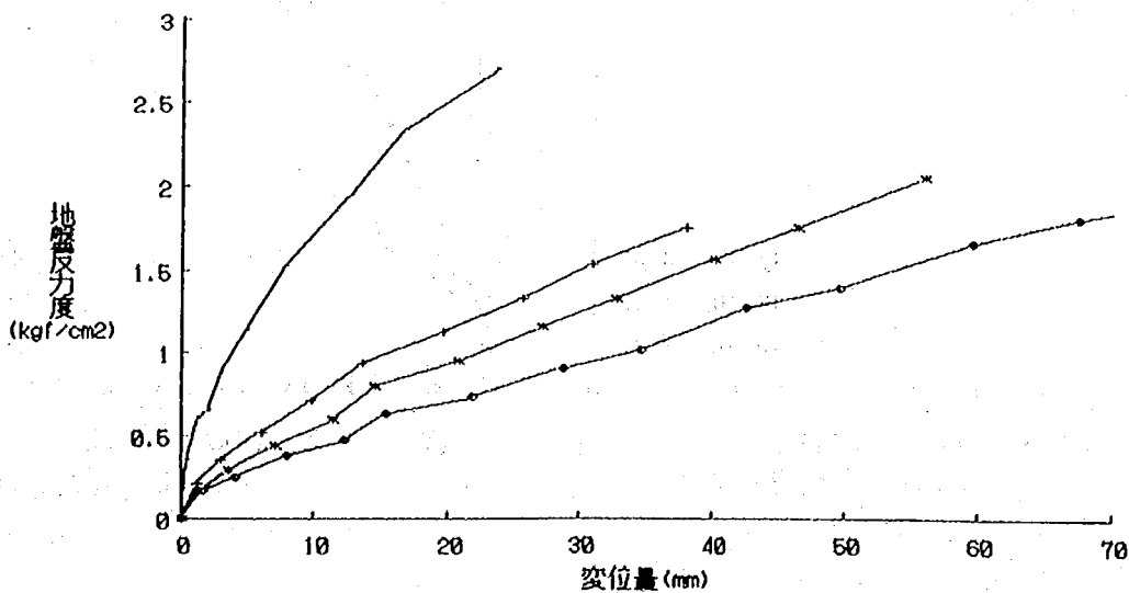
図一 3.4.30 地盤のP～y曲線比較 (9本組杭・中央列) 【深度GL-1.5 m】
