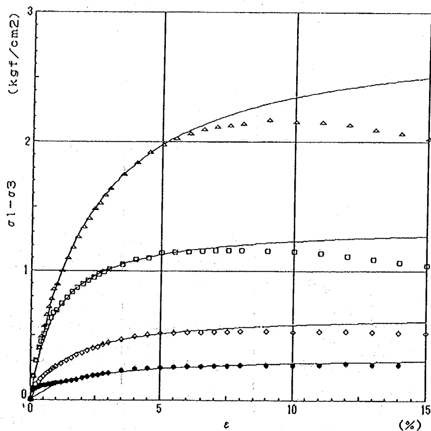
図一参-2.4 三軸圧縮試験の双曲線近似 (CASE 2 0.5 m)
