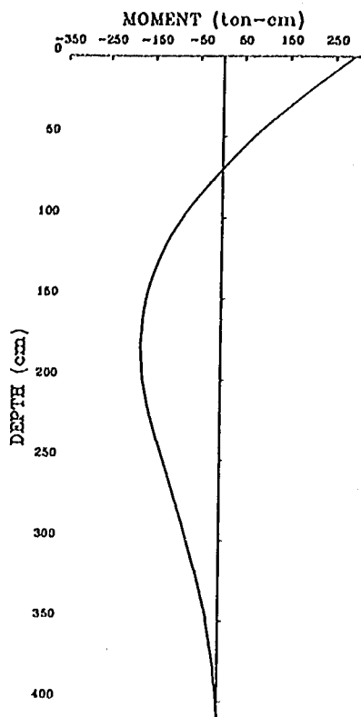
図-3.2.1 曲げモーメント分布図 (単杭)
