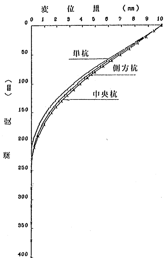
図一 3.3.1 杭体変位の比較 (3本並列杭) 【地表面変位量 10mm 時】
