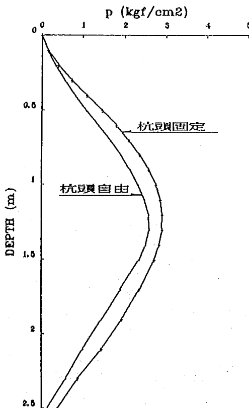
図-4.3.2 地盤反力度分布比較図
