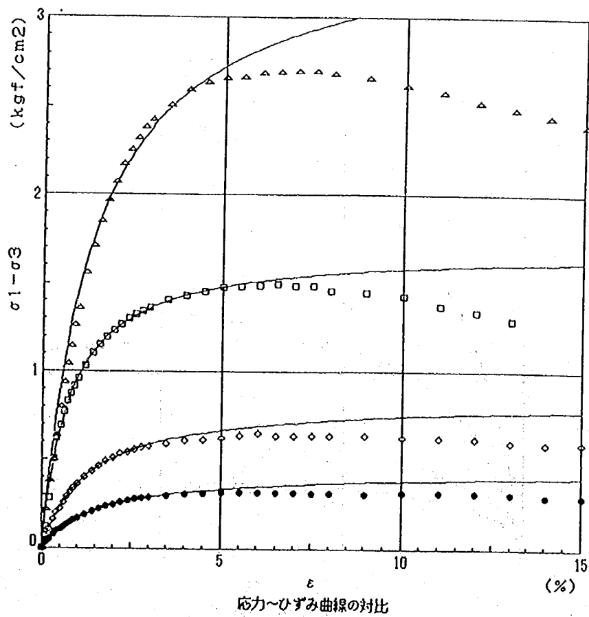
図一参—2.6 三軸圧縮試験の双曲線近似 (CASE 3 0.5 m)
