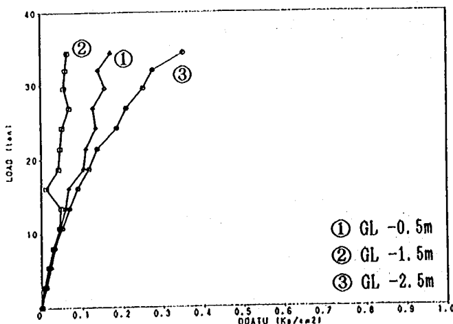
図-3.5.3 荷重-側圧曲線 (9本組杭・載荷方向壁)
