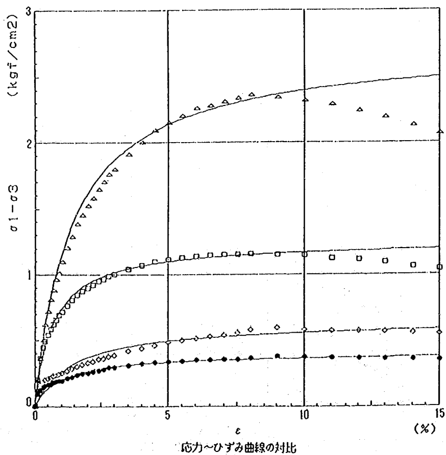
図一参一2.13 三軸圧縮試験の双曲線近似 (CASE 6 1.0 m)
