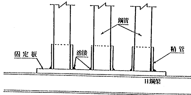
図-2.5.2 杭先端部の固定方法(断面図)
