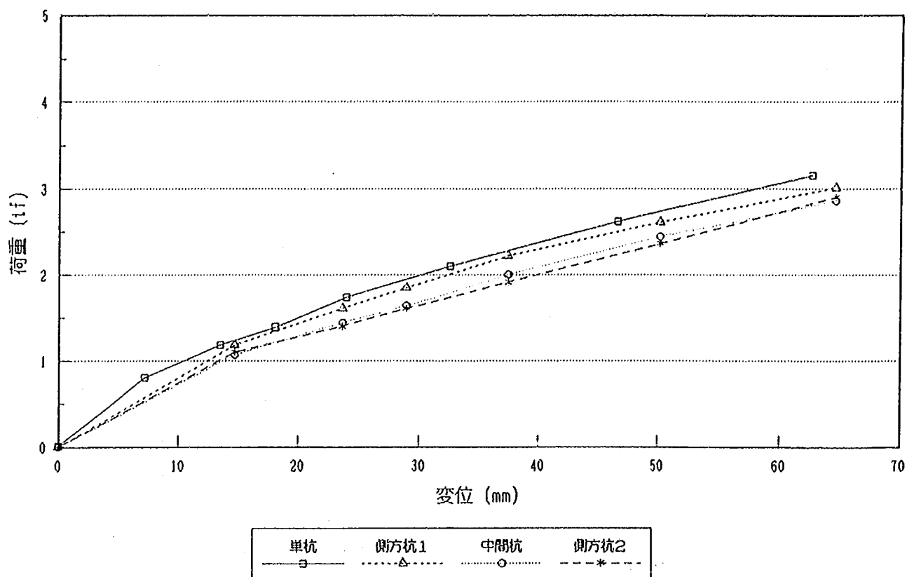
图— 3. 1.10 杭頭荷重—変位量曲線 (3 本並列杭)
