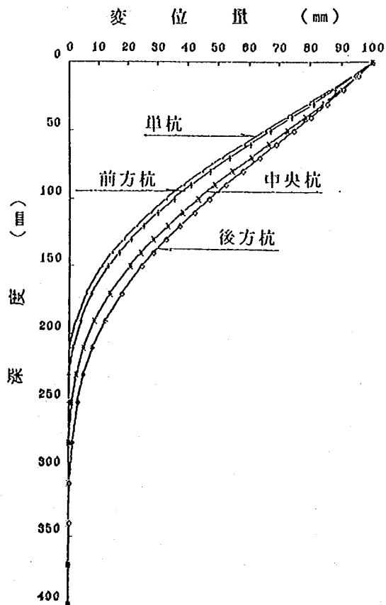
図一 3.3.4 杭体変位の比較 (3本直列杭) 【地表面変位量 100mm時】
