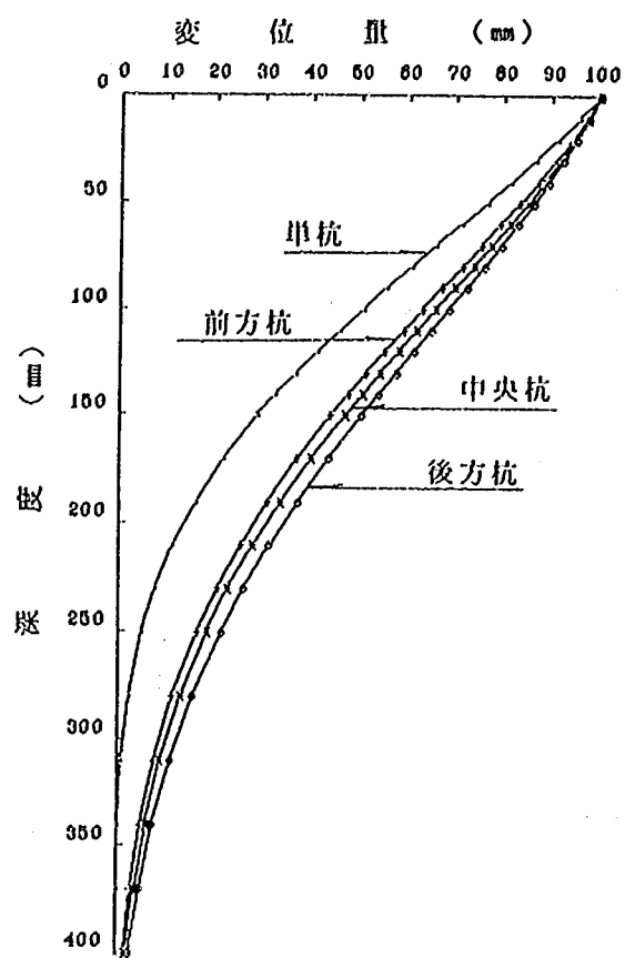
図一3.3.6 杭体変位の比較 (9本組杭・中央列) 【地表面変位量 100mm時】
