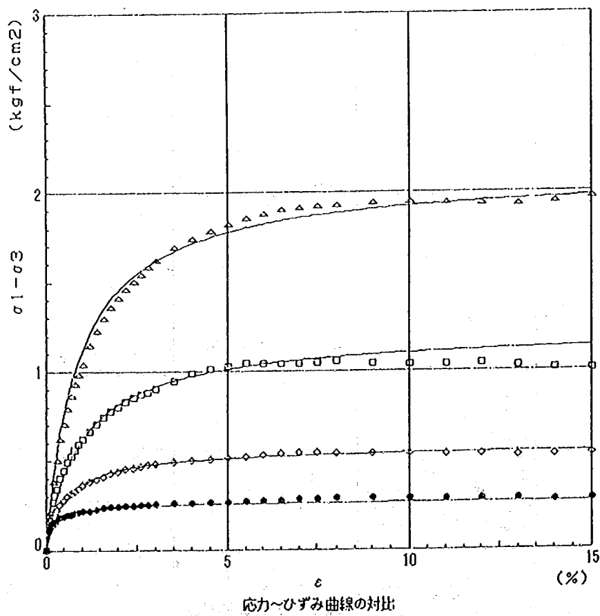
図一参—2.5 三軸圧縮試験の双曲線近似 (CASE2 1.0 m)
