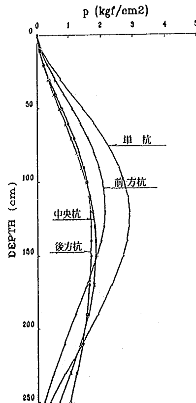
圖—3.4.5 地盤反力度分布比較 (9本組杭・側方列)
