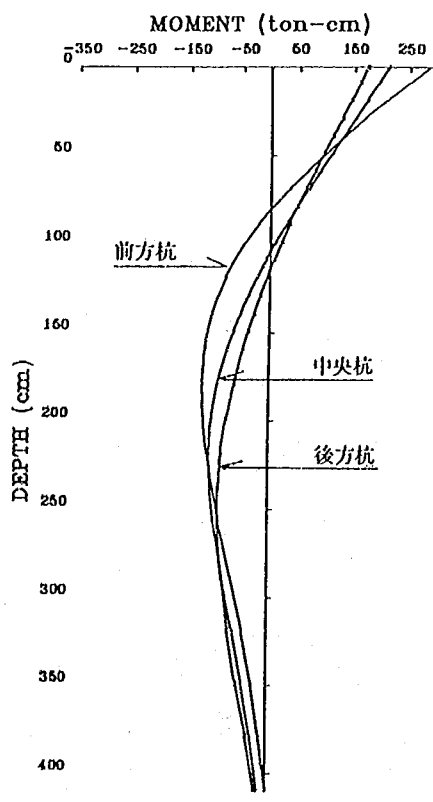
図-3.2.5 曲げモーメント分布図 (3本直列杭)
