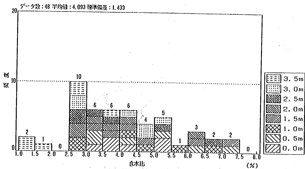
図一参-2.25 三軸圧縮試験 \sigma_t , \rho_d W の頻度分布図 (CASE 6)
