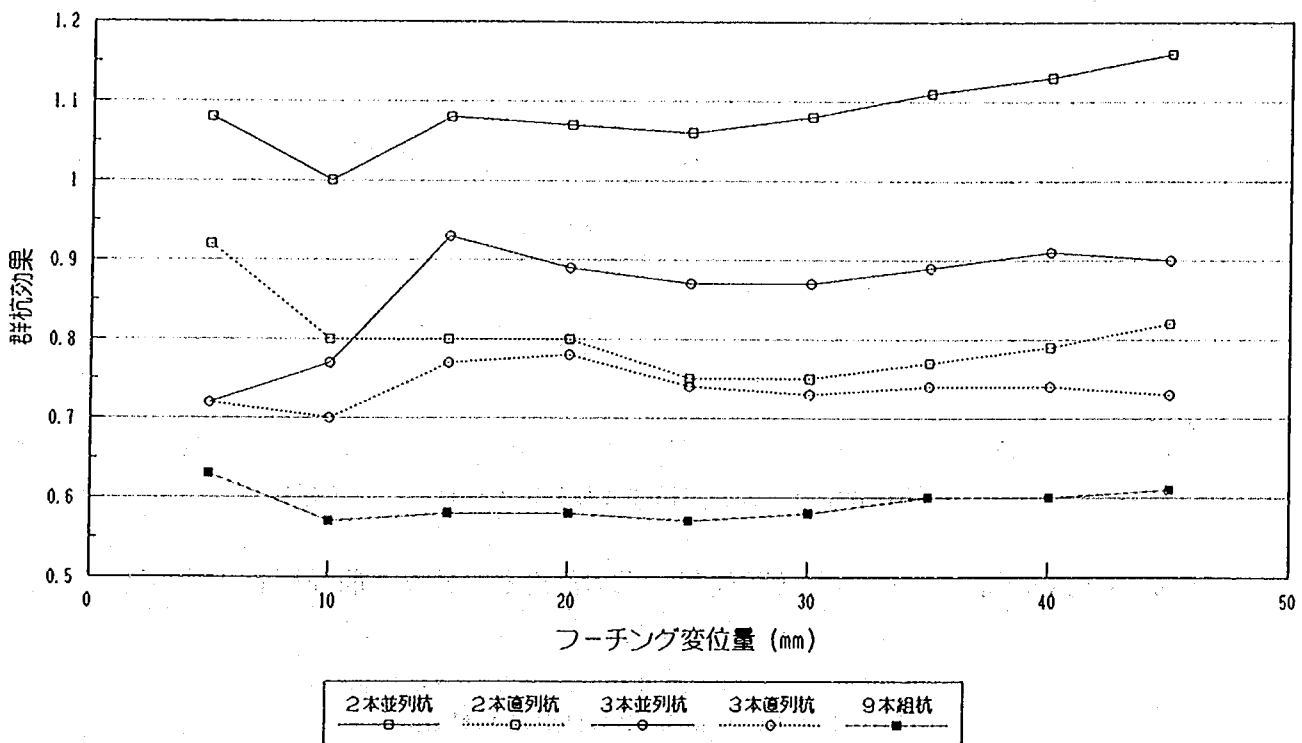
図-4.1.1 群杭効率
