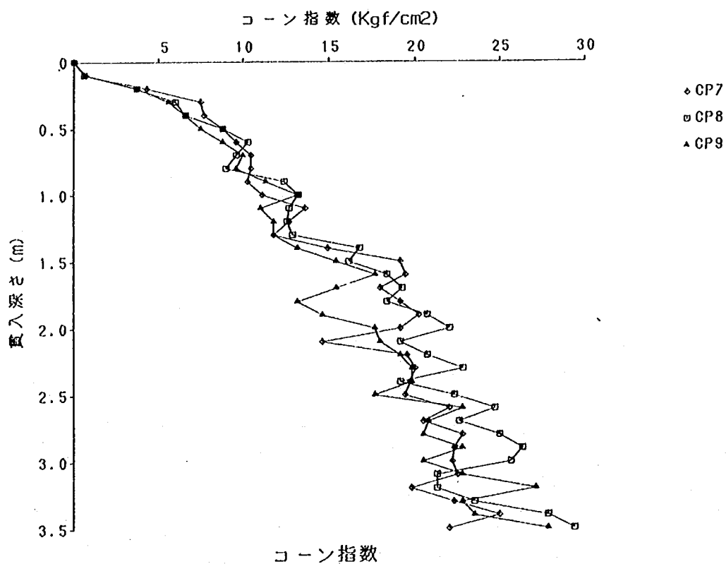
図一参-2.29 コーン指数 (CP7~9)
