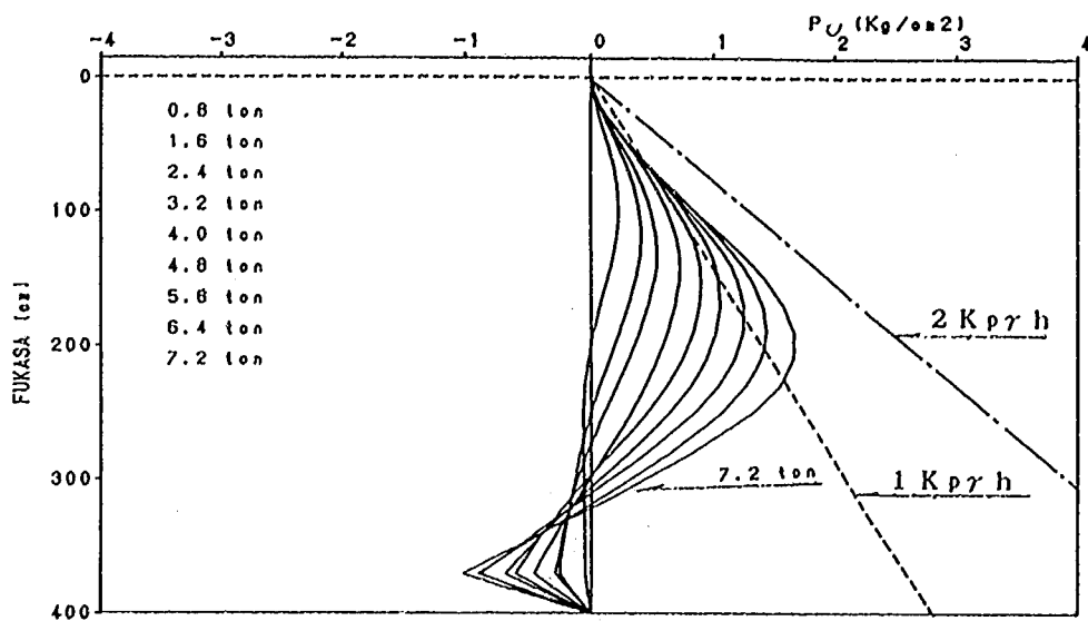
図一 3.4.10 地盤反力度分布 (2本直列・後方杭)
