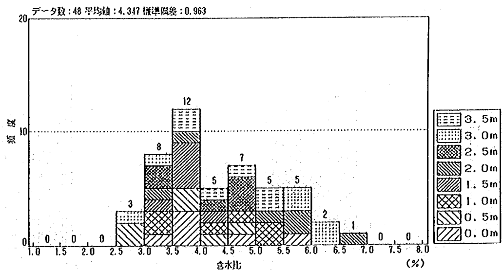
図一参一2.23 三軸圧縮試験 \sigma_t , \rho_d W の頻度分布図 (CASE 4)
