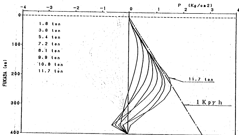
図一 3.4.15 地盤反力度分布 (3本直列・後方杭)
