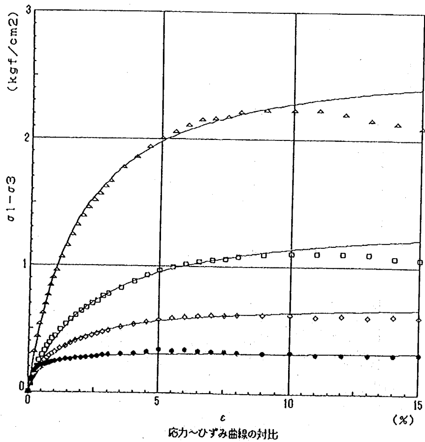
図一参-2.11 三軸圧縮試験の双曲線近似 (CASE5 1.0 m)
