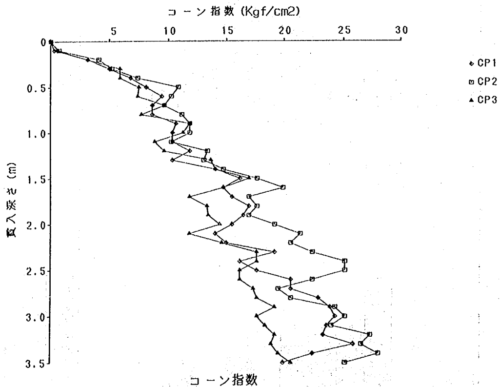
図一参-2.27 コーン指数 (CP1～3)
