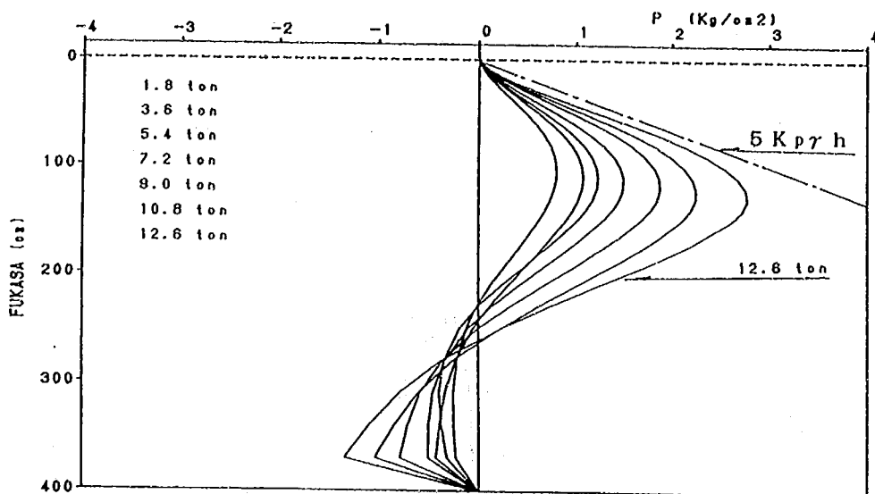
図一 3.4.11 地盤反力度分布 (3本並列・側方杭)
