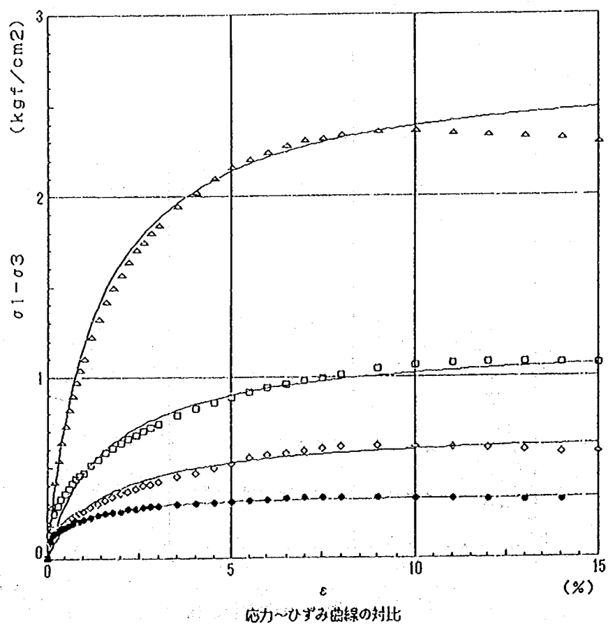
図一参一 2.9 三軸圧縮試験の双曲線近似 (CASE 4 1.0 m)
