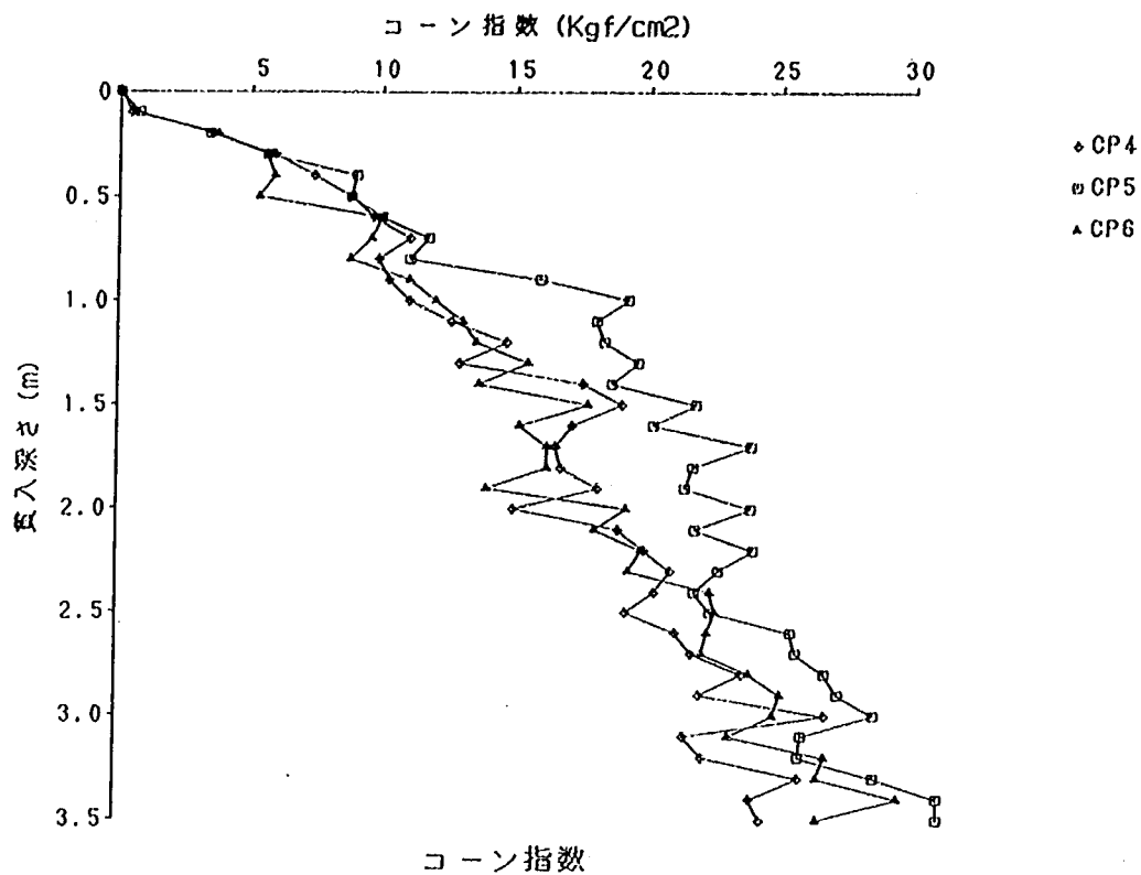
図一参-2.28 コーン指数 (CP4~6)
