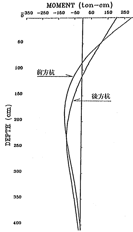
図-3.2.3 曲げモーメント分布図 (2本直列杭)
