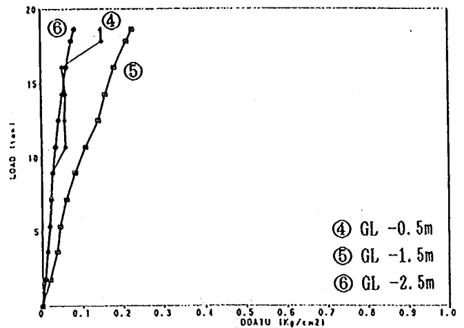
図-3.5.2 荷重-側圧曲線 (3本並列杭・載荷直角方向壁)
