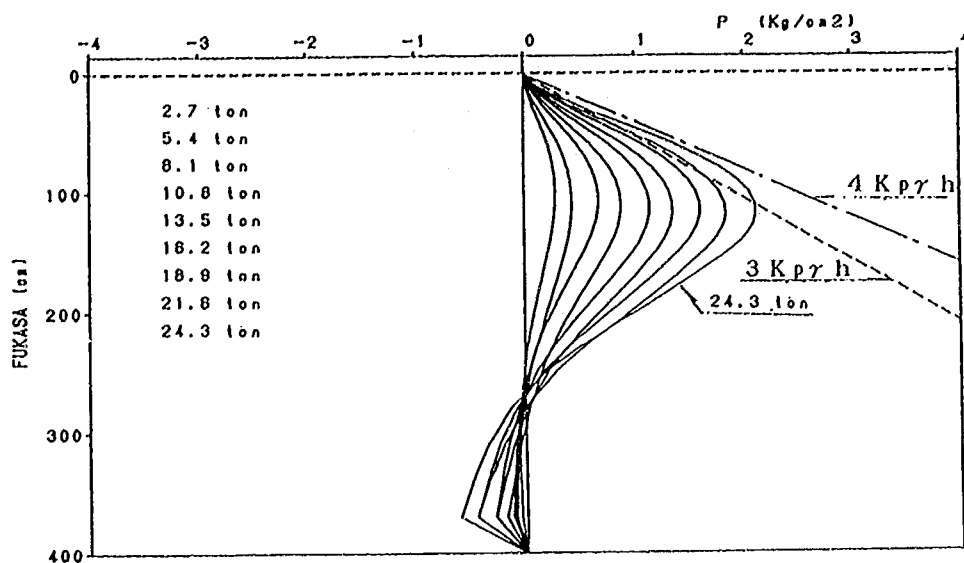
図一 3.4.16 地盤反力度分布 (9本組杭・側方列・前方杭)
