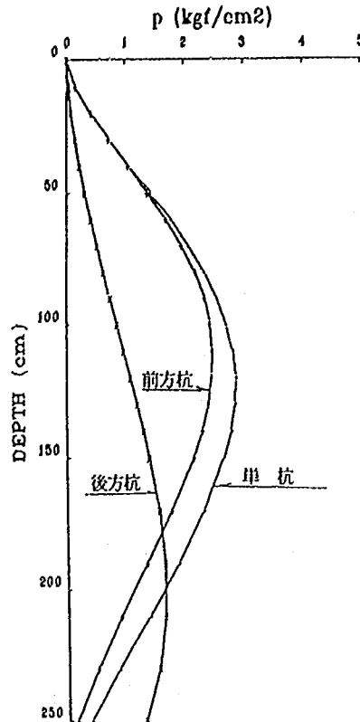
圖—3.4.2 地盤反力度分布比較 (2本直列杭)
