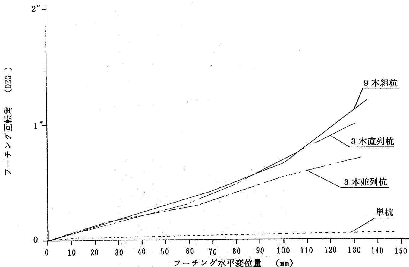
図-3.7.1 変位～フーチング回転角曲線
