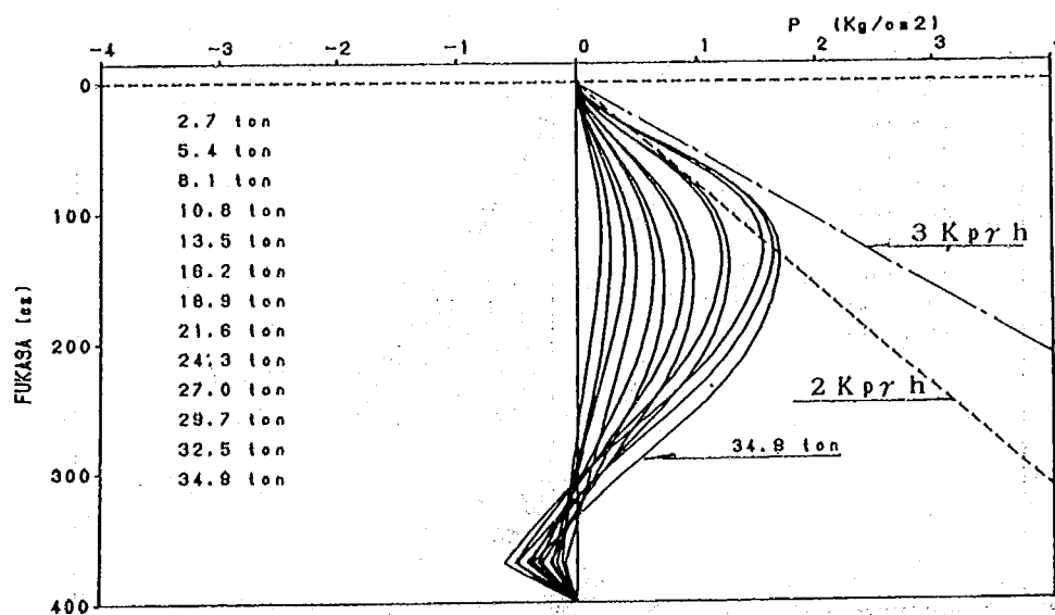
図一 3.4.18 地盤反力度分布 (9本組杭・側方列・後方杭)
