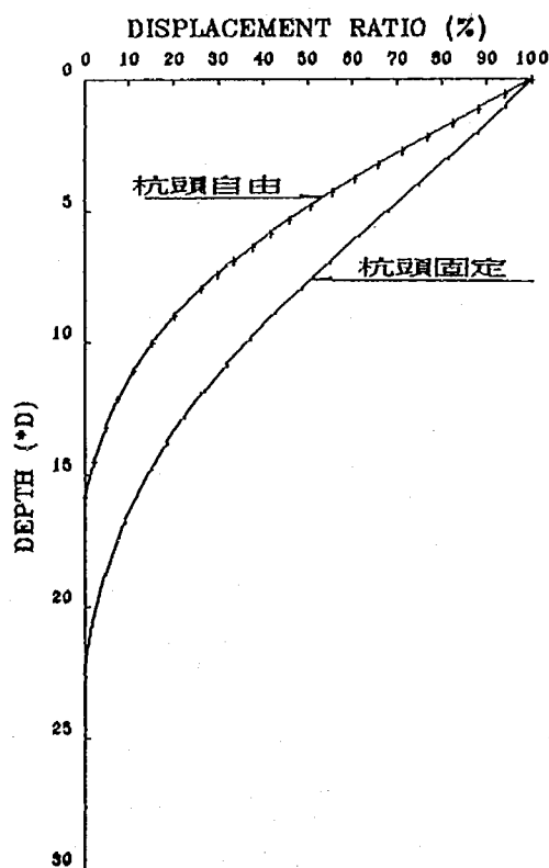
図-4.3.1 変形形状比較図
