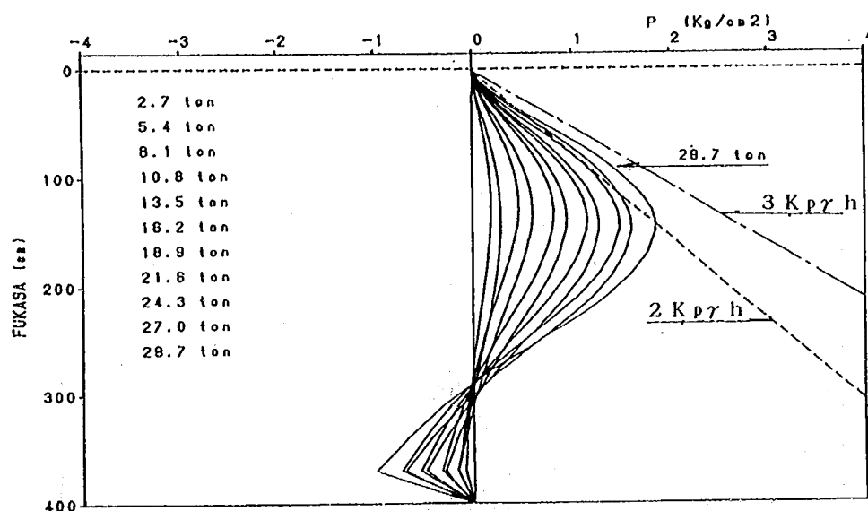
図一 3.4.17 地盤反力度分布 (9本組杭・側方列・中央杭)
