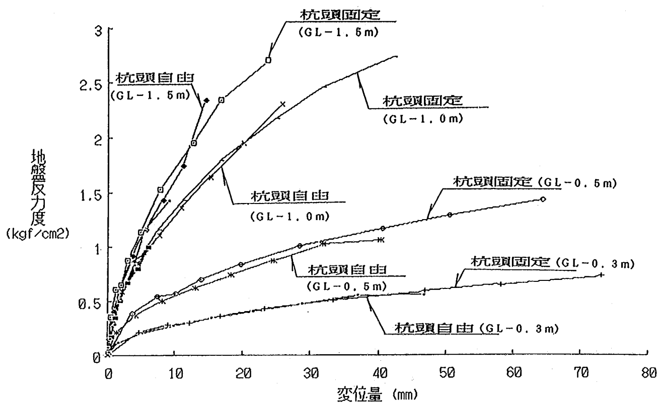
図一 4.3.3 水平地盤反力度～水平変位量曲線比較
