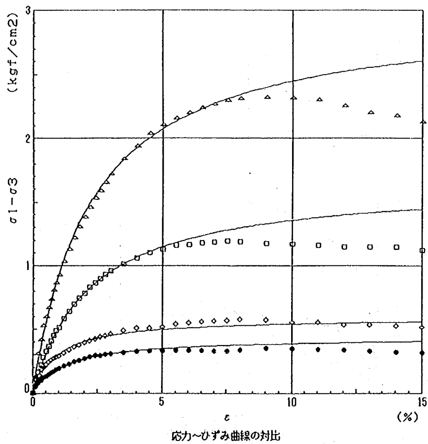
図一参一2.7 三軸圧縮試験の双曲線近似 (CASE 3 1.0 m)
