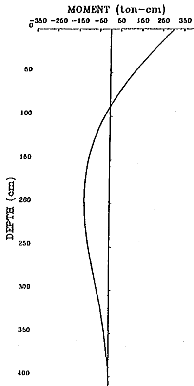
図-3.2.2 曲げモーメント分布図 (2本並列杭)
