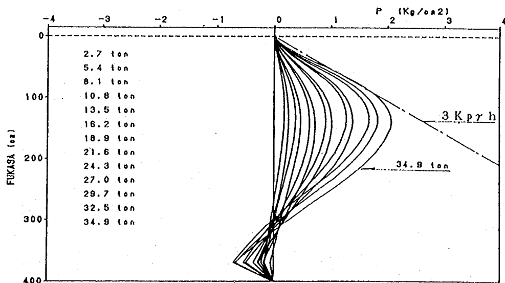
图—3.4.21 地盤反力度分布 (9本組杭・中央列・後方杭)
