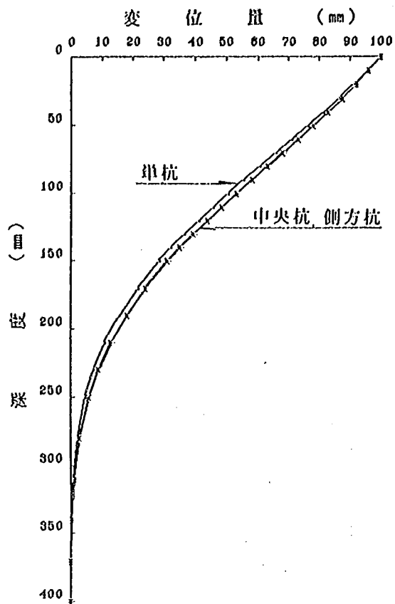
図一 3.3.2 杭体変位の比較 (3本並列杭) 【地表面変位量 100mm時】
