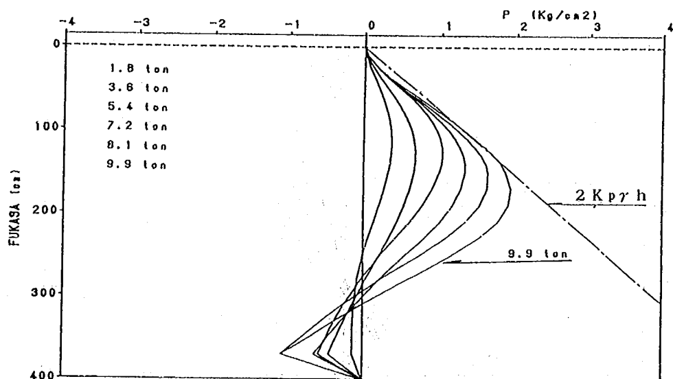
図一 3.4.14 地盤反力度分布 (3本直列・中央杭)
