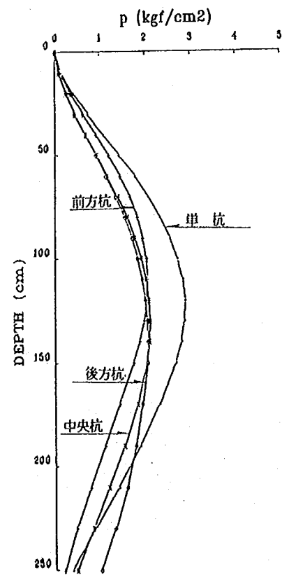
圖—3.4.6 地盤反力度分布比較 (9本組杭・中央列)
