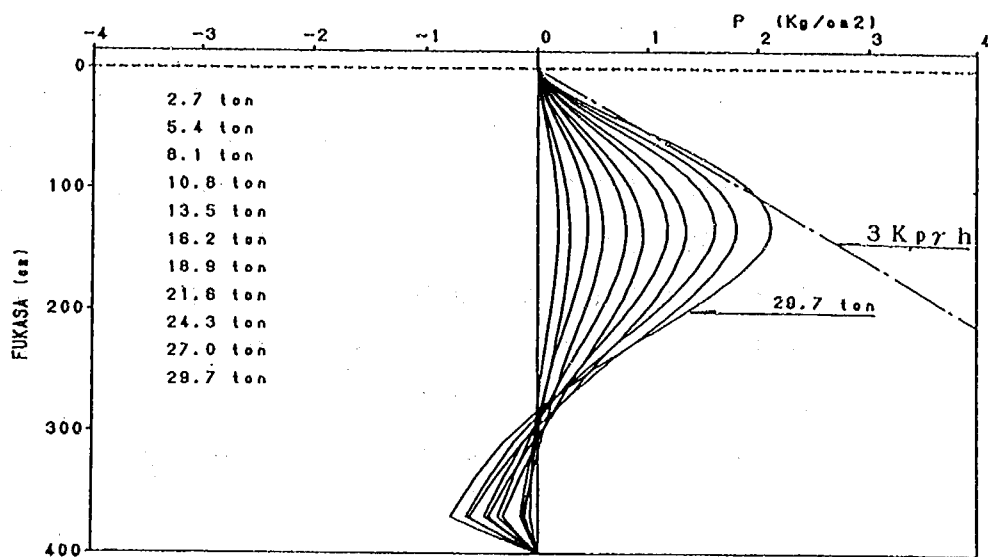
图—3.4.20 地盤反力度分布 (9本組杭・中央列・中央杭)
