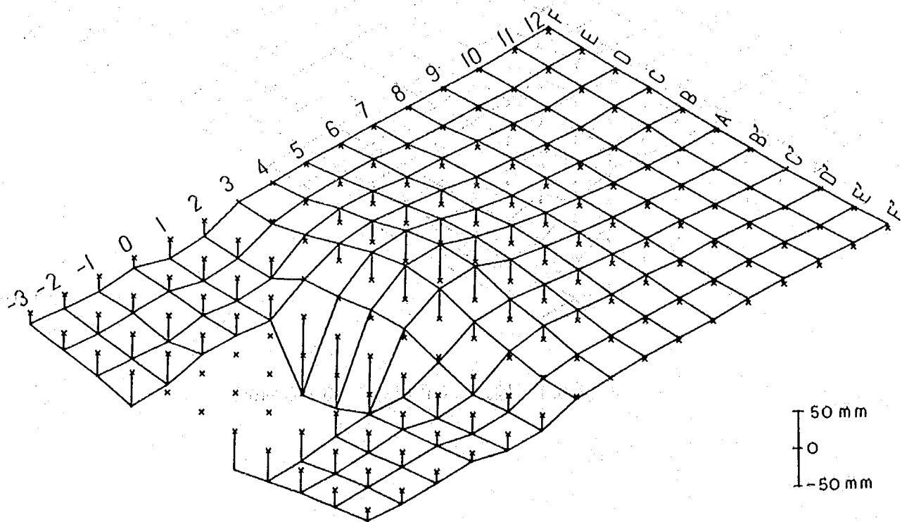
圖—3.6.3 地表面變位觀察圖（9本杭）
