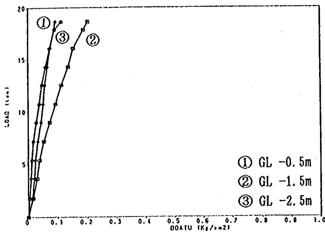
図-3.5.1 荷重-側圧曲線 (3本並列杭・載荷方向壁)
