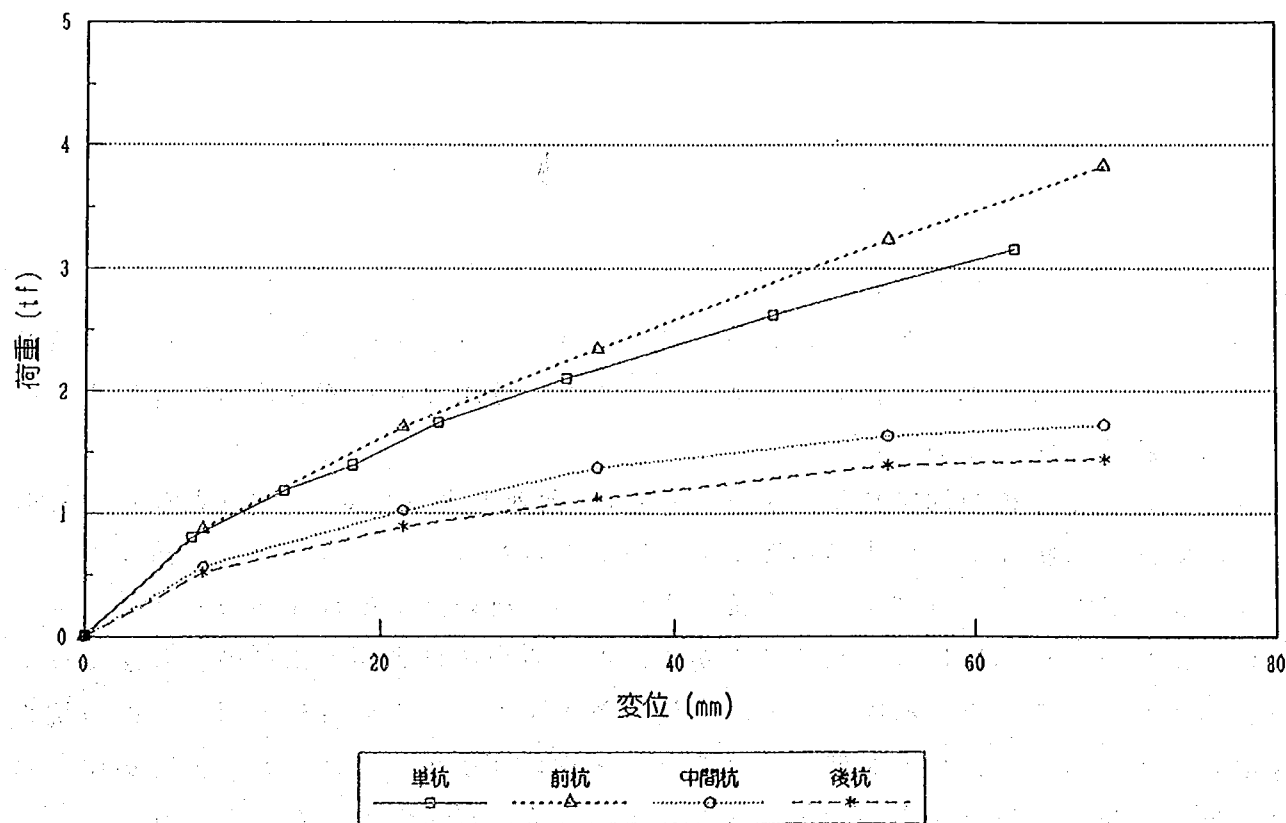
图— 3. 1.11 杭頭荷重—変位量曲線 (3 本直列杭)
