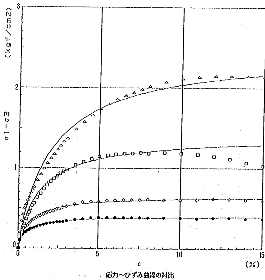
図一参一 2.12 三軸圧縮試験の双曲線近似 (CASE 6 0.5 m)
