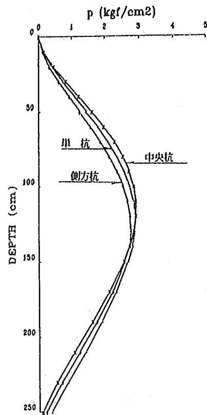
圖—3.4.3 地盤反力度分布比較 (3本並列杭)
