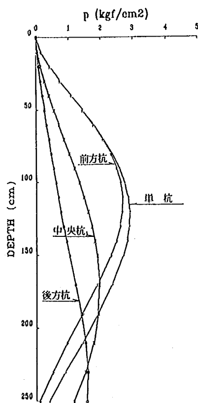
圖—3.4.4 地盤反力度分布比較 (3本直列杭)
