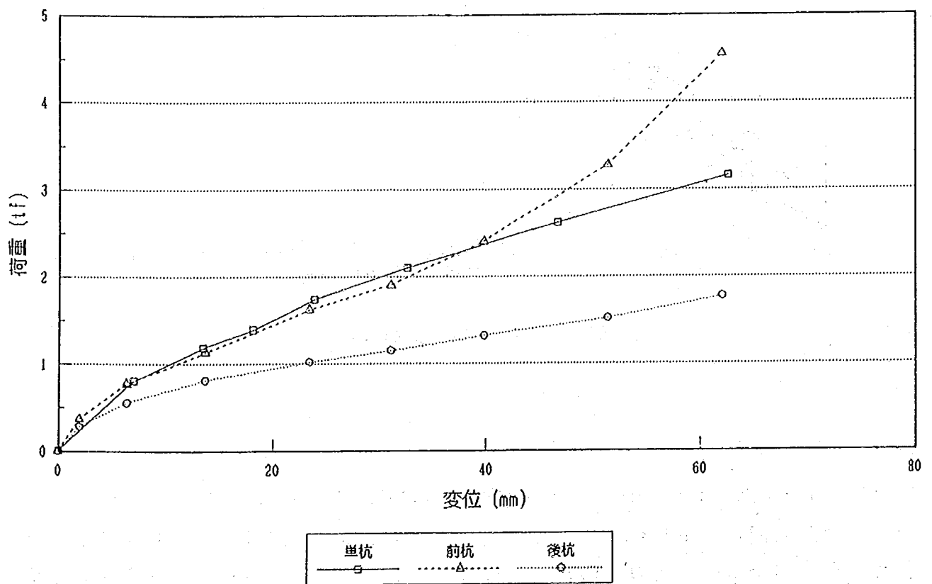
图—3.1.9 杭頭荷重—變位量曲線（2本直列杭）
