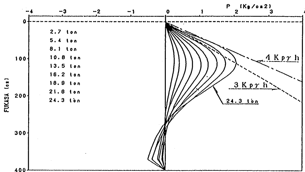
图—3.4.19 地盤反力度分布 (9本組杭・中央列・前方杭)
