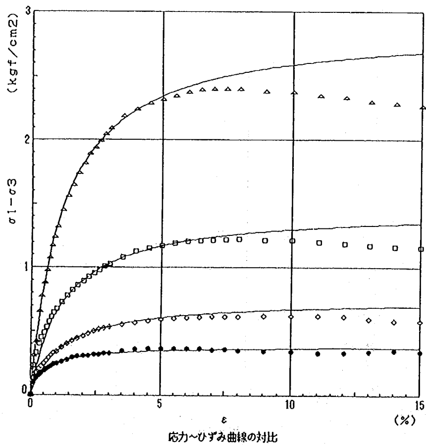
図一参一2.3 三軸圧縮試験の双曲線近似 (CASE1 1.0 m)
