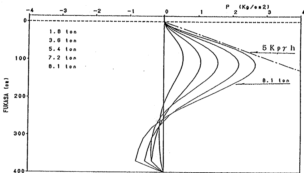
図一 3.4.13 地盤反力度分布 (3本直列・前方杭)
