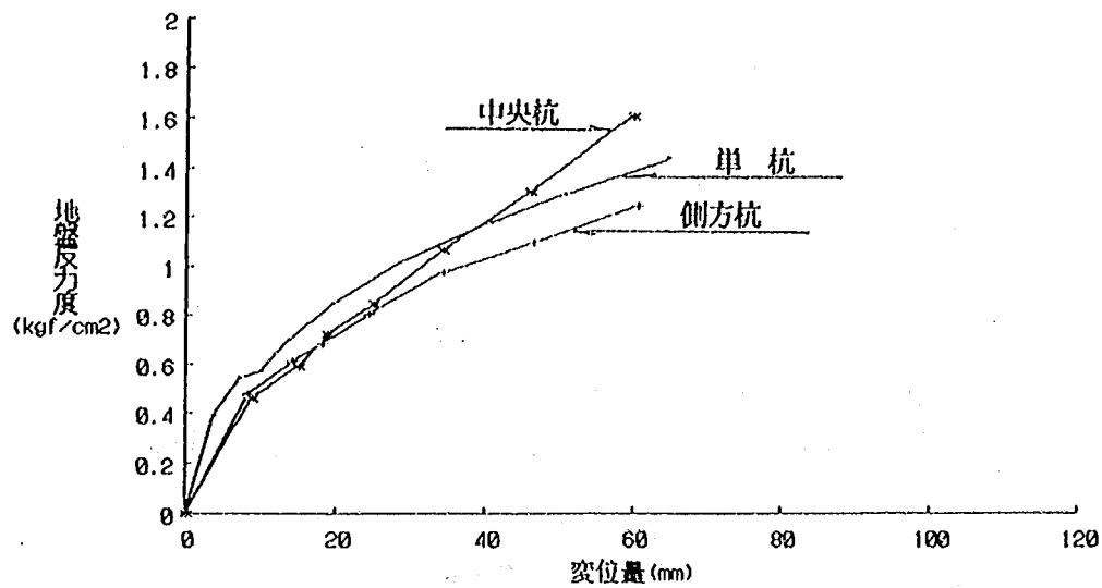
図-3.4.22 地盤のP～y曲線比較 (3本並列杭) 【深度GL-0.5 m】
