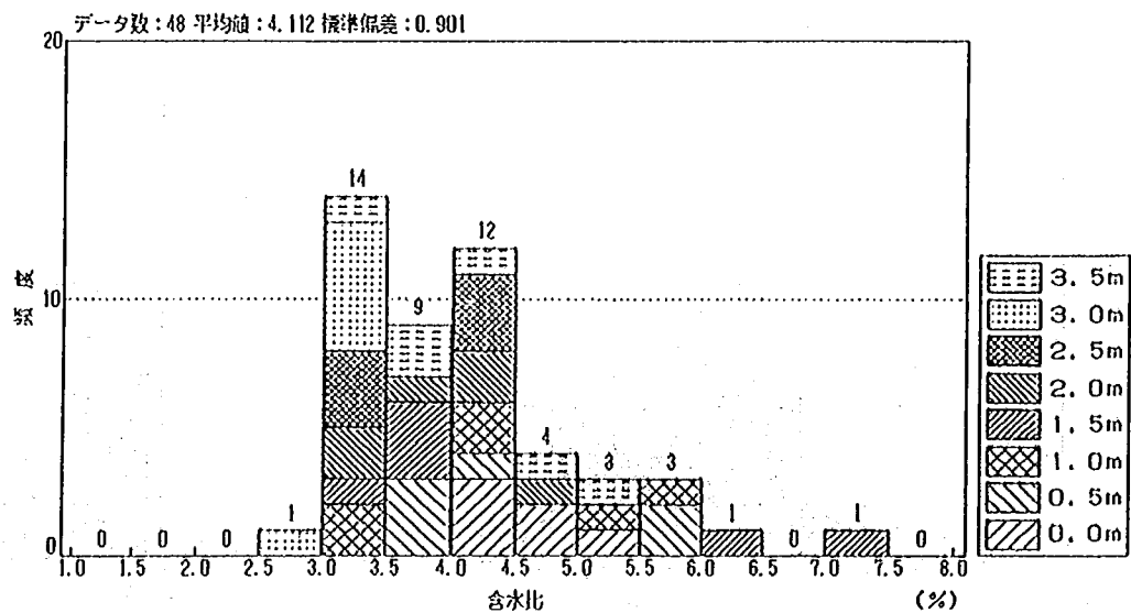
図一参-2.24 三軸圧縮試験 \sigma_t , \rho_d W の頻度分布図 (CASE5)
