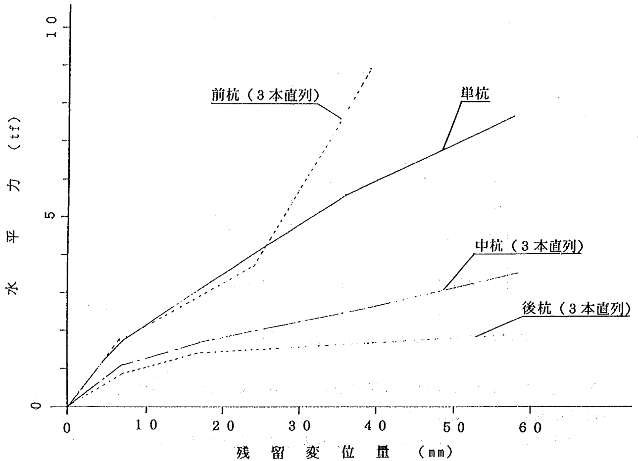
図-4.5.1 荷重～変位量曲線
