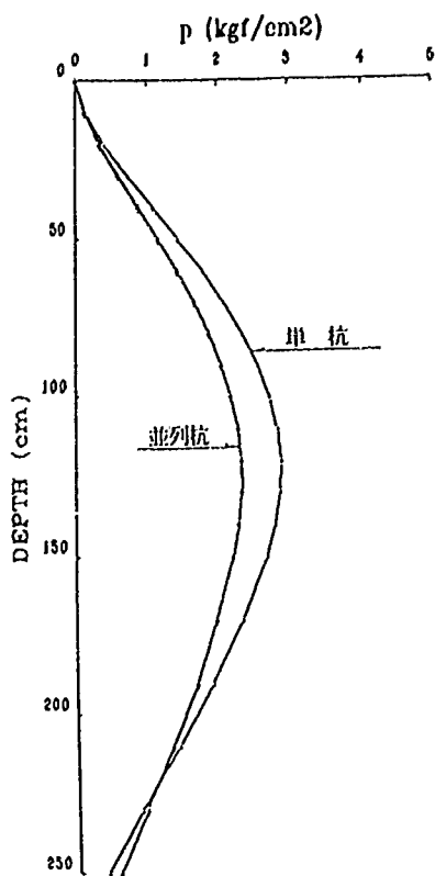
圖—3.4.1 地盤反力度分布比較 (2本並列杭)
