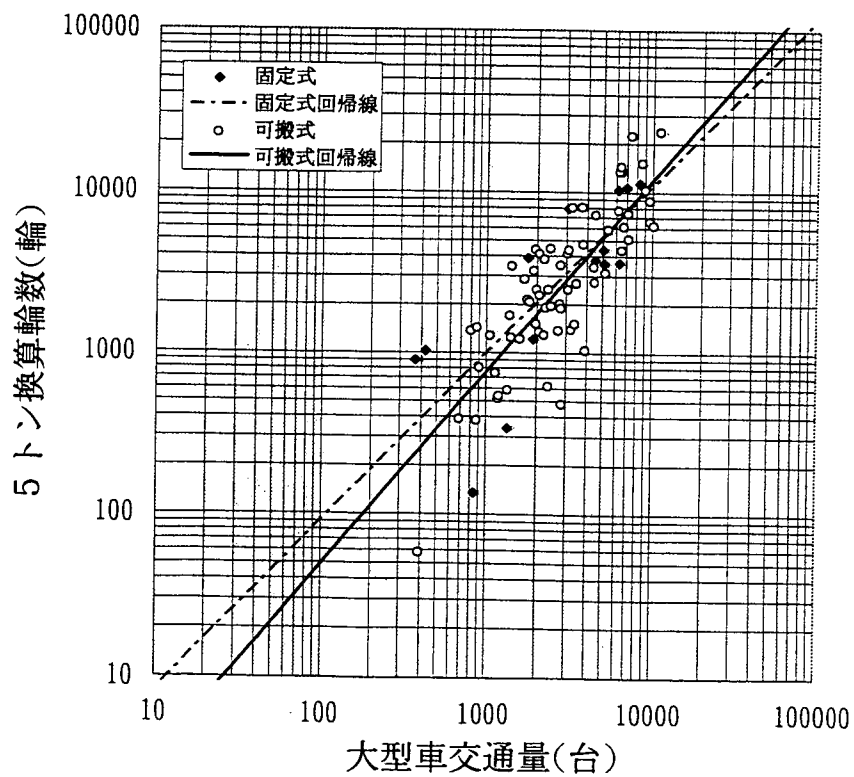
図-16 大型車交通量と5トン換算輪数(平成4年度)
