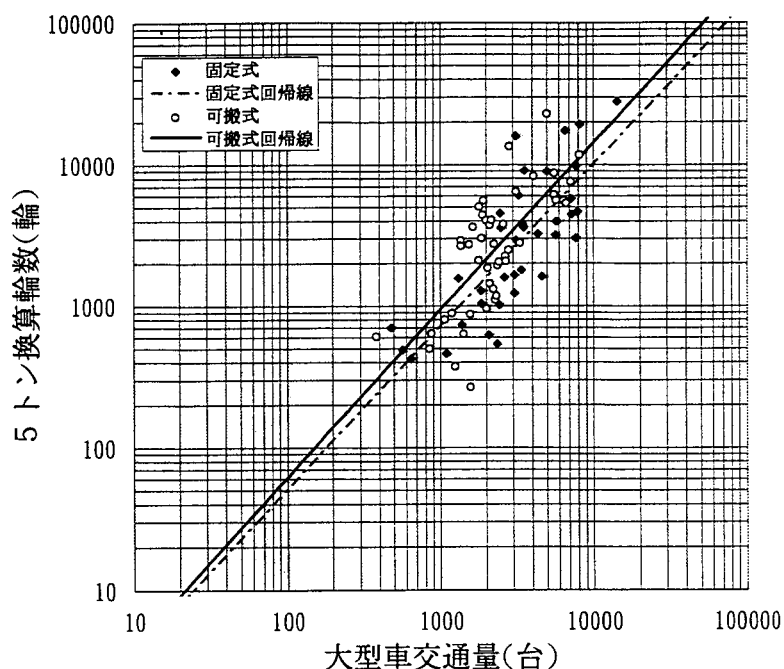
図-13 大型車交通量と5トン換算輪数(平成元年度)
