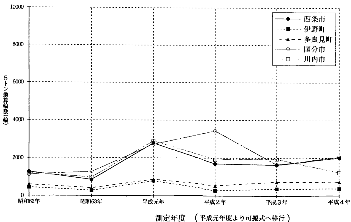
図 - 12 固定式から可搬式に移行した箇所における5トン換算輪数の推移（その2）
