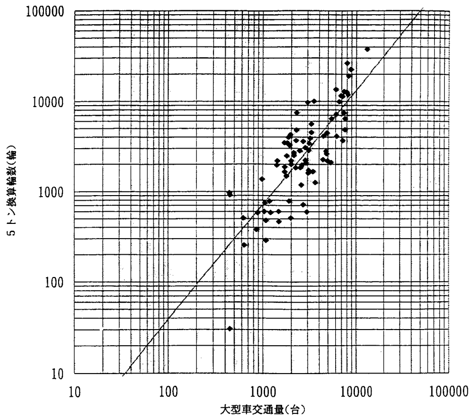
図-7 大型車交通量と5トン換算輪数(平成3年度)
