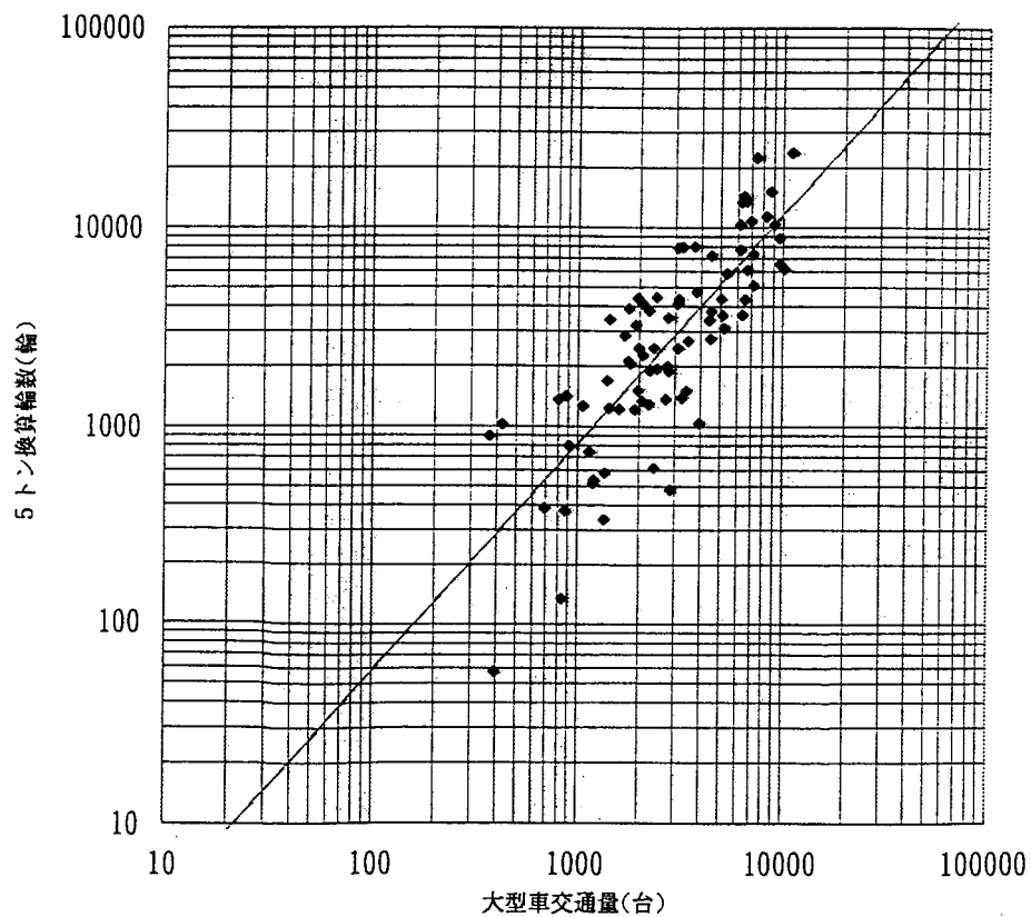
図-8 大型車交通量と5トン換算輪数(平成4年度)
