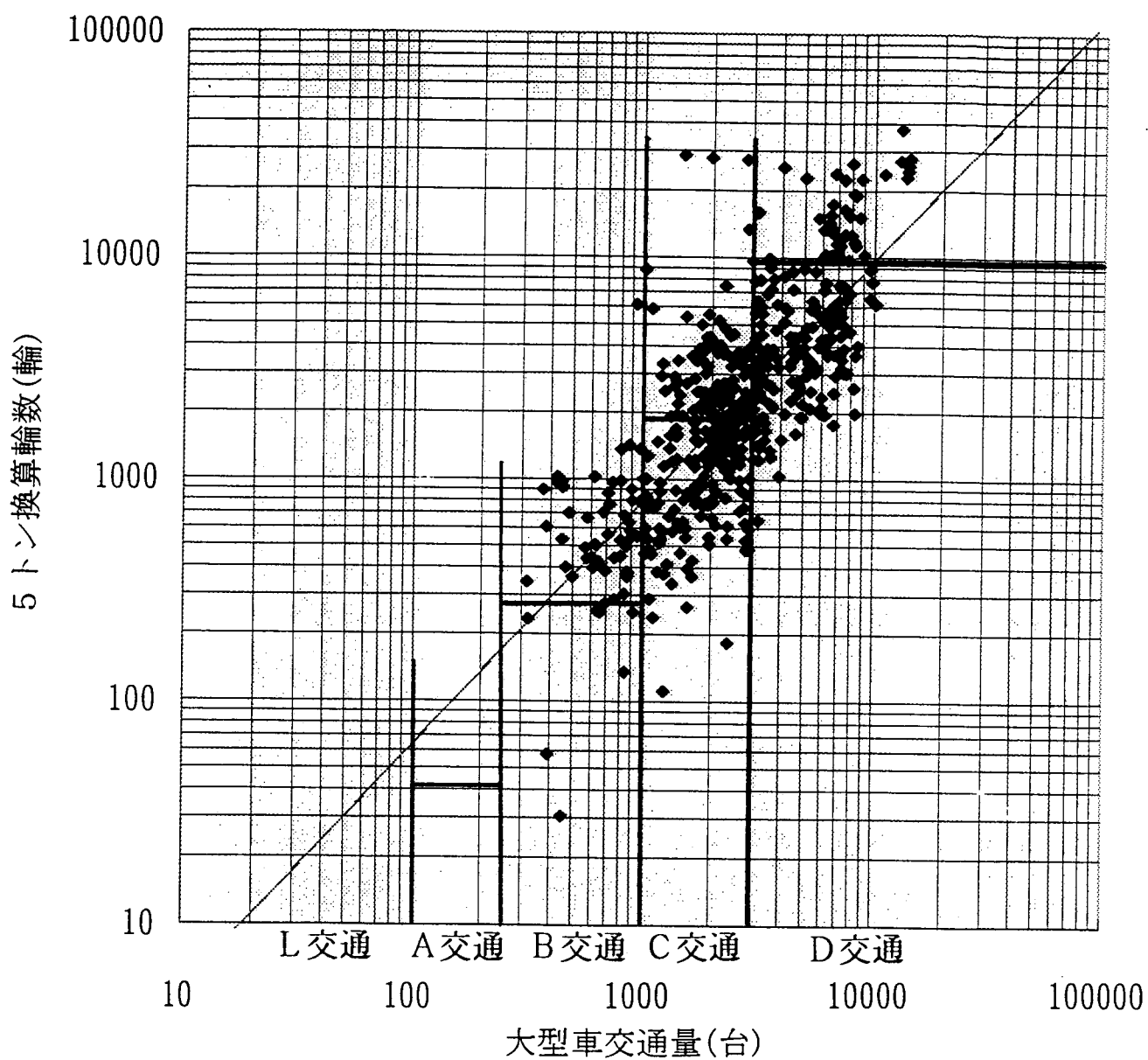
図-17 大型車交通量と5トン換算輪数(昭和62年～平成4年)
