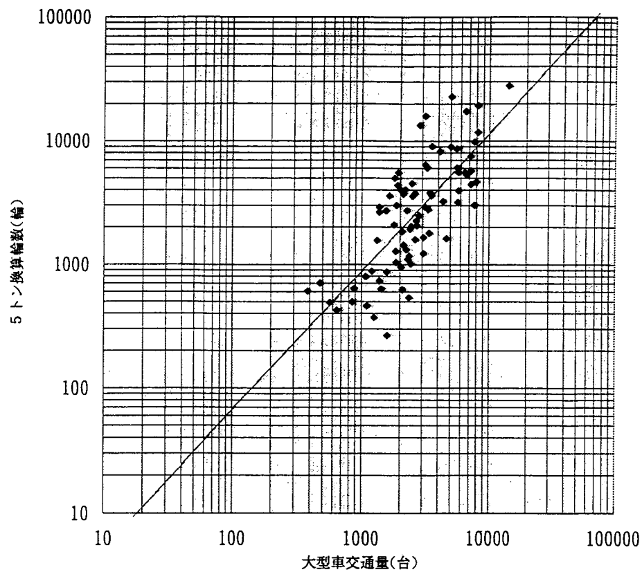
図-5 大型車交通量と5トン換算輪数(平成元年度)
