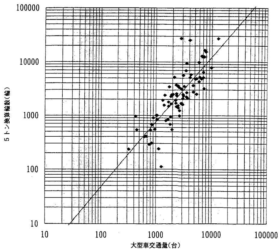
図-6 大型車交通量と5トン換算輪数(平成2年度)
