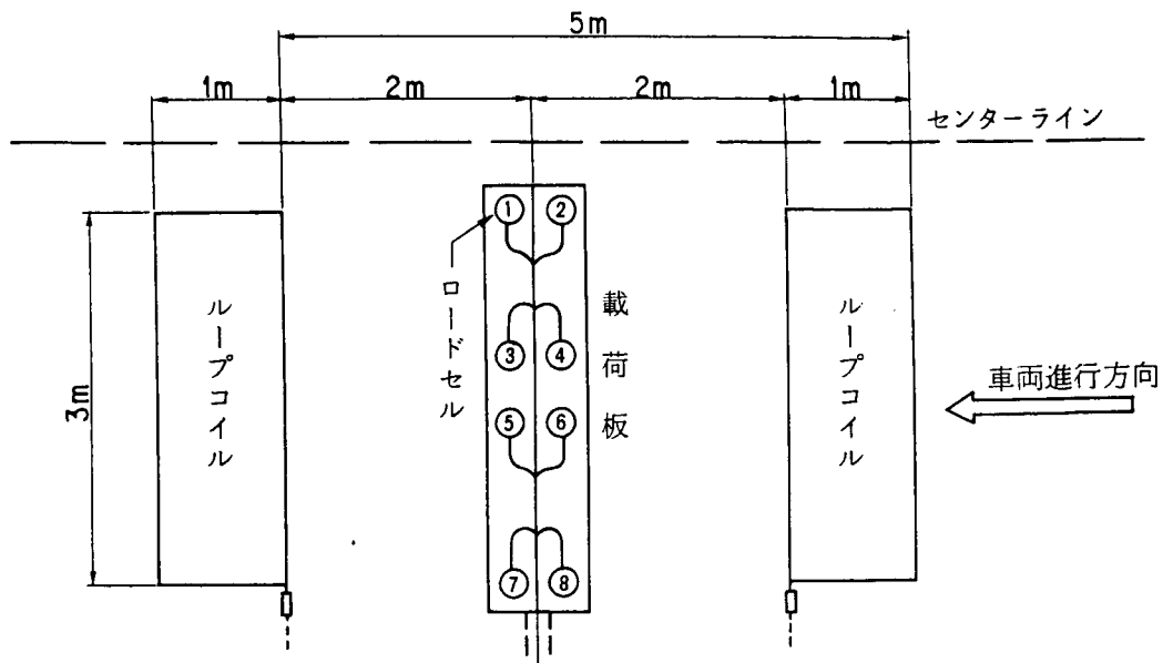
図-1 固定式測定機の構成
