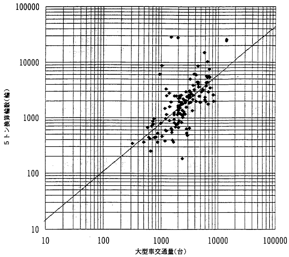
図-3 大型車交通量と5トン換算輪数(昭和62年度)
