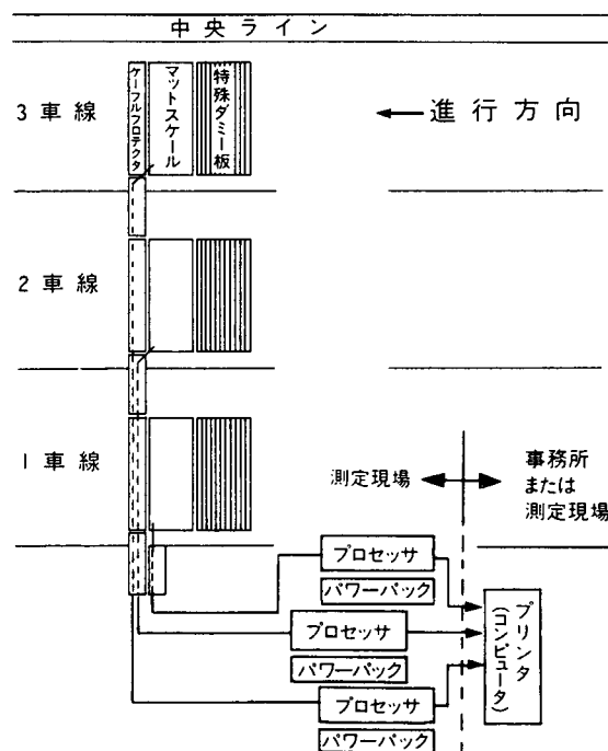
図-2 可搬式測定機の構成
