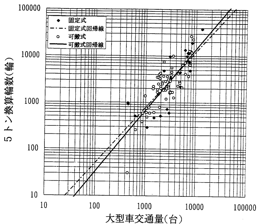
図-15 大型車交通量と5トン換算輪数(平成3年度)
