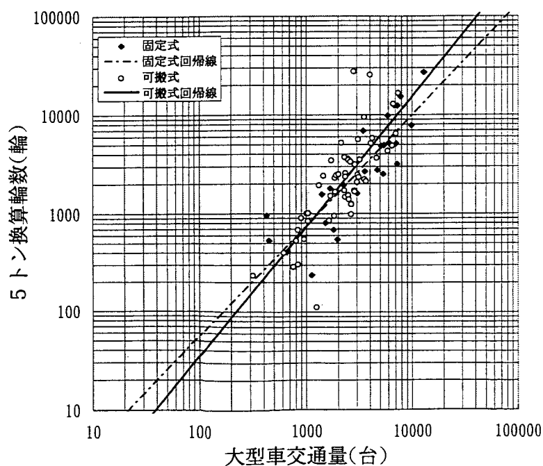
図-14 大型車交通量と5トン換算輪数(平成2年度)
