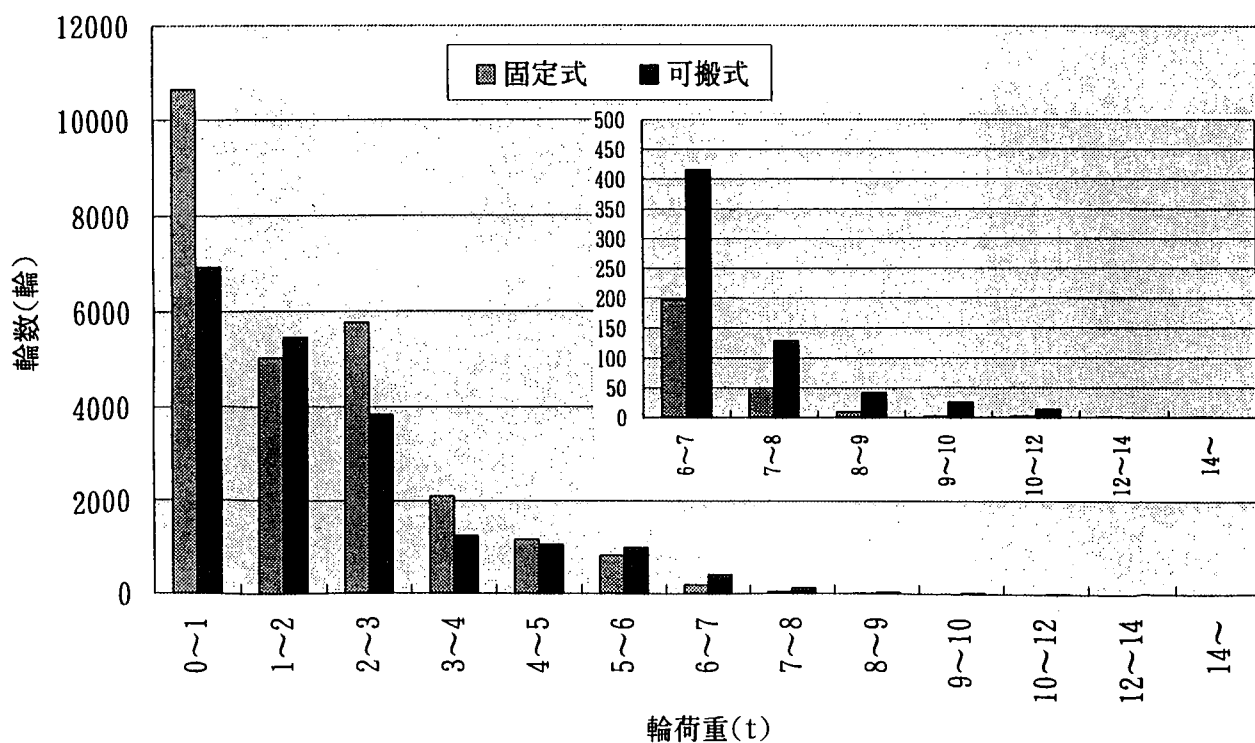
図-10 固定式、可搬式同時測定箇所における輪荷重分布の比較（東広島市）
