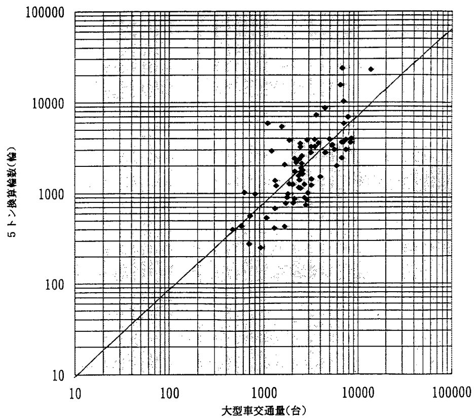
図-4 大型車交通量と5トン換算輪数(昭和63年度)
