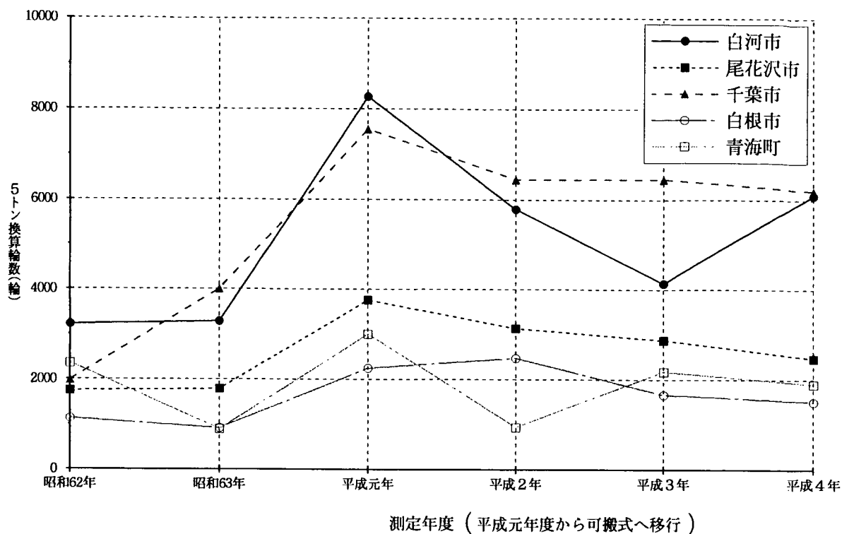
図 - 11 固定式から可搬式に移行した箇所における5トン換算輪数の推移（その1）
