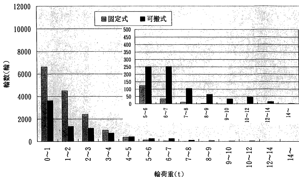
図-9 固定式、可搬式同時測定箇所における輪荷重分布の比較（北海道幕別町）
