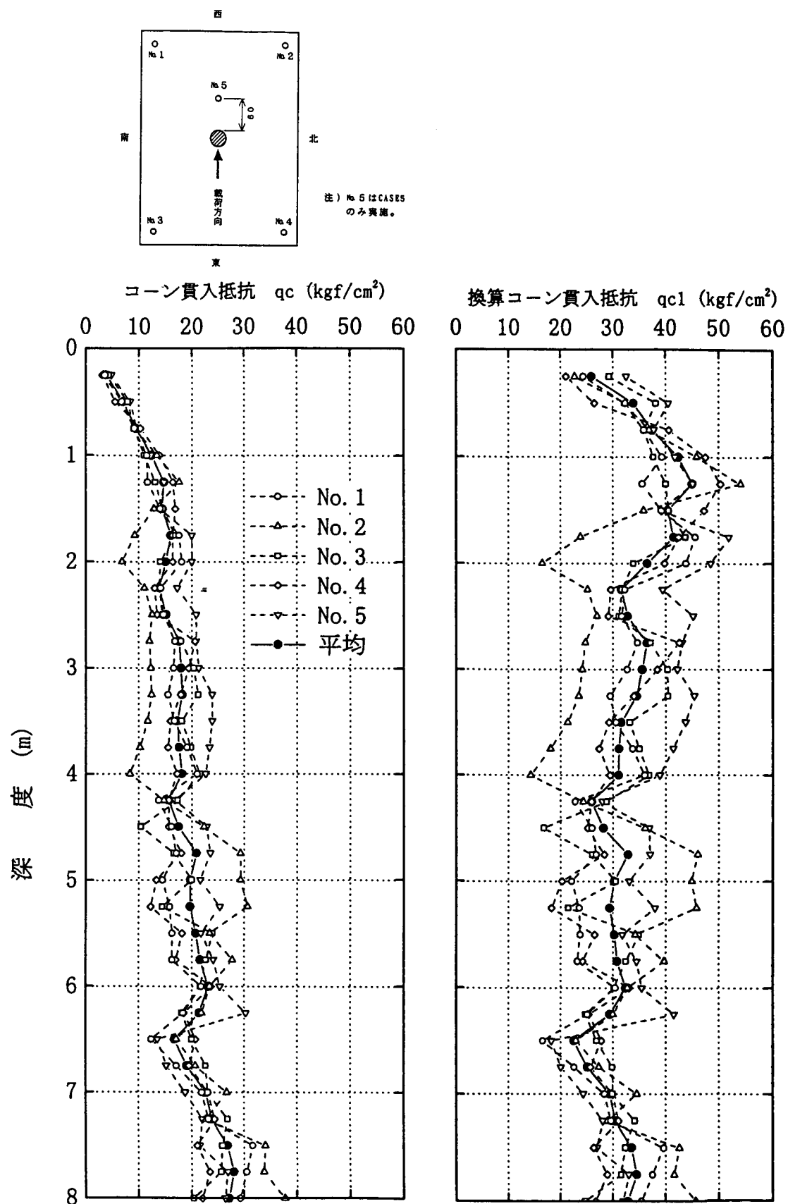
図-参-5 コーン貫入試験結果 (ケース 5)
