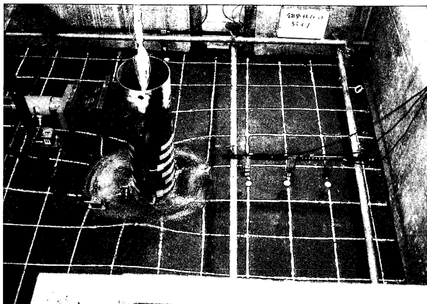
写真-参-7 載荷 (5 δ°: ケース2)
