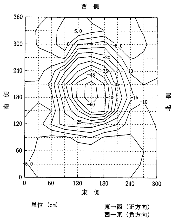
図-参-17 試験終了時の地表面等高線 (ケース 1) 西 側
