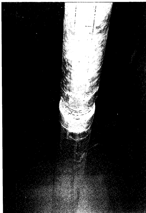
写真-参-17 杭体損傷状況③（ケース4：PHC杭コンクリート除去後）
