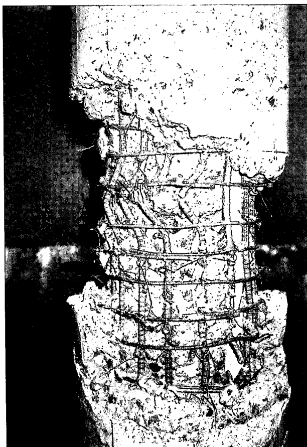
写真-参-18 杭体損傷状況④（ケース5：鉄筋コンクリート杭コンクリート除去後）
