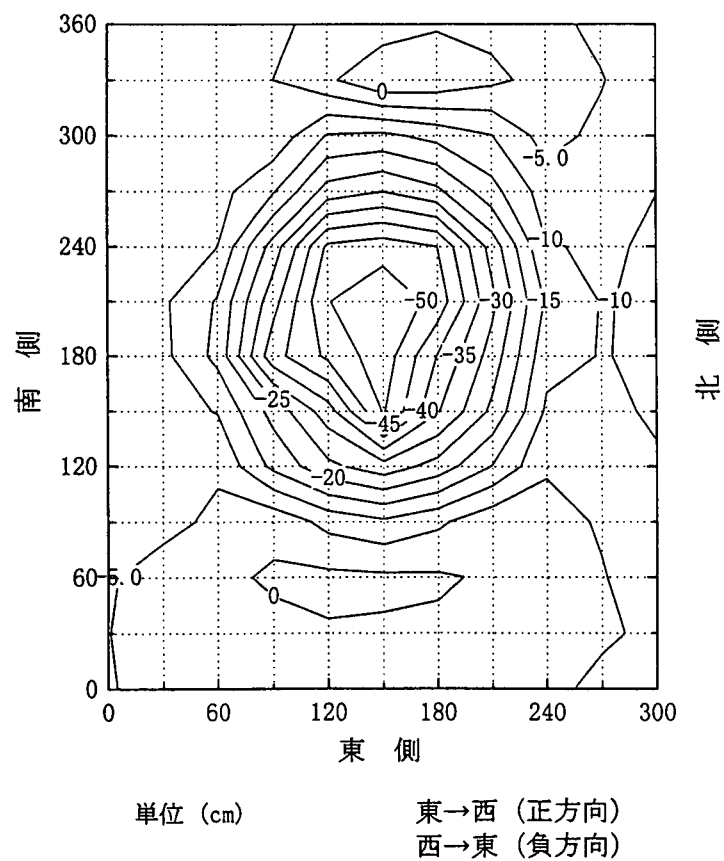
図-参-18 試験終了時の地表面等高線 (ケース 2)
