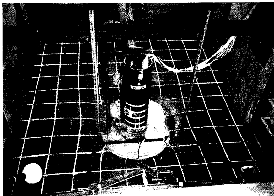
写真-参-4 載荷 (5 δ ° : ケース 1)
