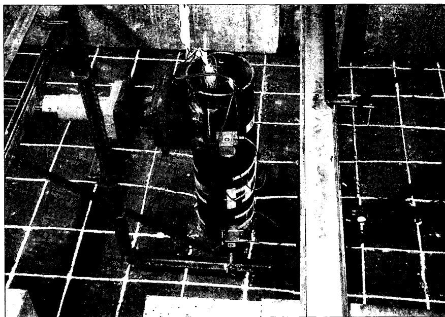
写真-参-3 載荷 (1 δ ° : ケース 1)
