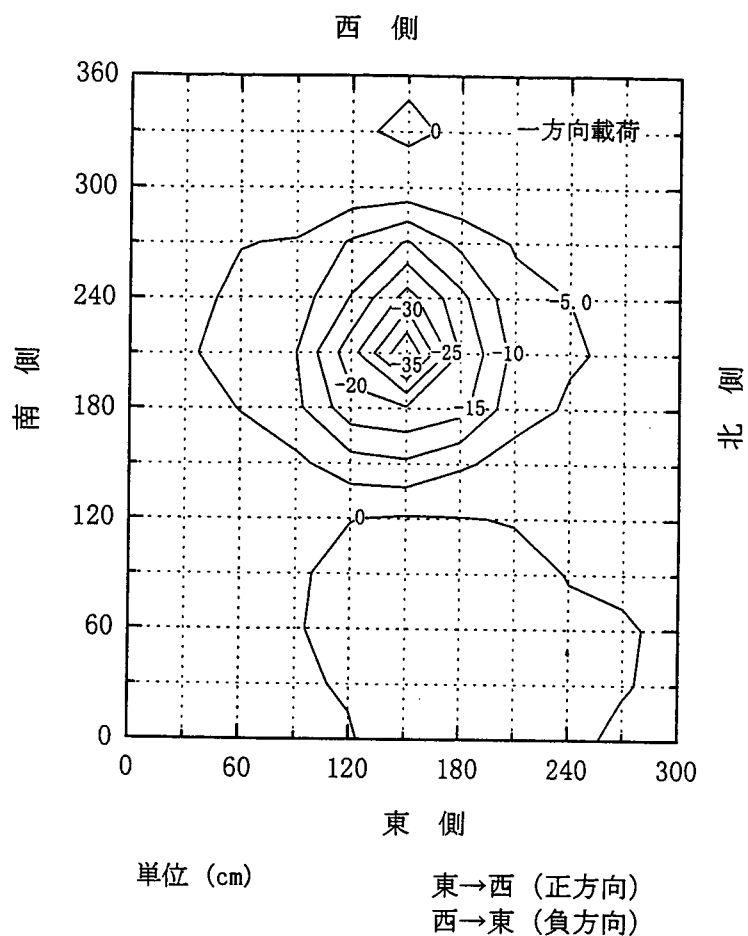
図-参-19 試験終了時の地表面等高線 (ケース 3)
