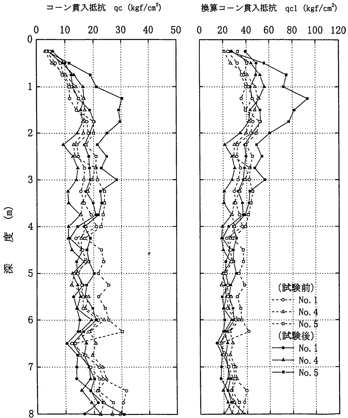
図-4-12 载荷試験前後のコーン貫入試験結果 (ケース 5)
