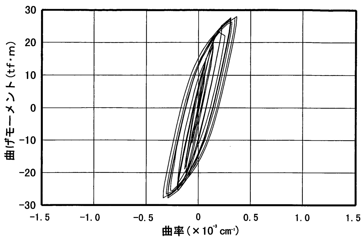
図-3-2 鋼管杭の曲げモーメント～曲率履歴曲線
