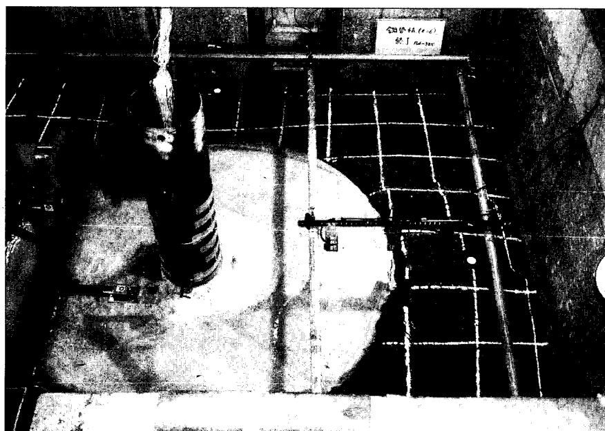
写真-参-8 載荷終了 (16 δ°: ケース2)
