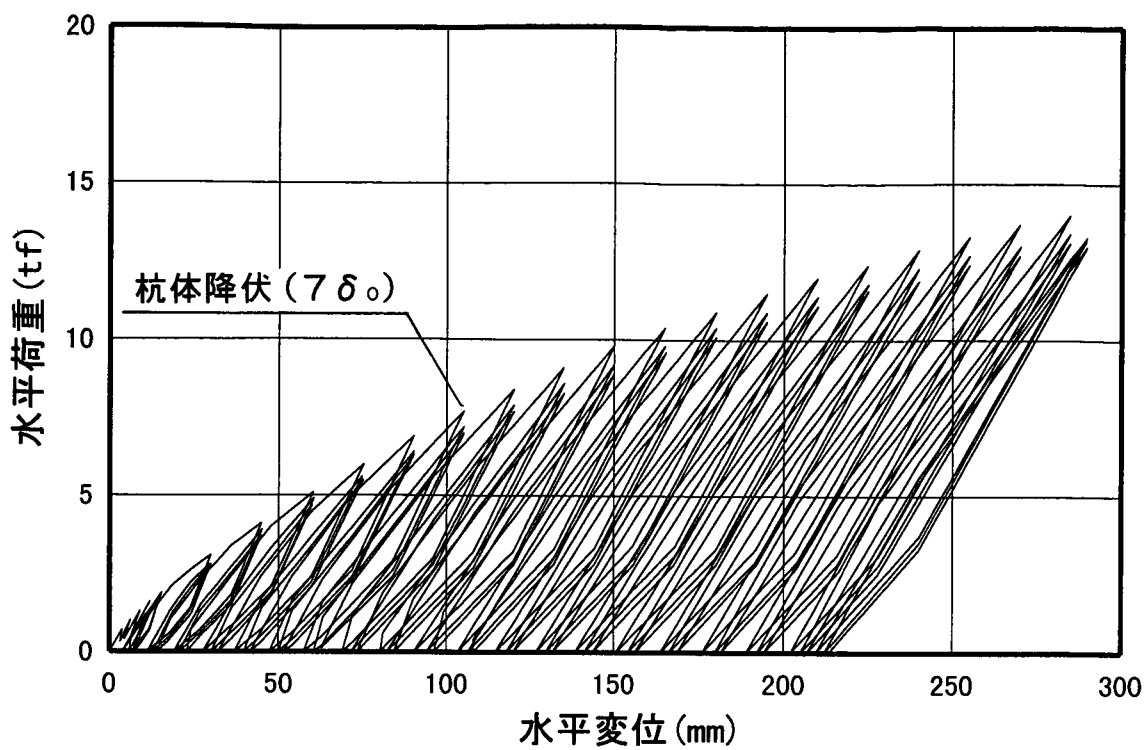
図-4-3 水平荷重～水平変位履歴曲線（ケース 3）
