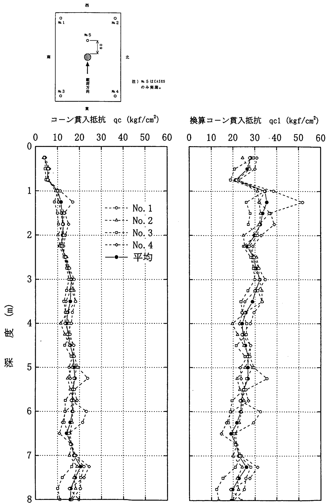
図-参-3 コーン貫入試験結果 (ケース3)
