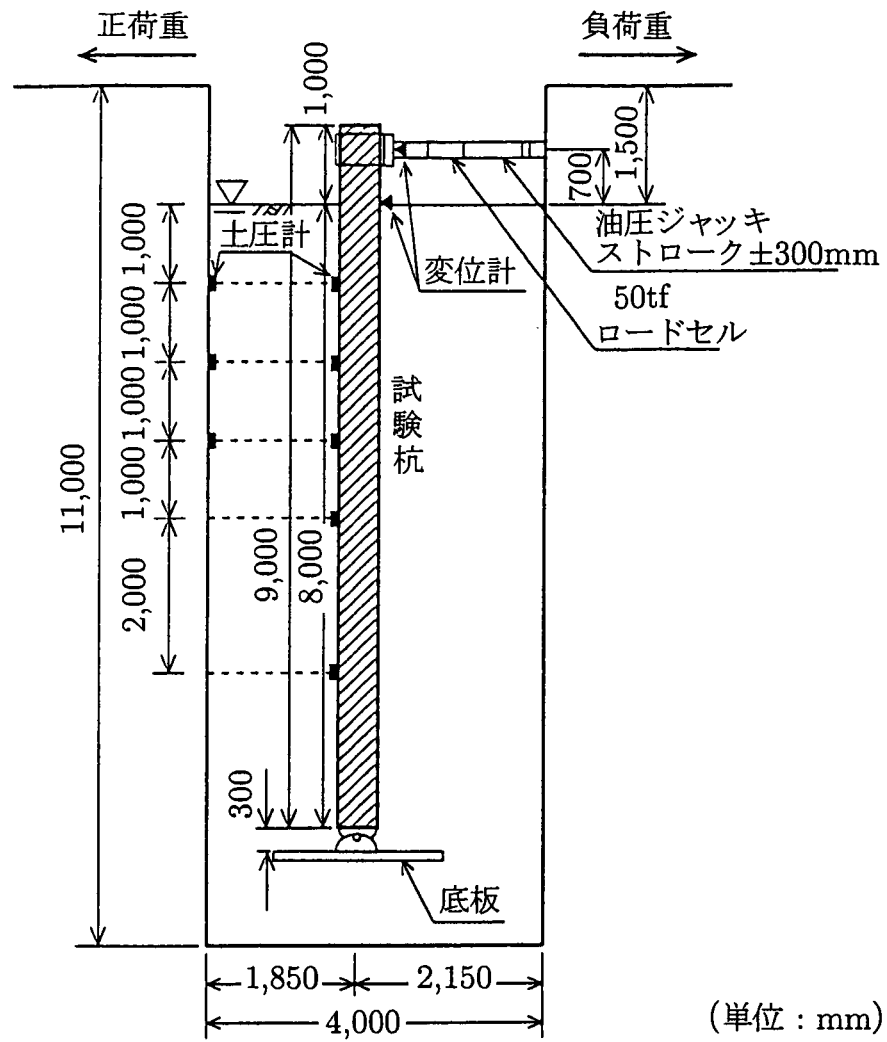
図-2-1 試験概要
