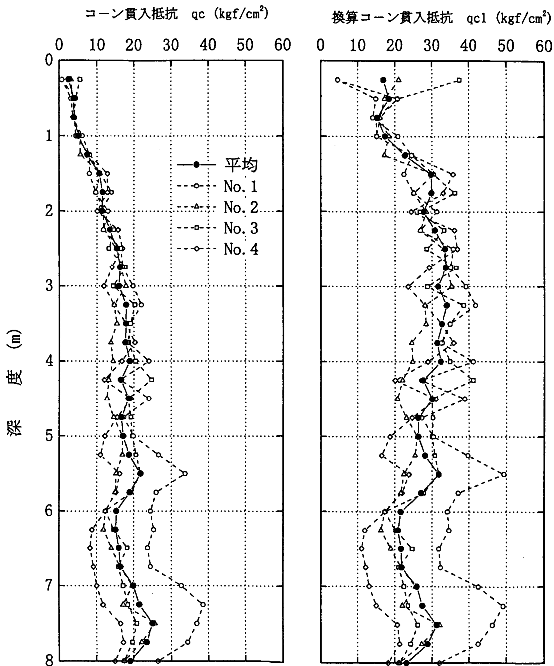
図-参-1 コーン貫入試験結果 (ケース1)
