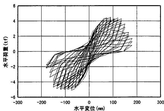
(a) 地盤中の杭の水平載荷試験
