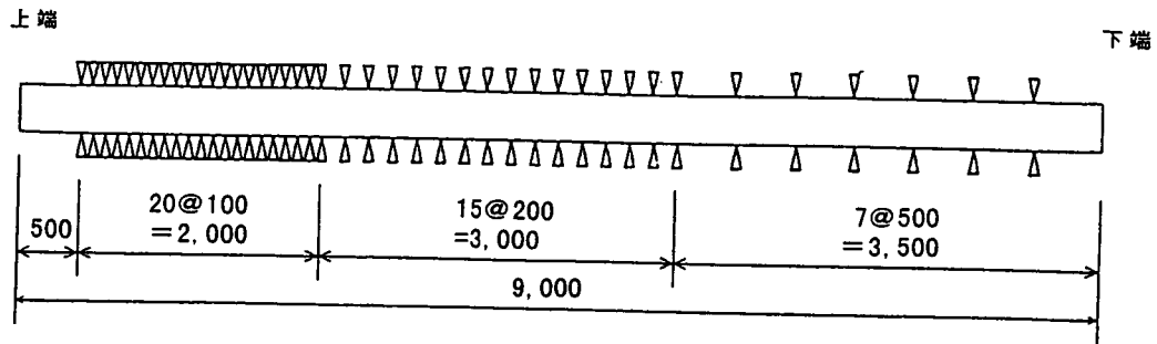
(a) 鋼管杭 (ケース 1 ~ 3)
