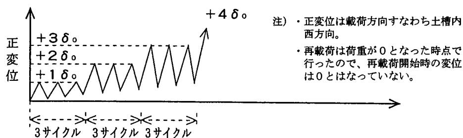
(b) 一方向水平載荷試験（ケース 3）
