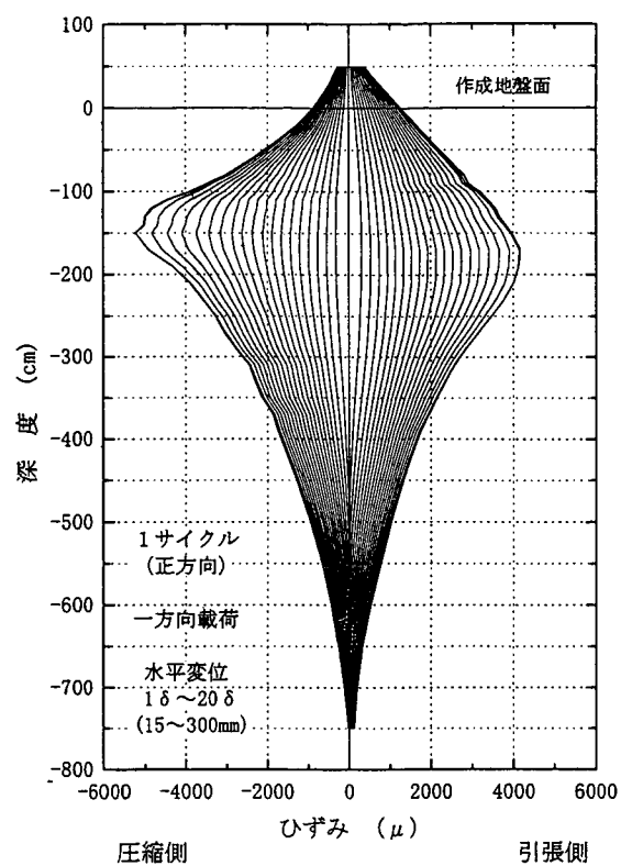
図-4-10 曲げひずみの深度方向分布 (ケース 3)
