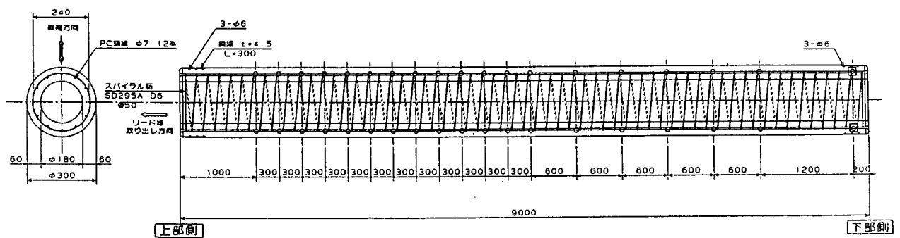
(b) PHC 杭 (ケース 4)
