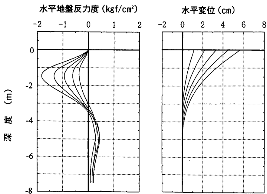
(c) 水平地盤反力度
