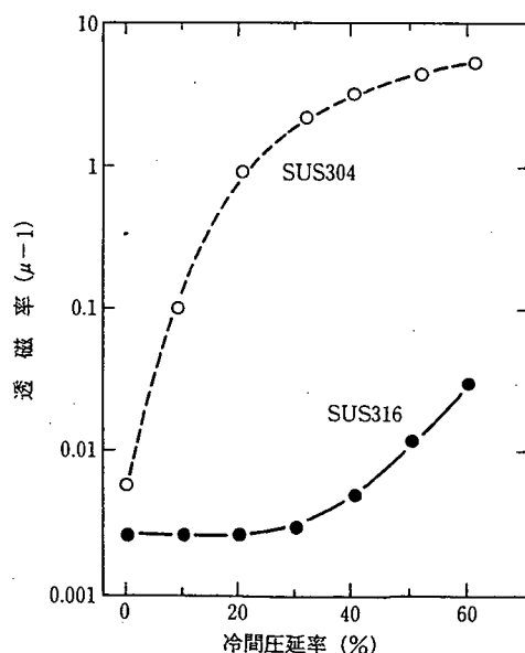
図解-2.6 透磁率に及ぼす冷間圧延率の影響 (ステンレス鋼便覧第3版)
