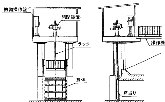
図解-5.4 ラック式開閉装置の例
