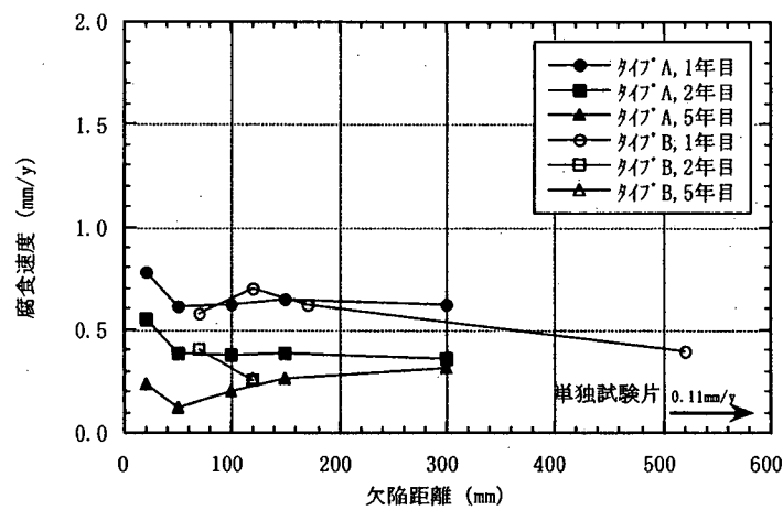
図解-3.1 塗装端からの欠陥距離とその位置での腐食速度
