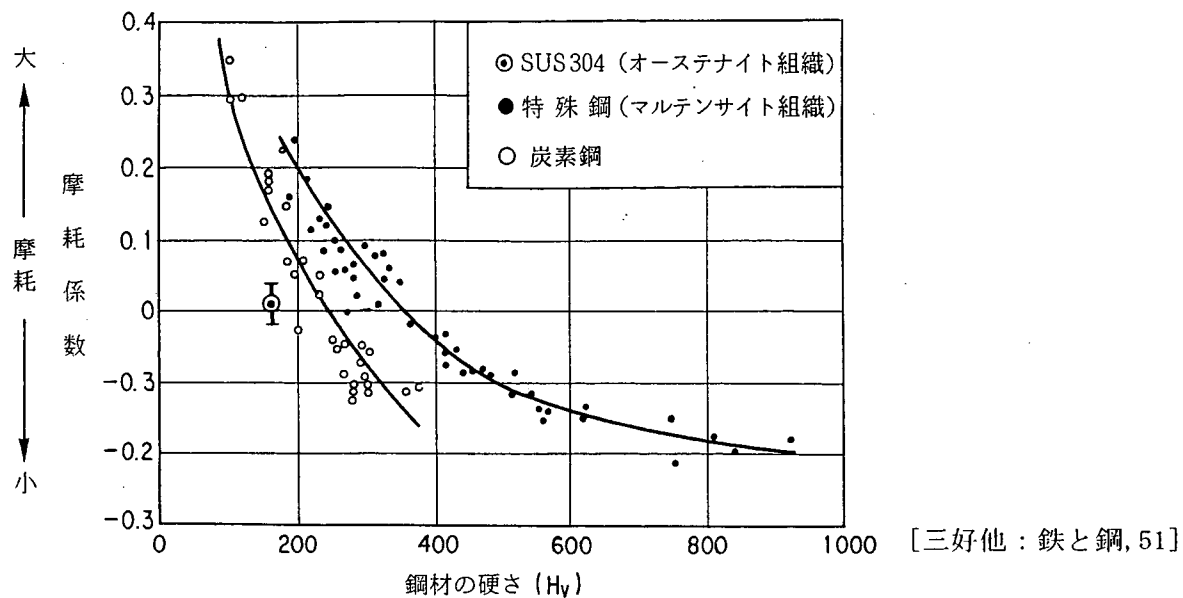
図解-2.9 鋼材の硬さと摩擦係数
