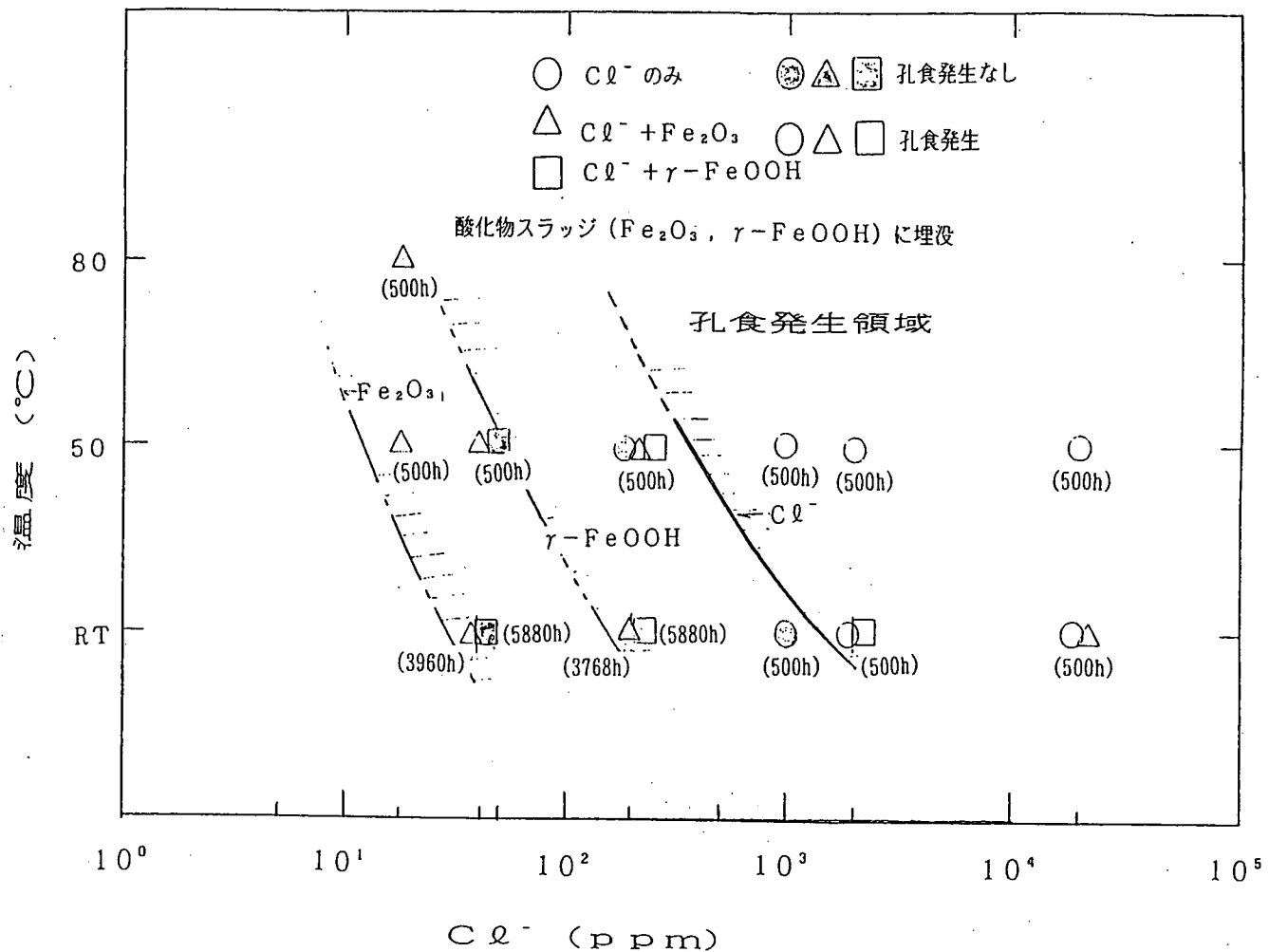
図解-2.28 SUS304の孔食感受性に及ぼすもらい錆の影響
