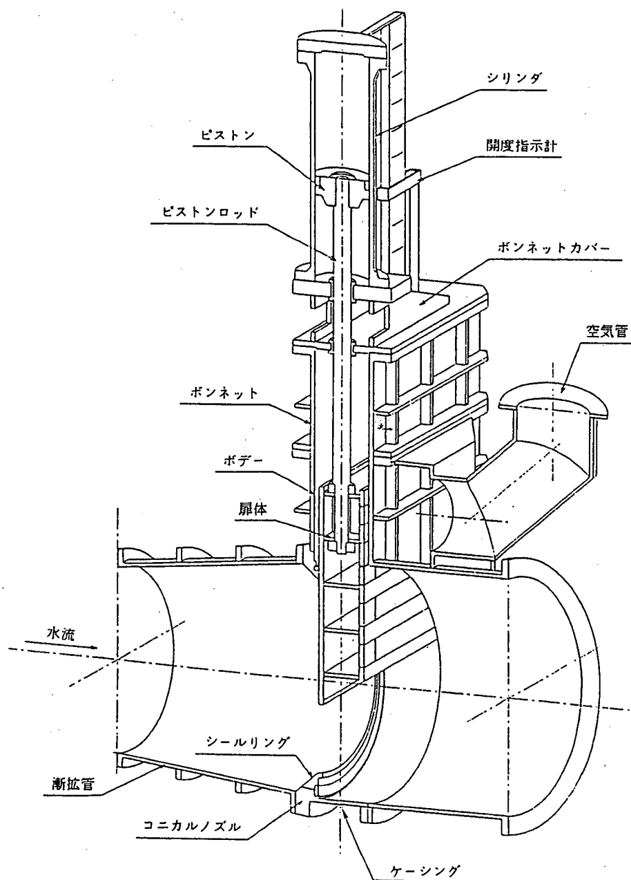
図解-3.13 バルブ（ジェットフローゲートの場合）
