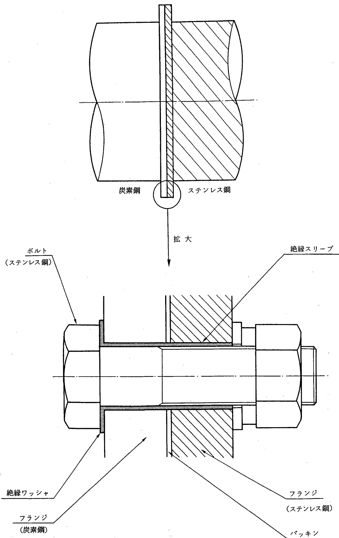
図解-3.3 フランジ接合部の絶縁
