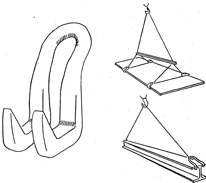
図解-4.15 ハッカーの例
