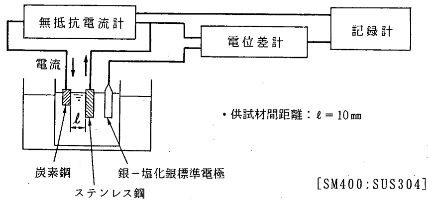
図解-2.21 カップル電流試験の試験方法
