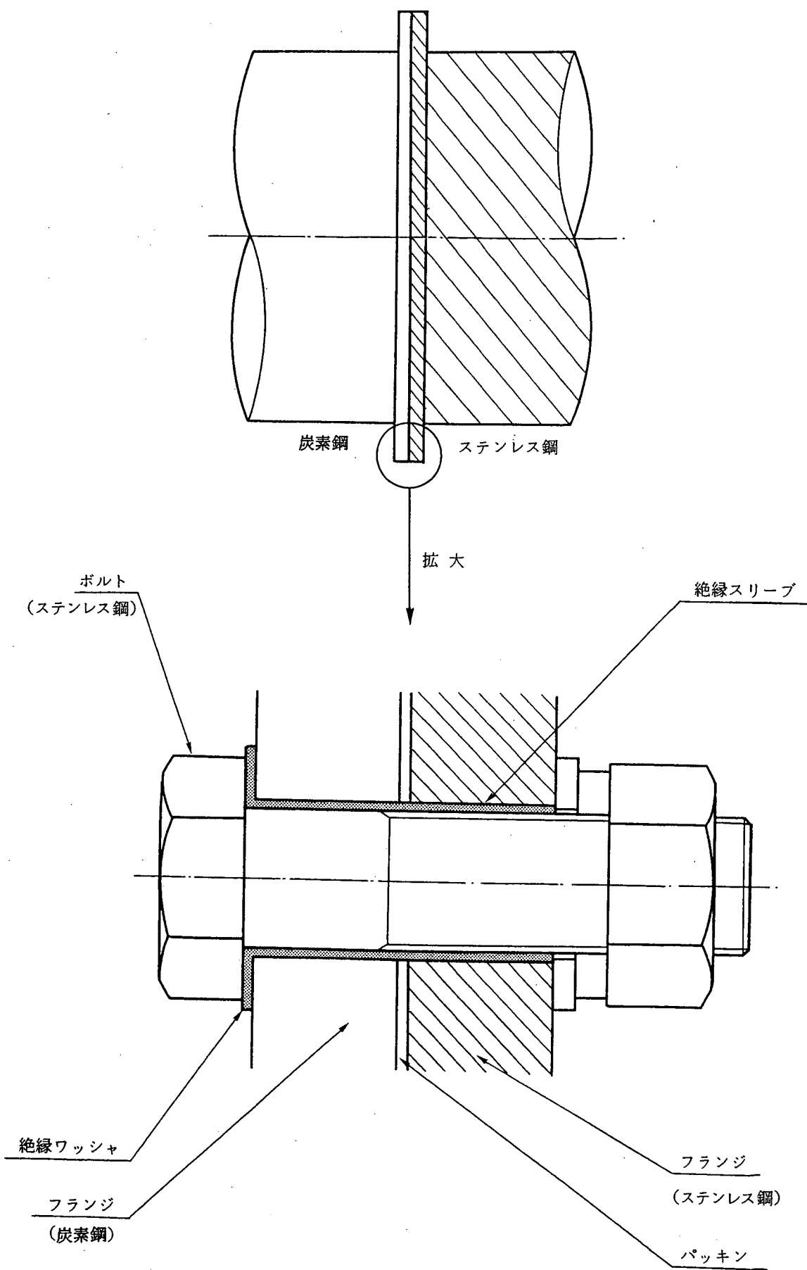
図解-5.11 フランジ接合部の絶縁
