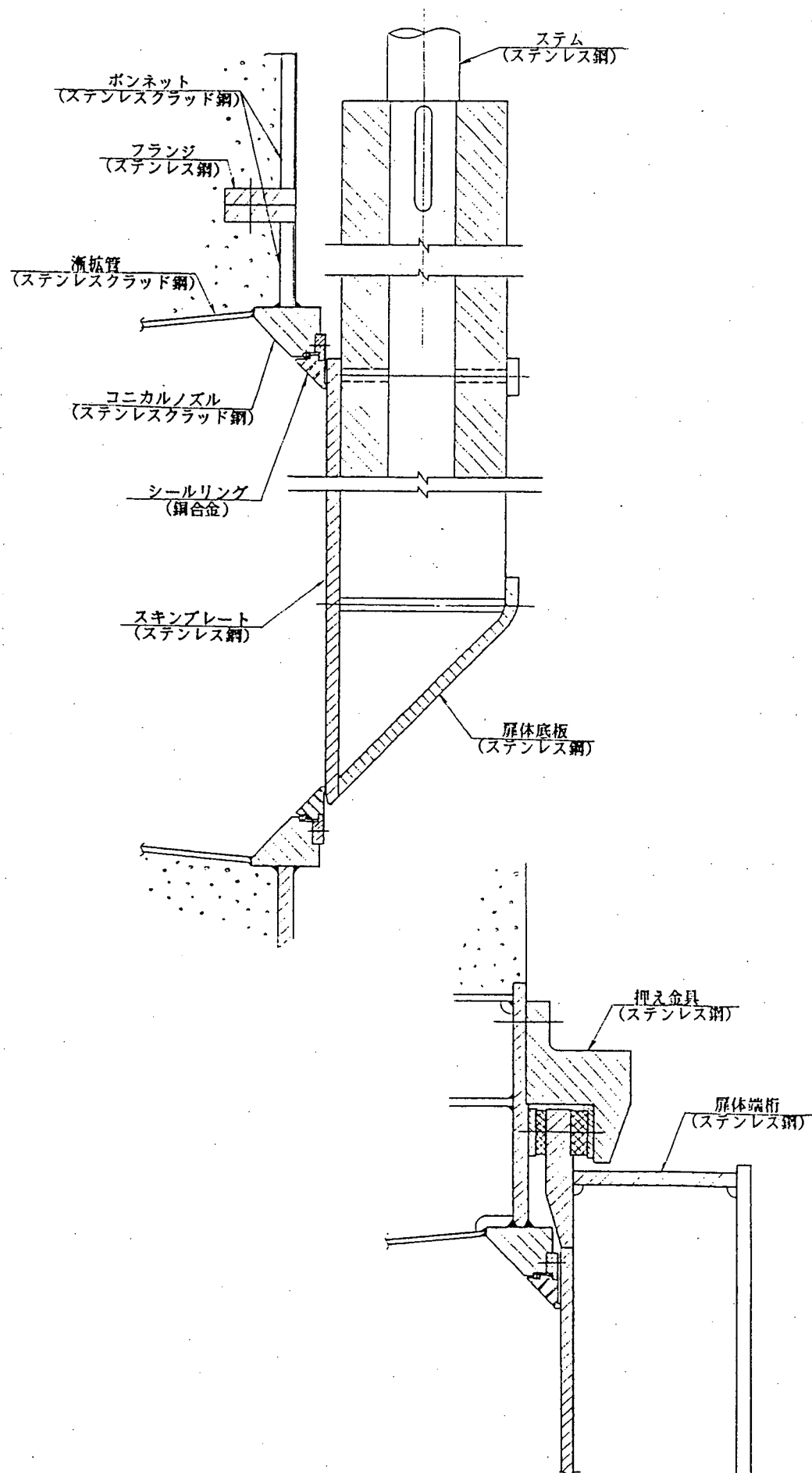
図解-3.14 扉体緒および水密部例 (ジェットフローゲートの場合)
