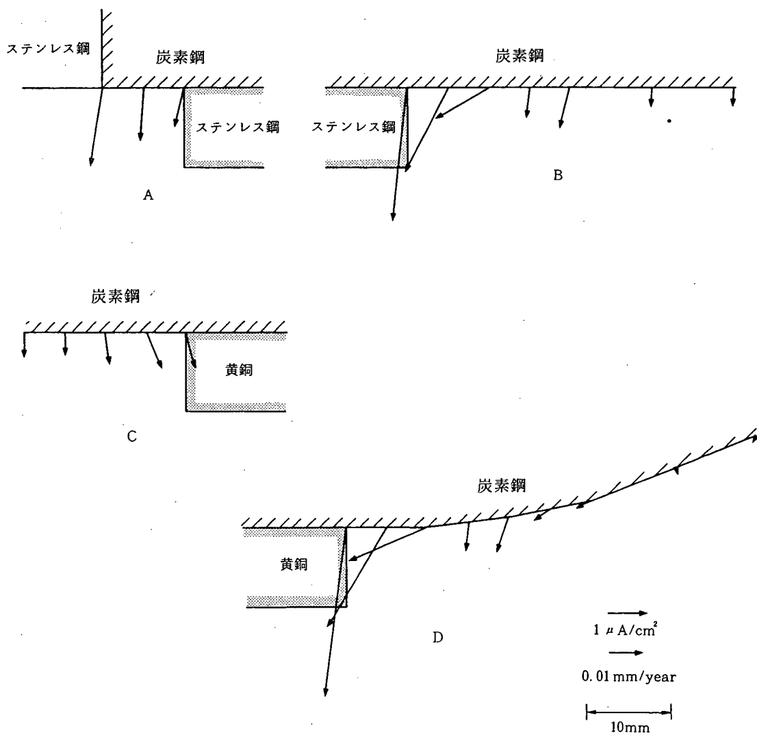
図解-2.25 戸当り部の電位分布および腐食電流の計算結果
