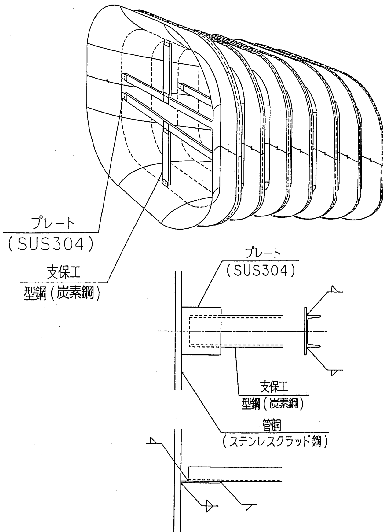
図解-4.3 支 保 工
