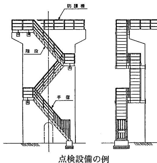
図解—5.7 その他の設備の例
