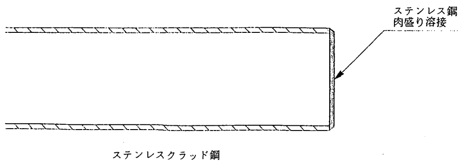
図解-3.4 ステンレスクラッド鋼の端面処理
