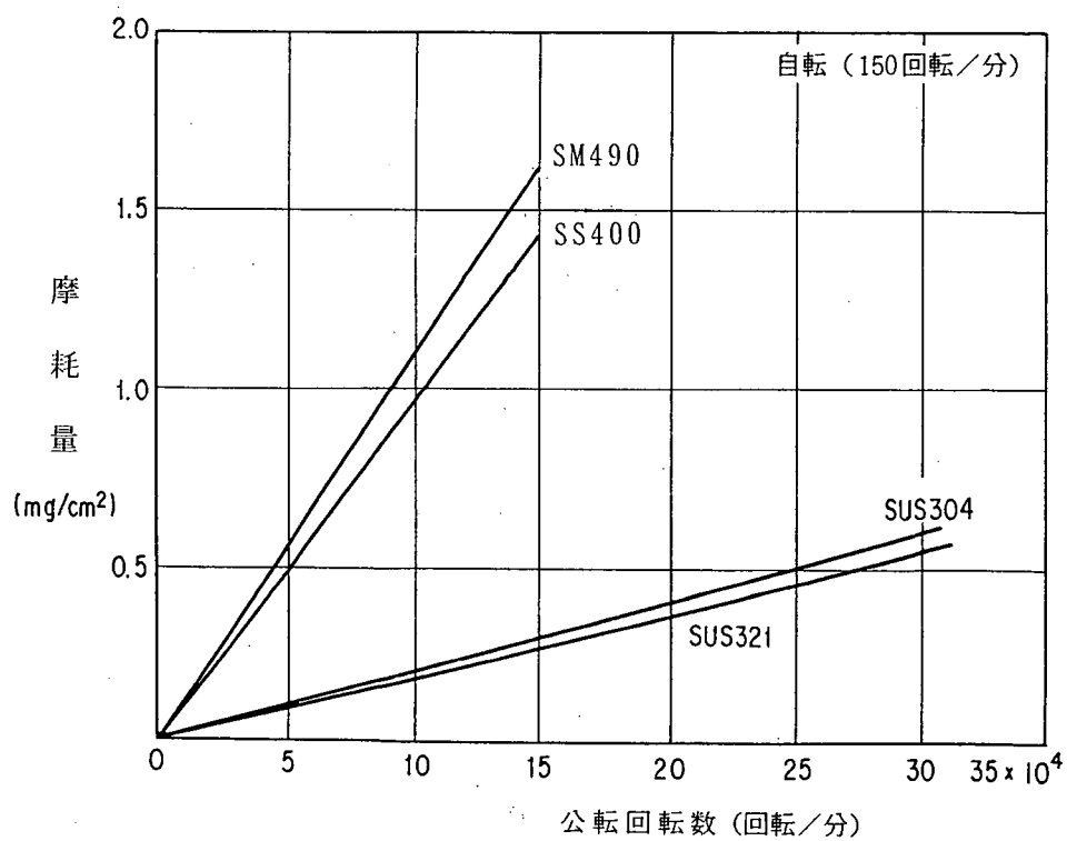
図解-2.10 鋼材の土砂摩擦
