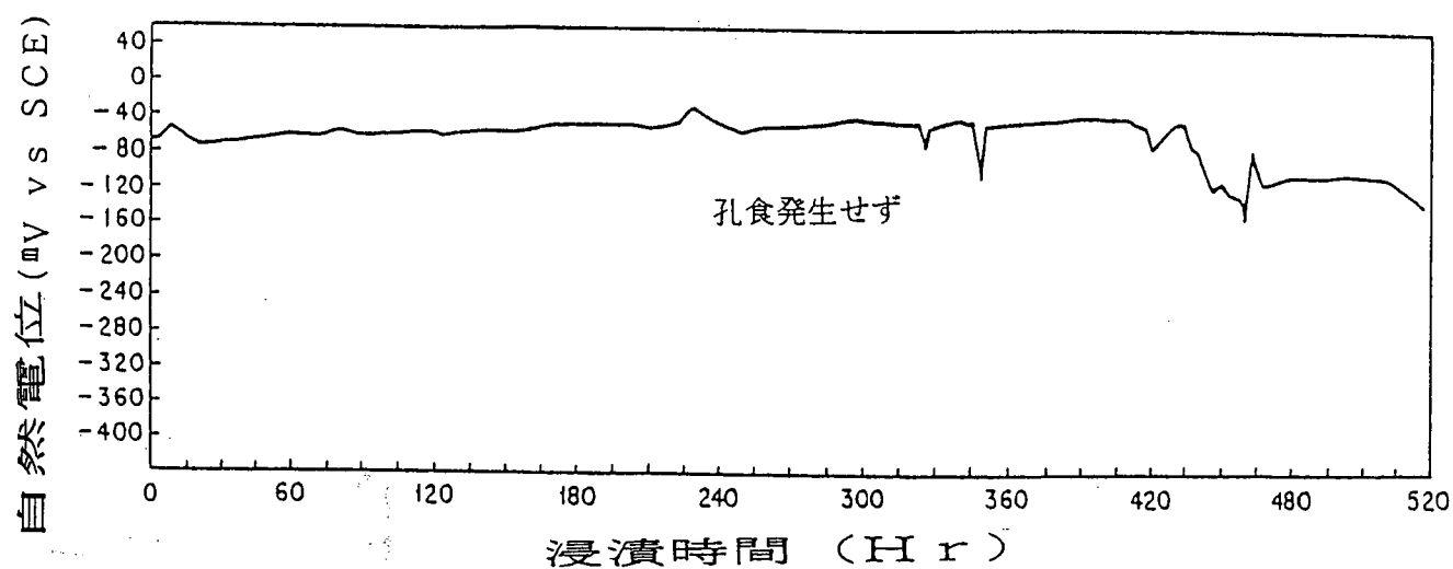
図解-2.29 20ppmCl - 単味溶液中でのSUS304の自然電位の経時変化
