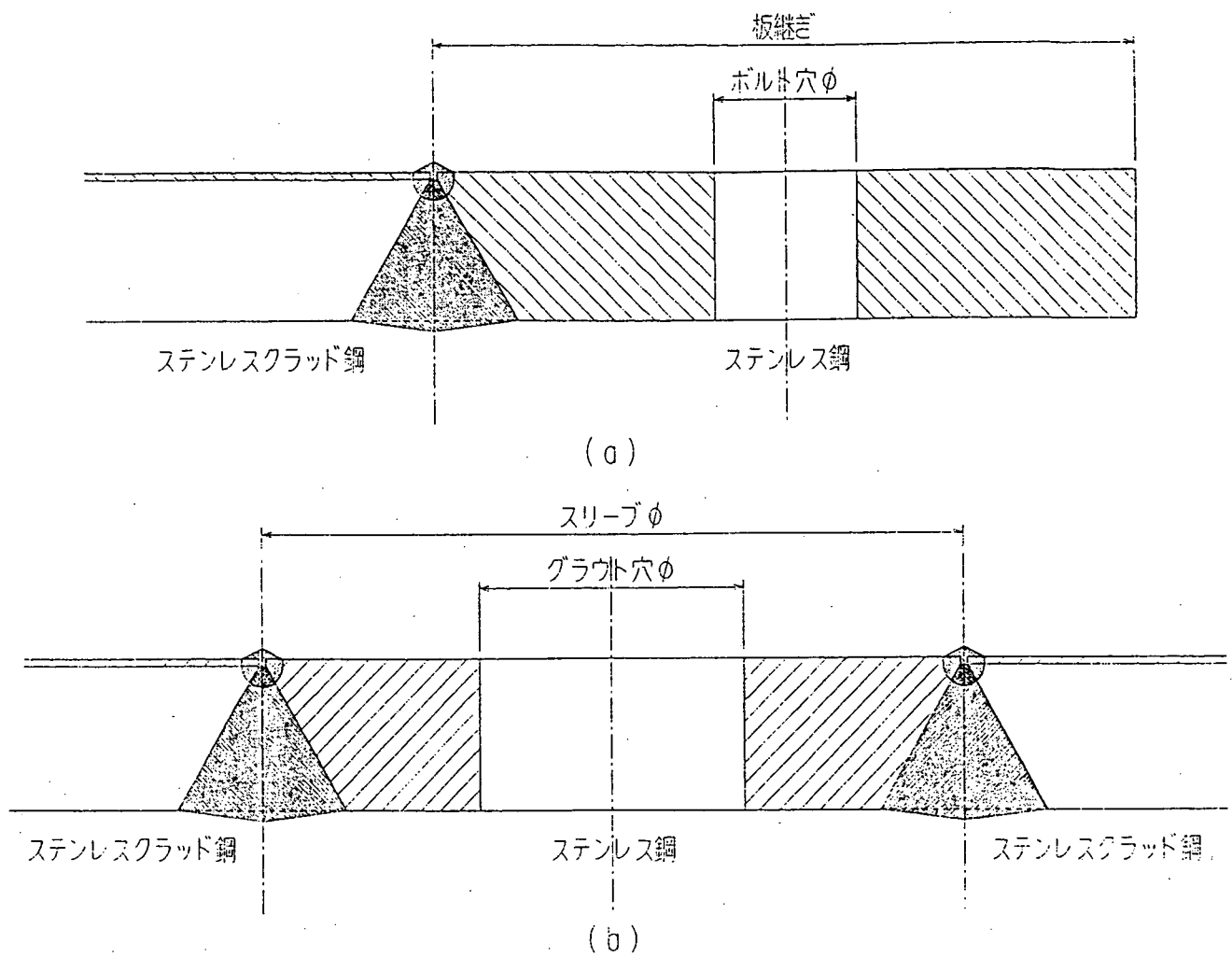
図解-3.5 ステンレスクラッド鋼に孔明けを行うときの処理
