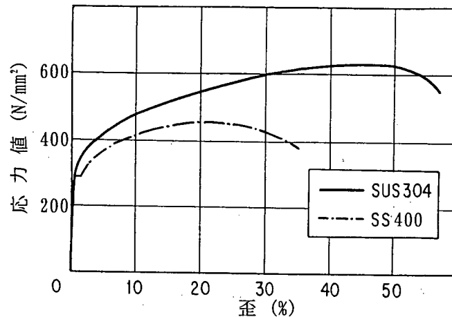
図解-2.7 応力～ひずみ曲線
