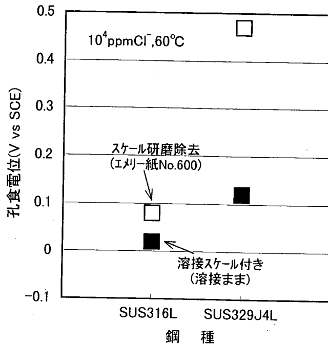
図解-2.32 ステンレス鋼の熱影響部の溶接スケールによる耐孔食性の劣化 10) (TIG共金溶接材) (ステンレス鋼便覧第3版)
