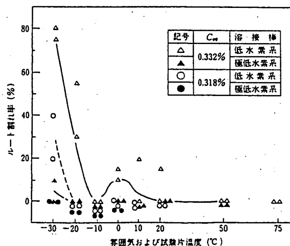
図解-4.9 低温雰囲気における溶接割れ試験結果 (山崎・北田:溶接学会講演概要第139集)
