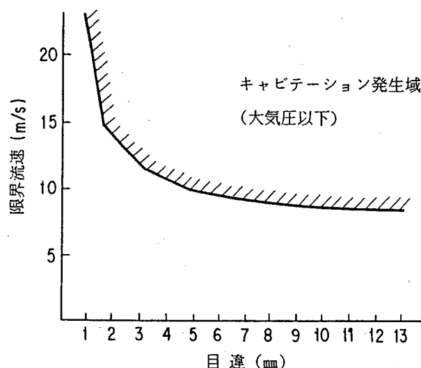
図解-3.12 突起高さとキャビテーション発生限界流速（ダム・堰施設設計基準（案））
