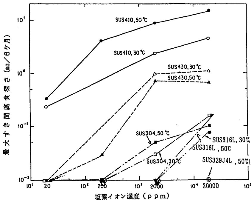
図解 3.18 すき間腐食深さに及ぼす塩素イオン濃度の影響
