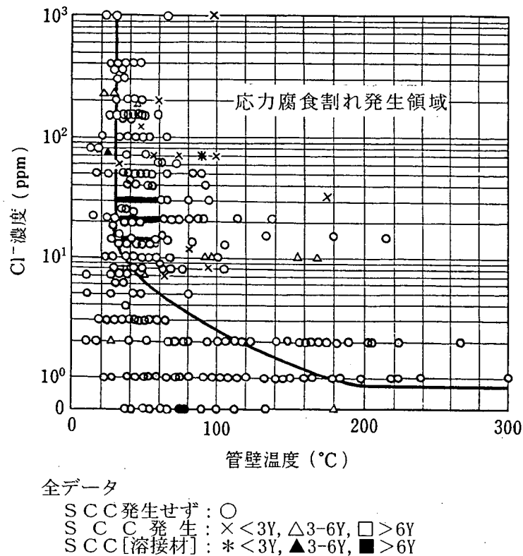
図解-2.18 ステンレス鋼熱交換器における冷却/加熱媒体中の Cl - 濃度・管壁温度とSCCとの関係(SUS304)
