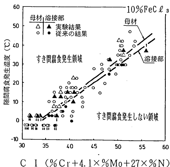
図解-2.16 C I とすき間腐食発生温度との関係
