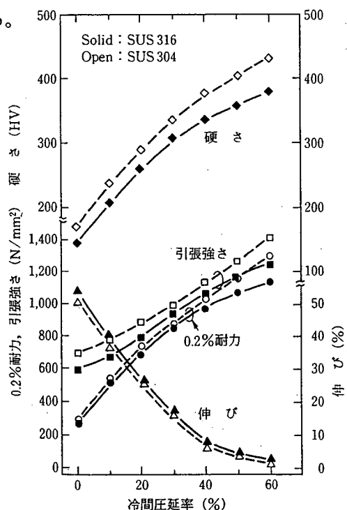
図解-2.5 引張特性に及ぼす冷間圧延の影響 (ステンレス鋼便覧第3版)
