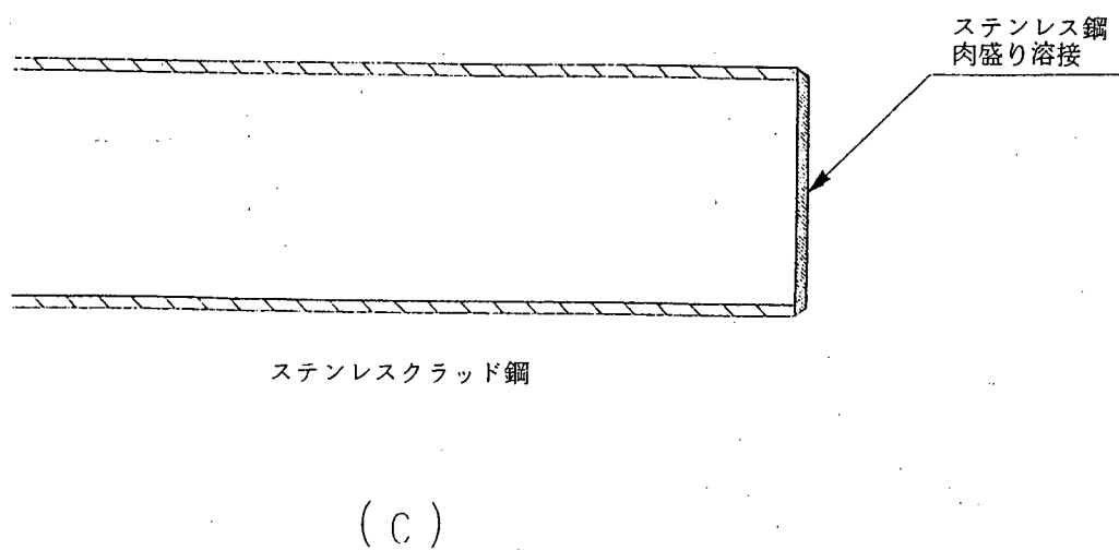
図解-5.12 ステンレスクラッド鋼の端面処理
