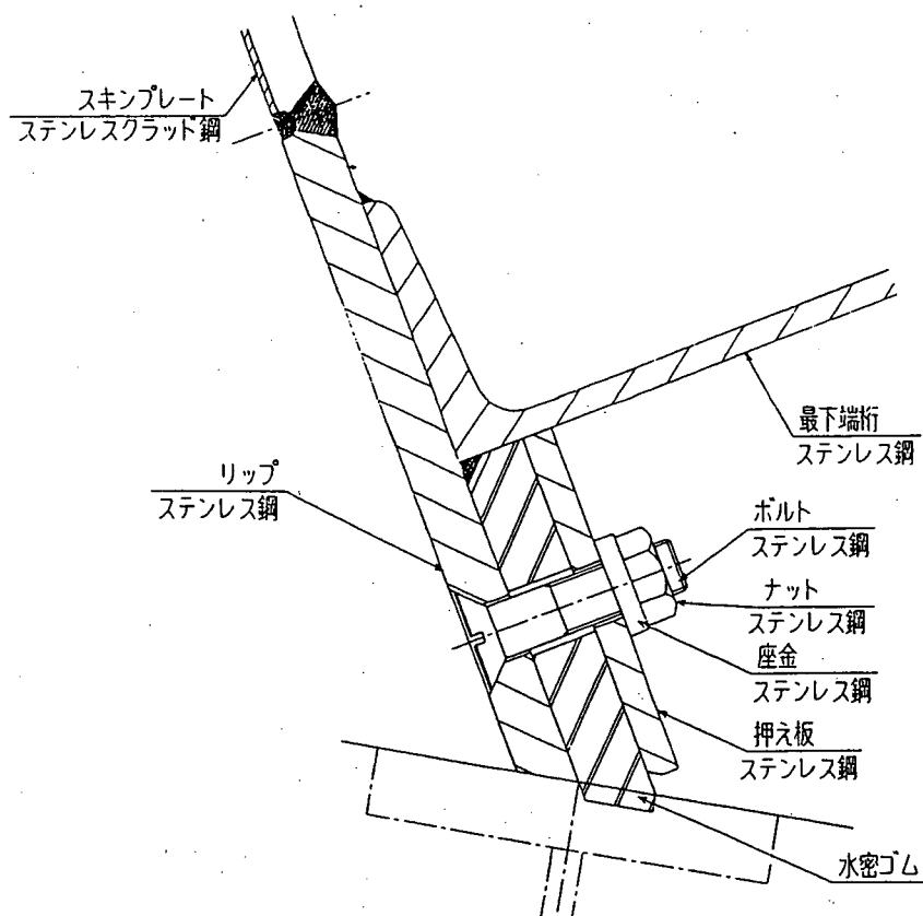
図-3.7 扉体下部例（クレストラジアルゲートの場合）
