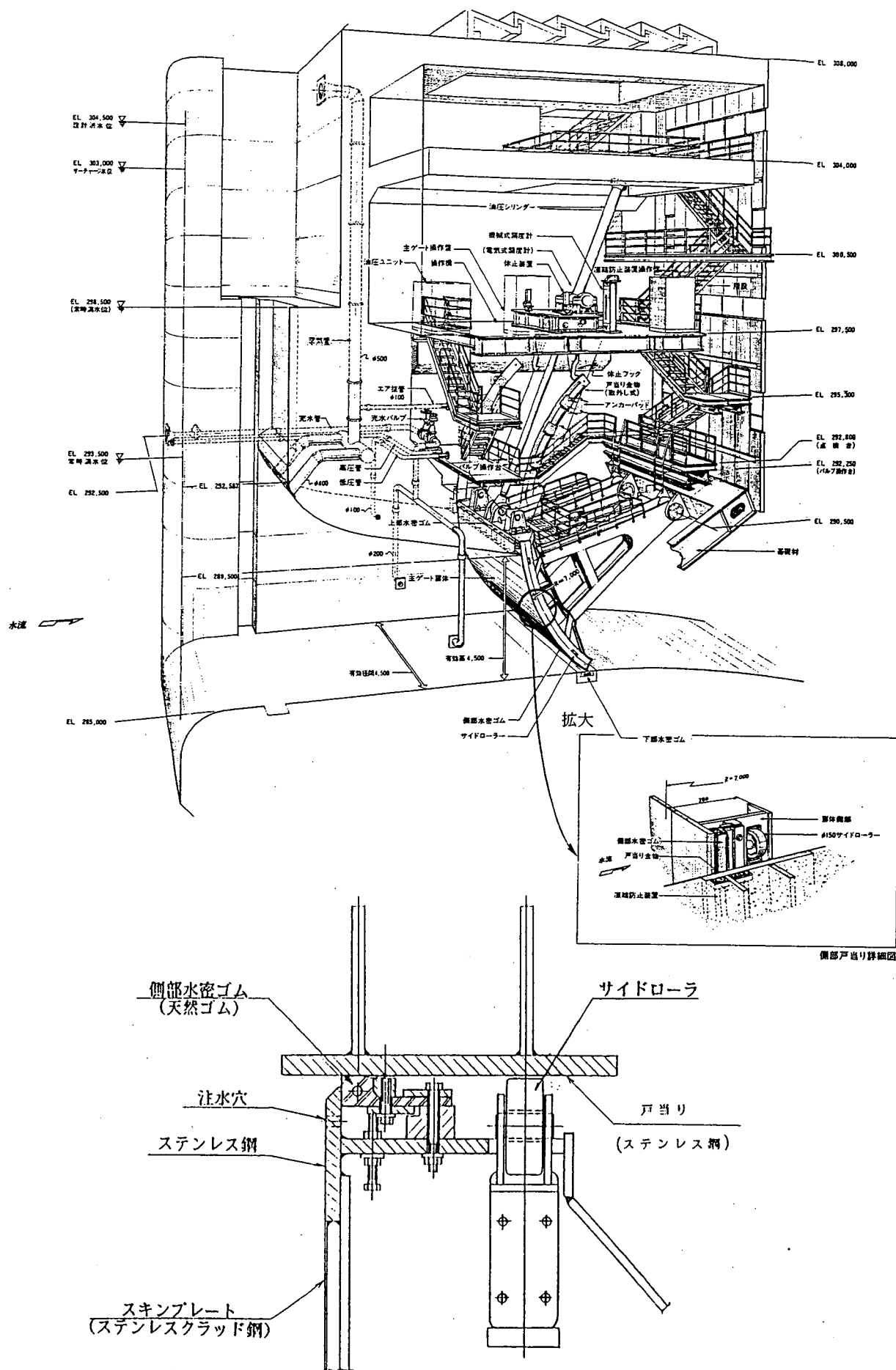
図解-3.6 扉体端部の例 (高圧ラジカルアーゲートの例)
