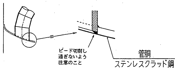
管胴継手部詳細
