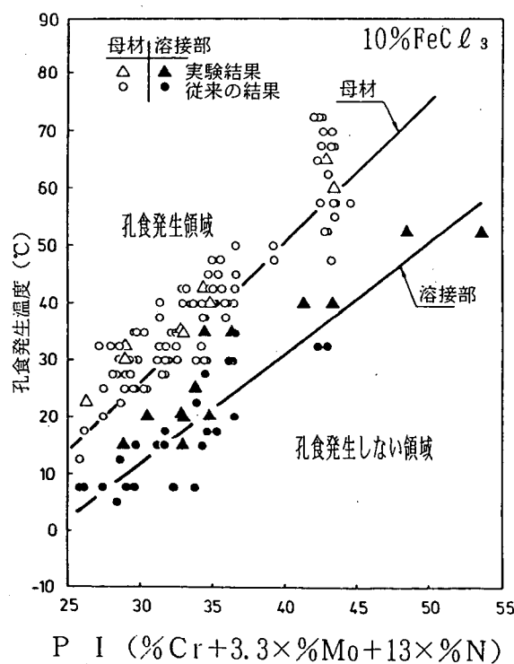
図解-2.15 P I と孔食発生温度との関係
