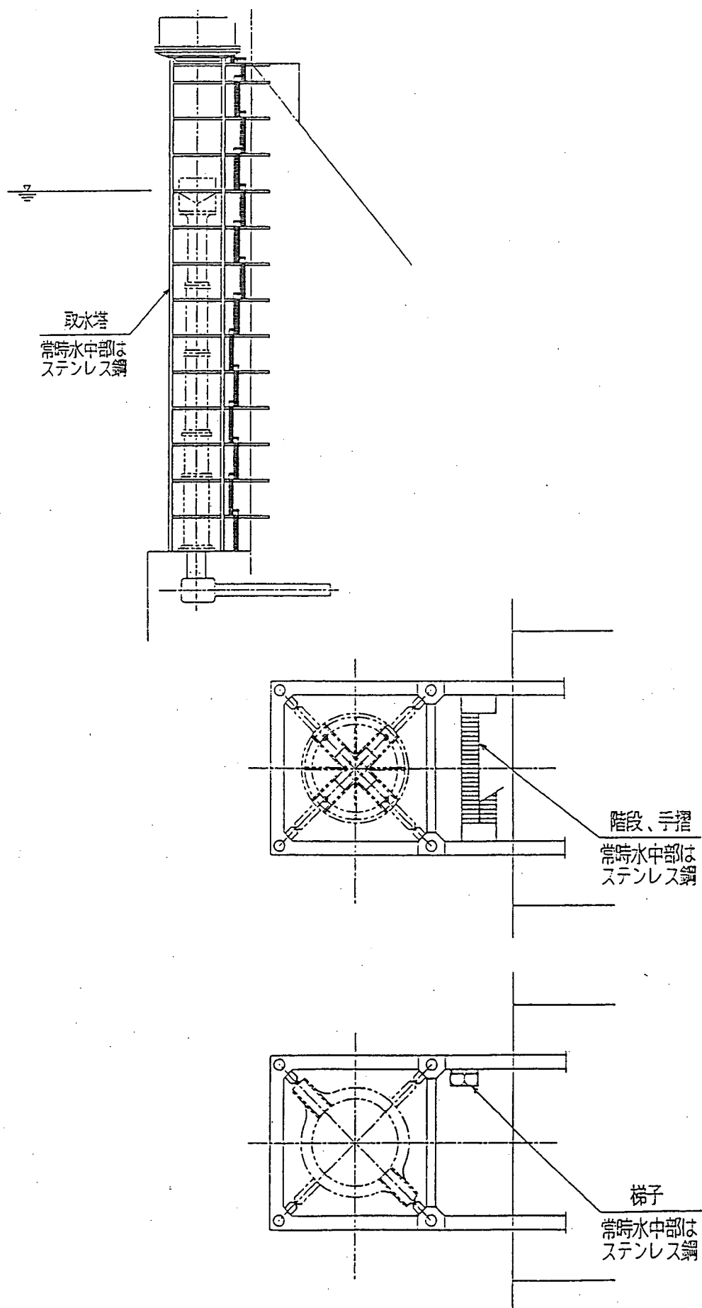
図解-3.16 鋼製取水塔（堤体付きの例）
