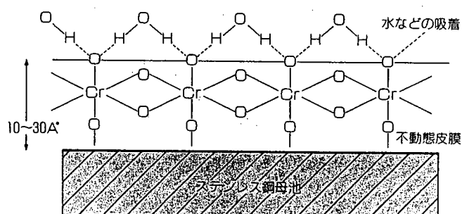
図解-2.11 不動態皮膜の概念図
