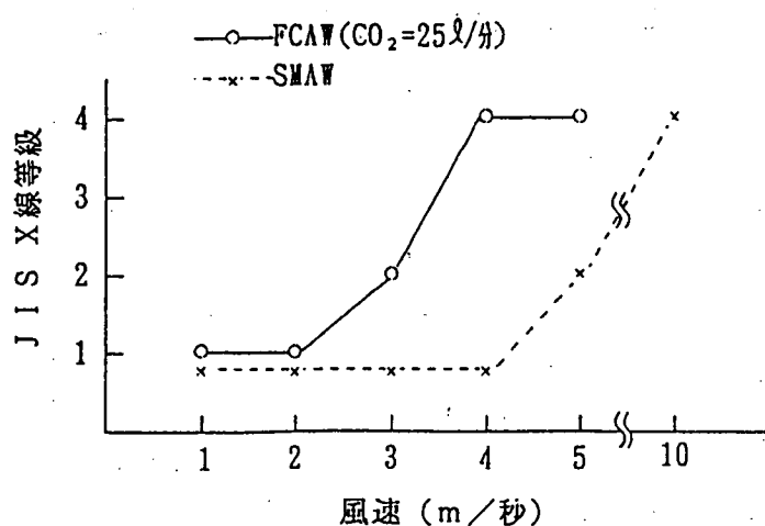
図解-4.8 溶接欠陥と風速の関係 (溶接協会・溶接棒部会資料)
