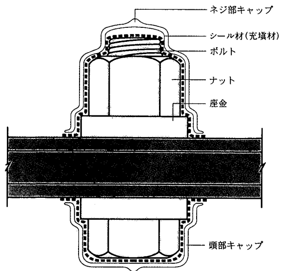
図解-5.13 ボルトキャップの取付状況
