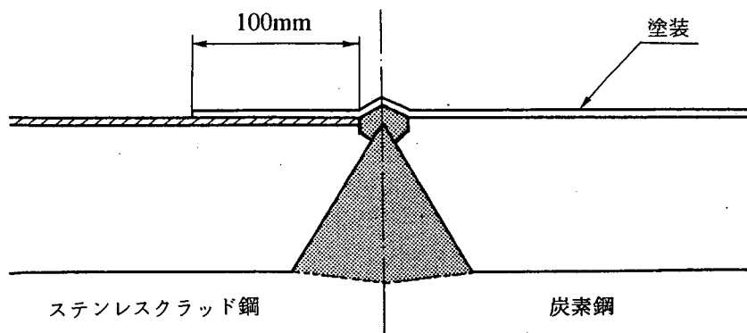
図解-3.2 塗装の塗り越し
