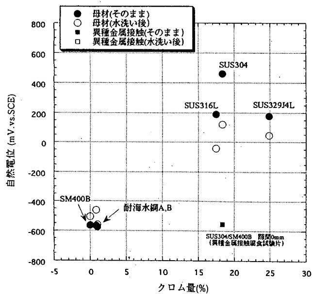
図解-2.37 母材腐食試験における自然電位 (江戸川上流水中部)
