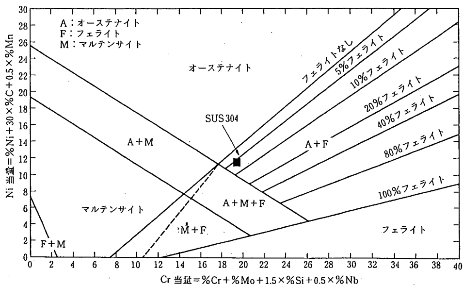
図解-2.4 シェフラーの組織状態図
