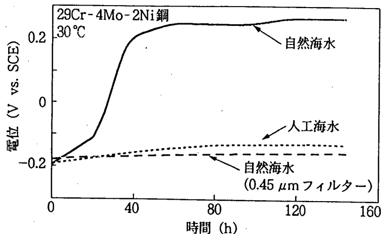
図解-2.34 自然海水および人工海水中でのステンレス鋼の自然電位変化
