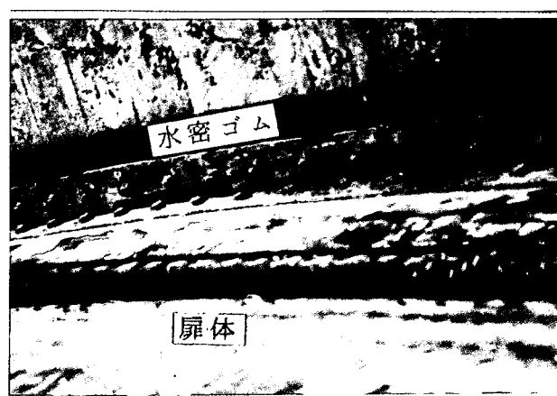
写真解—5.2 水密ゴム押え板および扉体吊金物(常時水中部)の腐食例
