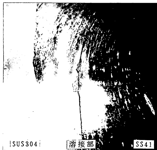
写真解-5.4 放流管溶接線(炭素鋼とステンレス鋼との溶接)付近の塗装部(炭素鋼側)の塗膜のふくれ例
