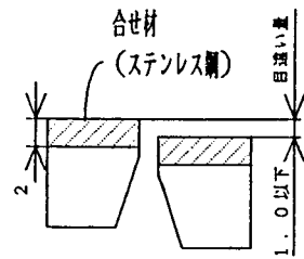
図解-4.10 ステンレスクラッド鋼の目違い量
