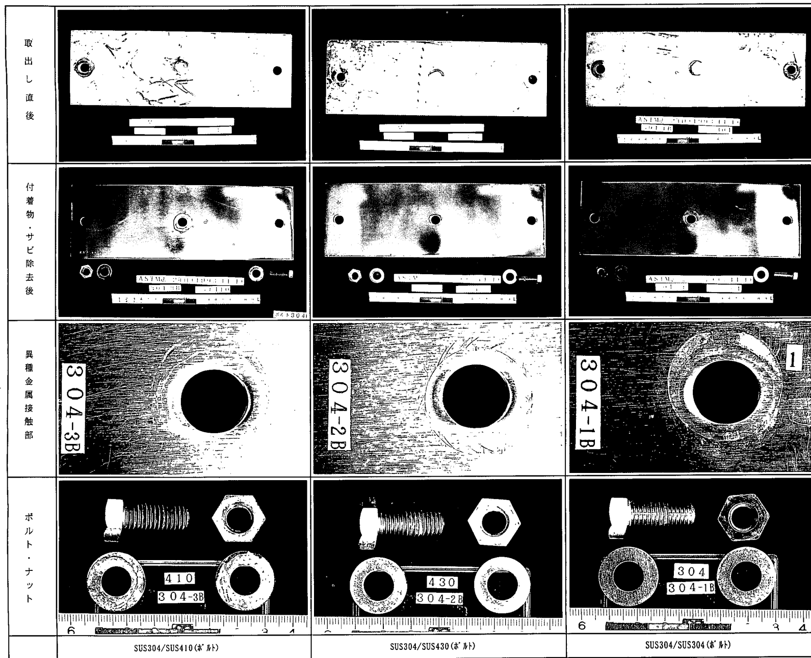
写真-2.3 異種金属ボルトによるすき間腐食試験後の腐食状況 [七が宿ダム湖, 2年間暴露データ]
