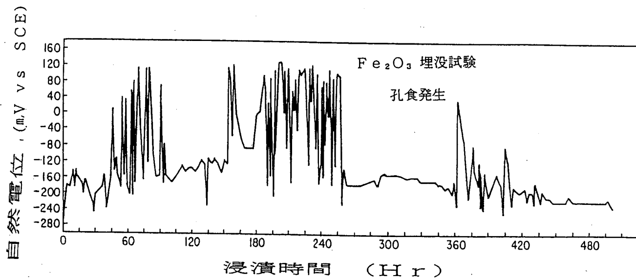
図解-2.30 Fe 2 O 3 に埋没したSUS304の自然電位の経時変化
