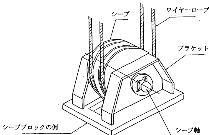
図解-3.8 シーブブロックの例
