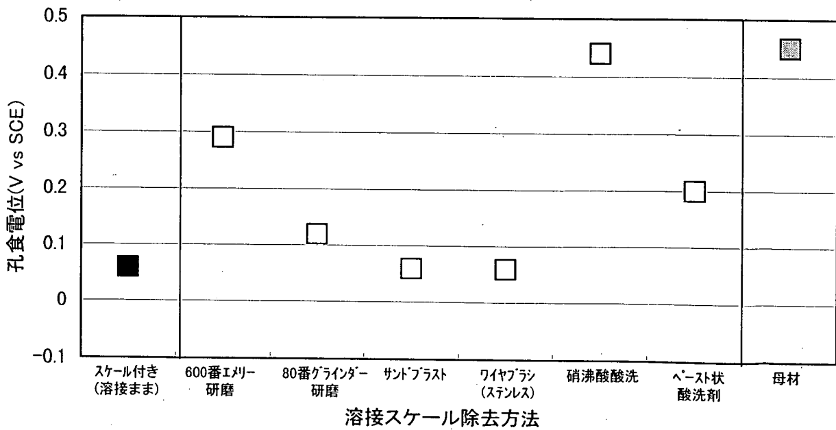
図解-2.33 耐孔食性に及ぼす溶接スケール除去方法の効果 1) [SUS329J4L, TIG共金溶接材, 人工海水, 80°C] (幸英昭: 材料と環境 40(1991))
