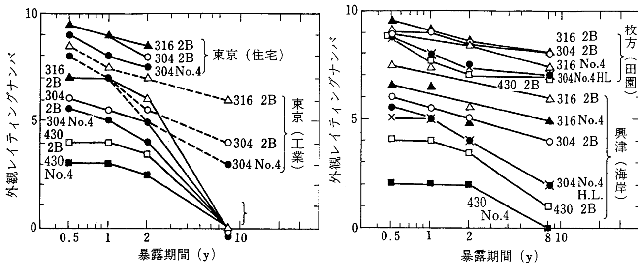
図解-2.12 各種環境におけるステンレス鋼の耐候性 (外観レーティングナンバー経時変化)
