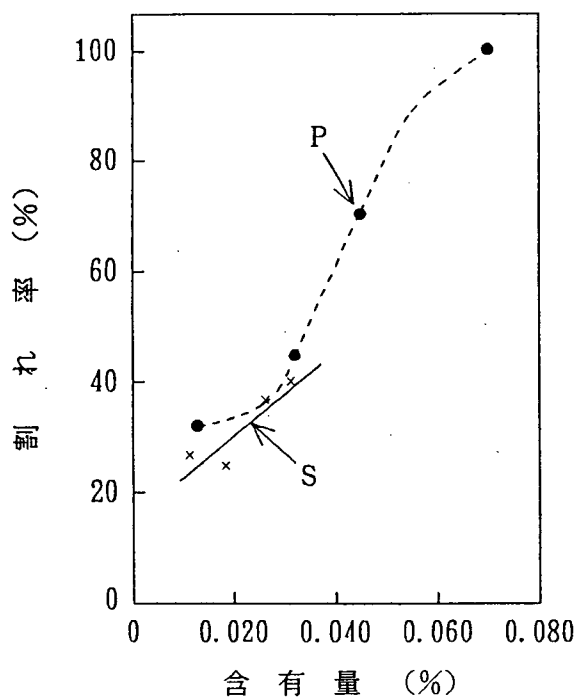
図解-4.12 溶接金属中のPおよびSのビード割れに及ぼす影響 (D316)
