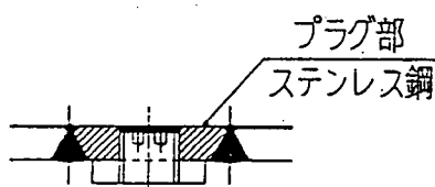
図解-3.11 ステンレスクラッド鋼使用上の留意箇所（主放流設備の場合）
