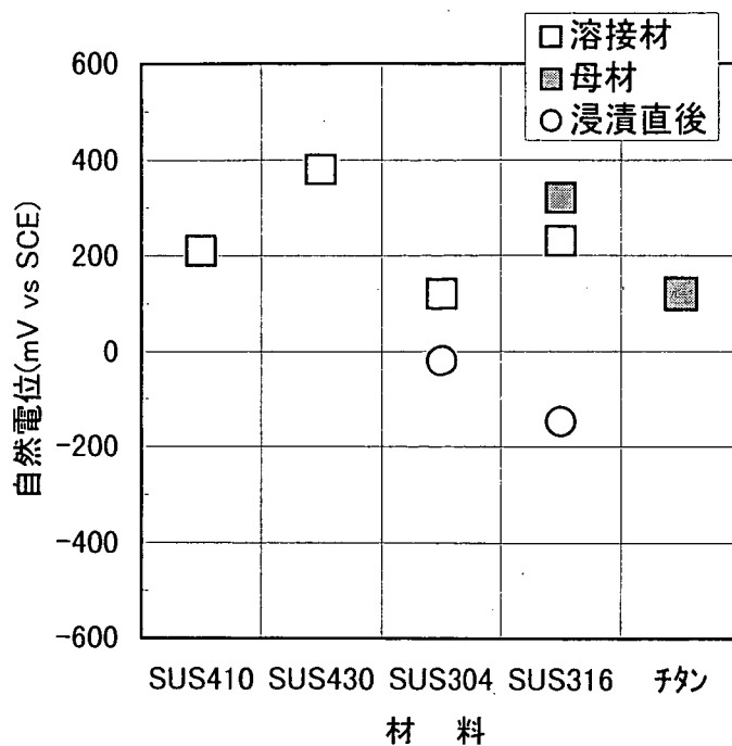
図解-2.36 セヶ宿ダム湖暴露試験3年経過後の自然電位測定結果
