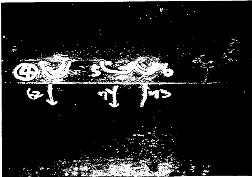
写真解-5.1 扉体桁上の孔食(鋼材+塗装部)の例
