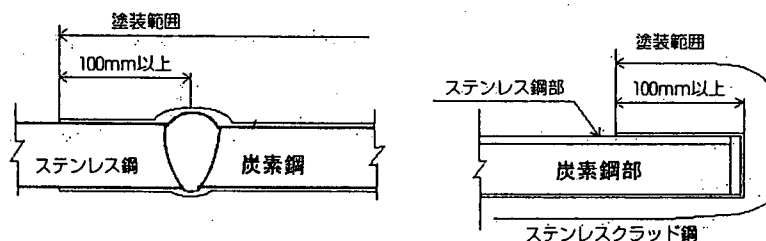
図解－5.8 ステンレス鋼と炭素鋼の接触部の塗装例
