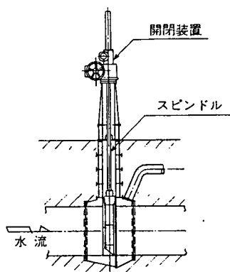
図解-5.3 スピンドル式開閉装置の例
