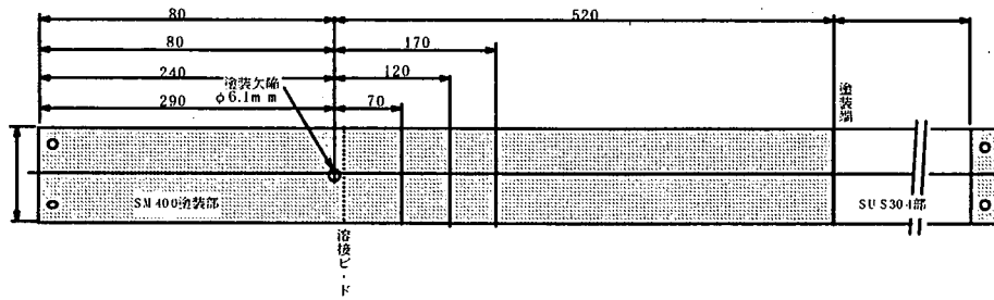
タイプ B 暴露試験片（ステンレス鋼側塗装）
