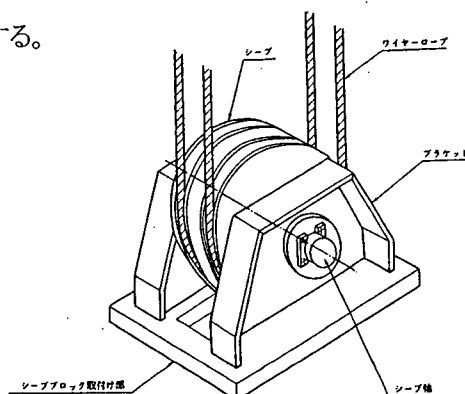
図解-5.2 扉体付シーブブロックの例
