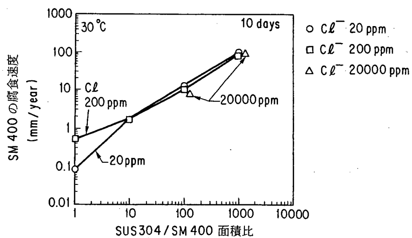
図解-2.22 異種金属接触腐食に与える面積比（ステンレス鋼：炭素鋼）の影響
