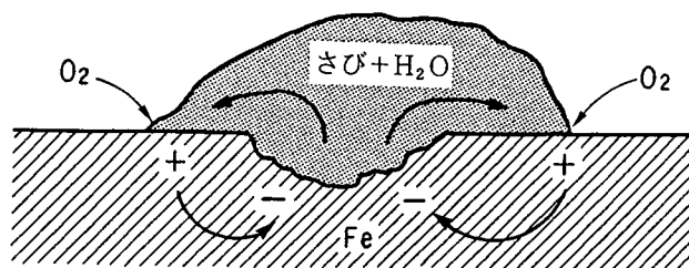
図解-2.27 鉄の表面に存在するさびによって形成された通気差電池 (腐食反応とその制御)
