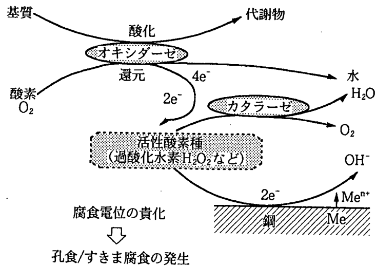
図解-2.35 海水中におけるステンレス鋼の微生物腐食メカニズム (好気性バクテリアによる微生物腐食)
