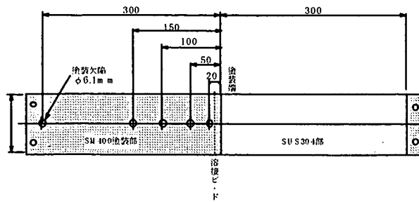
タイプ A 暴露試験片（炭素鋼側塗装）
