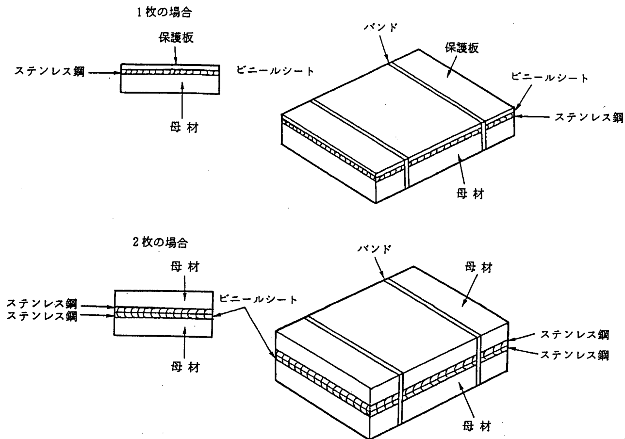
図解-4.1 ステンレスクラッド鋼板の荷姿例（工場納入時）
