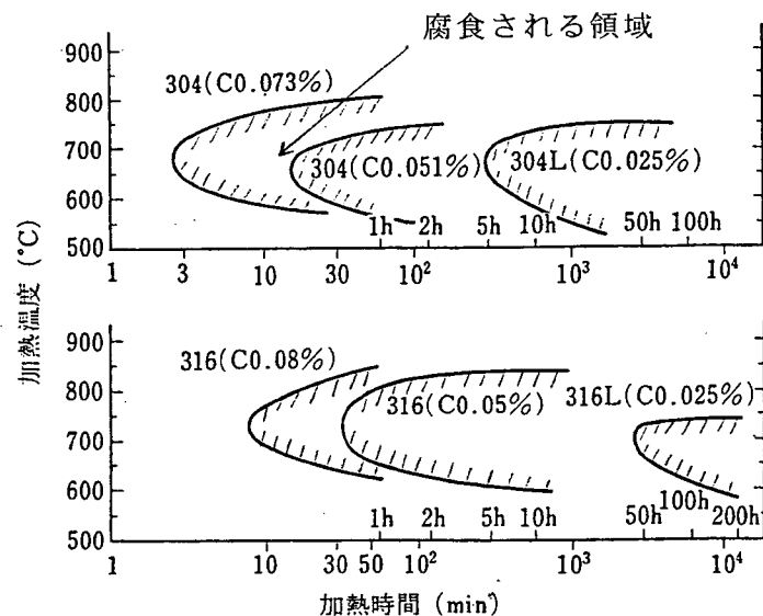
図解-2.17 SUS304・SUS316系ステンレス鋼のT T S 曲線 (硫酸・硫酸銅試験) ハッチ部：鋭敏化域
