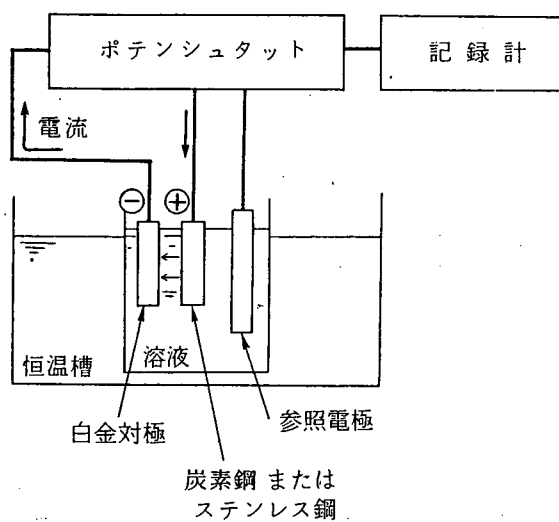
図解-2.23 分極測定の方法
