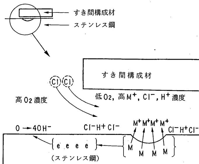
図解-2.26 すき間内部での腐食反応の概念図 (防食技術便覧)
