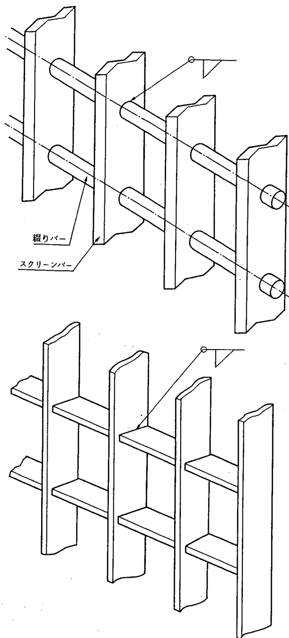
図解-3.15 スクリーンパネルの構造 (溶接構造の例)
