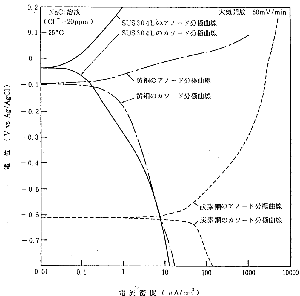
図解-2.24 分極測定結果（20ppm NaCl溶液中）
