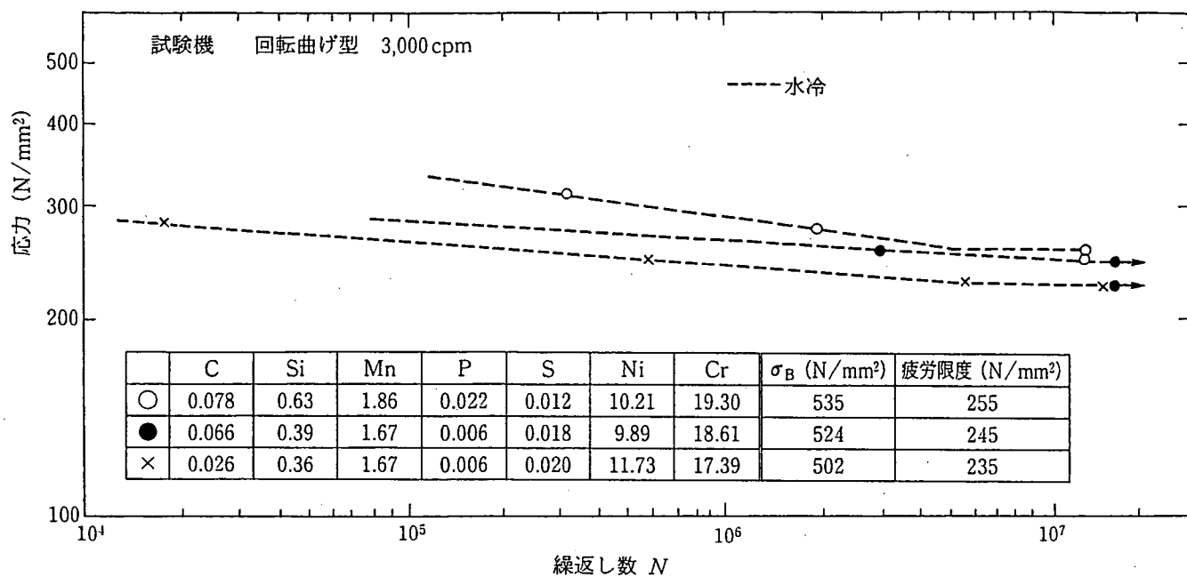
図解-2.8 SUS304のS-N曲線
