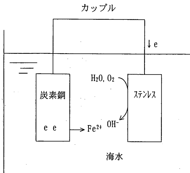
図解-2.20. 異種金属接触腐食現象
