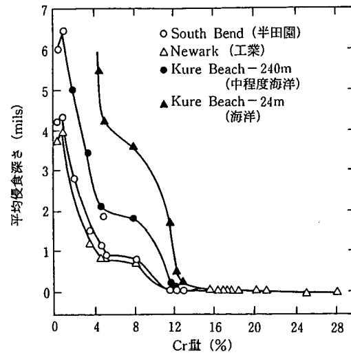
図解-2.3 Fe-Cr合金の8年間大気暴露結果
