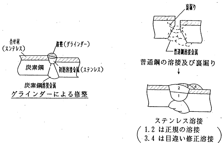
図解-4.7 目違いが大きい場合の溶接方法の例
