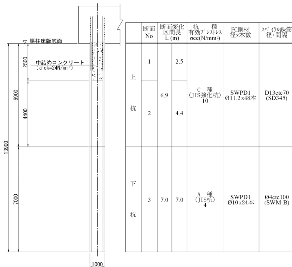
図-3.2.10 PHC 杭の各断面の定数
