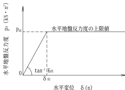
図-3.3.18 杭の軸直角方向抵抗特性
