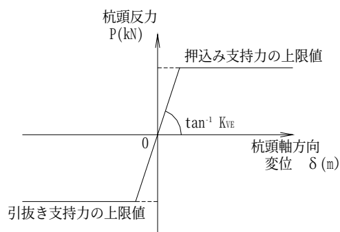
図-3.3.17 杭の軸方向の抵抗特性
