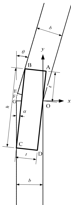
図-付 3.3 厳密解法の考え方（水流方向）
