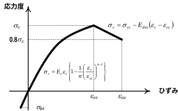
図-2.4.1 コンクリートの応力度－ひずみ関係（ \sigma_{cc} ：横拘束筋で拘束されたコンクリートの強度 ( \text{N/mm}^2 )、 \varepsilon_{cc} ：コンクリートが最大圧縮応力に達するときのひずみ、 \varepsilon_{cu} ：横拘束筋で拘束されたコンクリートの終局ひずみ、 E_c ：コンクリートのヤング係数 ( \text{N/mm}^2 )、 E_{des} ：下降勾配 ( \text{N/mm}^2 )）
