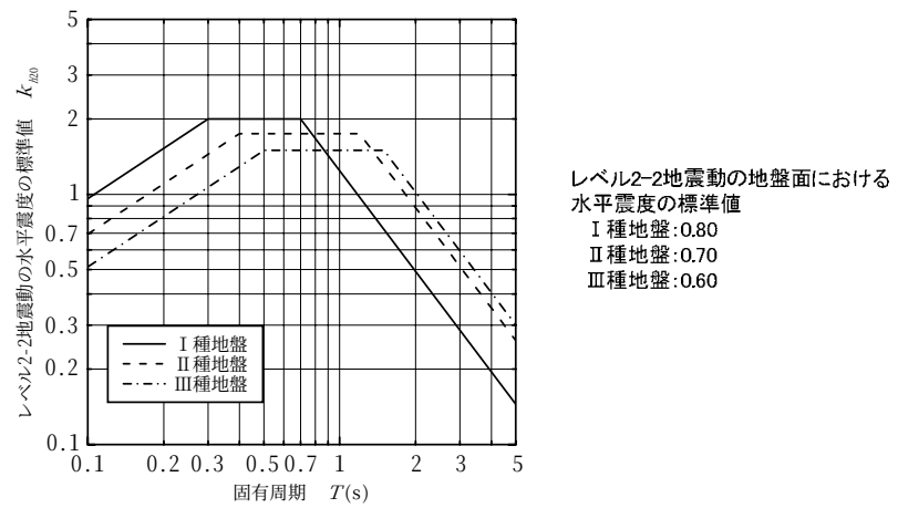
図-2.5.2 レベル 2-2 地震動の水平震度の標準値
