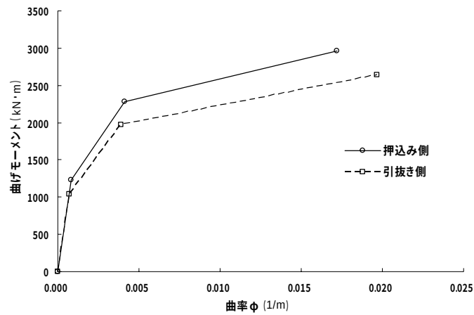
図-3.2.37 杭体の曲げモーメントー曲率関係（断面 No.1）
