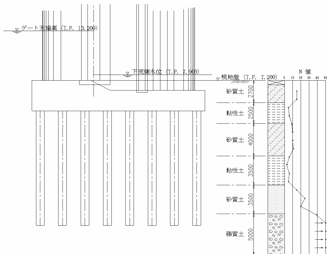
図-3.2.11 土質柱状図
