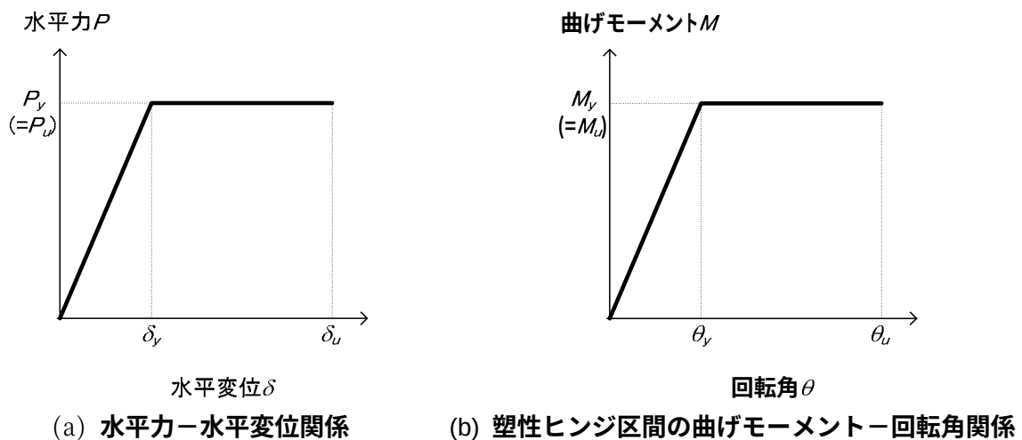
図-付 2.2 地震時の全水平荷重の作用重心における水平力－水平変位関係とそれに等価な塑性ヒンジ区間の曲げモーメント－回転角関係
