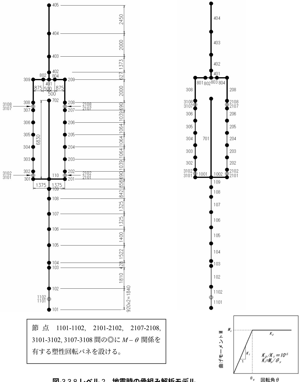
図-3.3.8 レベル 2 地震時の骨組み解析モデル
