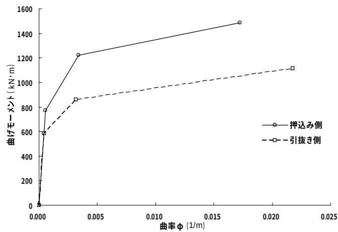
図-3.2.39 杭体の曲げモーメントー曲率関係（断面 No.3）
