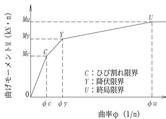
図-3.3.19 杭体の曲げモーメントー曲率関係
