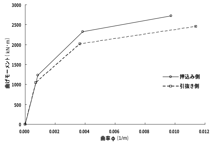
図-3.2.38 杭体の曲げモーメントー曲率関係（断面 No.2）
