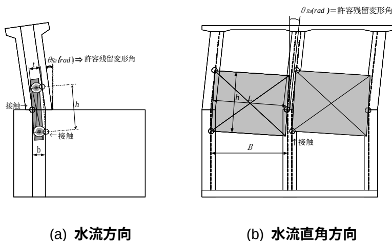
図-付 3.1 ゲートの開閉を妨げない門柱の許容残留変形角の算出方法の例 (指針（案）IV編 図解-4.5.1)
