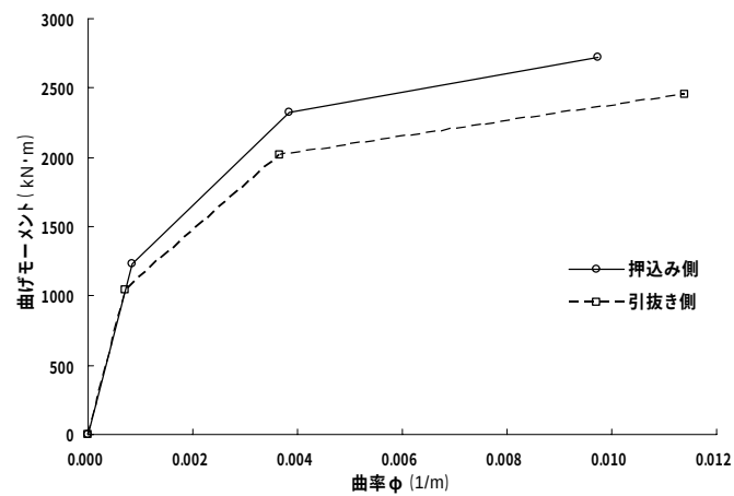
図-3.3.21 杭体の曲げモーメントー曲率関係（断面 No.2）
