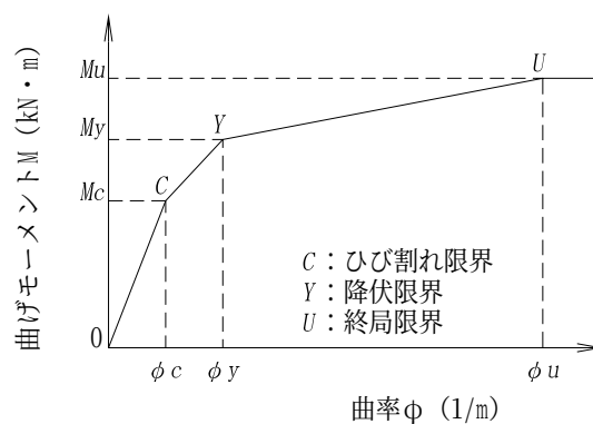
図-3.2.36 杭体の曲げモーメントー曲率関係
