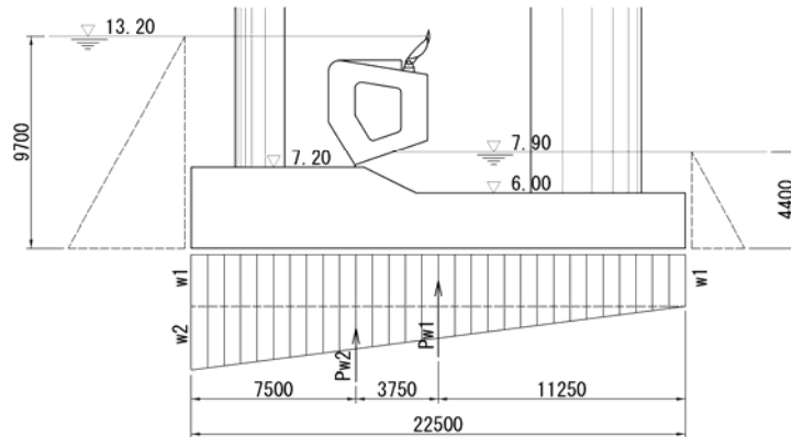
図-3.2.20 揚圧力
