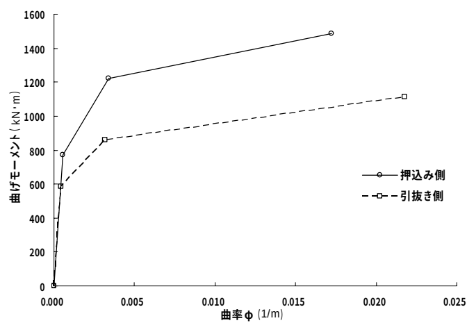
図-3.3.22 杭体の曲げモーメントー曲率関係（断面 No.3）
