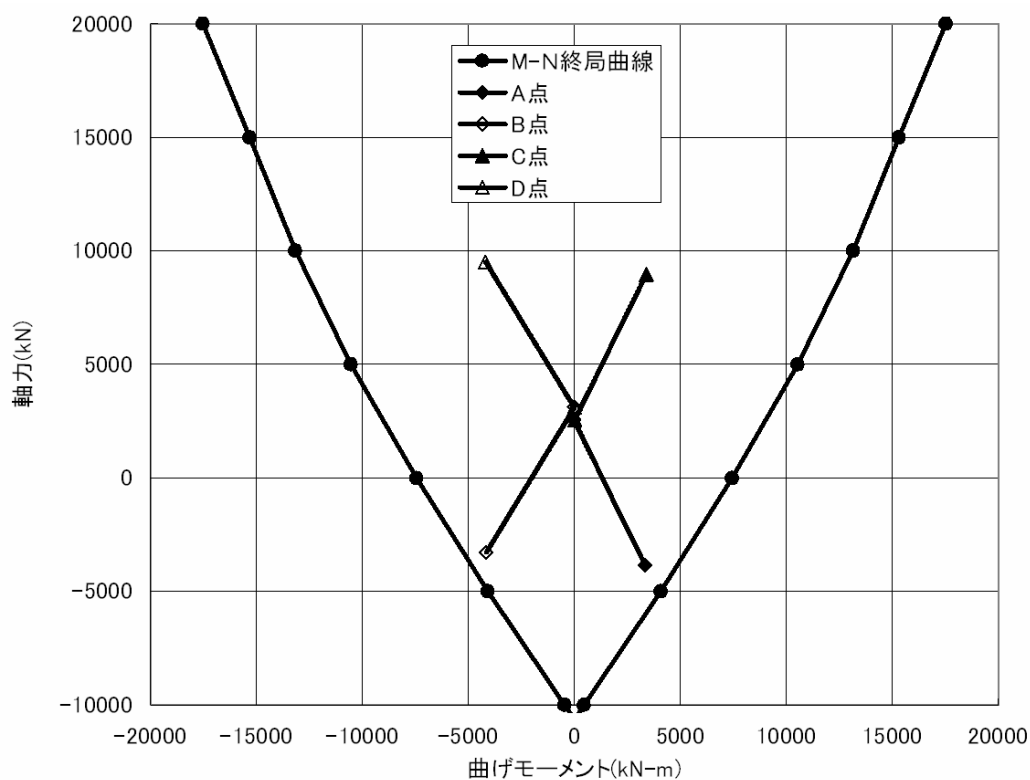
図-3.3.14 N-M_u 相関関係と発生 N-M (レベル 2-2 地震動)
