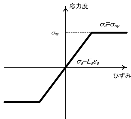
図-2.4.2 鉄筋の応力度 \sigma_s －ひずみ \varepsilon_s 関係（ \sigma_{sy} ：鉄筋の降伏点 ( \text{N/mm}^2 )、 E_s ：鉄筋のヤング係数 ( \text{N/mm}^2 )）
