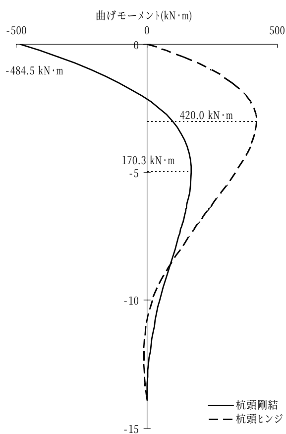
図-3.3.6 曲げモーメント図
