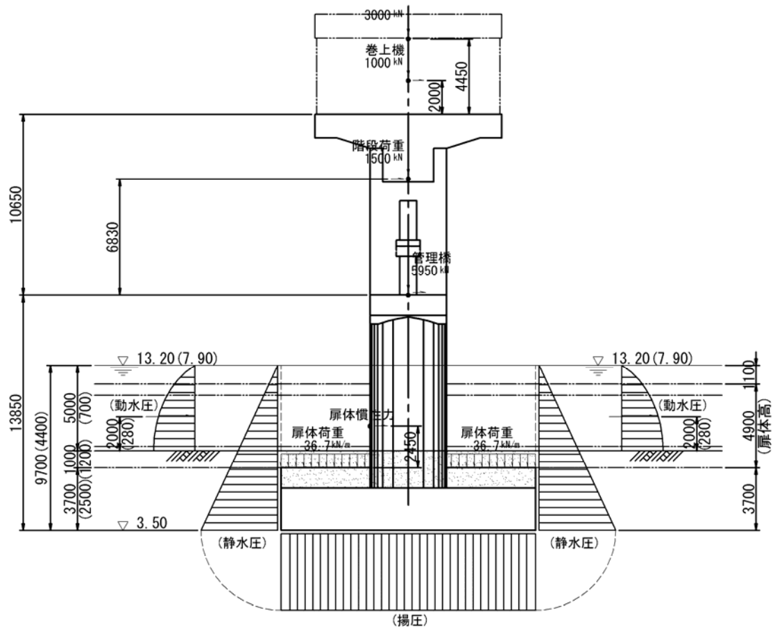
图-3.3.1 荷重条件（中央堰柱）
