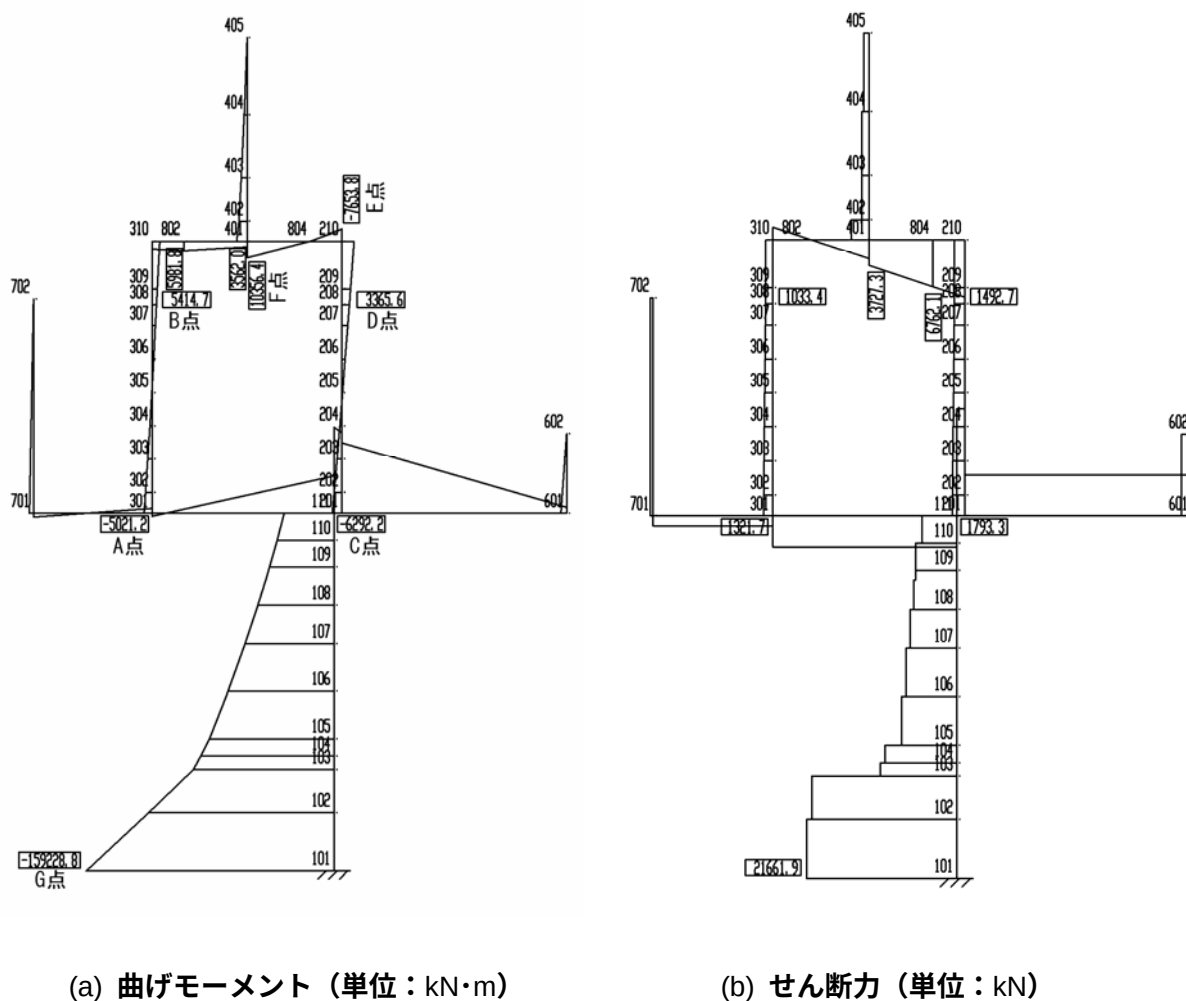
図-3.2.23 各部材に生じる断面力
