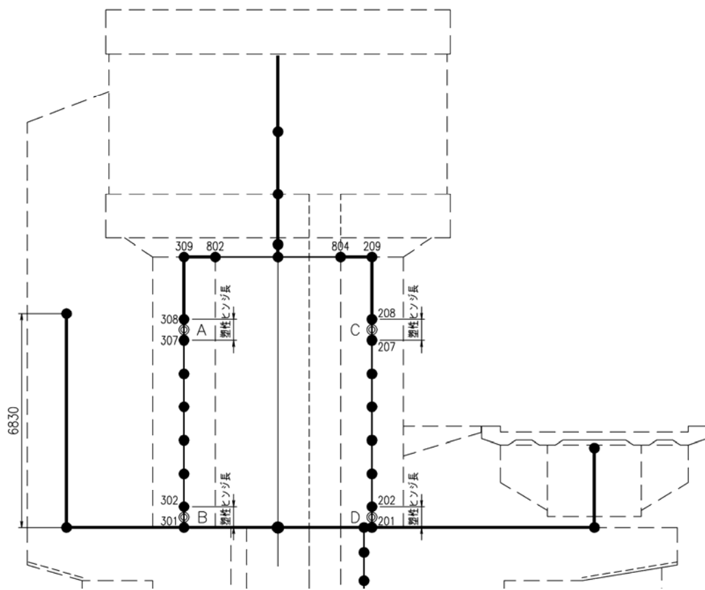
図-3.2.29 門柱のモデル化
