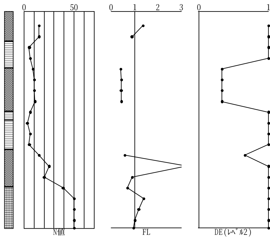
図-3.2.12 液状化の判定結果（レベル 2-1 地震動）
