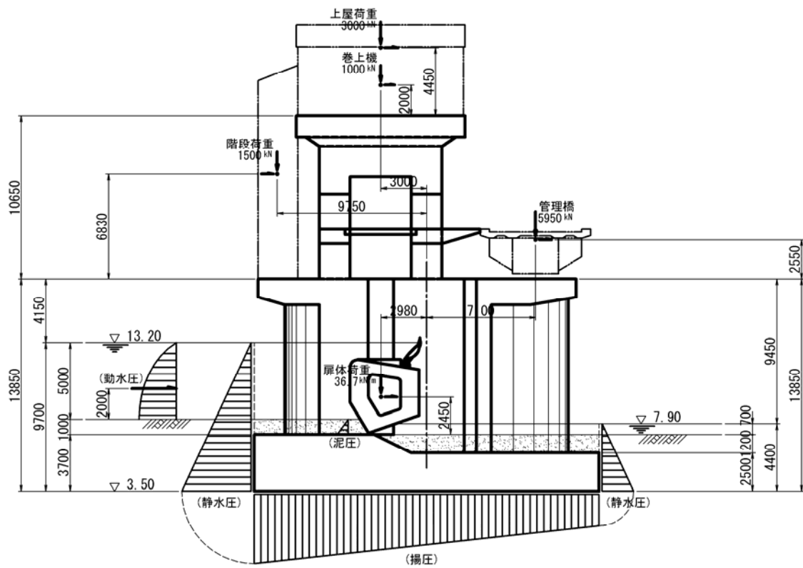
図-3.2.15 荷重条件 (中央堰柱)
