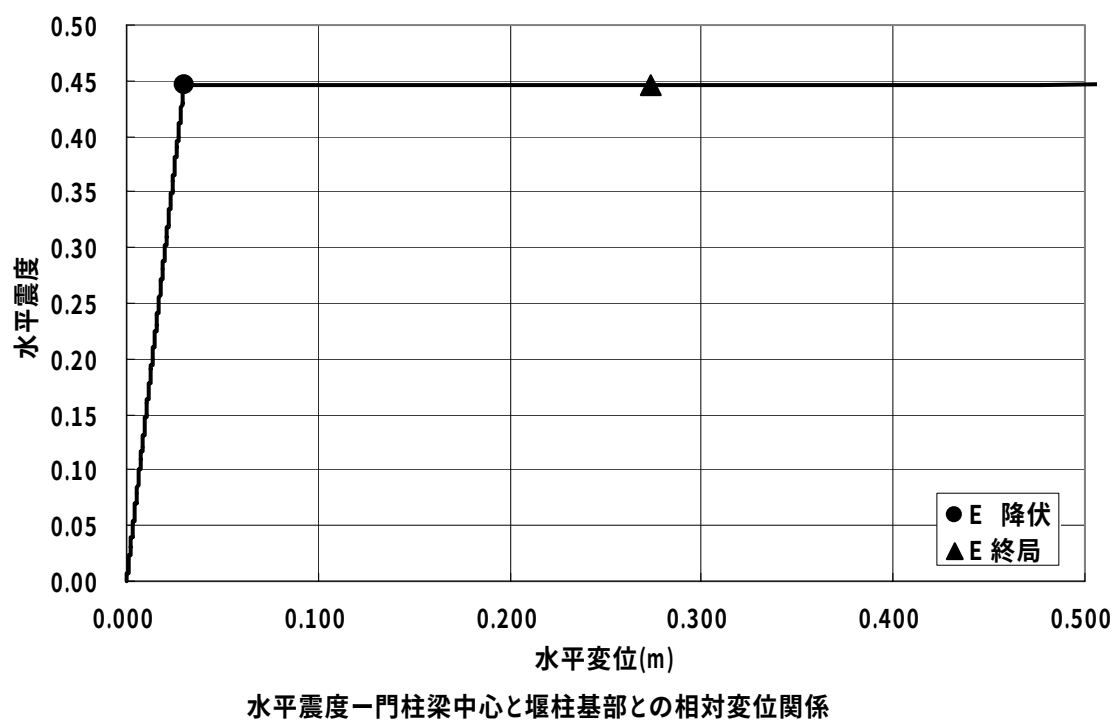
図-3.3.12 水平震度 k_h - 水平変位 \delta 関係(レベル 2-1 地震動、レベル 2-2 地震動)
