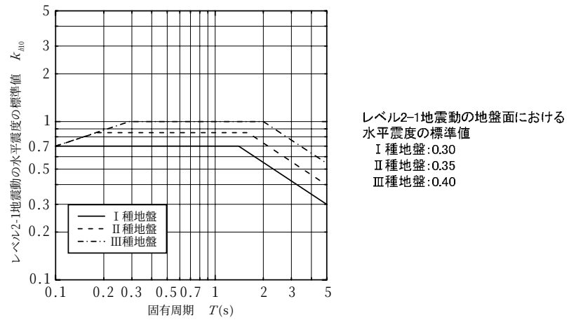
図-2.5.1 レベル 2-1 地震動の水平震度の標準値
