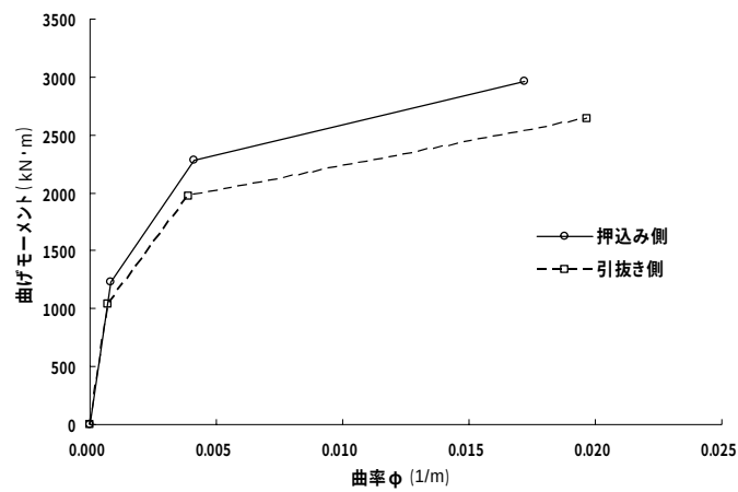
図-3.3.20 杭体の曲げモーメントー曲率関係（断面 No.1）
