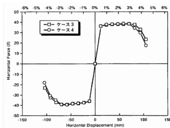
図-3.7 ケース 3 とケース 4 の荷重変位曲線の比較 14)
