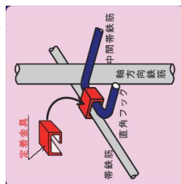
(c) クリップ式定着
