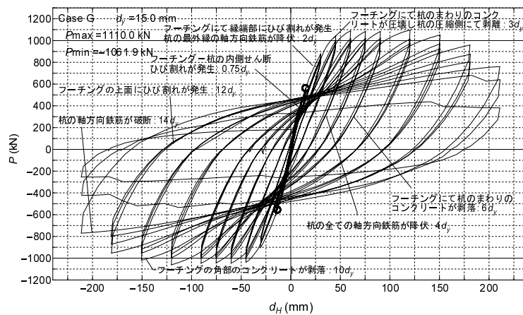
図-5.15 Case G：荷重変位関係
