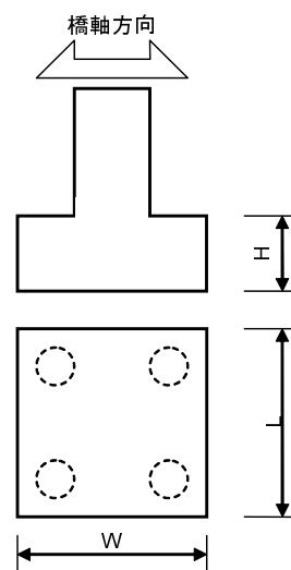
図-5.16 フーチング諸元の模式図
