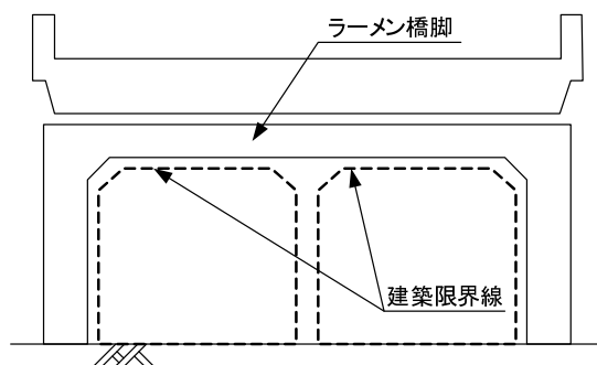
図-2.5 ラーメン橋脚の建築限界による断面寸法の制約 (模式図)
