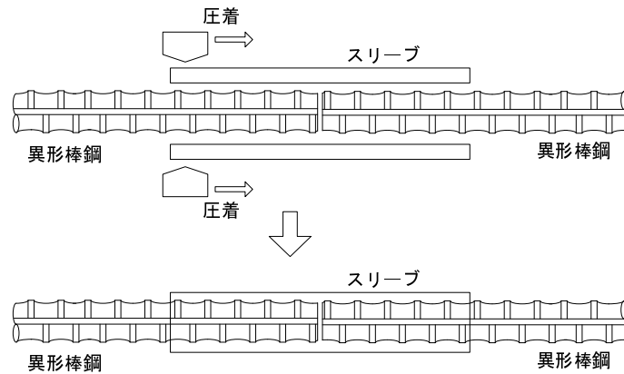
図-4.1 スリーブ圧着継手の例 (模式図)
