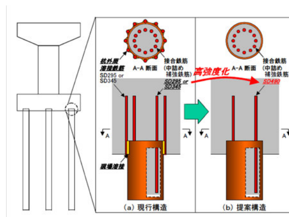
図-6.3 杭頭結合部の構造細目に関する提案
