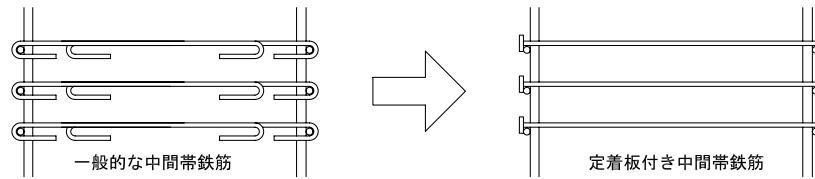
図-2.6 定着体付き鉄筋による中間帯鉄筋の形状変更
