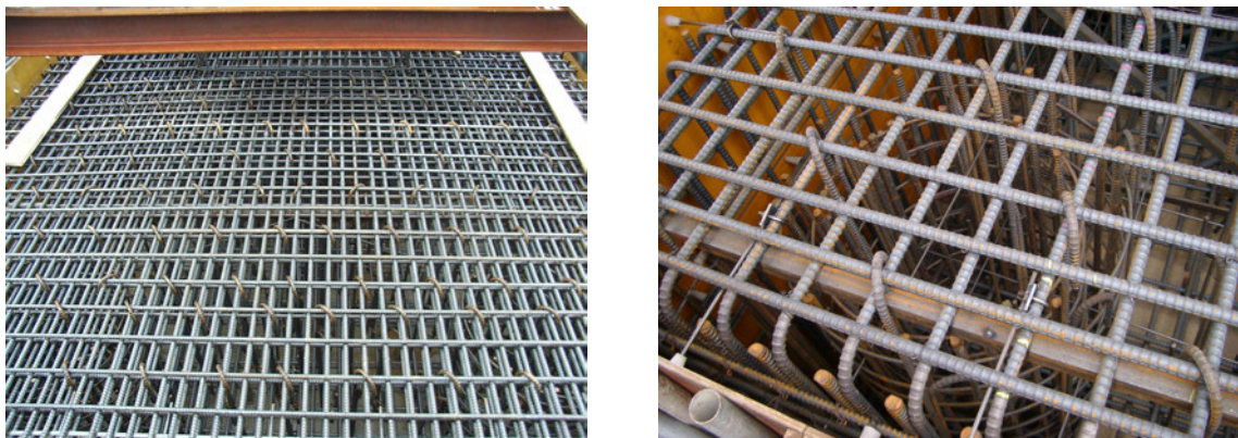
写真-2.3 フーチングのスターラップ配置状況
