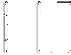
図-2.1 施工承諾によるスターラップ形状の変更 図-2.2 フーチングの主なスターラップ形状
