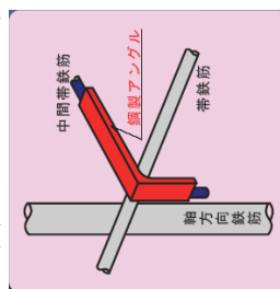
(d) 鋼製アングル式定着
