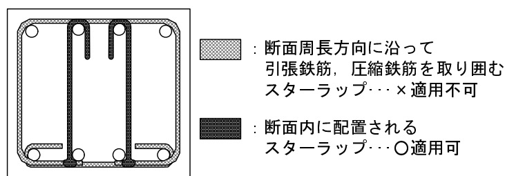
図-3.13 定着体付き鉄筋のはりのスターラップへの適否
