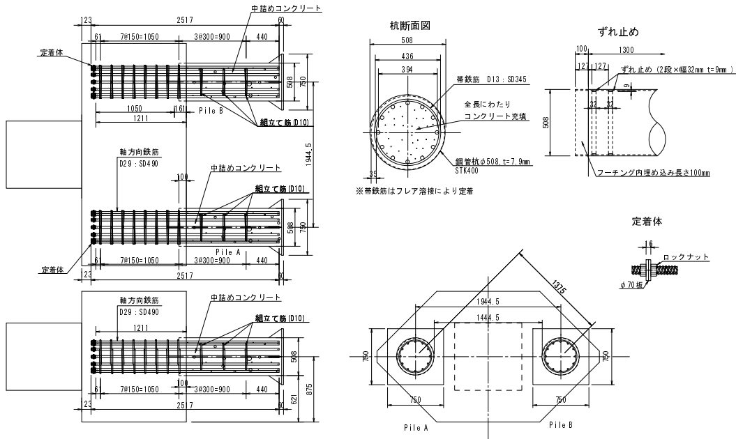
図-5.12 実験供試体配筋図 (Case F)
