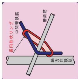
(a) リング式定着
