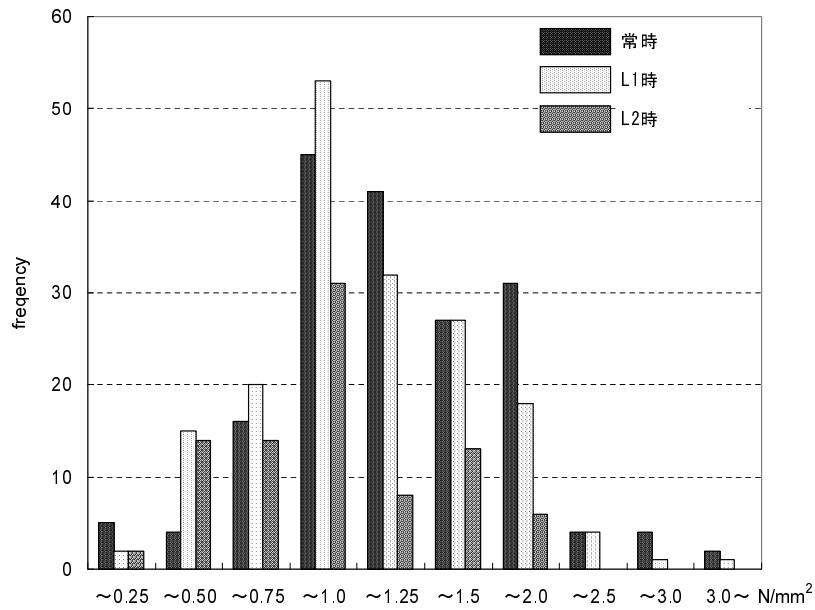
図-3.2 橋脚の設計で考慮される軸力状態 (土研資料 4037 号 13) の調査データより)
