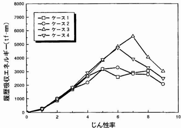
図-3.8 各供試体の履歴吸収エネルギーとじん性率の関係 14)
