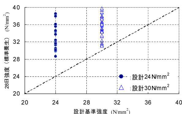
図-5.17 設計基準強度と 28 日強度の関係
