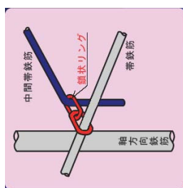
(b) 鎖状リング式定着
