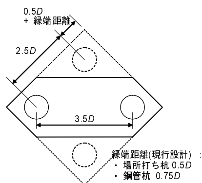
図-5.2 供試体のイメージ図
