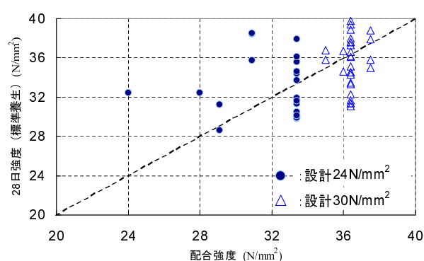
図-5.18 配合強度と 28 日強度の関係
