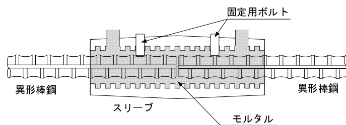
図-4.2 モルタル充てん継手の例 (模式図)
