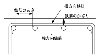
図-5.1 試算対象の部材断面図
