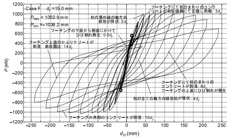
図-5.14 Case F：荷重変位関係
