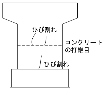
図-2.8 橋脚柱におけるひび割れ発生箇所の例
