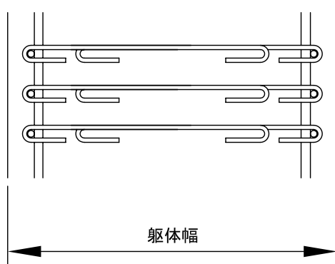
図-2.3 柱及び壁部の中間帯鉄筋の配置
