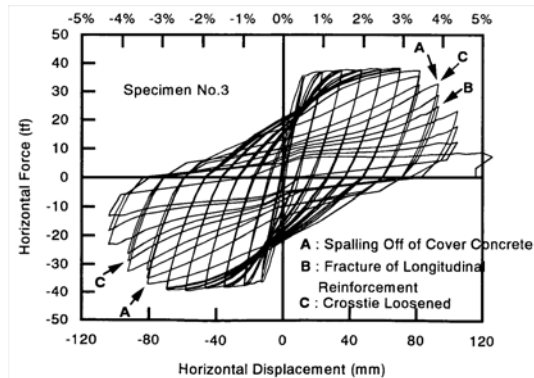
図-3.5 ケース 3 の水平荷重-変位関係 14)
