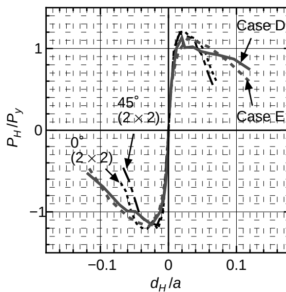
図-5.11 荷重-変形角関係の包絡線の比較 (Case D, E, 0°, 45°)
