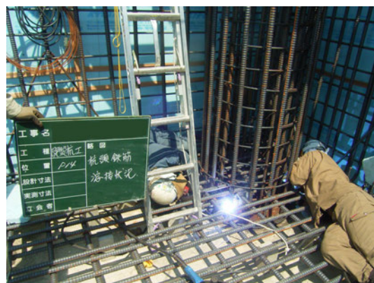
写真-2.1 杭頭補強鉄筋とフーチング鉄筋の干渉 写真-2.2 溶接による杭頭外周鉄筋の施工状況
