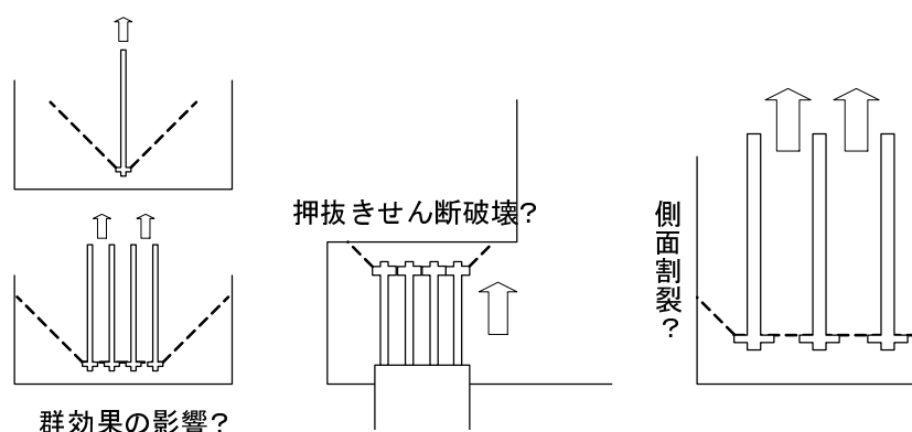
図-3.10 軸方向鉄筋端部への定着体の適用で想定される破壊形態
