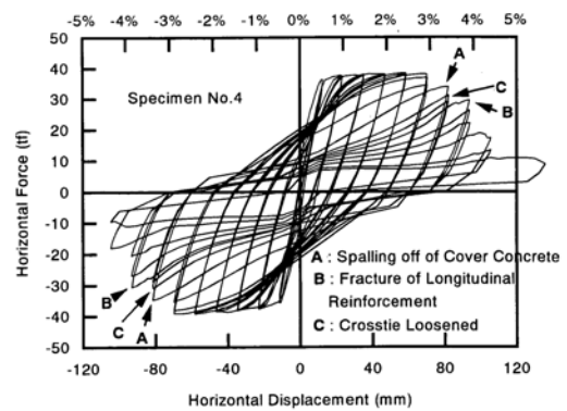
図-3.6 ケース 4 の水平荷重-変位関係 14)
