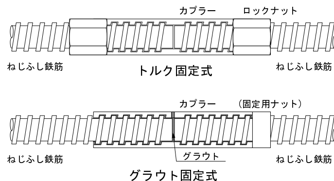
図-4.3 ねじ節鉄筋継手の例 (模式図)
