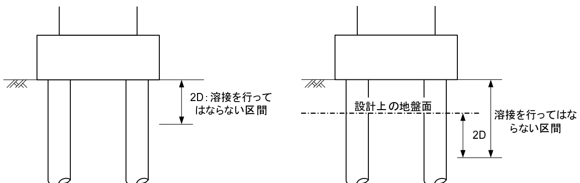
図-6.1 場所打ち杭の軸方向鉄筋に溶接を行ってはならない区間
