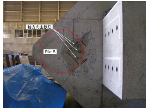
写真-5.3 Case D：試験終了時のフーチング上面の損傷状況
