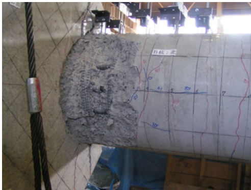
写真-5.2 Case D：試験終了時の杭体の損傷状況
