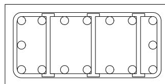
適用例 2 壁・柱の中間帯鉄筋への適用
