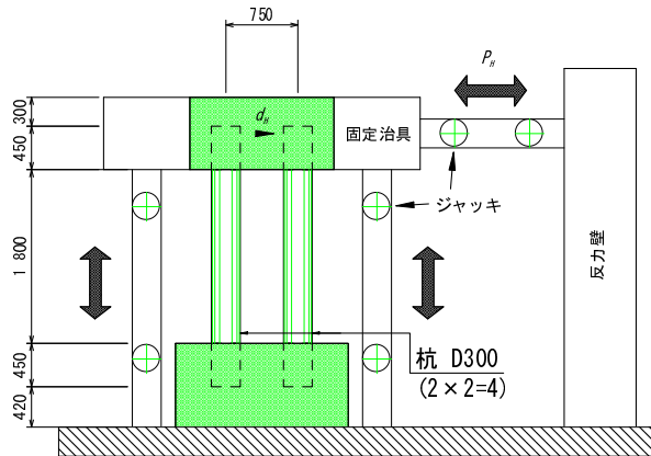
図-5.8 Case 0 ° 載荷試験概略図
