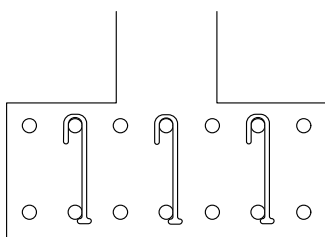
適用例 1 フーチングスターラップへの適用
