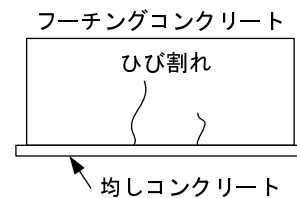
図-2.9 フーチング側面におけるひび割れ発生箇所の例
