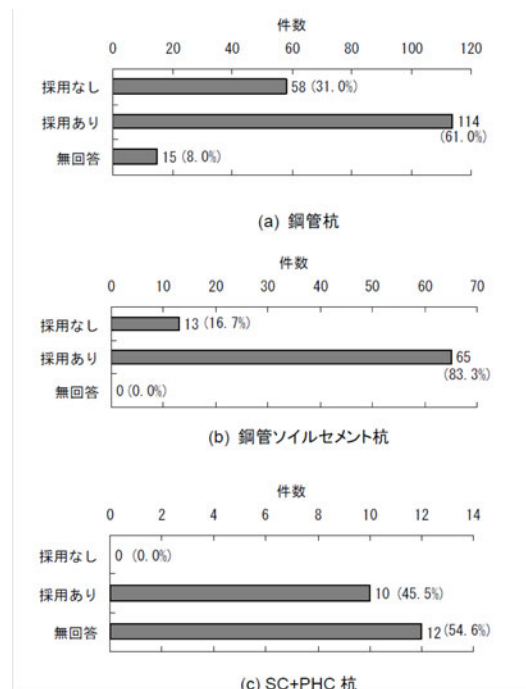
図-6.2 杭外周溶接の採用の有無 13)
