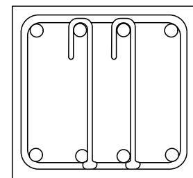
適用例 3 はりのスターラップへの適用
