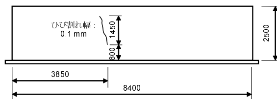
図-5.19 近畿 A：P6(30) のひび割れスケッチ
