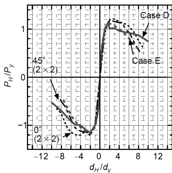
図-5.10 荷重-変位関係の包絡線の比較 (Case D, E, 0°, 45°)
