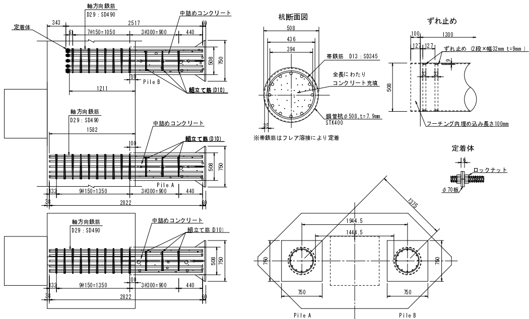
図-5.13 実験供試体配筋図 (Case G)
