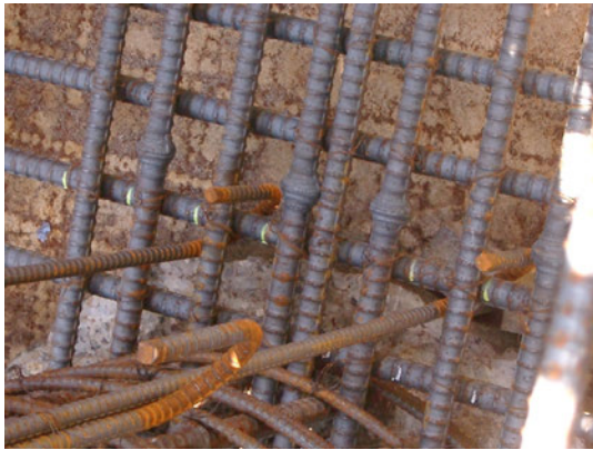
写真-2.9 ガス圧接継手の施工例
