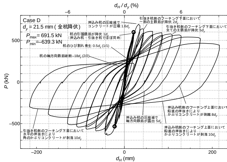
図-5.6 Case D：荷重変位関係
