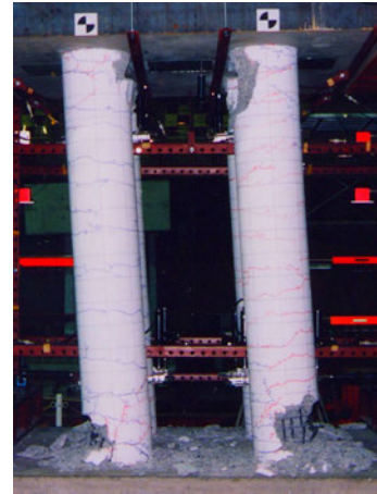
写真-5.5 Case 0 ° 載荷試験実施状況
