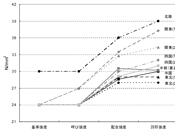
図-2.7 フーチングコンクリートの設計基準強度と施工時のコンクリート強度の関係
