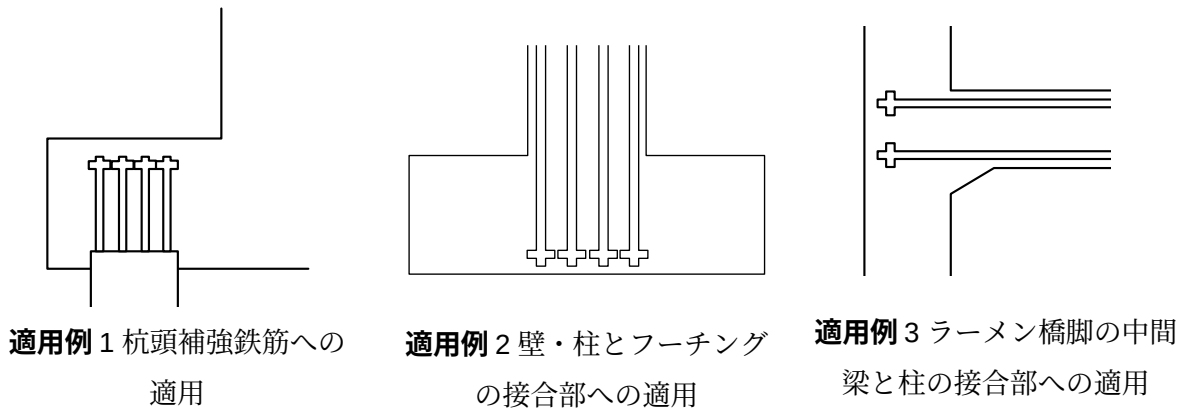
図-3.12 定着体付き鉄筋の軸方向鉄筋への適用例
