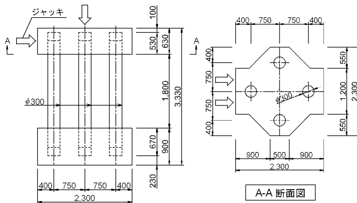
図-5.9 Case 45 ° 載荷試験概略図
