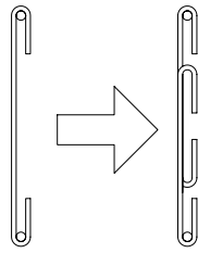
図-2.1 施工承諾によるスターラップ形状の変更 図-2.2 フーチングの主なスターラップ形状
