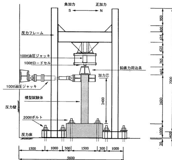
図-3.3 鉄筋コンクリート橋脚柱の正負交番載荷実験概要図 14)
