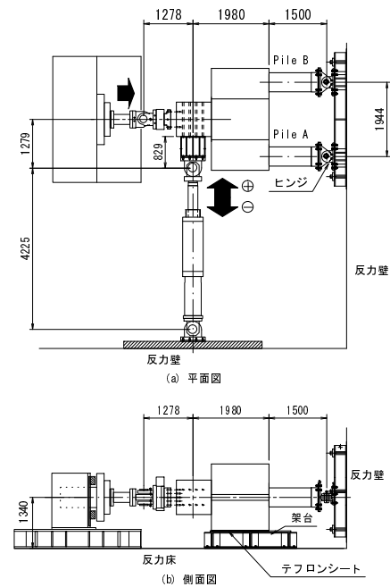
図-5.5 荷重試験概要図
