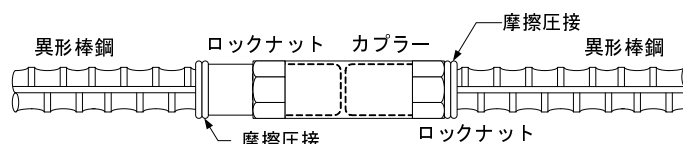
図-4.5 摩擦圧接ねじ継手の例 (模式図)
