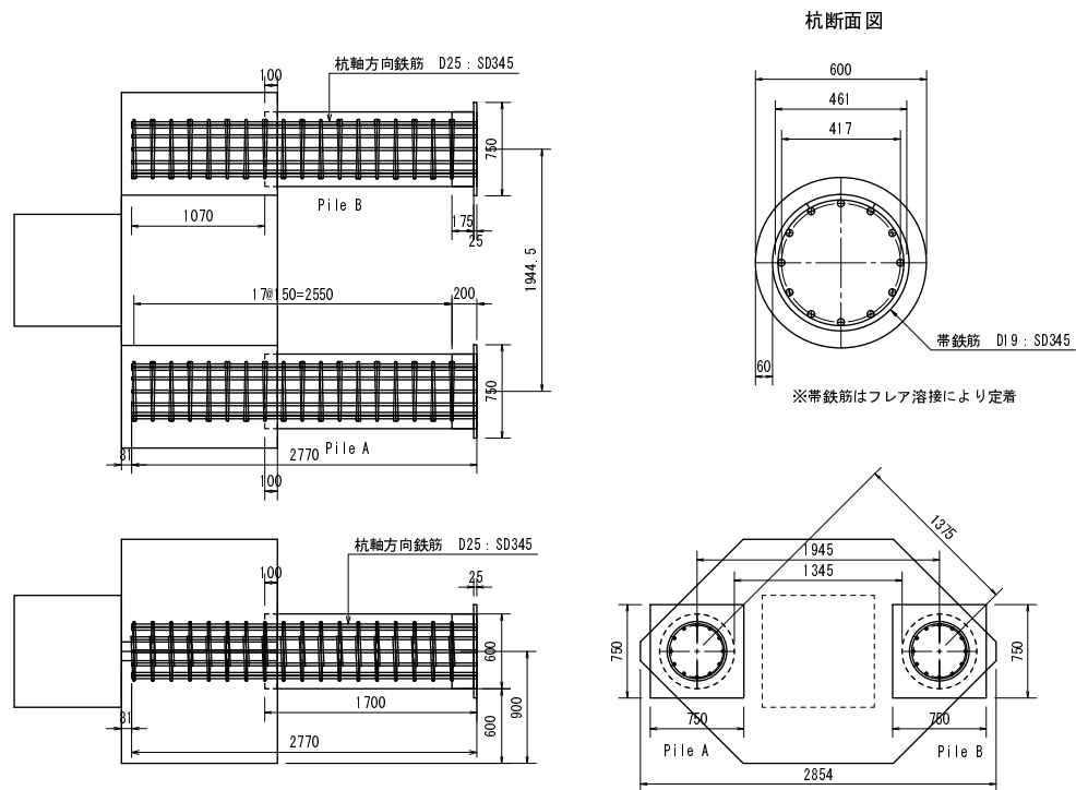
図-5.3 実験供試体配筋図 (Case D)
