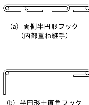
図-2.4 柱及び壁部の中間帯鉄筋形状
