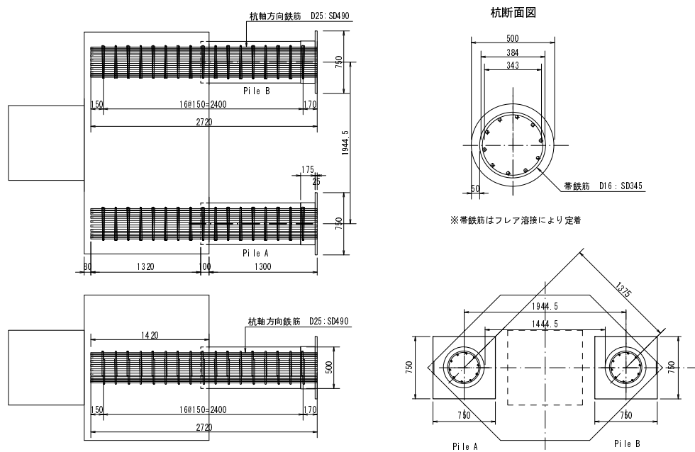
図-5.4 実験供試体配筋図 (Case E)
