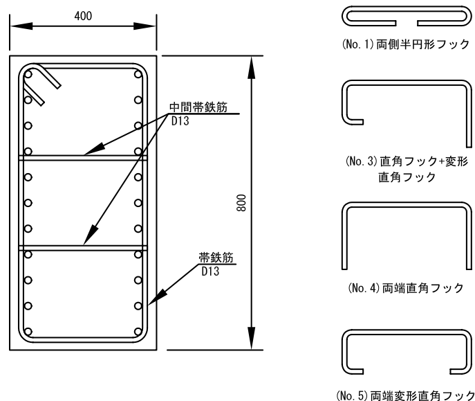
図-3.9 供試体の柱部断面と中間帯鉄筋形状 12)
