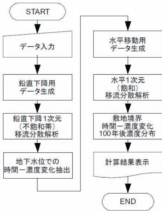
図-5.11 1DTRANSUの計算手順
