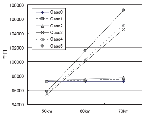
図-3.10 スラグの輸送距離による環境負荷
