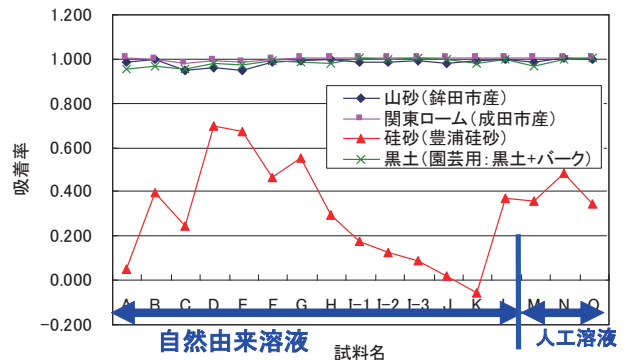
図-5.3 各吸着土におけるヒ素吸着率
