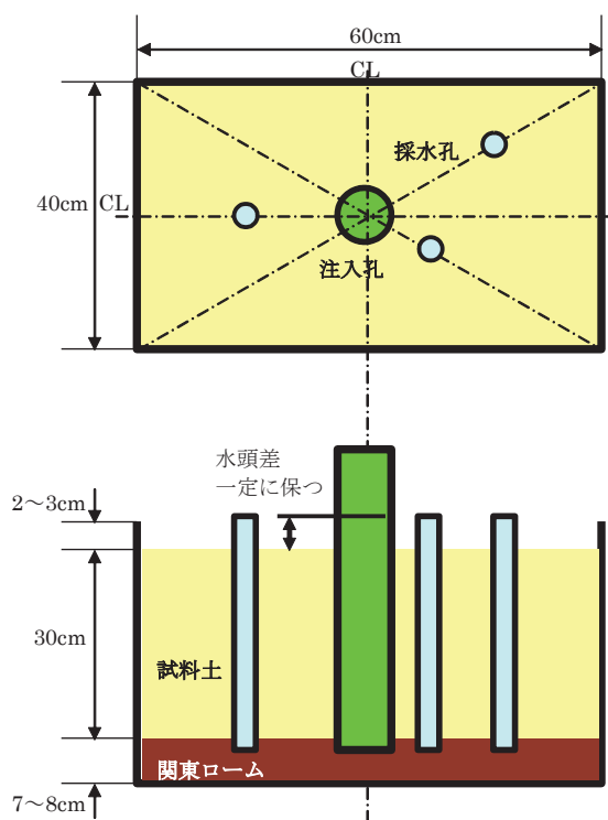
図-5.15 模型地盤
