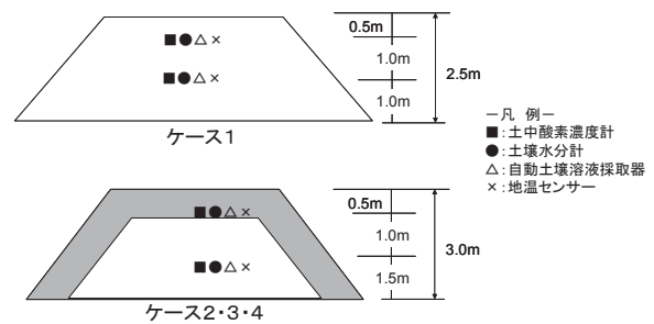
図-7.16 計測機器の設置位置
