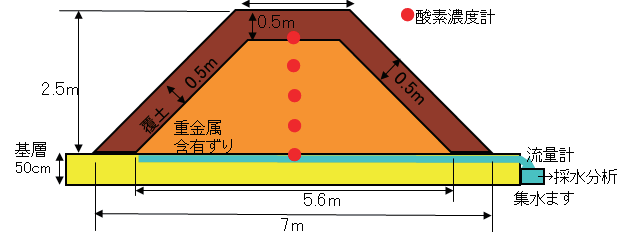
図-6.11 試験盛土の構造図
