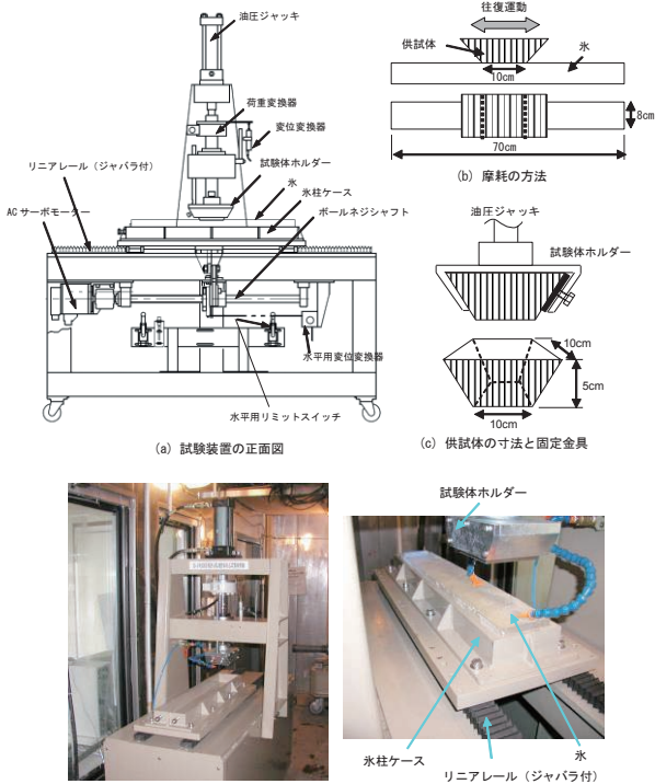
図-3.31 滑動式摩耗試験機の概要図
