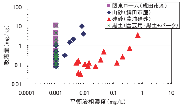
図-5.2 各吸着土におけるバッチ吸着曲線
