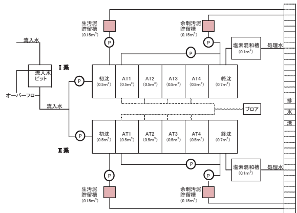
図-3.7 実験装置(概要)
