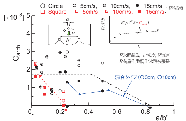
図-3.14 a/b' をパラメータとした場合のアイスアーチング形成状態 (複数の同一実験についてはそれらの平均値) [黒は○型氷群、赤は□型氷群を表す]
