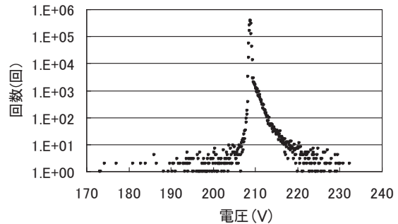
図-5.11 実験期間中に観測された全電圧の頻度分
