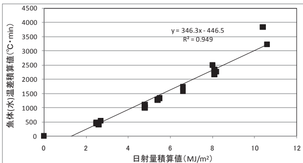
図-2.29 日射量積算値と魚体温差の関係
