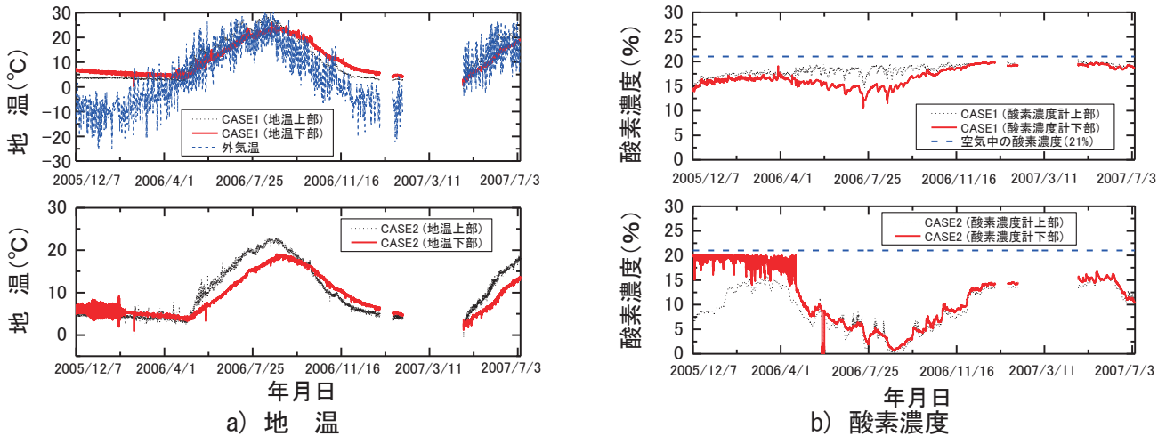
図-7.17 観測機器の計測結果例 (ケース1・2)
