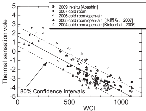
図-2.7 温冷感(T.S.V)と温熱指標値(WCI)との関係および過去の実験結果(Kioka et al., 2006 5) 、木岡ら、2007 7) との比較例(同一温熱環境下での全被験者平均をプロット)
