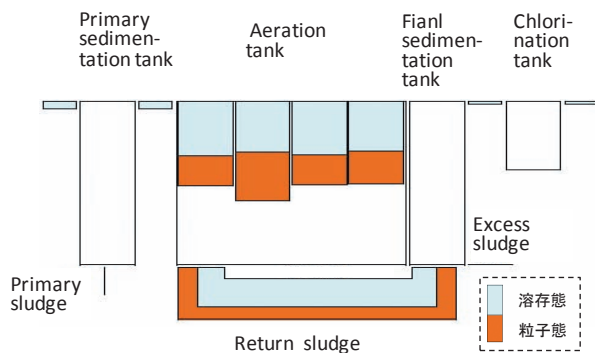
図-3.14 レボフロキサシンの処理プロセスにおける物質フロー
