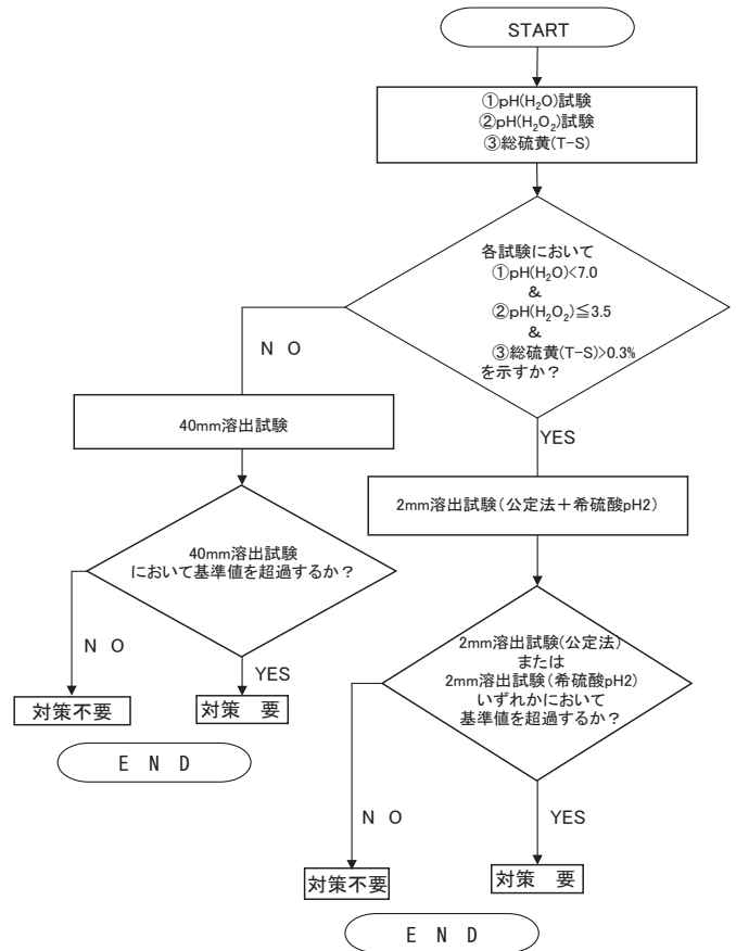
図-7.8 長期リスクを考慮した重金属溶出量評価フロー（素案）
