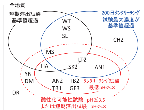
図-6.10 長期溶出試験と各種促進溶出試験結果の関係(2) タンクリーチング試験
