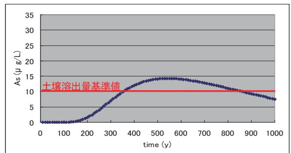
(2) 購入土
