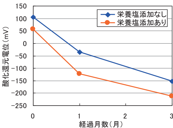
図-5.12 酸化還元電位(ORP)の経日変化
