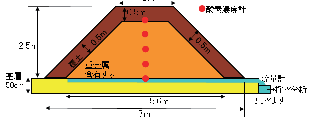
図-6.11 試験盛土の構造図
