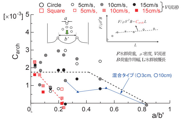
図-3.14 a/b' をパラメータとした場合のアイスアーチング形成状態 (複数の同一実験についてはそれらの平均値) [黒はO型氷群、赤は□型氷群を表す]
