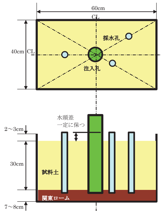
図-5.15 模型地盤
