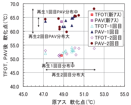
図-4.15 劣化と再生を繰り返したアスファルトの軟化点
