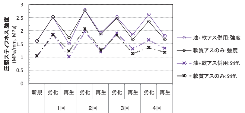
図-4.26 繰り返し再生による圧裂スティフネスの変化
