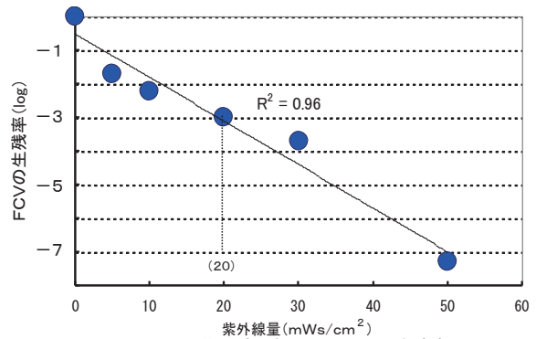
図-4.15 紫外線照射によるFCVの生残率
