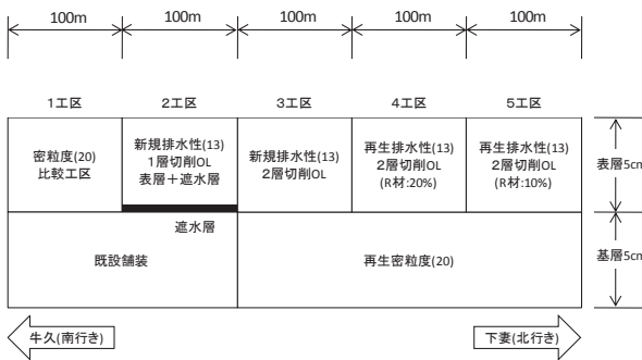
図-4.32 試験施工で評価した混合物/構造の種類(R408)
