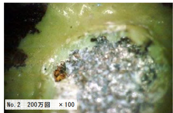
写真-資 6.18 位置損傷状況 (B018 試験体)
