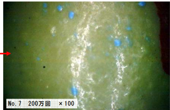
写真-資 6. 23 No. 7 位置損傷状況 (B018 試験体)
