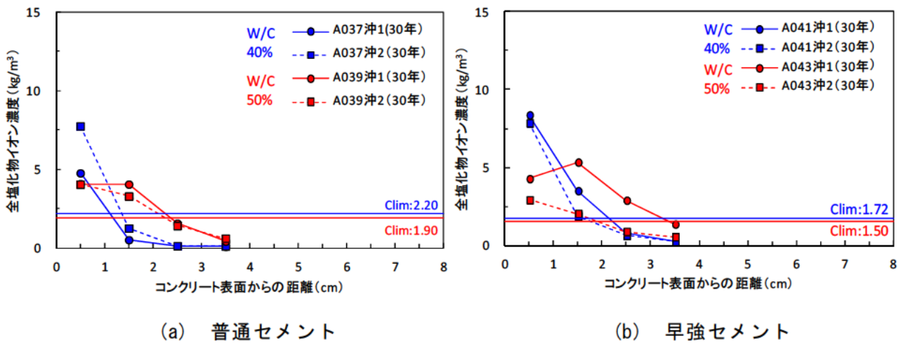
図-4.4.1 水セメント比の影響
