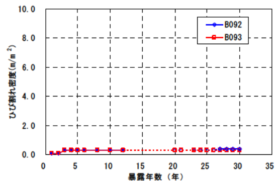
(b) ひび割れ密度
