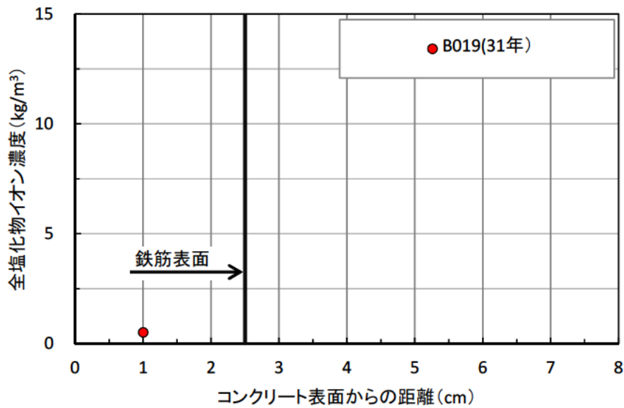
図-資 4.30 B019試験体の塩化物イオン濃度
