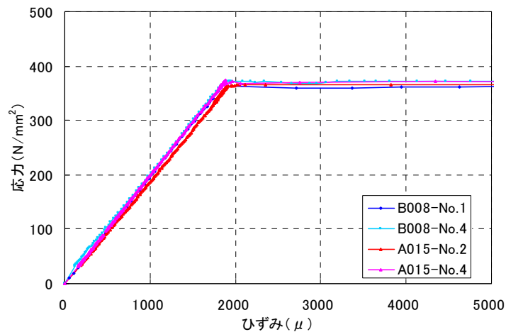
図-4.9.3 鉄筋の引張試験における荷重ひずみ関係
