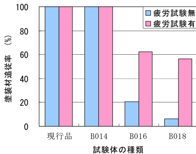
図-4.8.4 塗装材追従率
