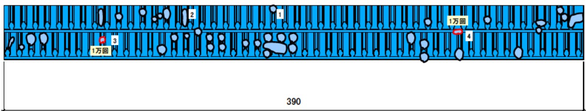
図-資 6.4 損傷状況 (B014 試験体)
