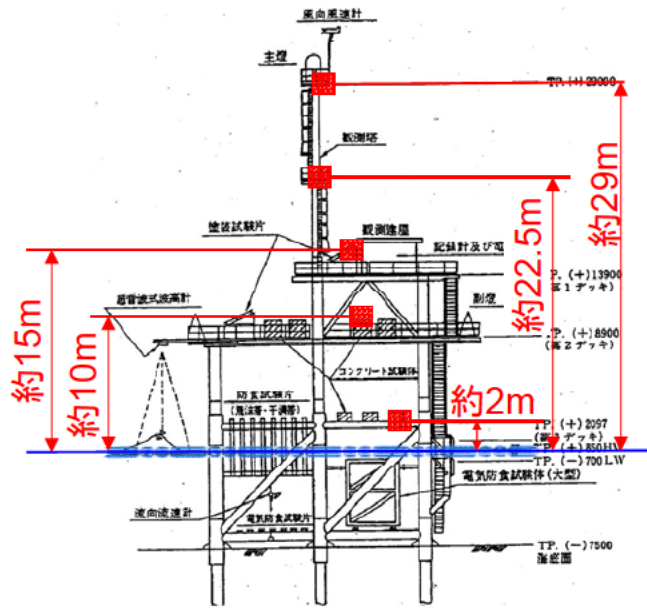
図-3.2.4 調査機器および供試体の海面からの設置高さ
