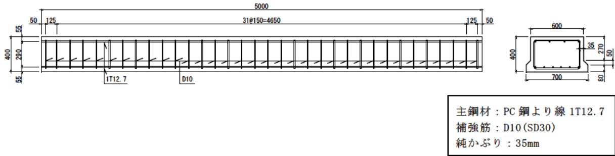
図-2.2.8 試験体形状（プレテンション方式大型試験体 スラブ型）
