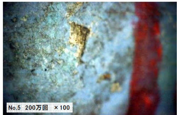
写真-資 6.13 No. 5 位置損傷状況 (B016 試験体)
