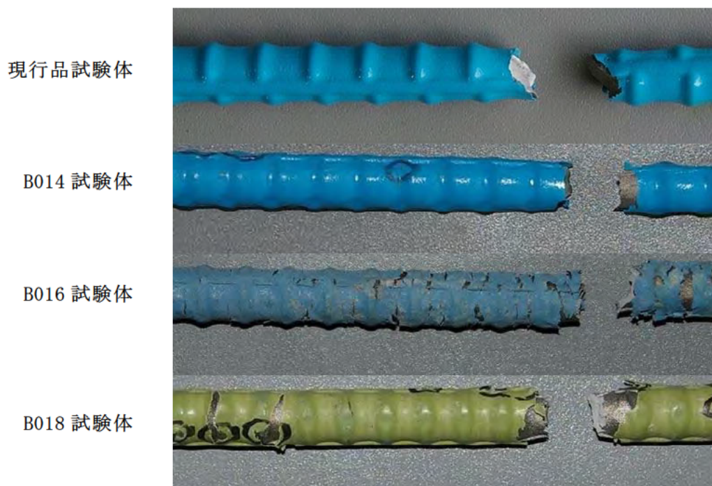
写真-4.8.2 破断状況
