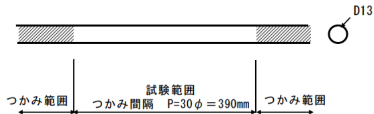
図-資 6.2 試験片寸法
