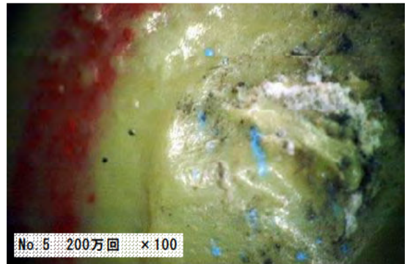
写真-資 6. 21 No. 5 位置損傷状況 (B018 試験体)
