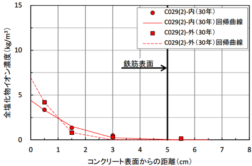
図-資 4.27 C029試験体の塩化物イオン濃度（暴露30年）
