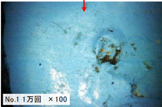
写真-資 6.4 No. 1 位置損傷状況
