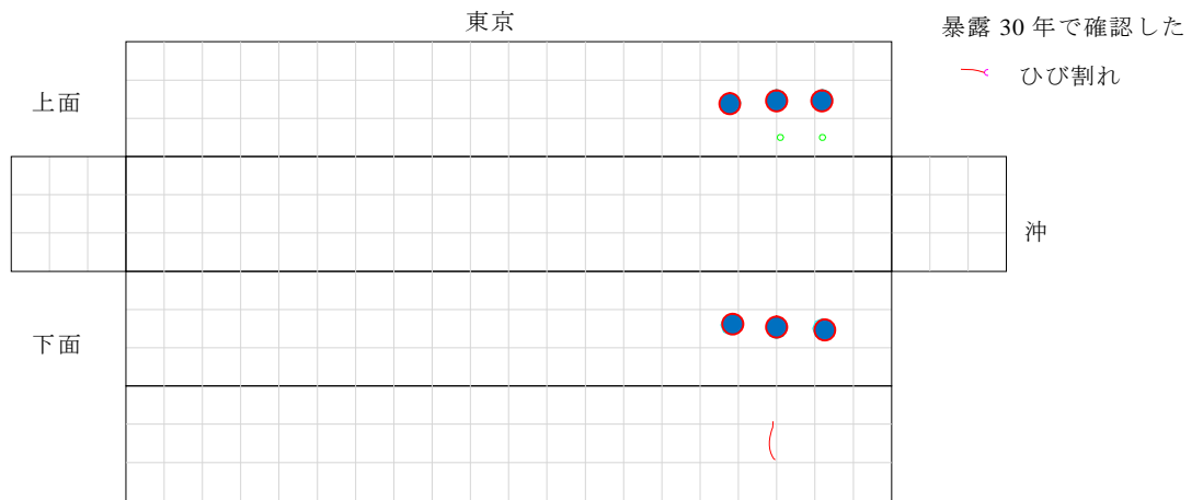
図-資 3.8 A043 供試体
