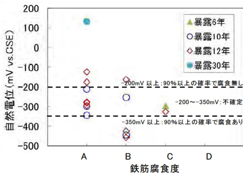
図-4.5.5 自然電位と鉄筋腐食度の関係
