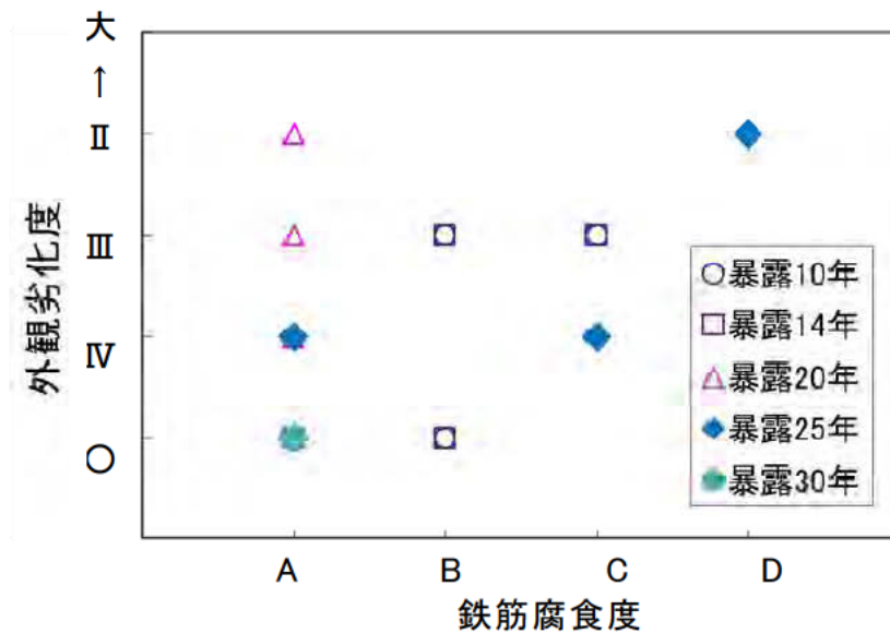
図-4.5.4 外観劣化度と鉄筋腐食度の関係
