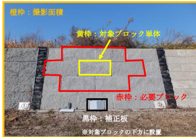
急傾斜用護岸ブロック
