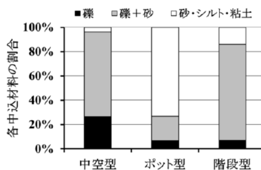
図-6.35 開口部の形状別に見た中込材料の適用割合
