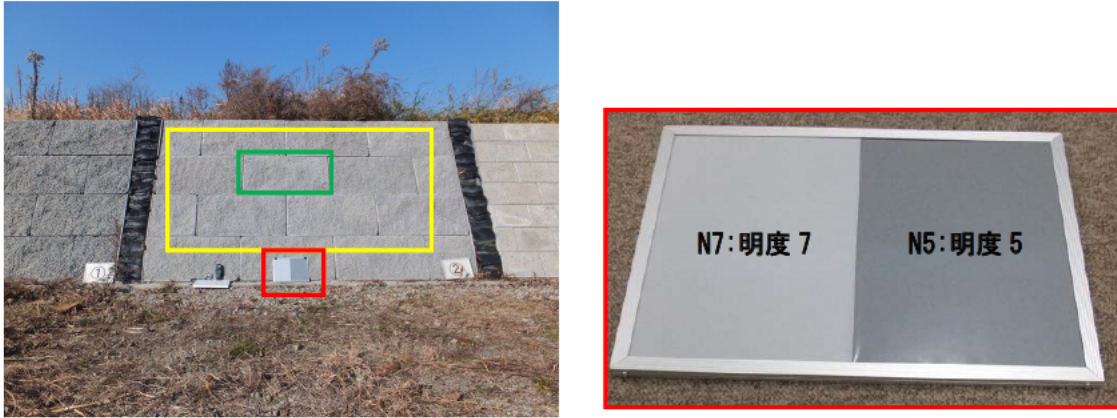
図-3.22 明度測定時の写真撮影例と補正板
