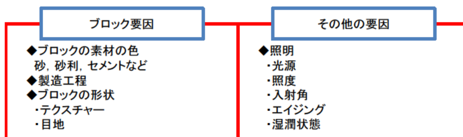
図-3.17 護岸ブロックの明度の決定要因
