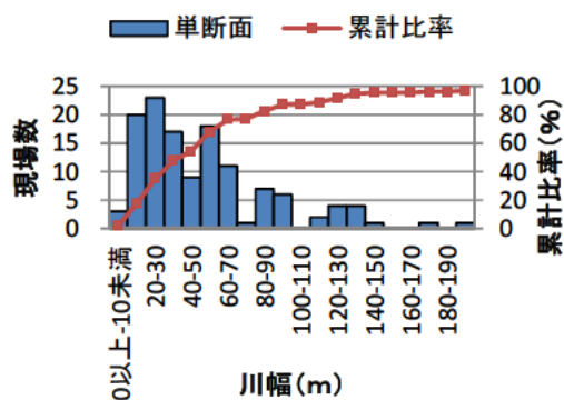
図-3.15 単断面の川幅
