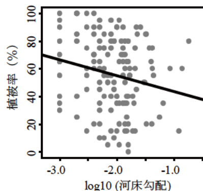
図-6.31 河床勾配と植被率との関係
