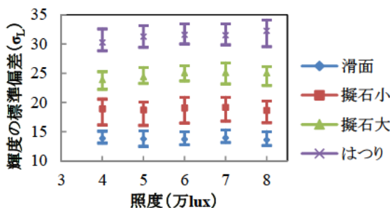
図-6.12 機種ごとの \sigma_L のばらつき（ \theta=45[°] ）
