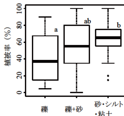
図-6.32 中込材料別にみた植被率
