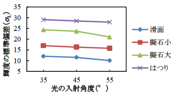
図-6.10 光の入射角度の影響（カメラ：No3, 80000lux）
