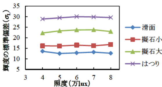
図-6.11 照度の影響（カメラ：No3, \theta=45[°] ）
