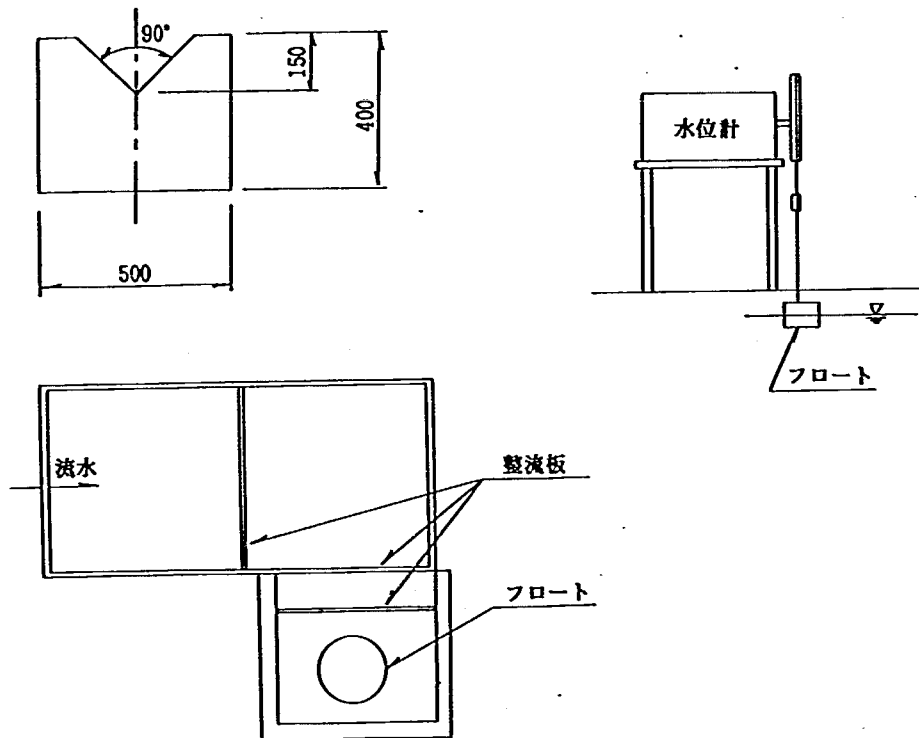
図 2-4 排水量測定図 (単位: mm)
