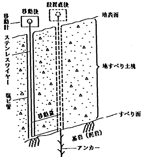
図 2-1 移動計設置図
