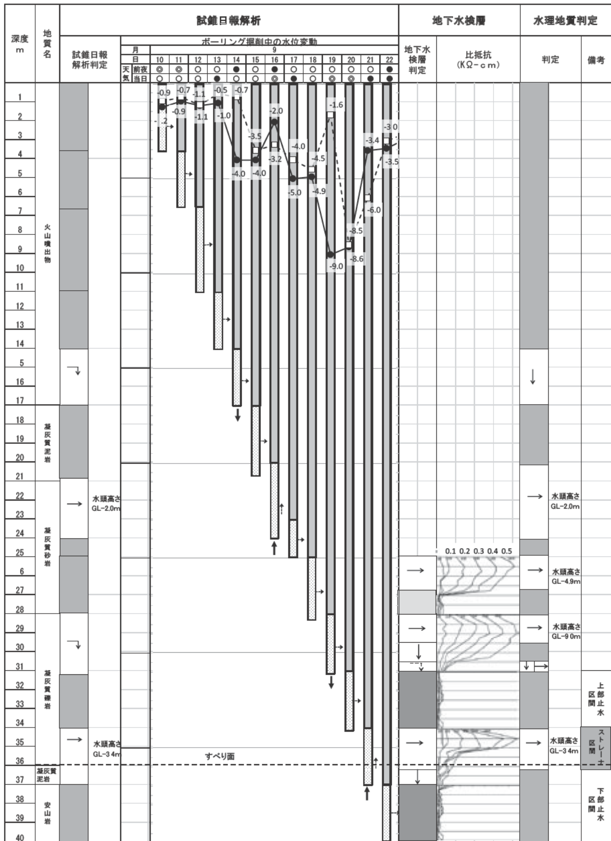
図 2-4 (1) 水理地質総括図
