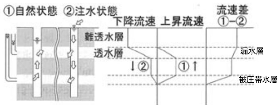
図 解 3-8 孔内微流速測定概念 1) に加筆
