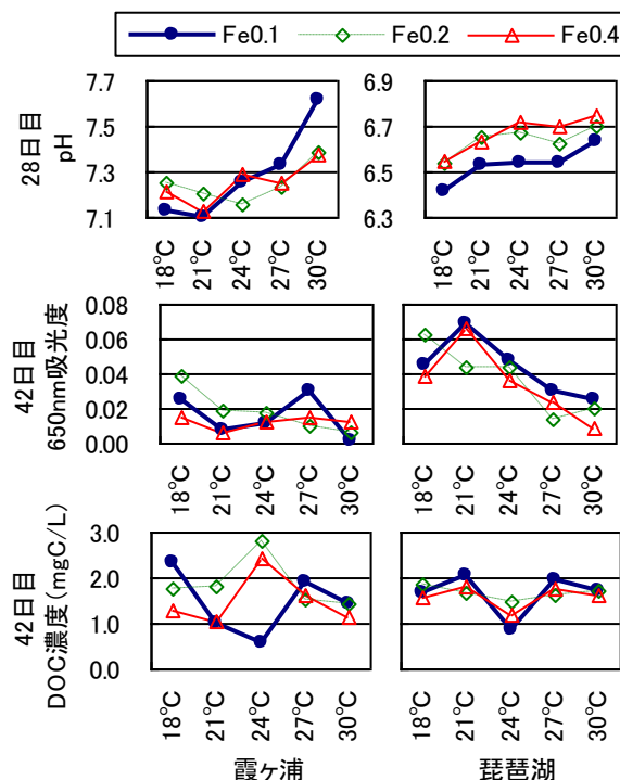
図 3.2-9 水温と、定常期 (14~28, 42 日目) の pH、650nm 吸光度、DOC 濃度の関係
