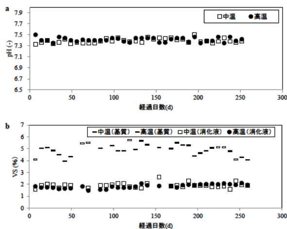
図1 連続式実験における pH(a) および VS(b) の経時変化
