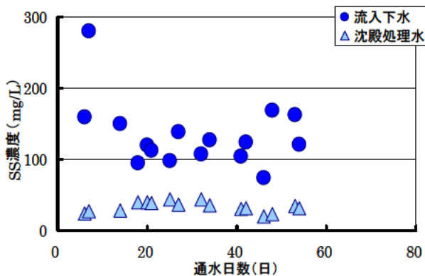
図-3 簡易沈殿処理によるSS濃度の推移
