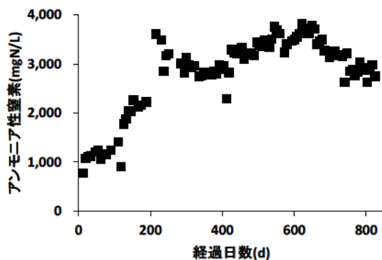
図4 反応器1におけるアンモニア性窒素濃度
