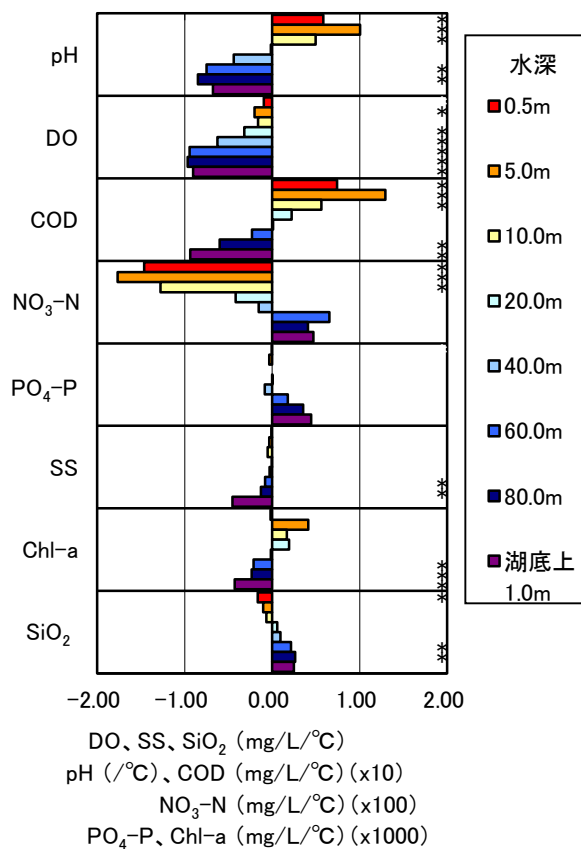
図 2.4-14 各水深における、水温上昇に対する主な水質項目の変化割合
