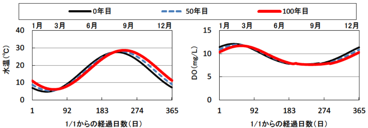
図 4.2-9 水温と DO の 0、50、100 年目の季節変化パターン
