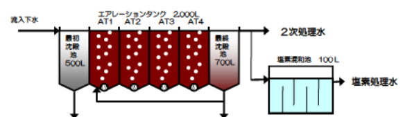
図-1 下水処理装置の概要
