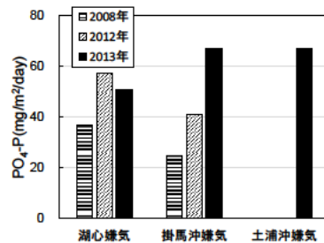
図21 PO 4 -Pの溶出速度
