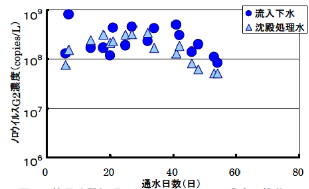
図-2 簡易沈殿処理によるノロウイルスG2濃度の推移
