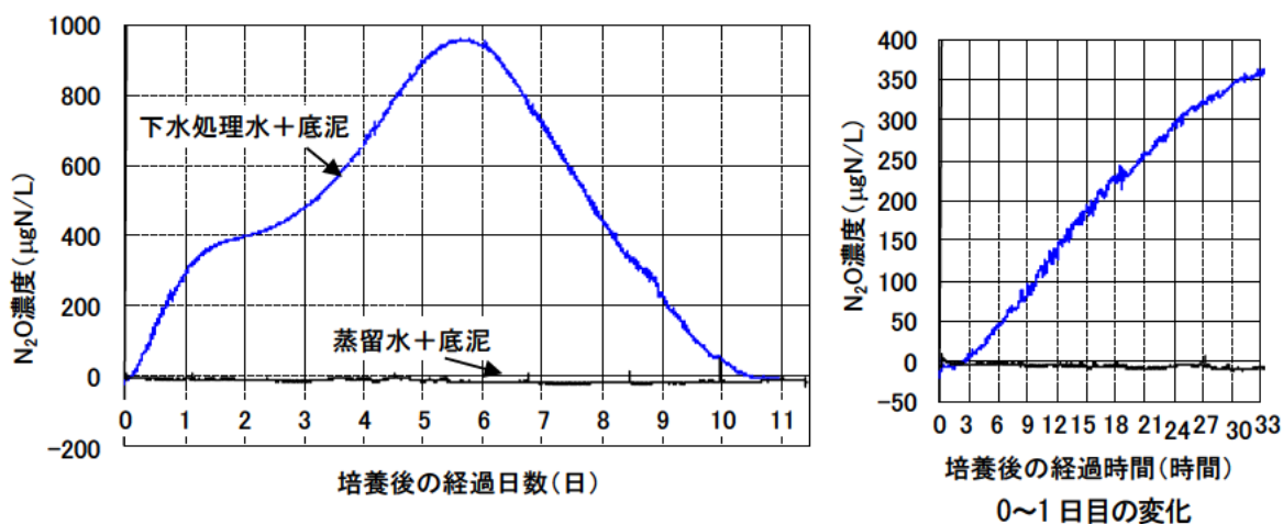
図 14 培養中の溶存 \text{N}_2\text{O} 濃度の変化
