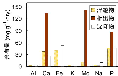
図 2-2 回収物の元素組成
