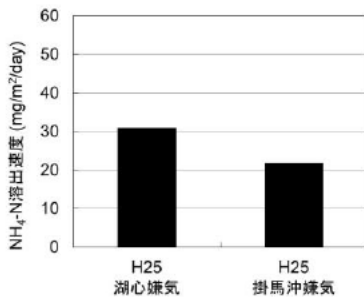
図 14 \text{NH}_4\text{-N} の溶出速度
