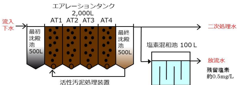
図-4 下水処理実験装置の概要
