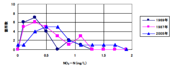
図 2.2-4 河川表流水の NO 3 -N 濃度分布の経年変化
