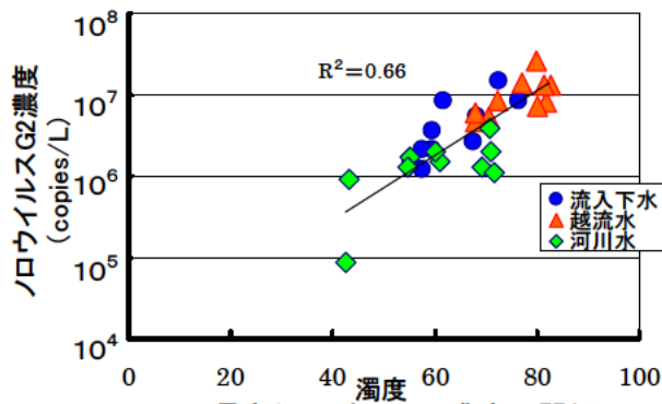
図-11 濁度とノロウイルス濃度の関係
