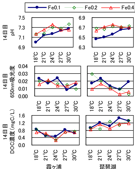
図 3.2-8 水温と、増殖期 (0~14 日目) の pH、650nm 吸光度、DOC 濃度の関係
