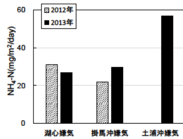
図20 NH 4 -Nの溶出速度
