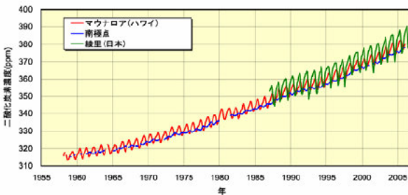
図 1-1 大気中二酸化炭素濃度の変化 2)
