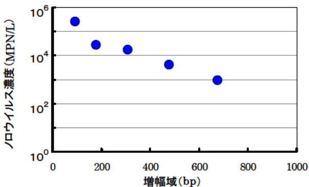
図-2 標的遺伝子の増幅域ごとのノロウイルス検出濃度
