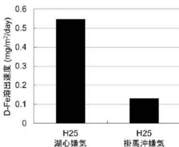
図 15 \text{D-Fe} の溶出速度
