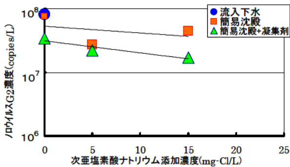
図-6 次亜塩素酸ナトリウム添加濃度に応じた各処理条件でのノロウイルスG2濃度
