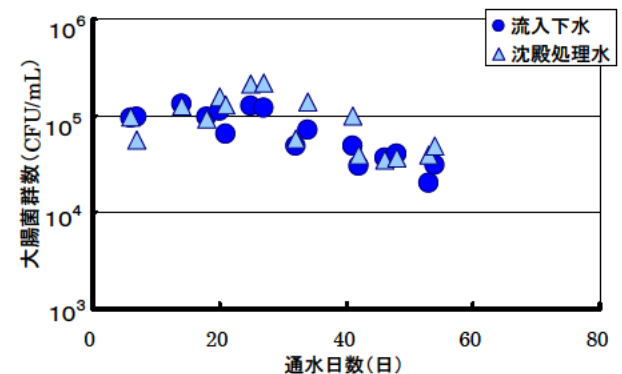
図-1 簡易沈殿処理による大腸菌群数の推移
