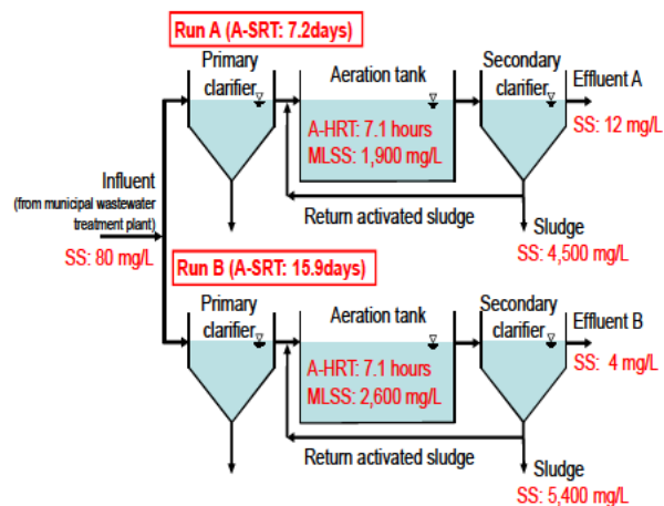
図 3 下水処理プラントの概略図
