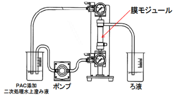
図5 膜ろ過装置
