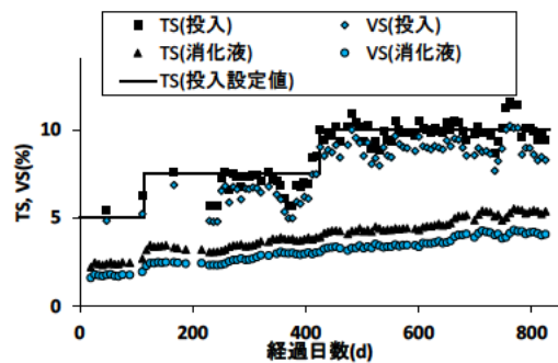
図1 反応器1におけるTSおよびVSの経時変化
