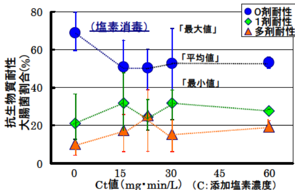
図-12 Ct値と抗生物質耐性大腸菌割合
