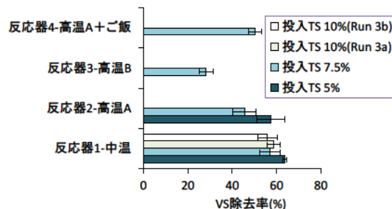
図2 連続実験におけるVS除去率
