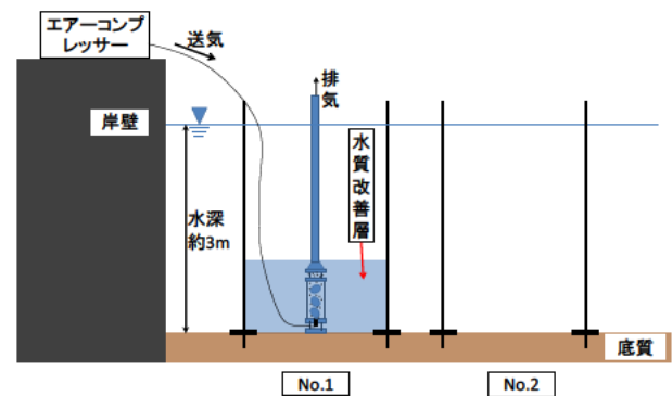
図1 実験概念図
