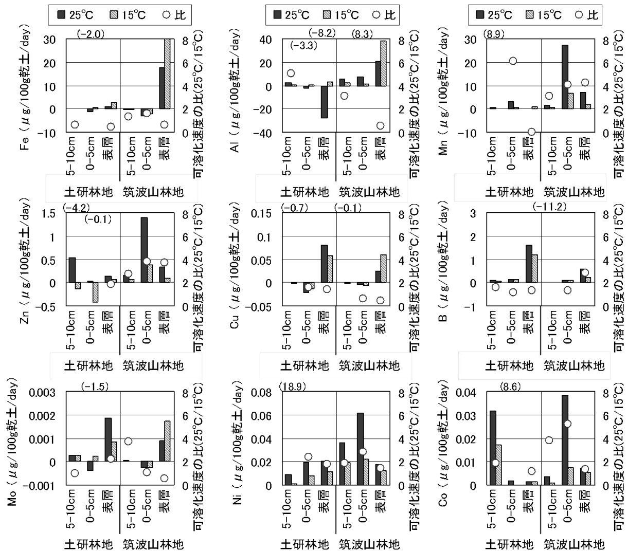
図 3.1-12 25°Cと 15°Cにおける金属の可溶化速度とその比
