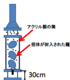
図2 担体処理装置
