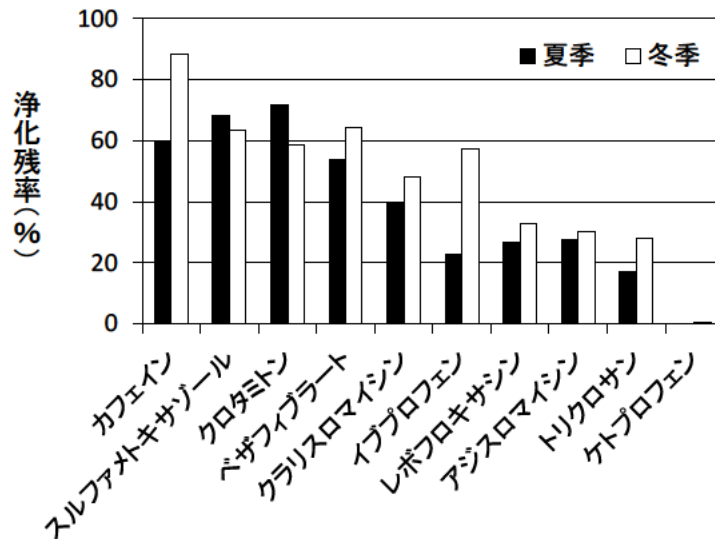
図-3 医薬品類 10 物質の浄化残率
