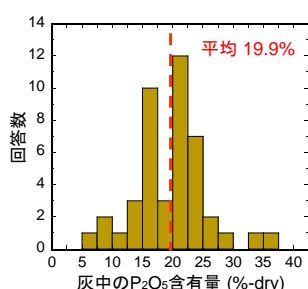
図 5-2 全国の下水汚泥焼却灰中のリン含有量(P 2 O 5 換算値)
