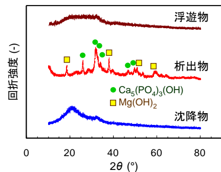
図 2-3 回収物の X 線回折
