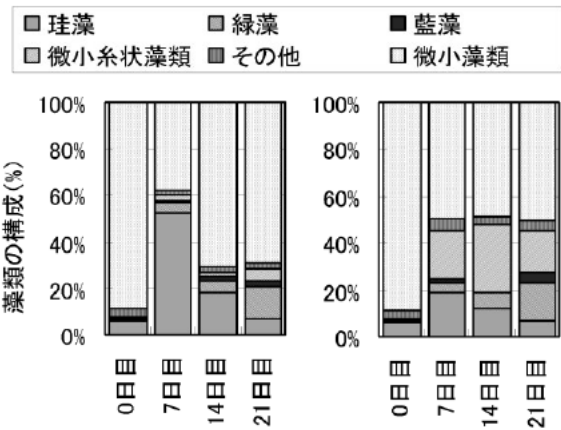
筑波山林地、表層、25°C 筑波山林地、表層、15°C 図 3.1-15 筑波山林地表面層の土壤溶出液で
