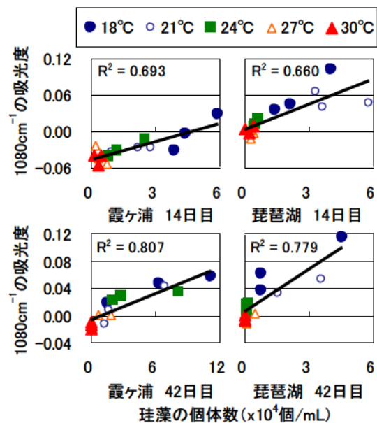
図 3.2-7 珪藻の個体数と 1080 -1 の吸光度の関係
