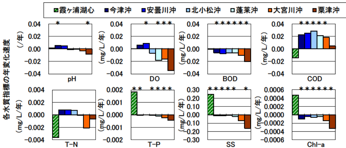
図 2.4-6 霞ヶ浦と琵琶湖の表層における主な水質項目の年平均値の経年変化
