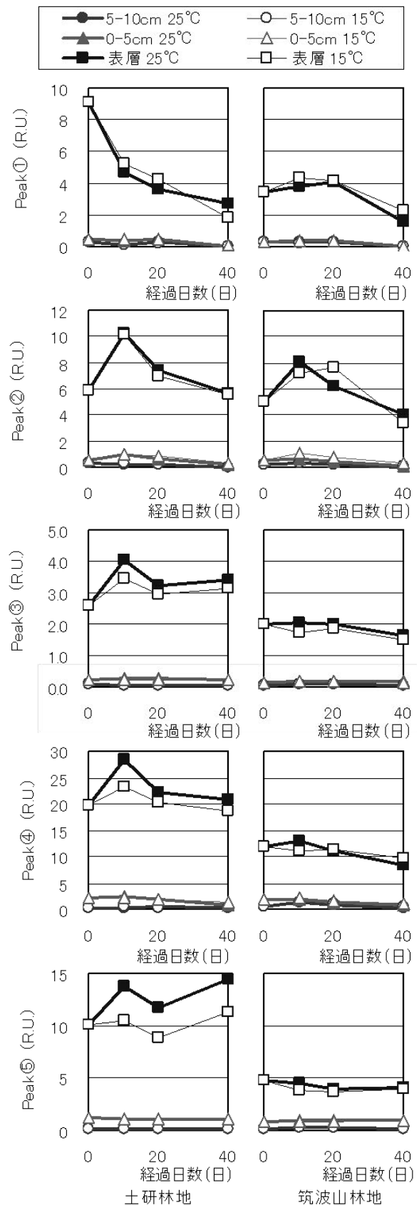
図3.1-8 土壤溶出液のEEMの主なピークの蛍光強度の変化
