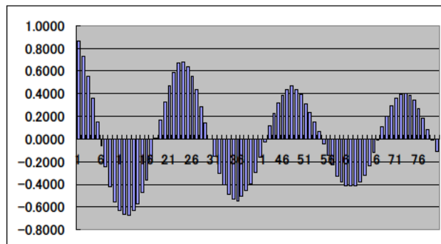
図 2.3-3 瀬田川の 2 箇所 DO とその 24 時間移動平均との差分のコレログラム
