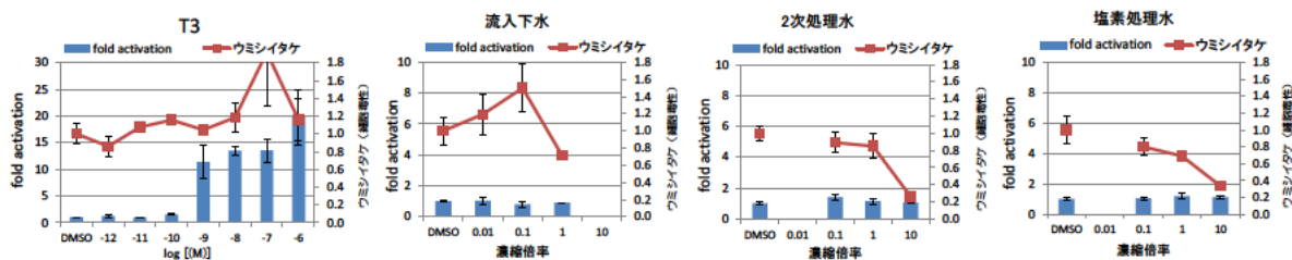
図-6 ヒトメダカ甲状腺ホルモンレセプター \beta を組み込んだレポーター遺伝子アッセイの結果
