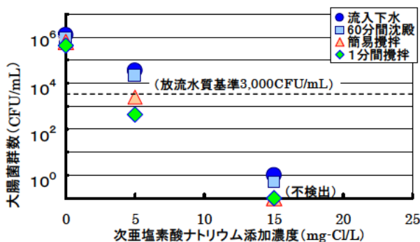
図-8 次亜塩素酸ナトリウム添加濃度に応じたPACの添加・攪拌条件ごとの大腸菌群数
