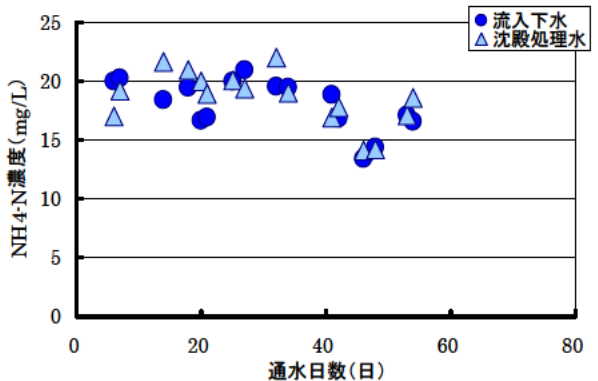
図-5 簡易沈殿処理によるNH 4 -N濃度の推移
