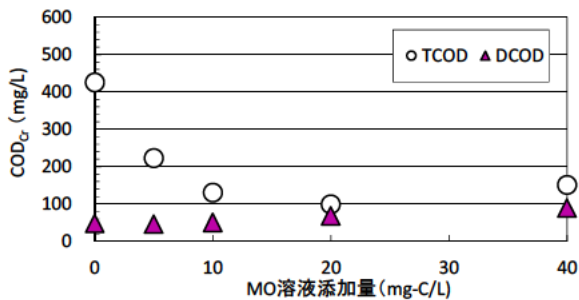
図6 MO溶液(pH調整無し)により凝集沈殿した試料の上澄みのTCODαとDCODα
