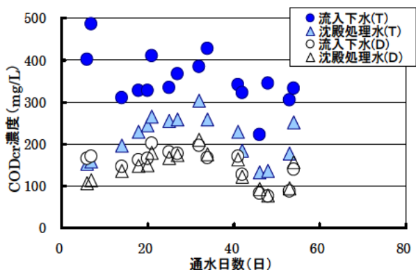
図-4 簡易沈殿処理によるCOD Cr 濃度の推移
