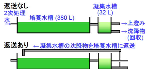
図 3-1 実処理場に設置した藻類培養・回収システムの写真(左側が返送なし、右側が返送ありの系列)およびフロー図
