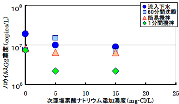
図-7 次亜塩素酸ナトリウム添加濃度に応じたPACの添加・攪拌条件ごとのノロウイルスG2濃度
