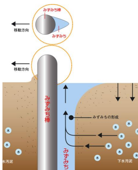
図-1 みずみち棒の効果の模式図
